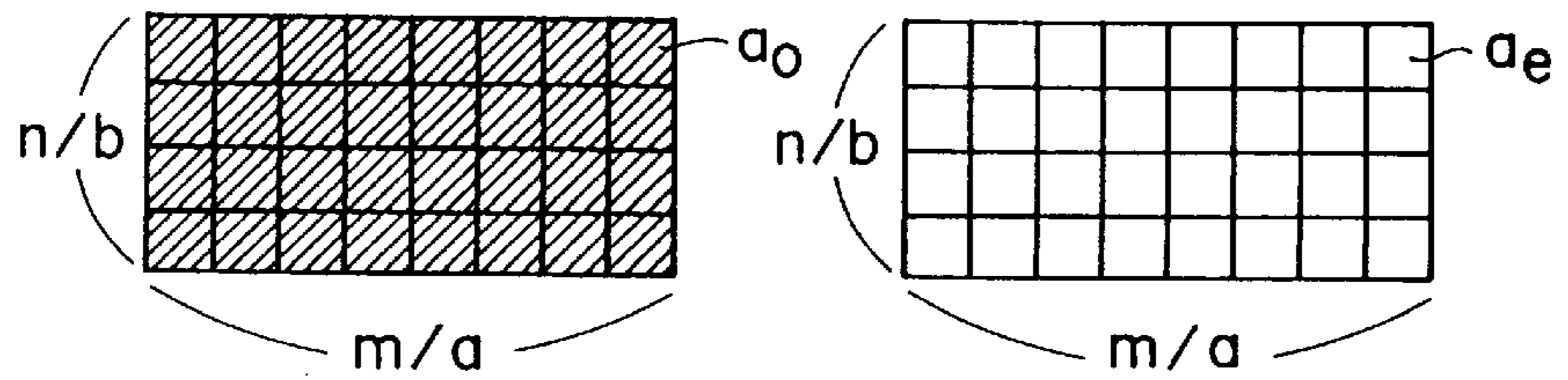
FIG. 5E FRAME MATCHING ELEMENTS
