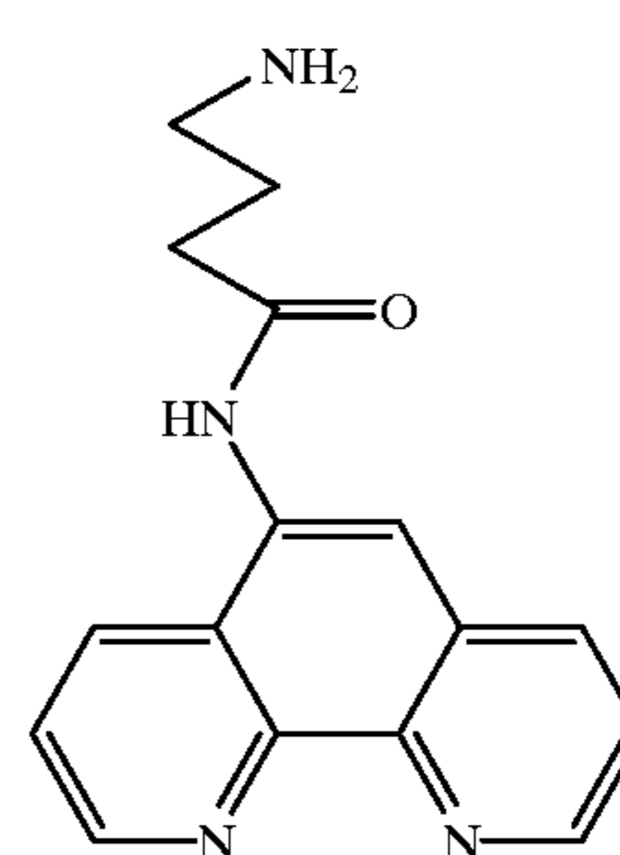
5-(3-aminopropionamido)-1,10-phenanthroline
