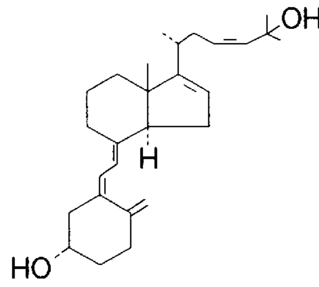
25-(OH)-16,23(Z)- diene-D 3
