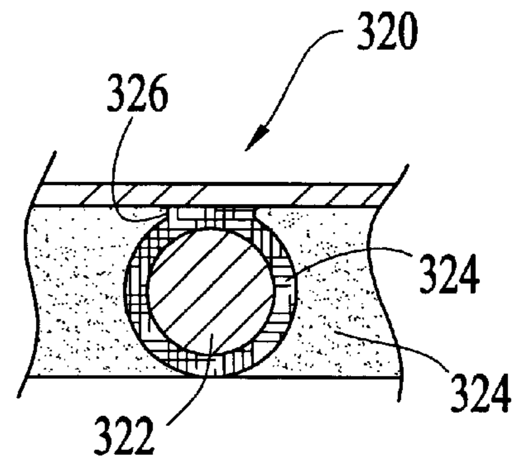
FIG. 18
