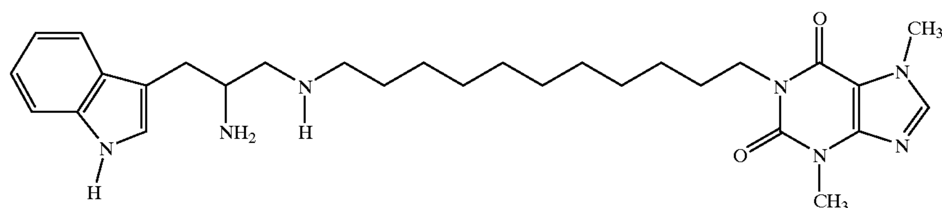
6515 1-(11-(2-amino-3-indolylpropylamino)undecyl)-3,7-dimethylxanthine
