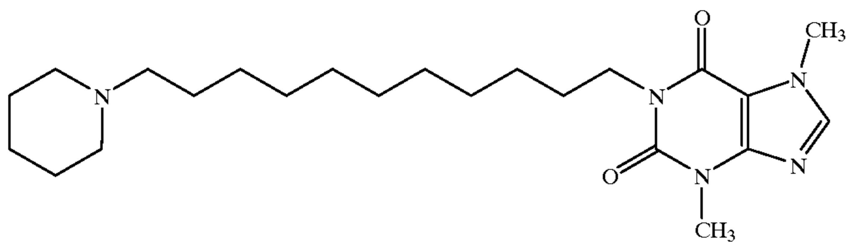
6543 1-[11-(Piperidiny)undecyl]-3,7-dimethylxanthine
