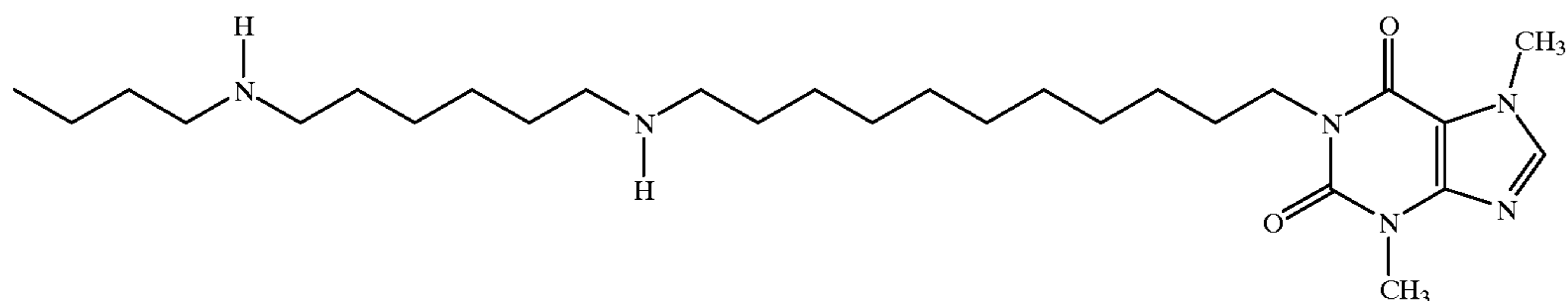
6557 1-(11-[6-Butylaminoethylamino]undecyl)-3,7-dimethylxanthine
