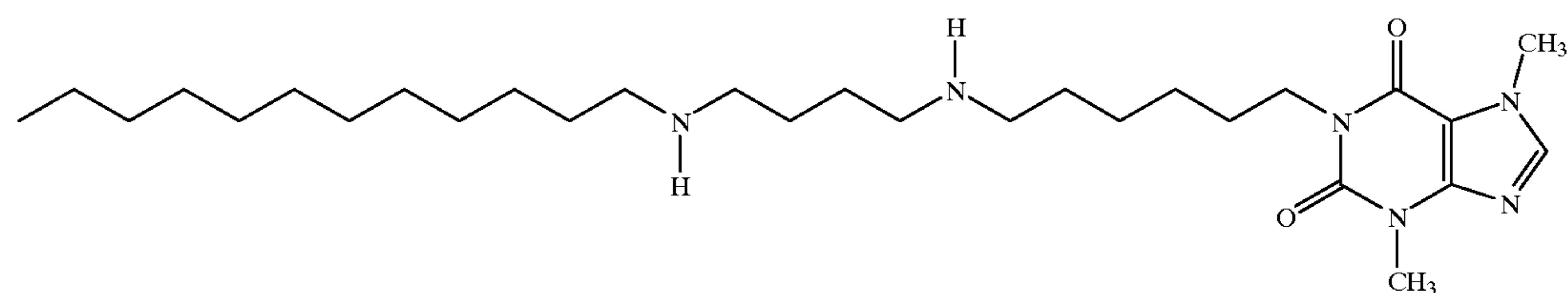
6560 1-(6-[4-Dodecylaminobutylamino]hexyl)-3,7-dimethylxanthine
