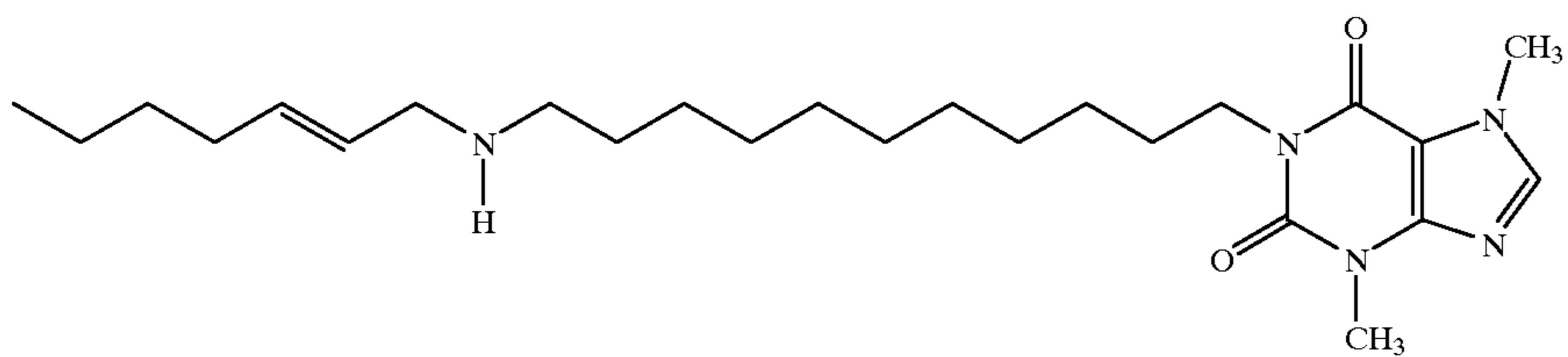
7511 1-[11-[(2-trans-Hepten-1-yl)amino]undecyl]-3,7-dimethylxanthine
