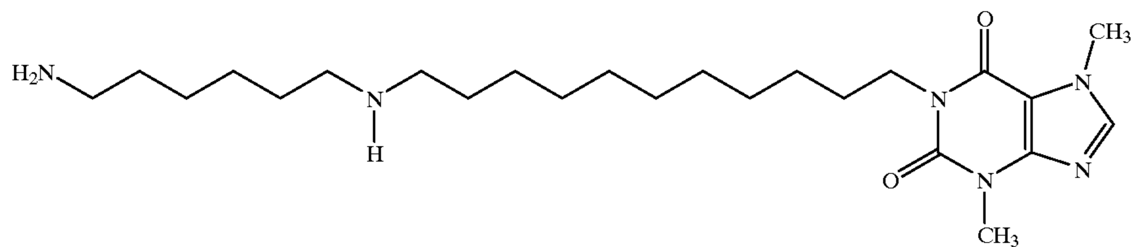
6556 1-(11-[6-Aminohexylamino]undecyl)-3,7-dimethylxanthine
