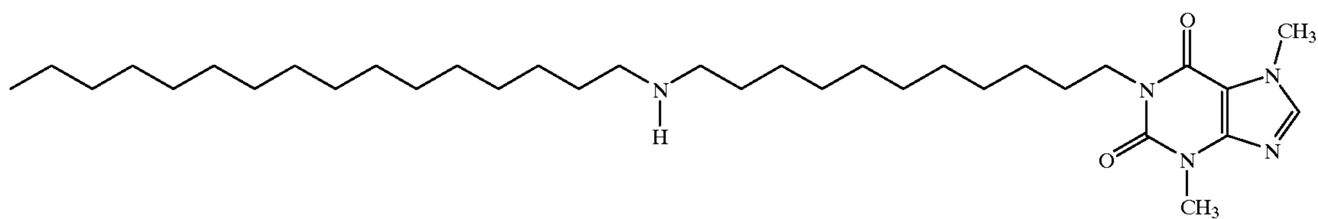
3584 1-(11-Hexadecylamino)undecyl)-3,7-dimethylxanthine
