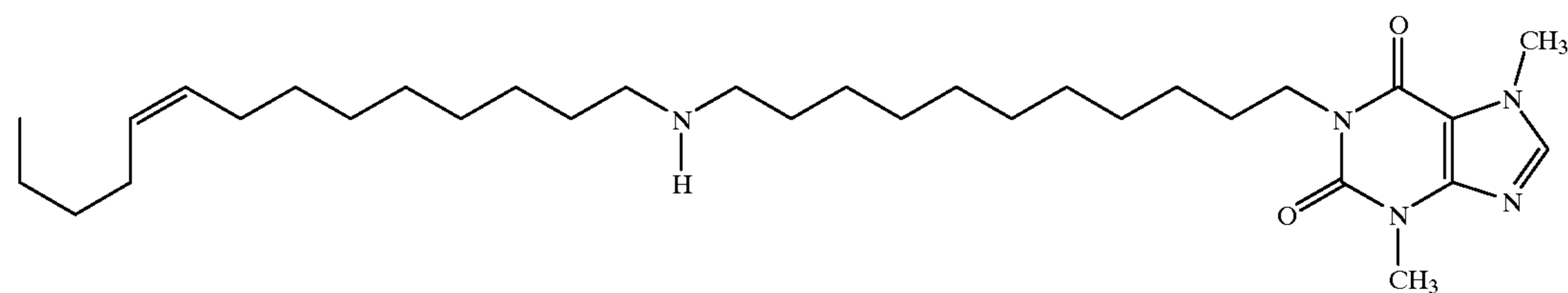
6570 1-[11-cis-9-Tetradecenylamino]undecyl]-3,7-dimethylxanthine
