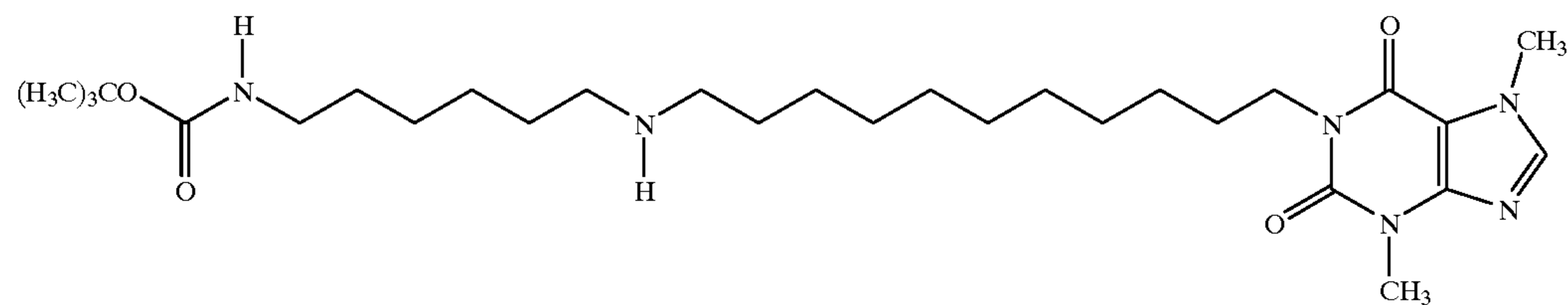
6555 1-(11-[6-Carbobutoxyaminohexylamino]undecyl)-3,7-dimethylxanthine
