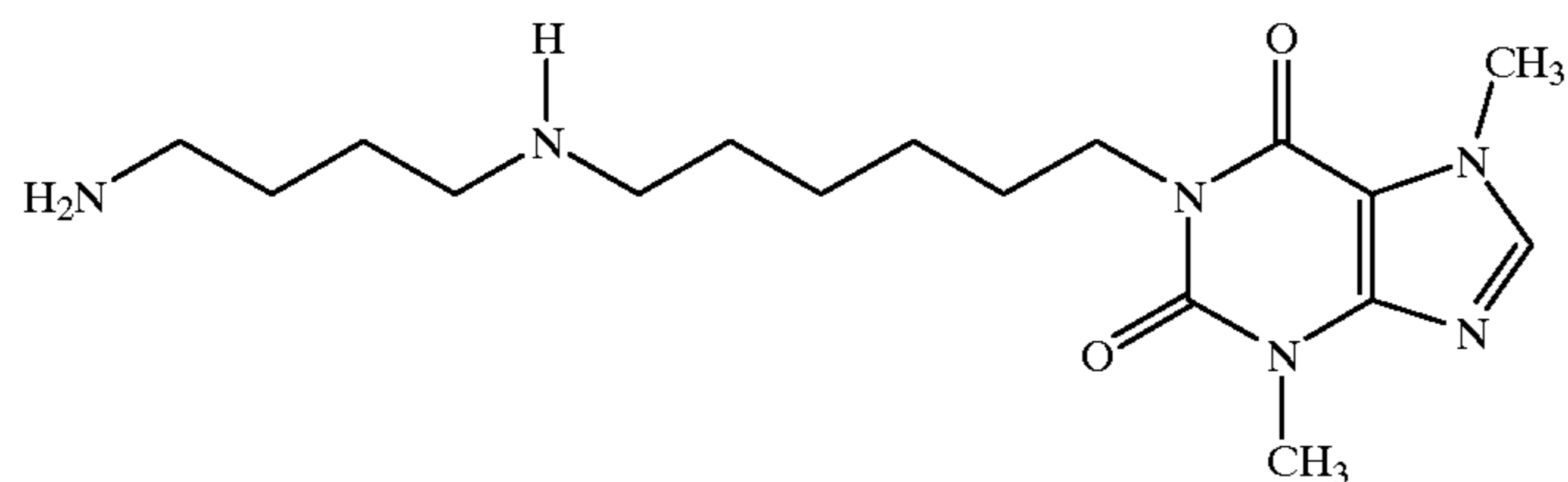
6559 1-(6-[4-Aminobutylamino]hexyl)-3,7-dimethylxanthine
