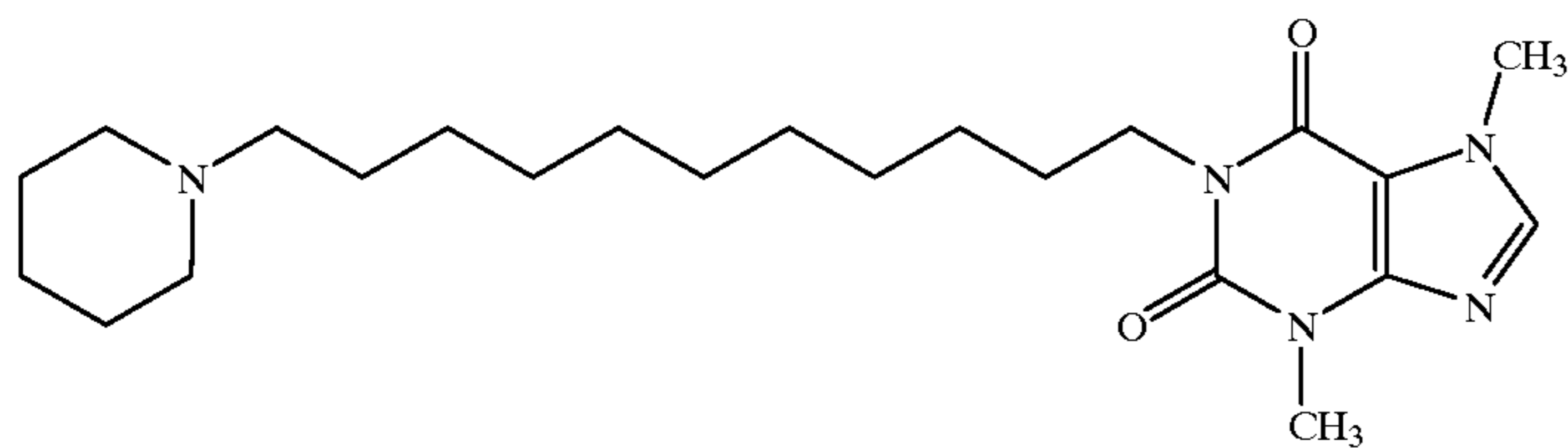
6543 1-[11-(Piperidiny)undecyl]-3,7-dimethylxanthine
