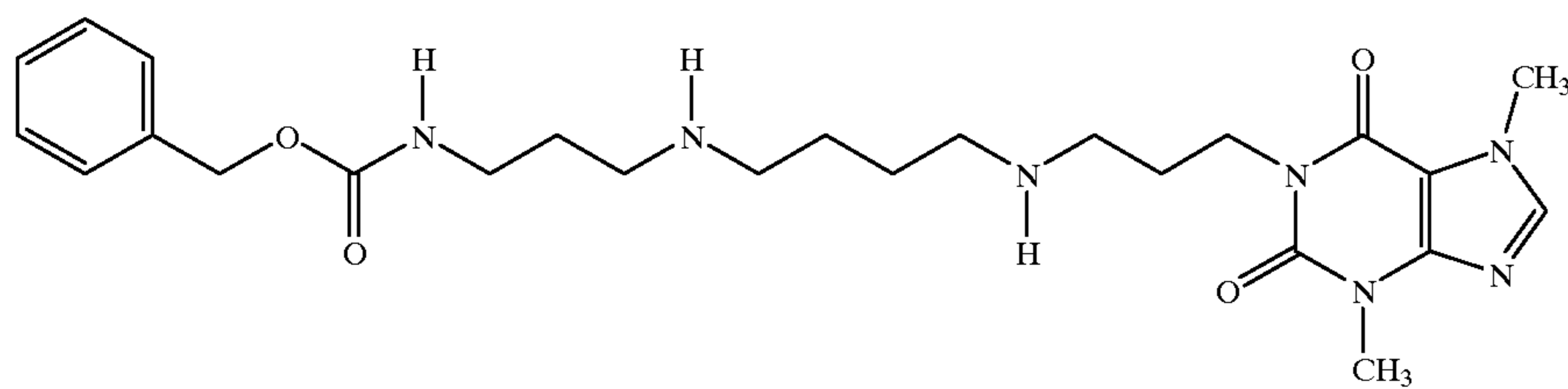
6552 1-(3-[4-(3-Carbobenzyloxyaminopropylamino)butylamino]propyl)-3,7-dimethylxanthine
