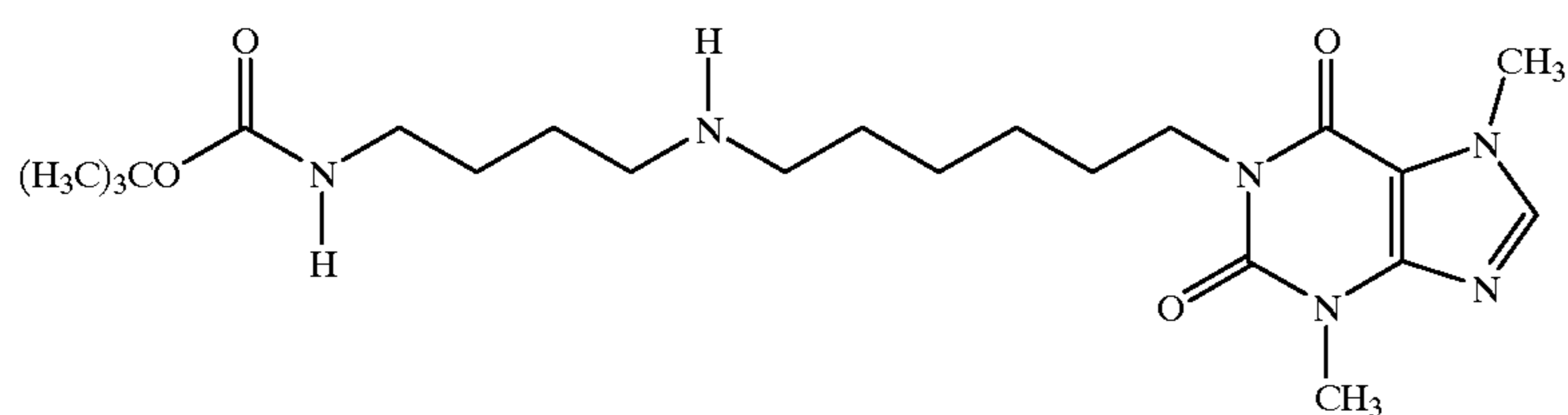
6558 1-(6-[4-Carbobutoxyaminobutylamino]hexyl)-3,7-dimethylxanthine
