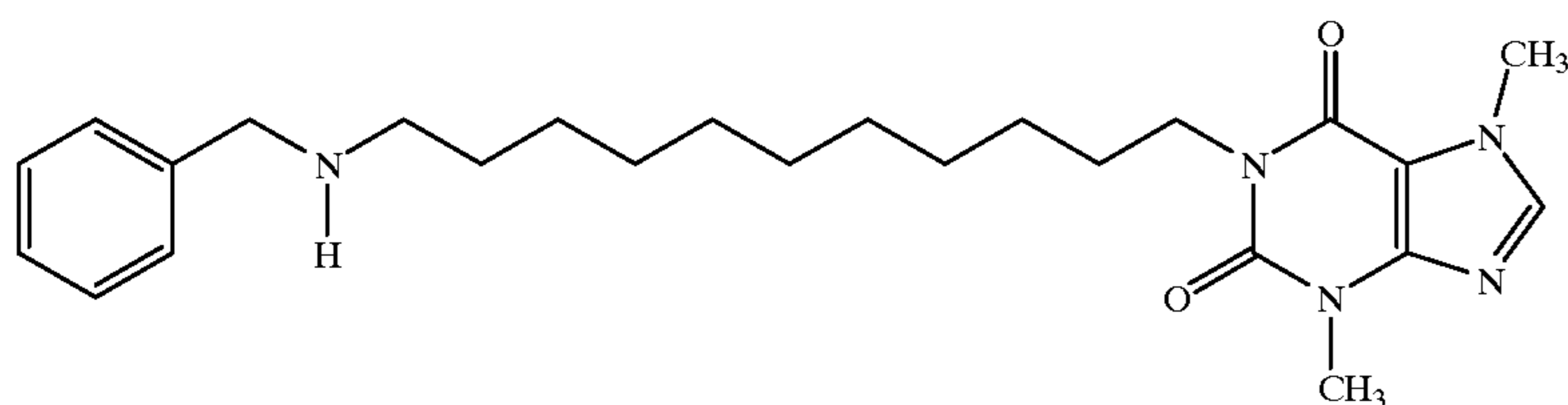
6531 1-[11-Benzylamino]undecyl]-3,7-dimethylxanthine
