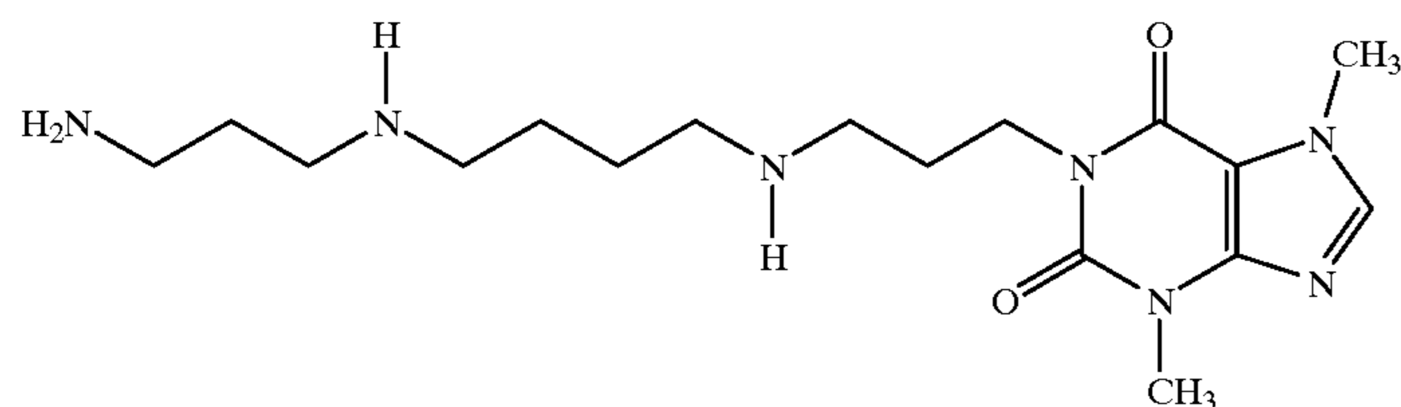
6553 1-(3-[4-(3-Aminopropylamino)butylamino]propyl)-3,7-dimethylxanthine
