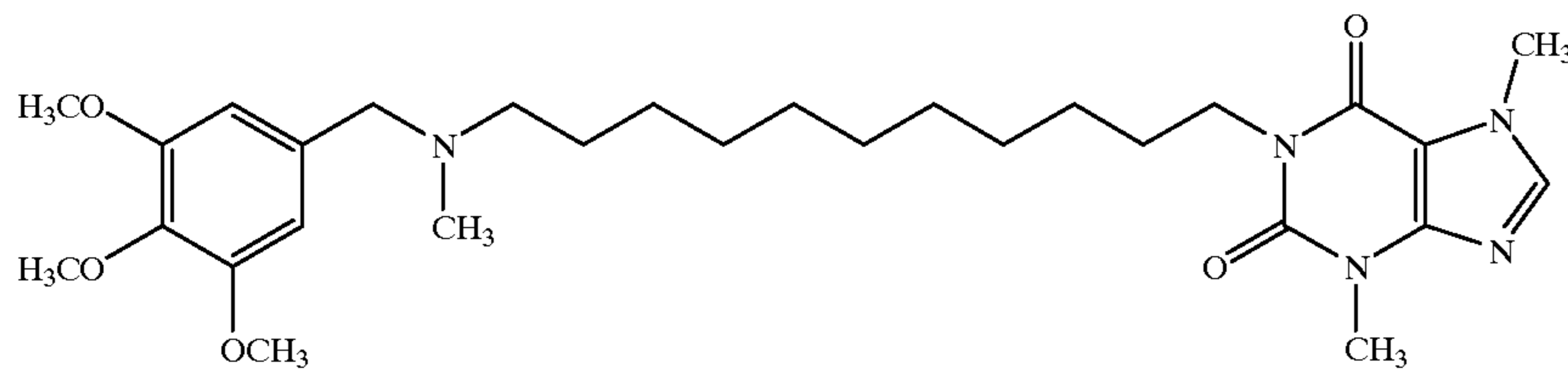
6571 1-[11-(N-Methyl-N-[3,4,5-trimethoxybenzyl]amino)undecyl]-3,7-dimethylxanthine
