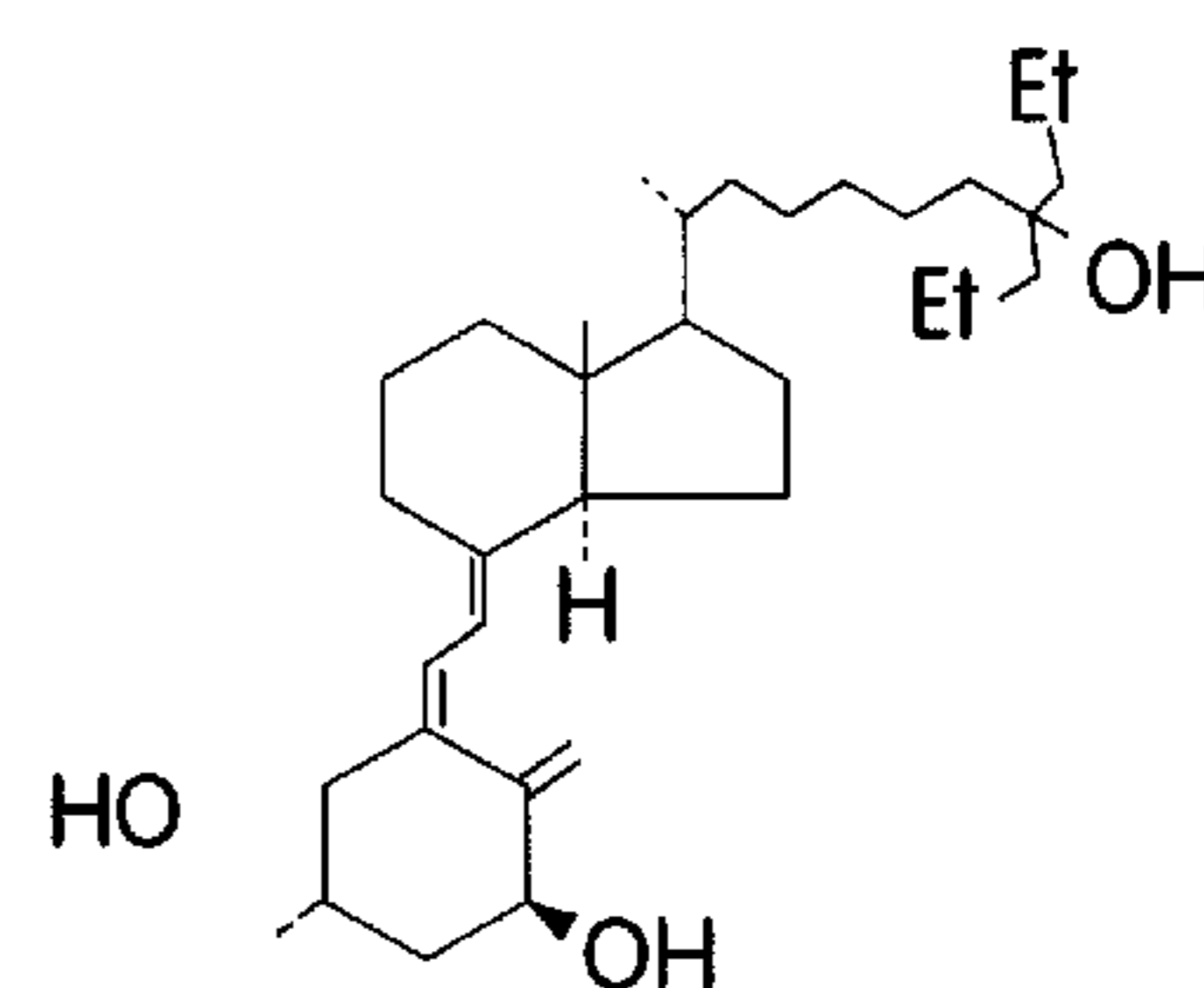
24-dihomo-26,27-diethyl- 1 \alpha ,25-(OH) 2 -D 3
