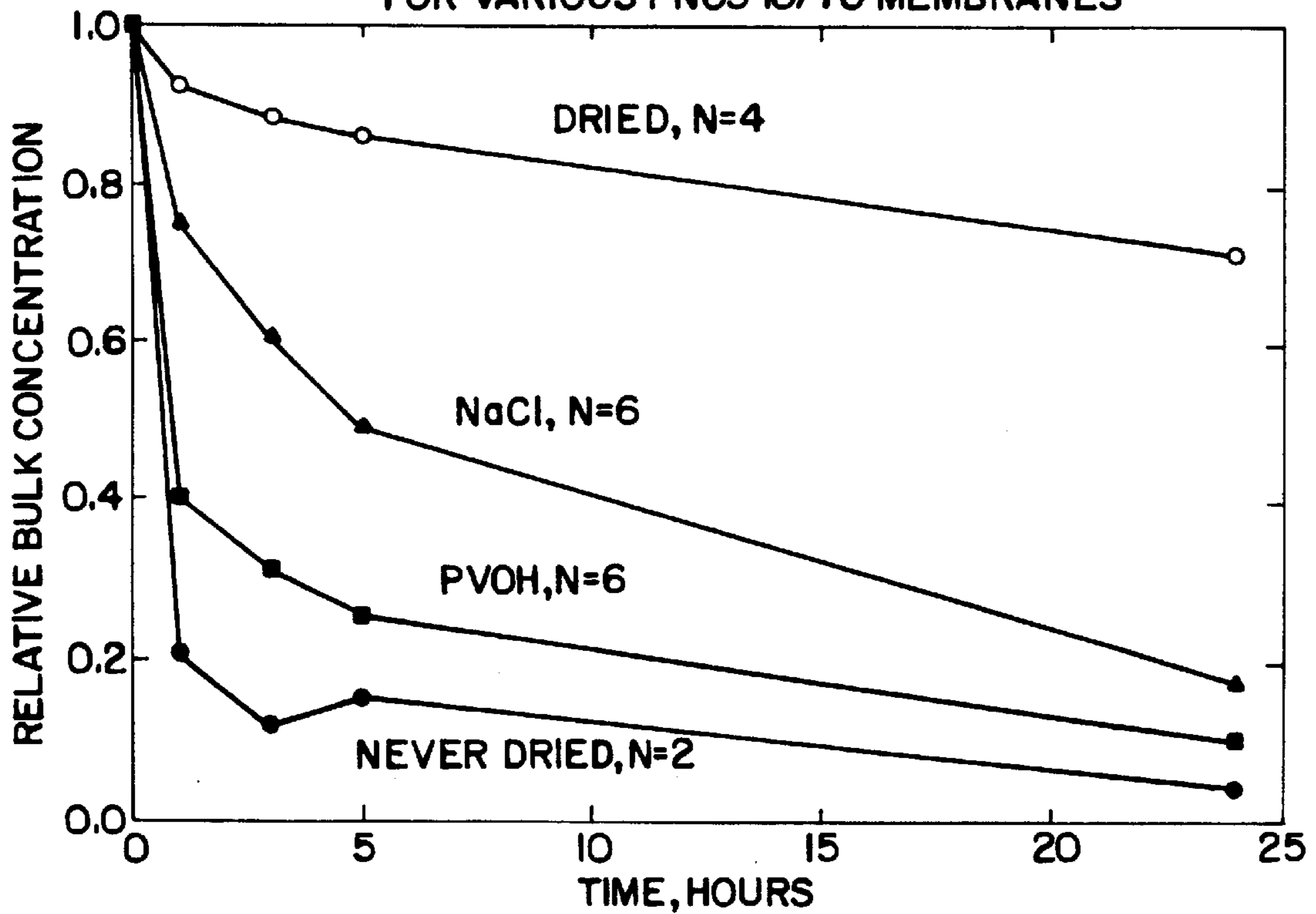
GLUTATHIONE SORPTION FOR VARIOUS PNO3 IO/70 MEMBRANES
