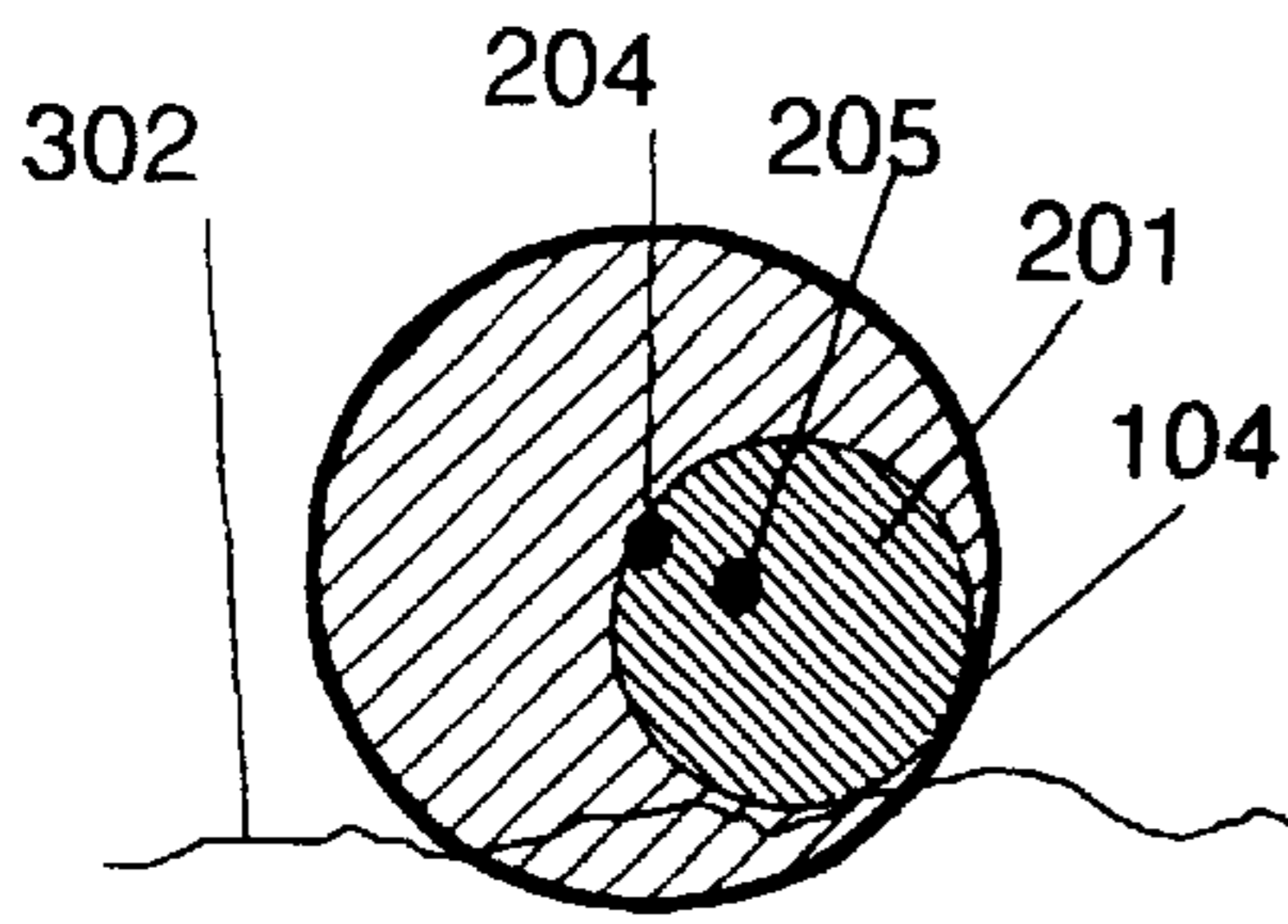
FIG. 2-A (section A-A)
