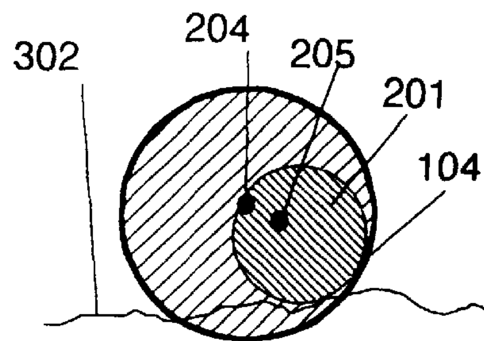
FIG. 2-A (section A-A)
