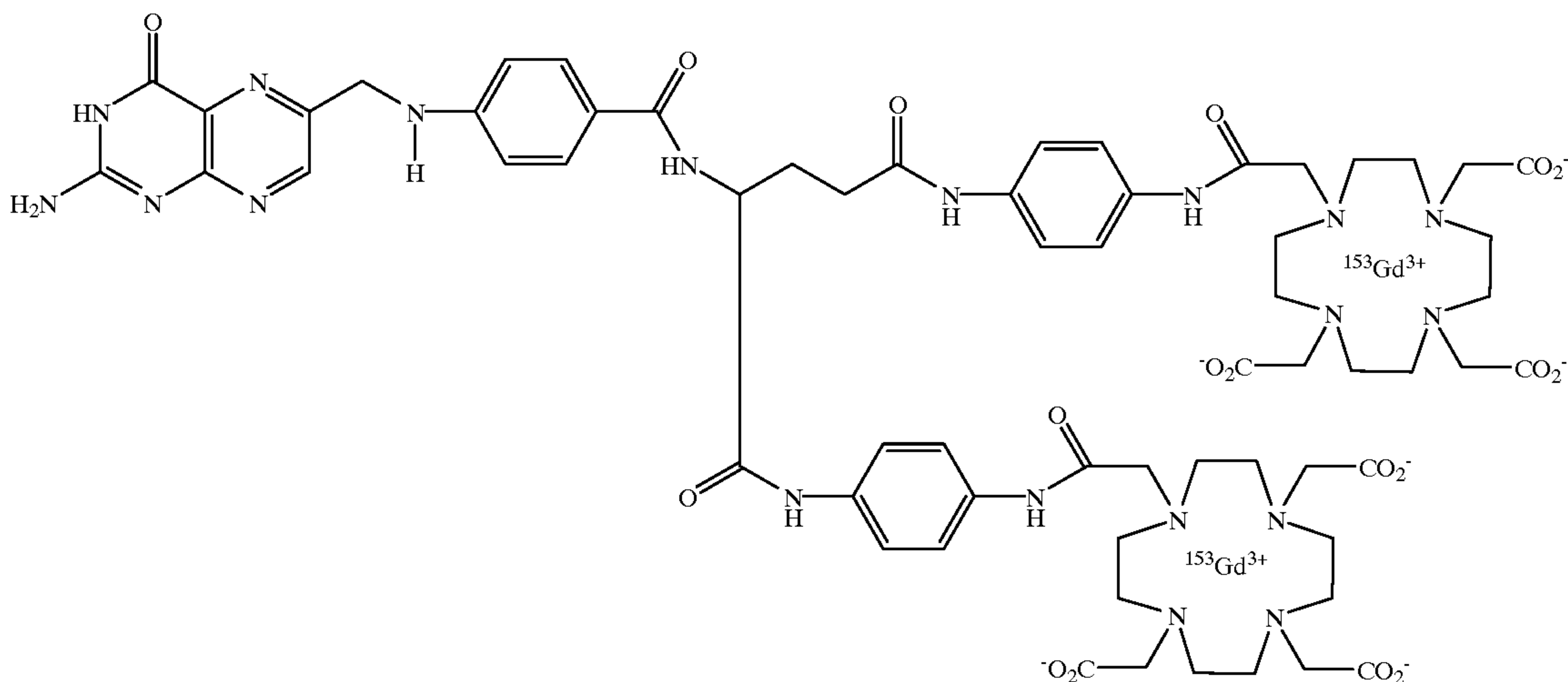
Bis( 153 Gd-DO3A-APA)-folate
