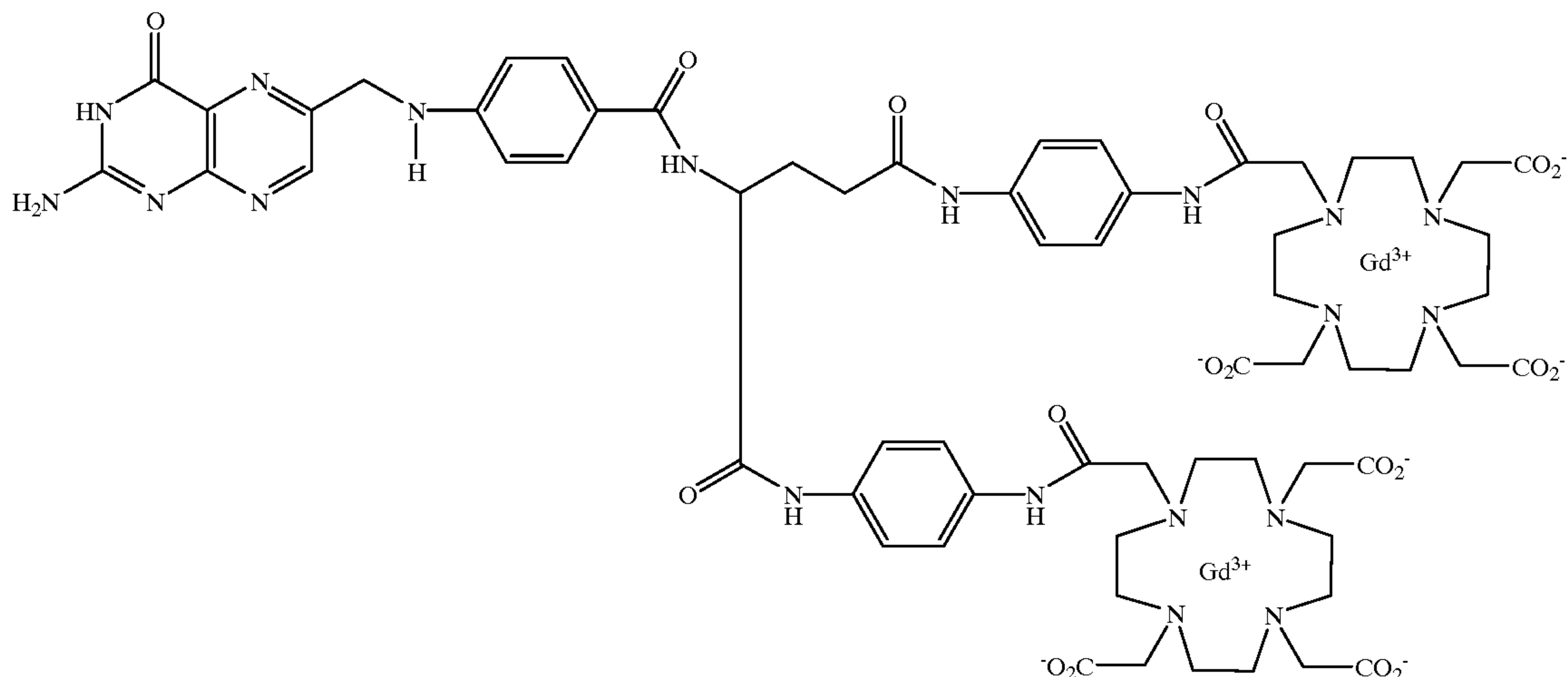
Bis(Gd-DO3A-APA)-folate
