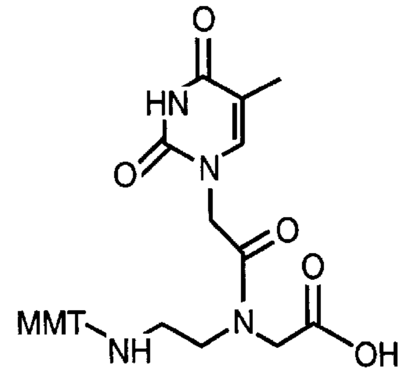
MMT-PNA-T
