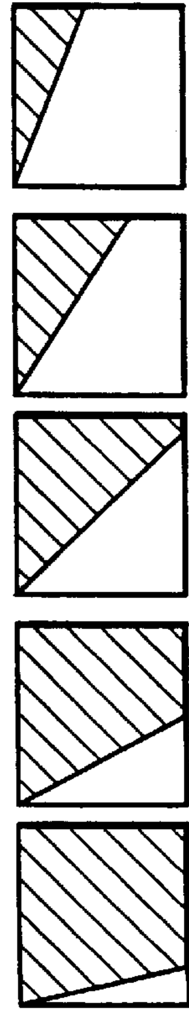
M=4
