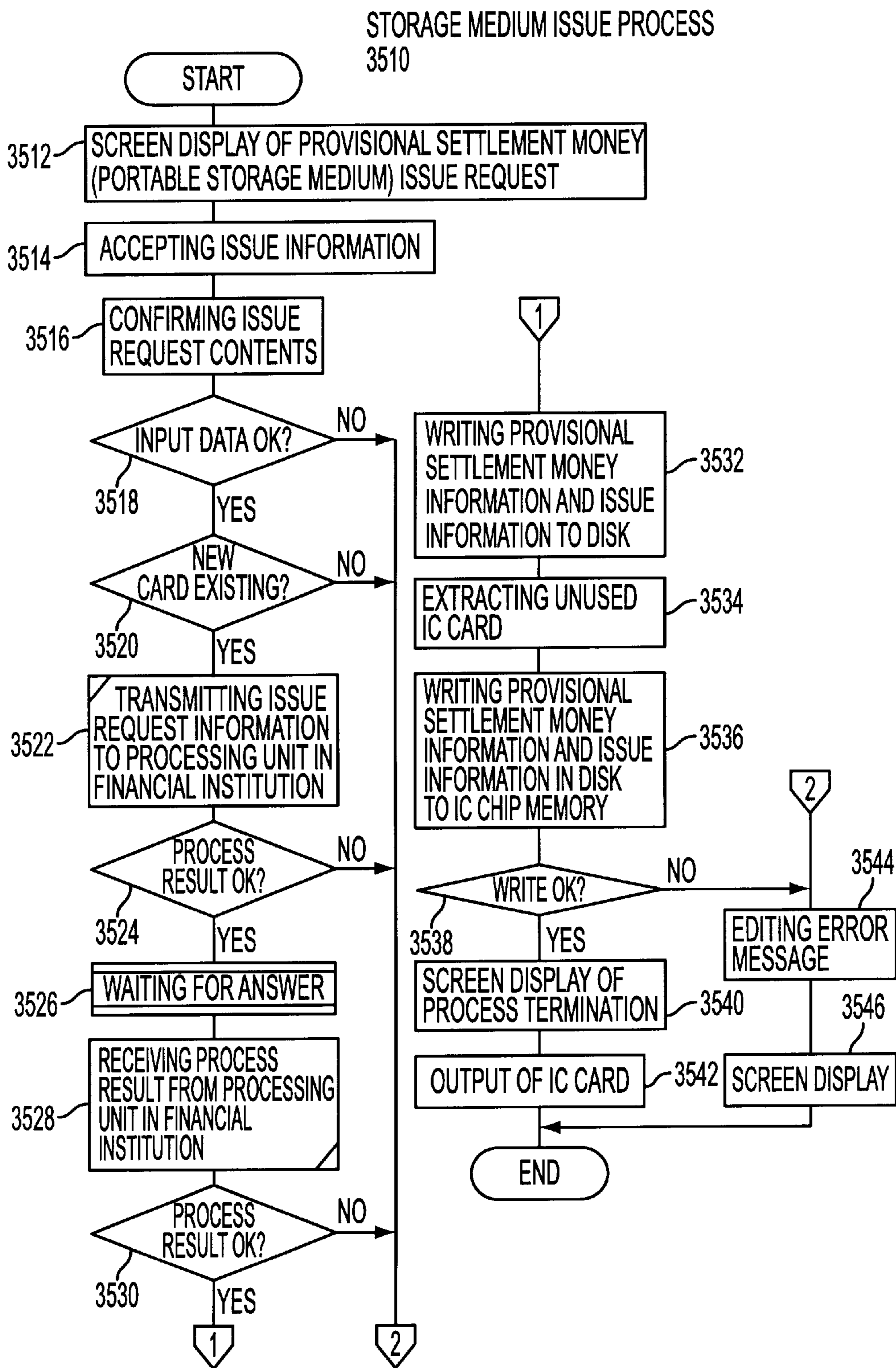
FIG. 48
