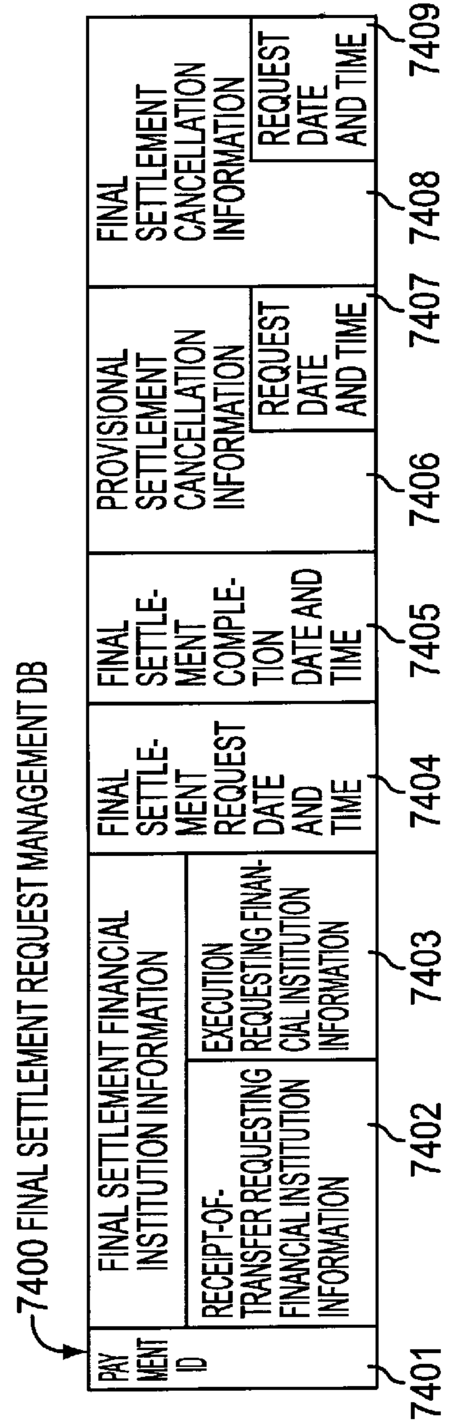
FIG. 81B
