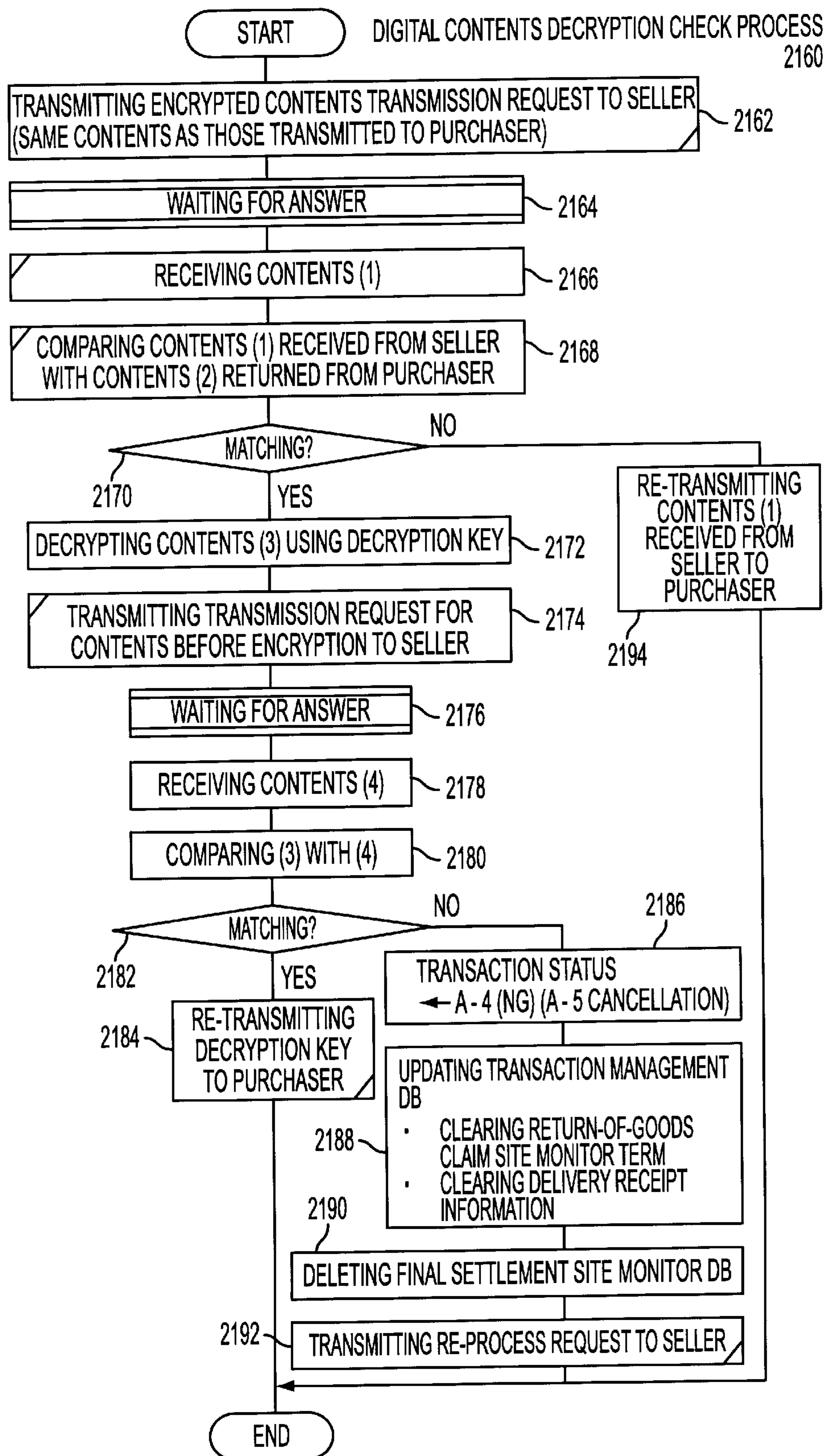
FIG. 39
