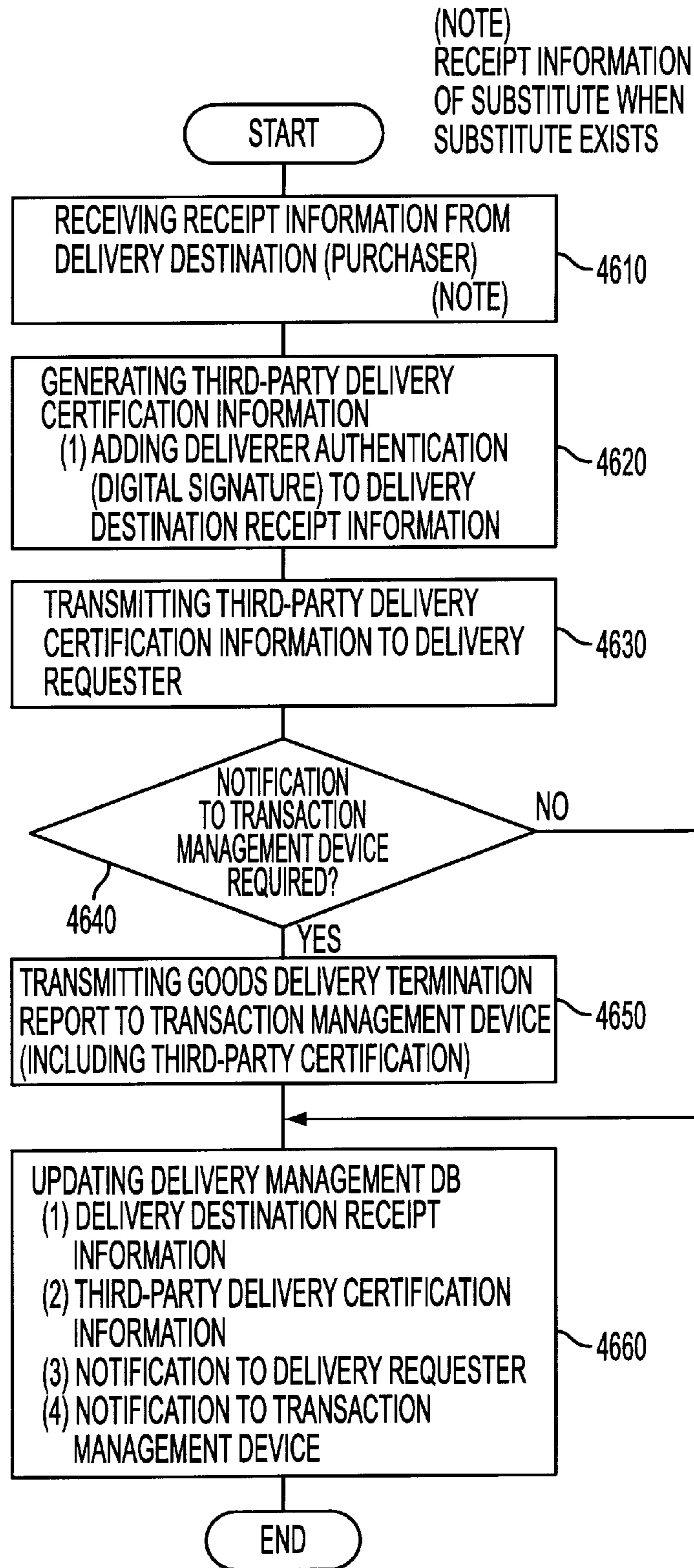
FIG. 55
