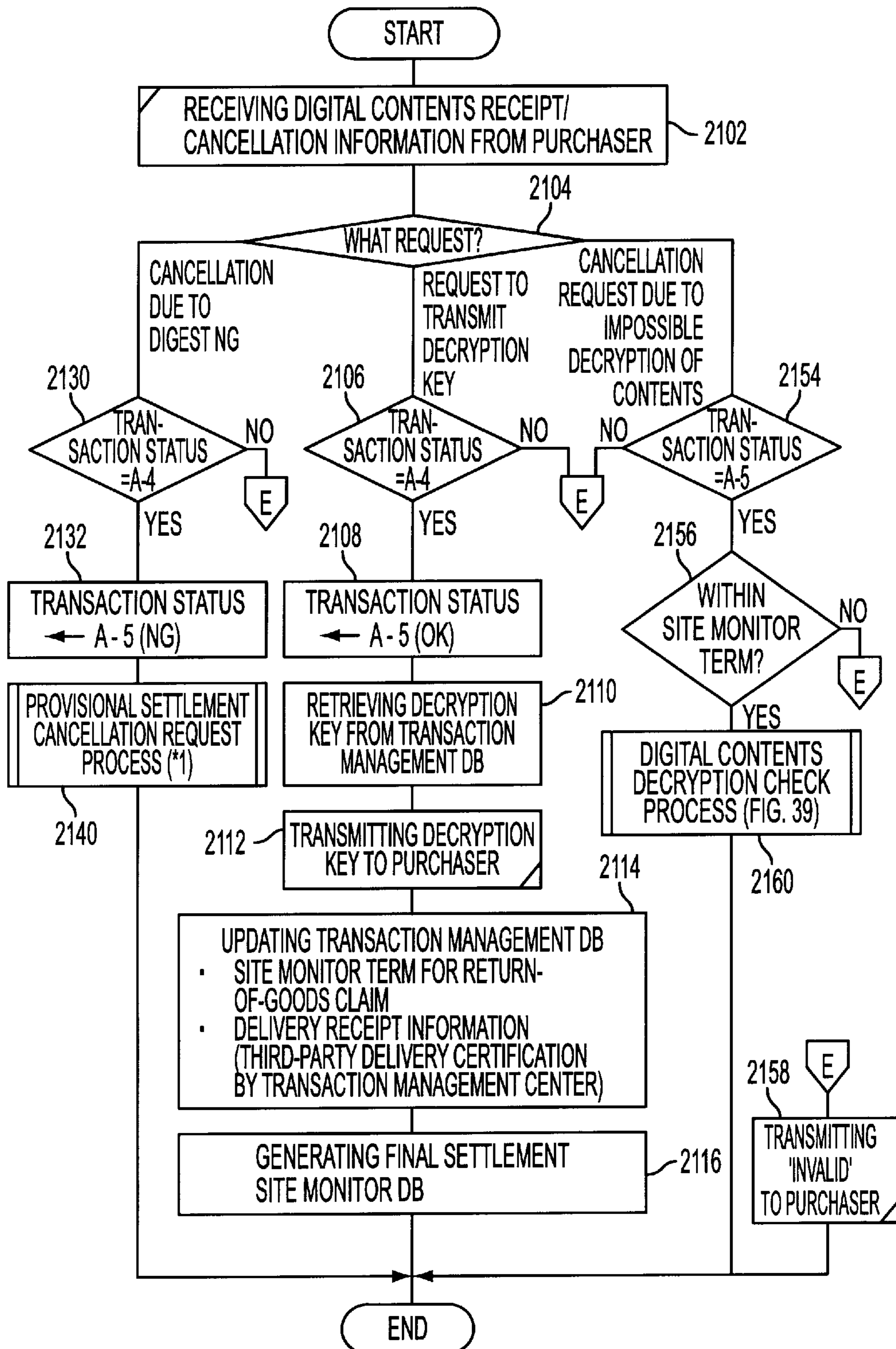
FIG. 37
