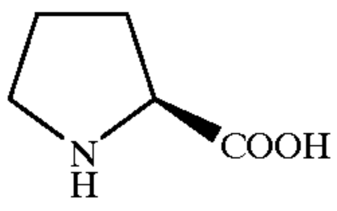
L-Pro
