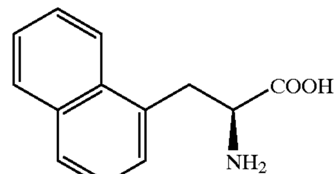
L-1-Nal
