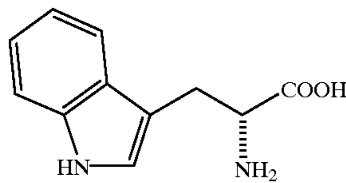
D-Trp
