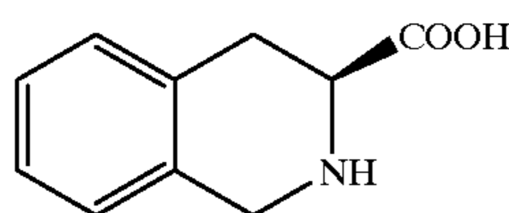
L-Tic
