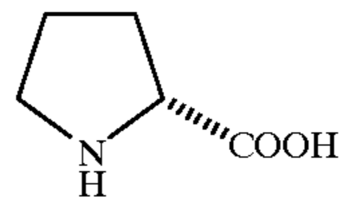
D-Pro
