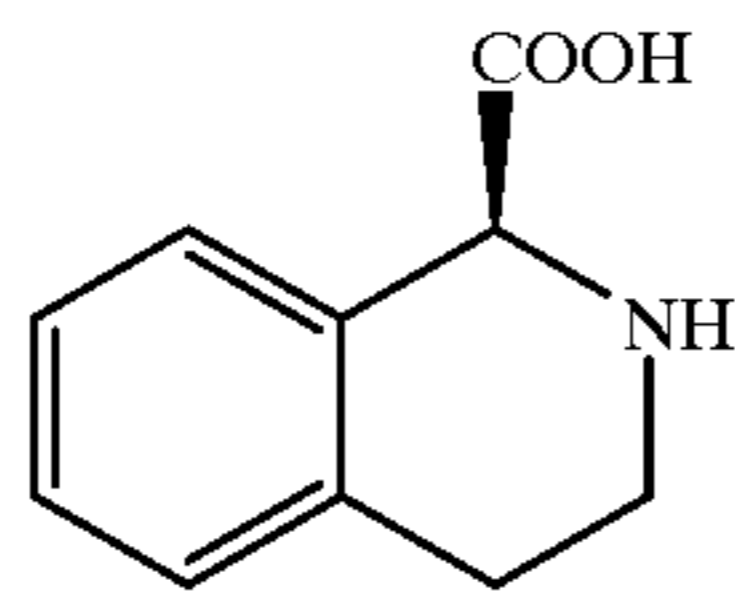
L-Tiq
