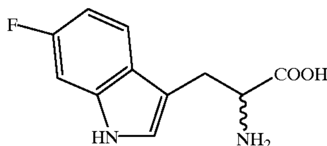
L-(Benzo[thienyl]-alanine
