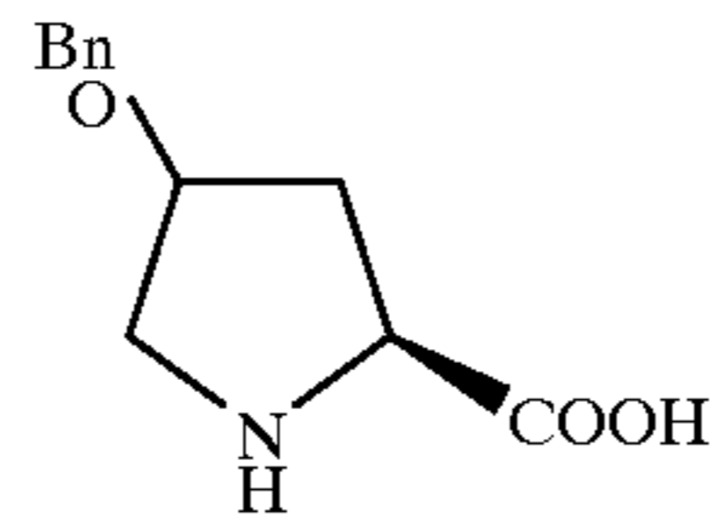
L-4-Hyp(OBn)
