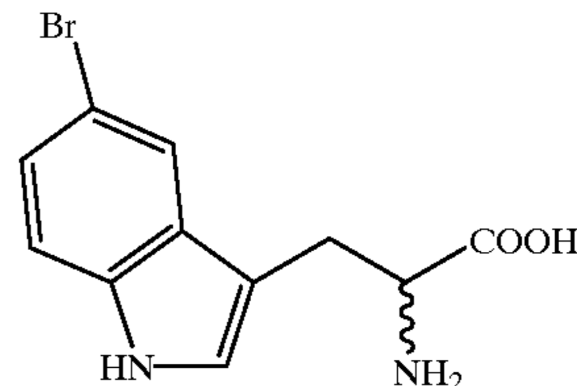
DL-5-Br-Trp
