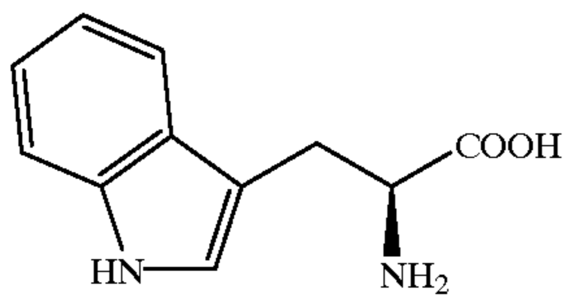
L-Trp
