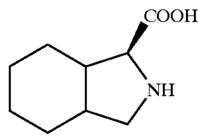
L-Oic
