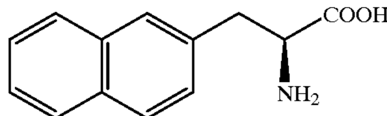
D-Trp
