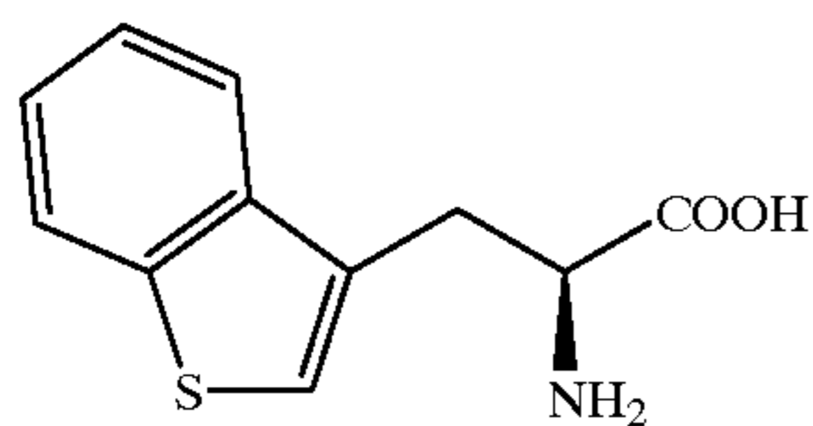
L-(Benzo[thienyl]-alanine
