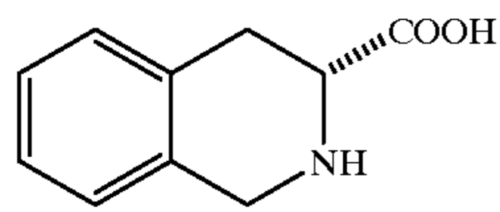
D-Tic
