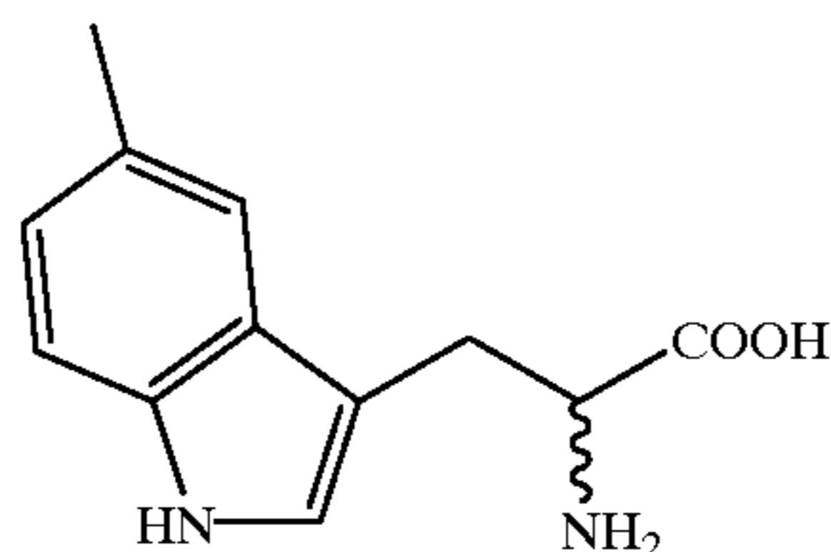
DL-5-Me-Trp
