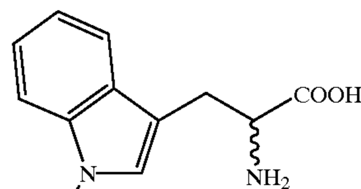
DL-1-Me-Trp
