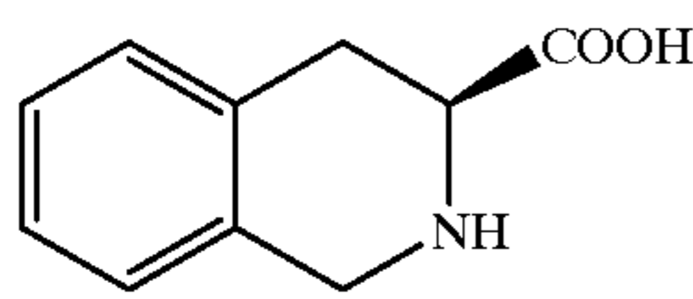
L-Tic
