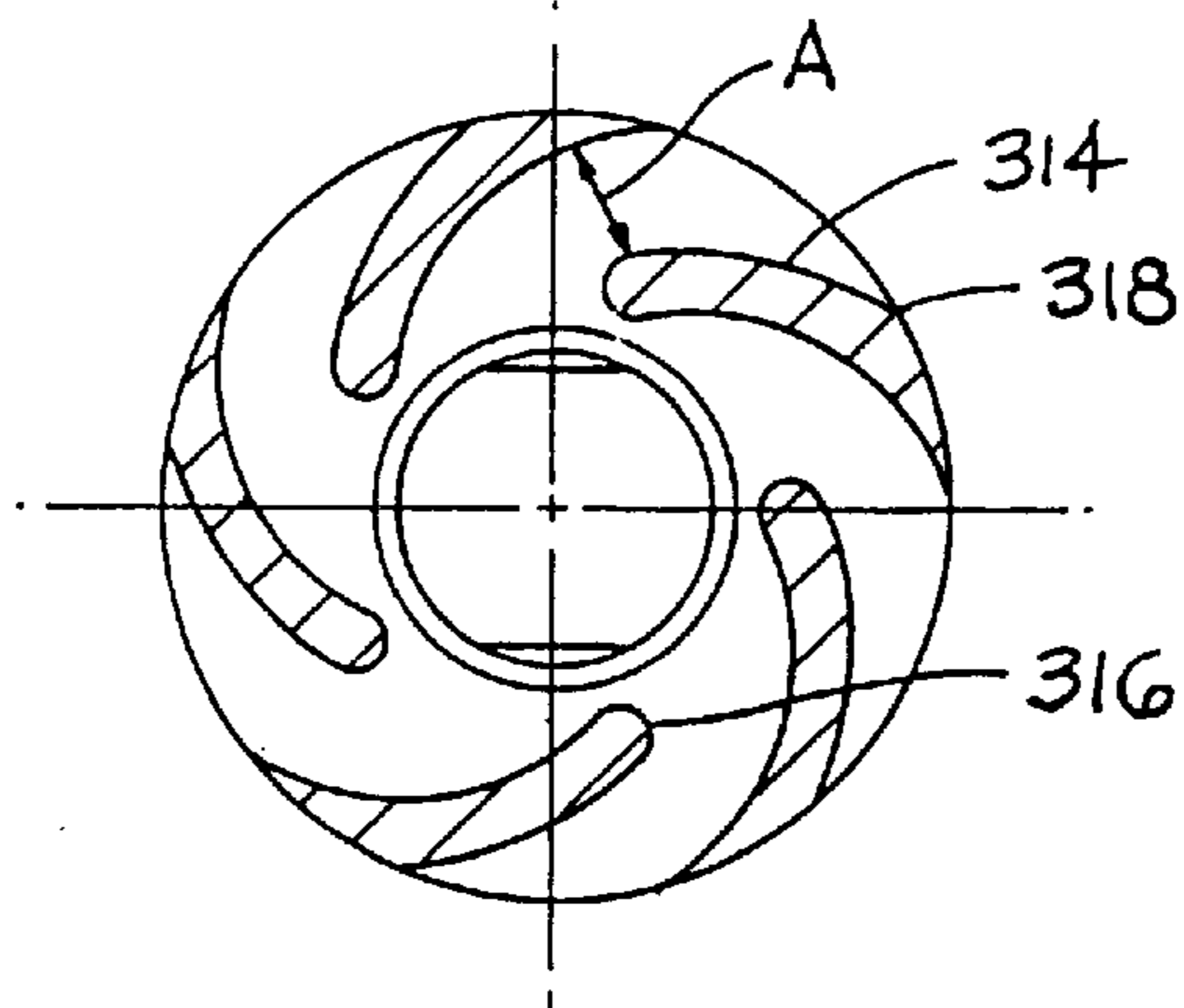
FIG. 15
