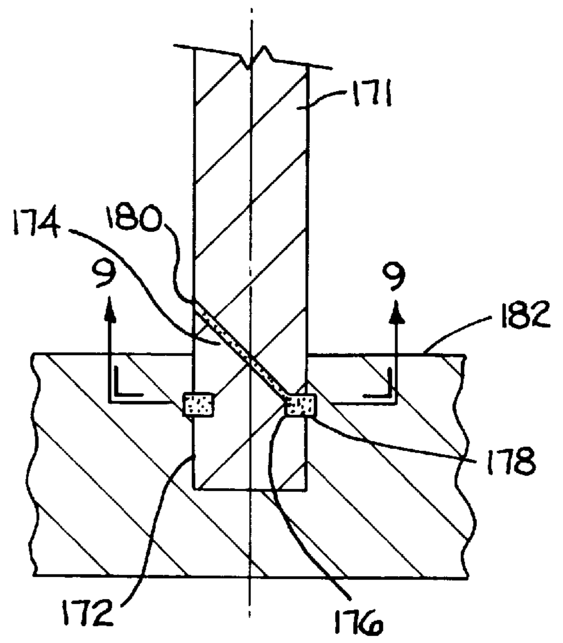
FIG. 8A
