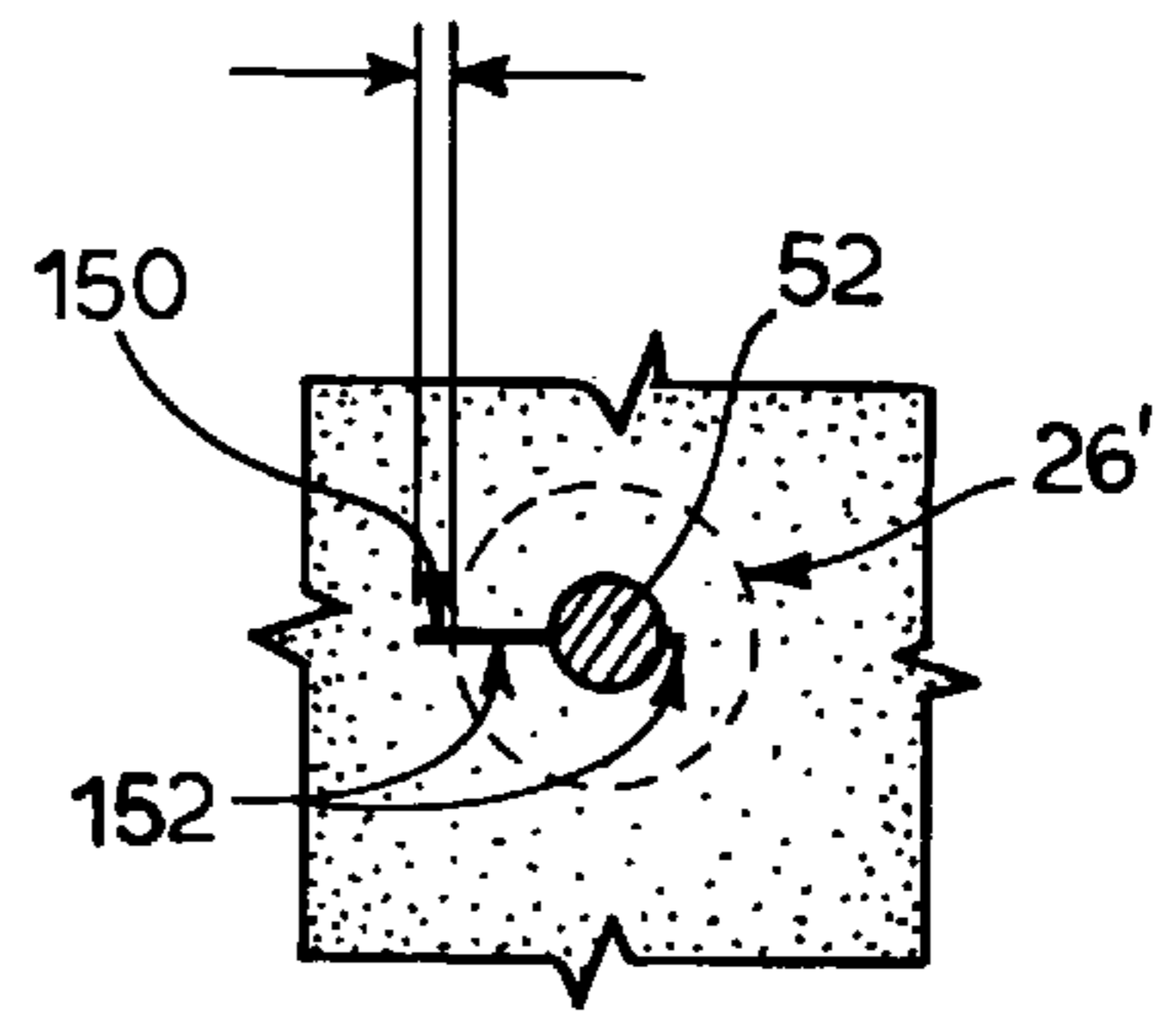
FIG.16. SECTION A-A
