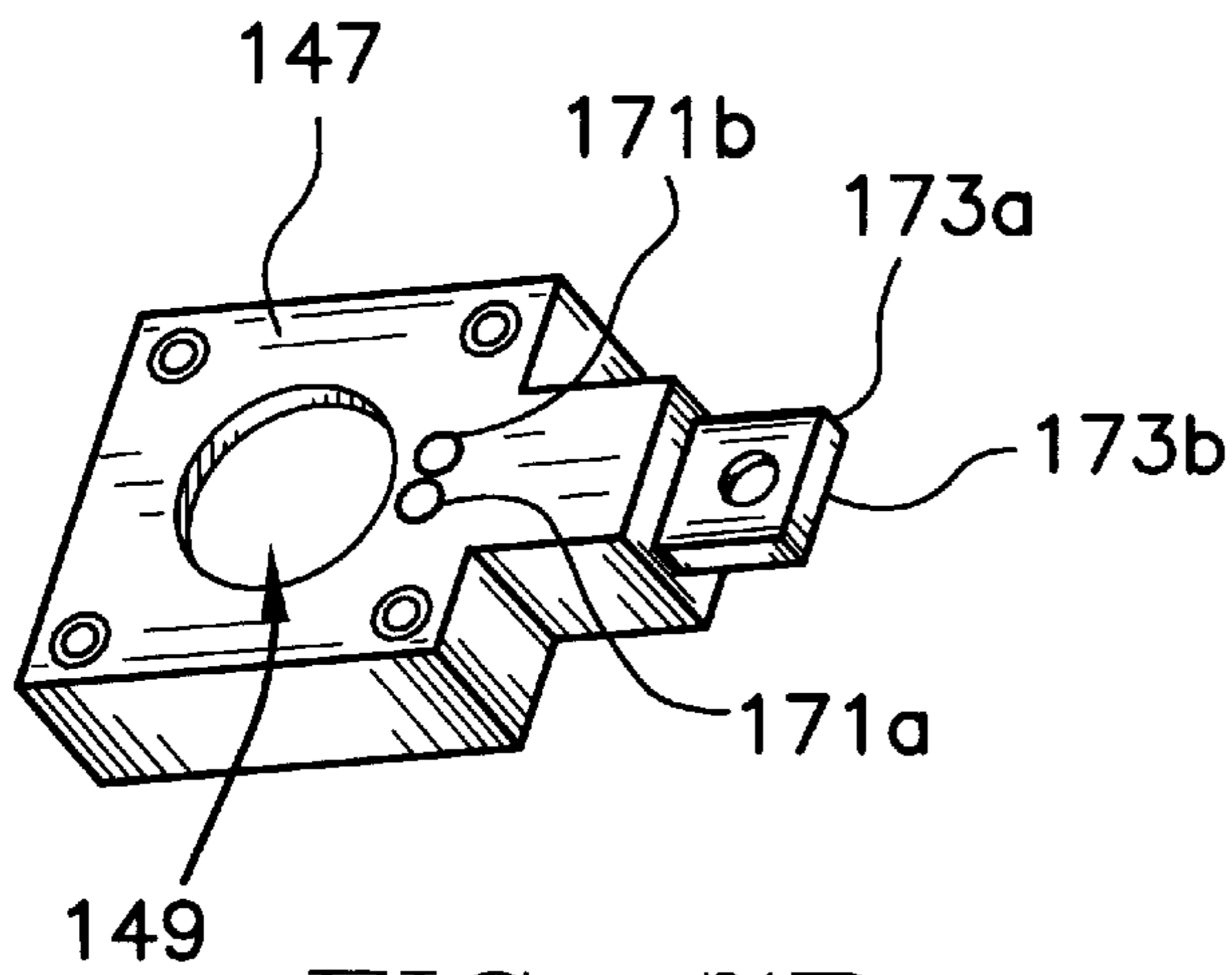
FIG. 7B
