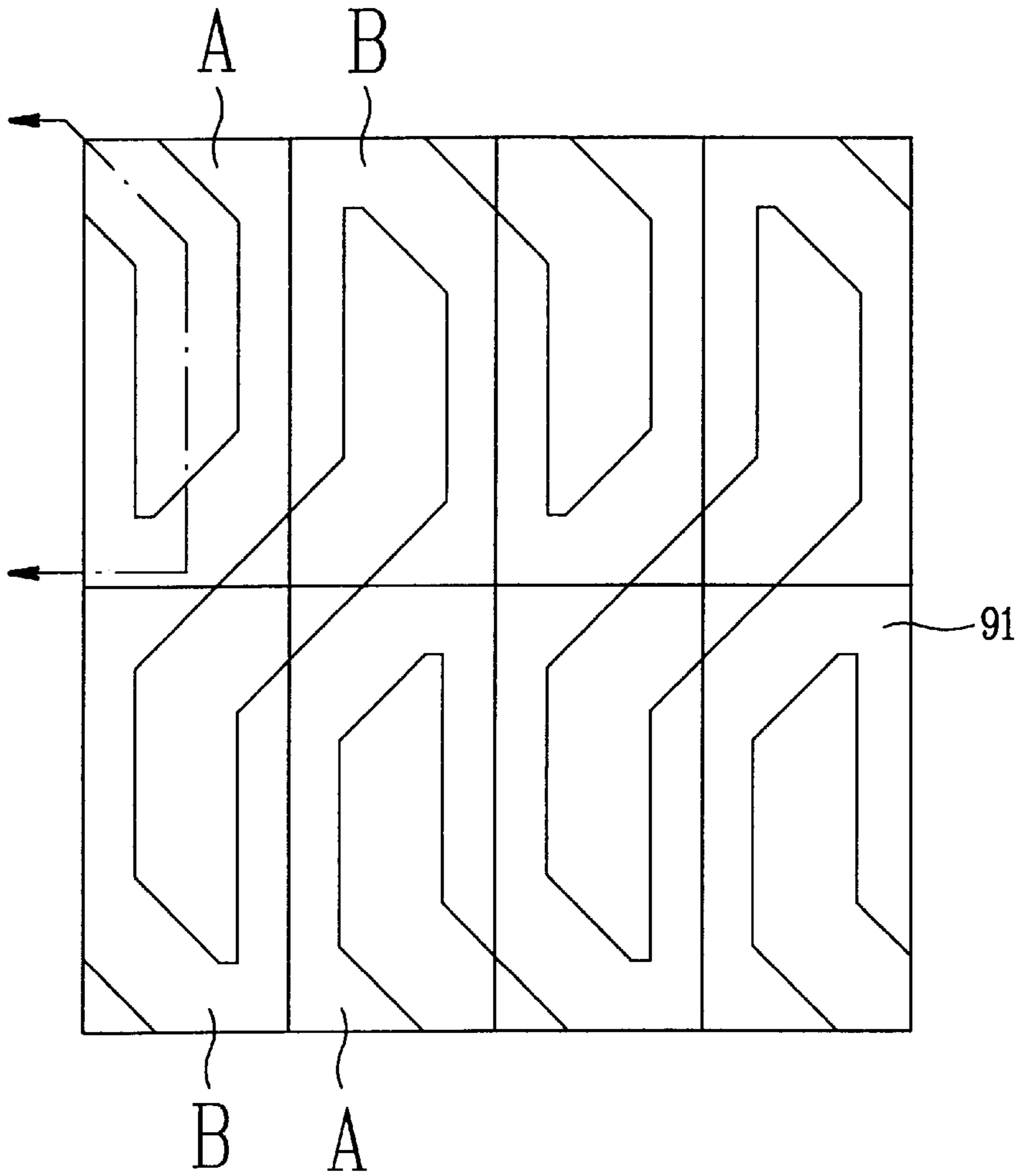
FIG. 9a
