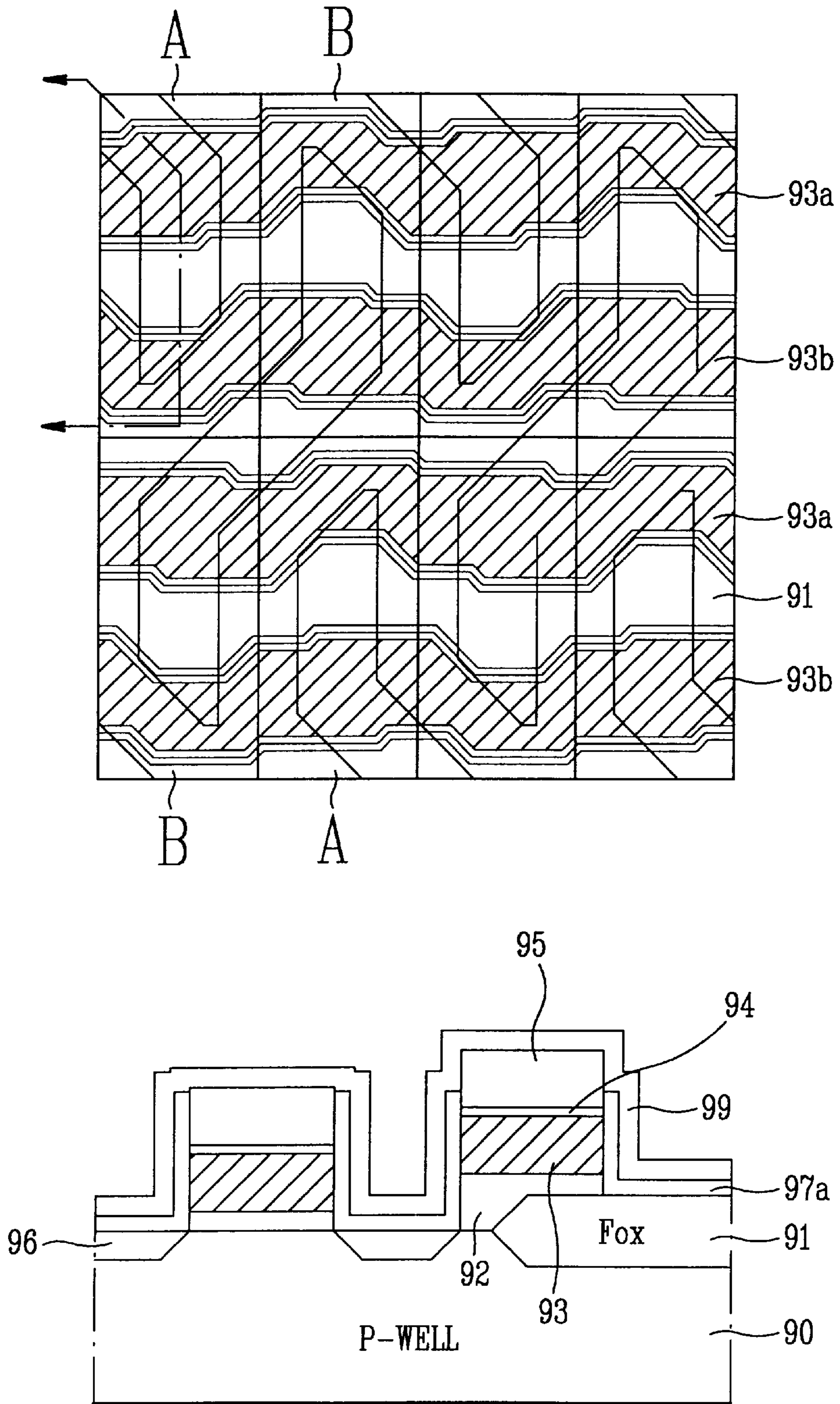
FIG. 10i
