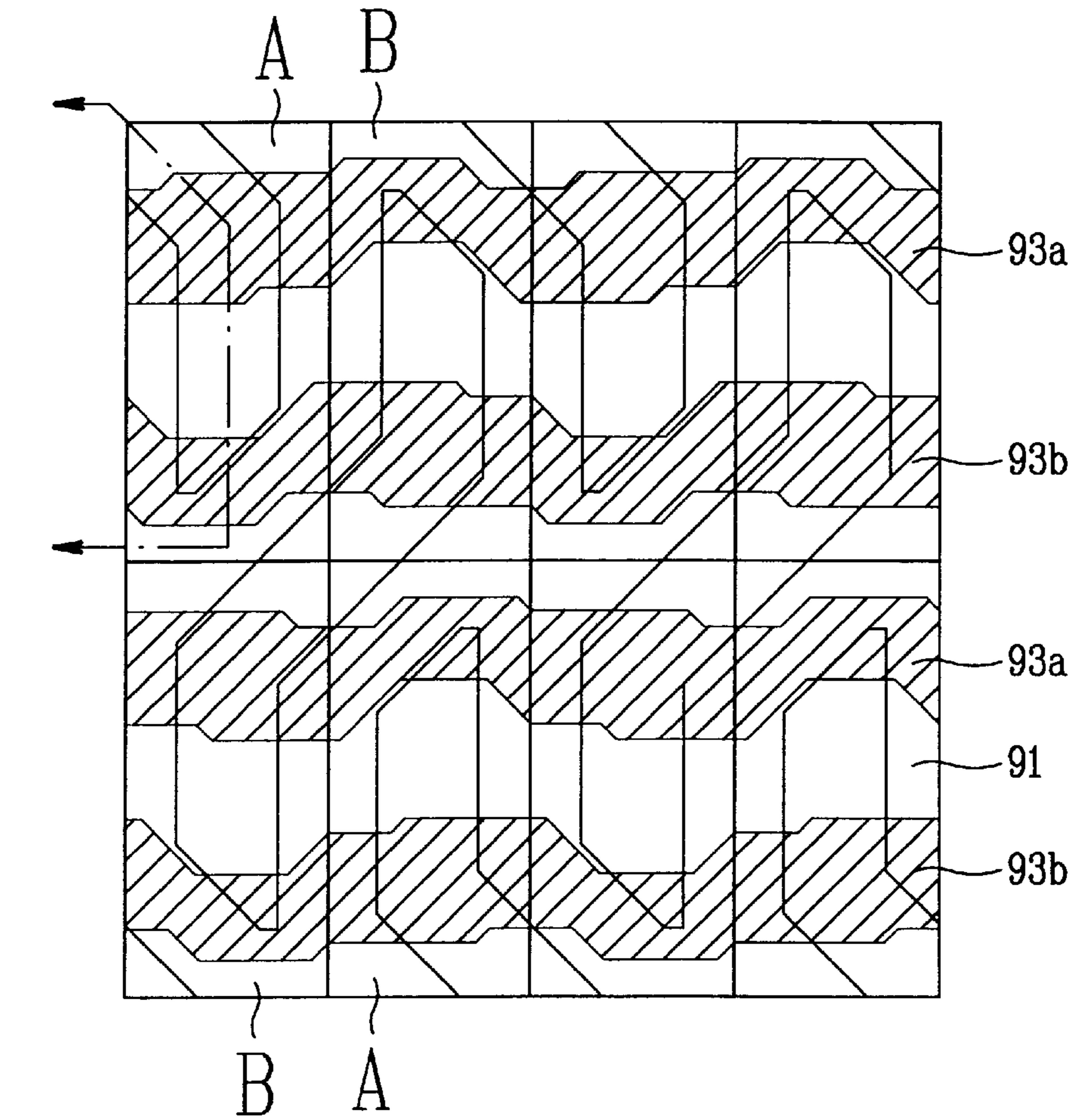
FIG. 9c
