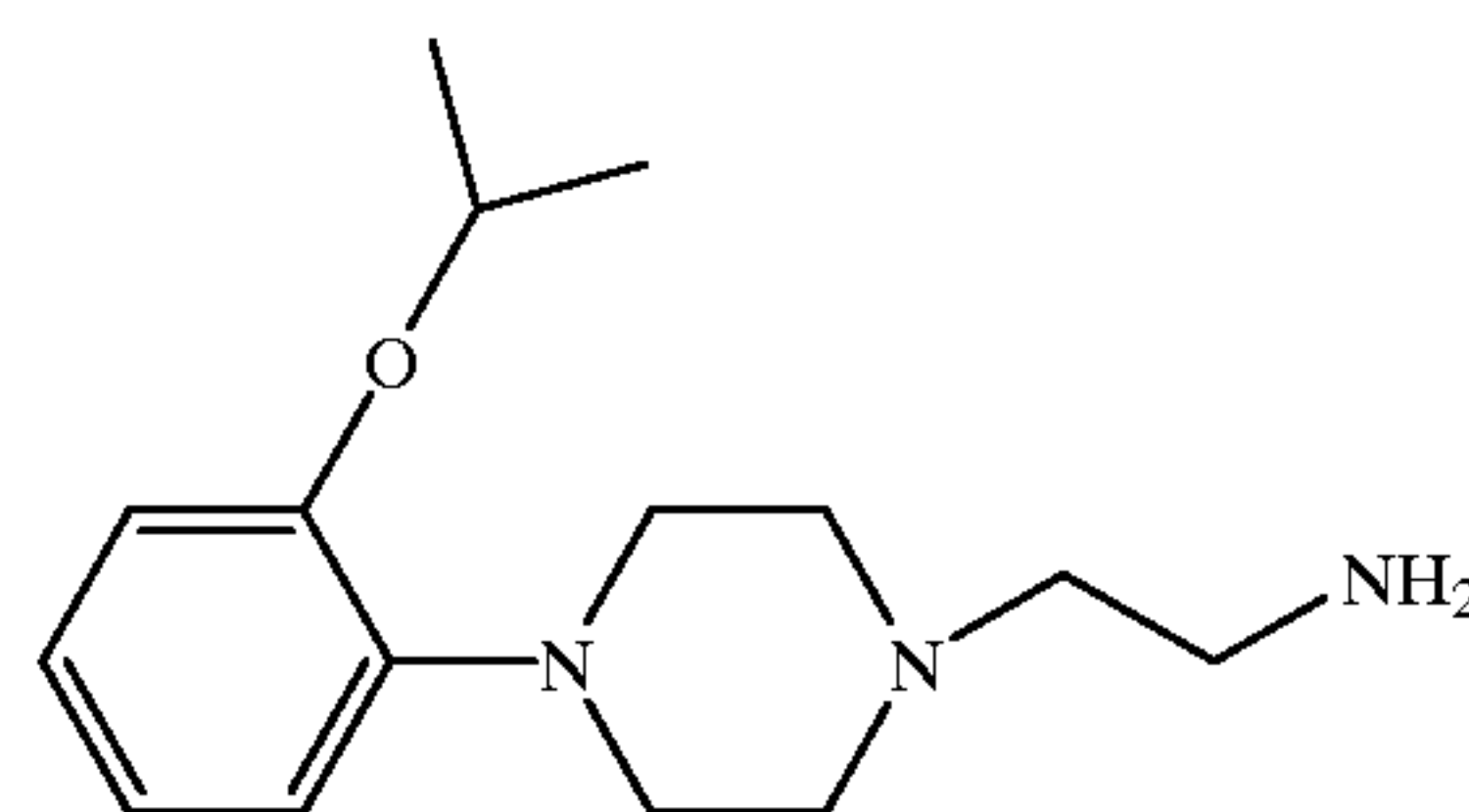
1-(2-Aminoethyl)-4-(2-2- iso-propoxyphenyl)piperazine
