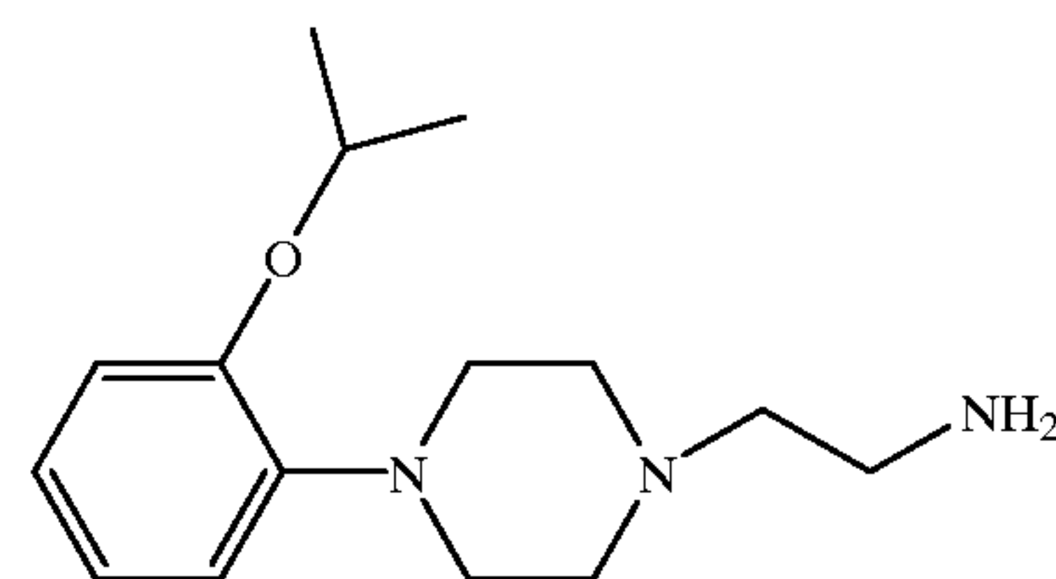
1-(2-Aminoethyl)-4-(2-isopropoxyphenyl) piperazine
