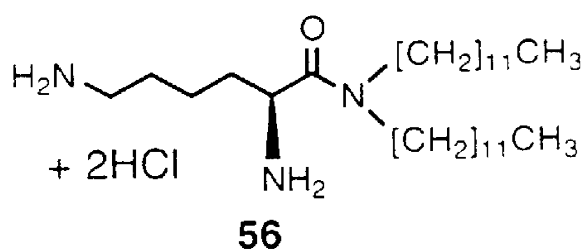
N 1 ,N 1 -dioctadecyl-1,2,6-triaminohexane tri HCl salt
