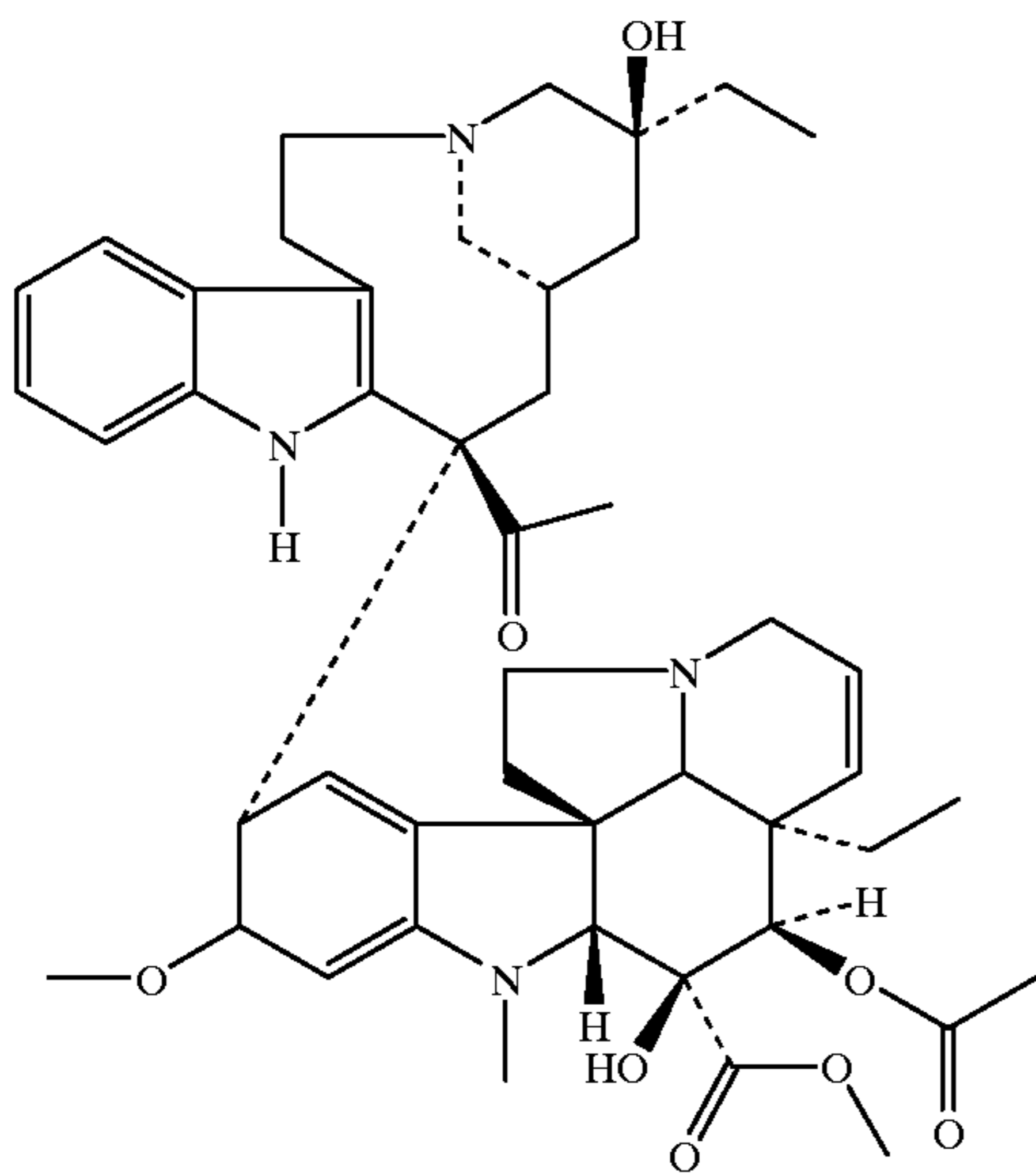
Vinblastine
