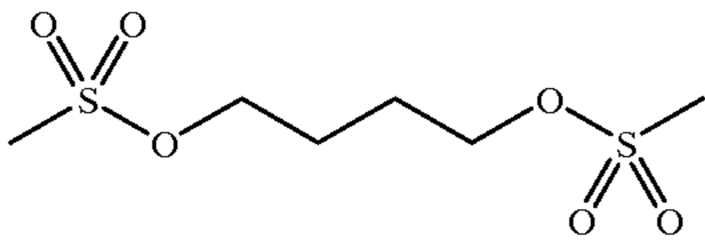
Busulfan
