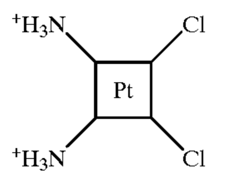
Cisplatin
