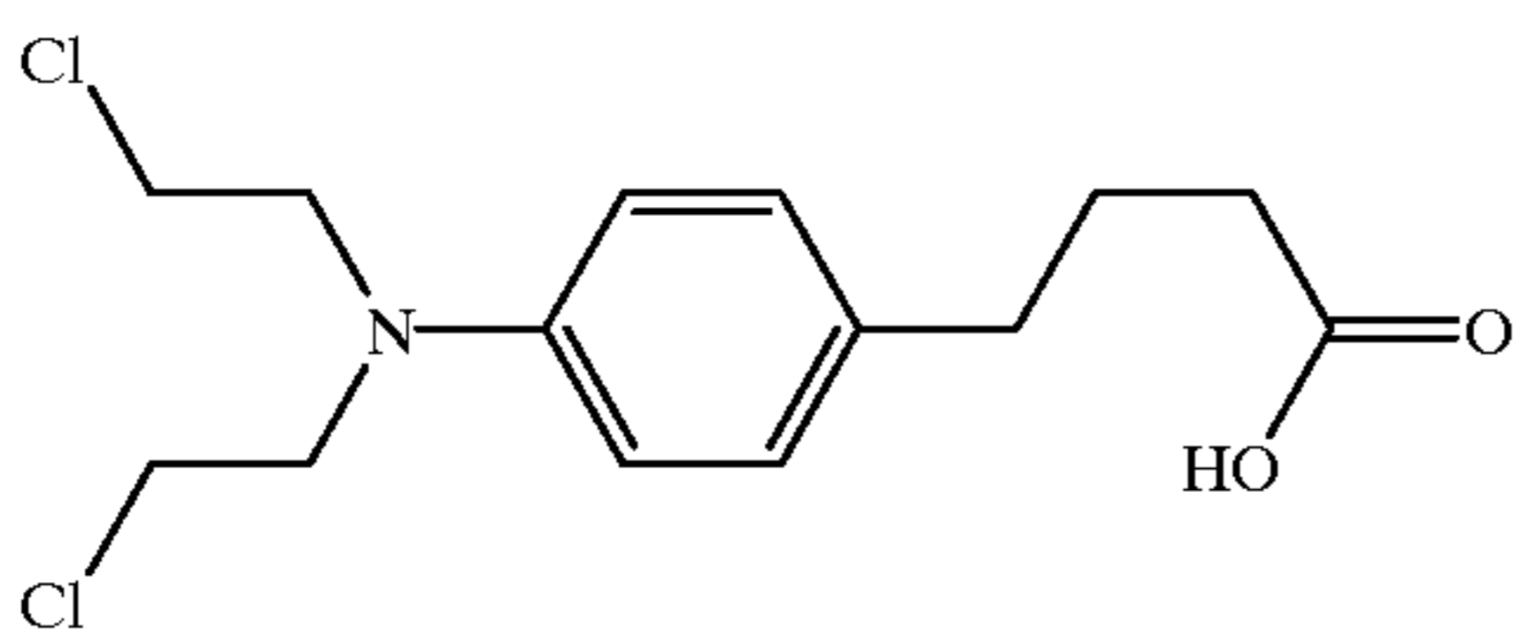
Chlorambucil
