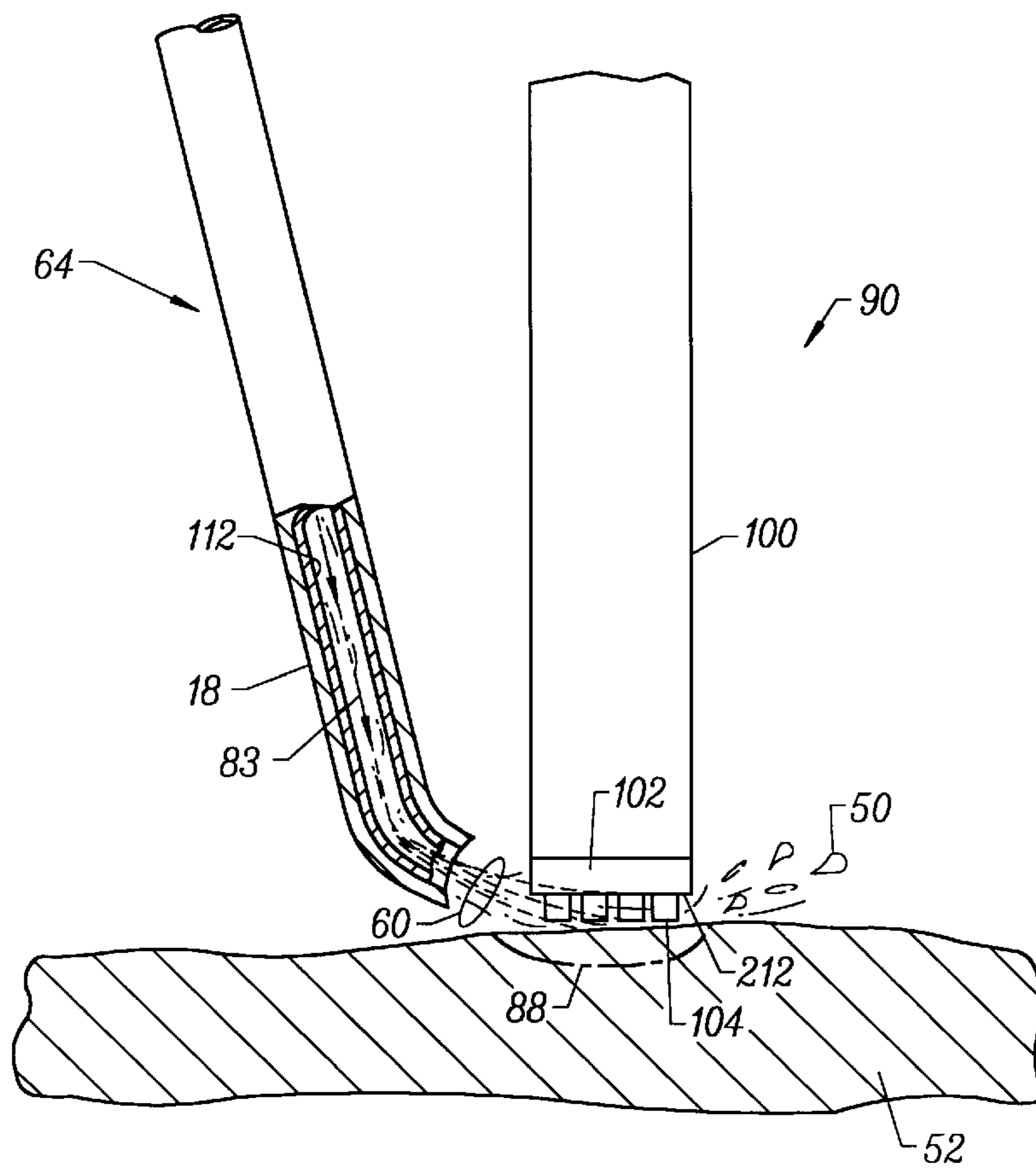
FIG. 15
