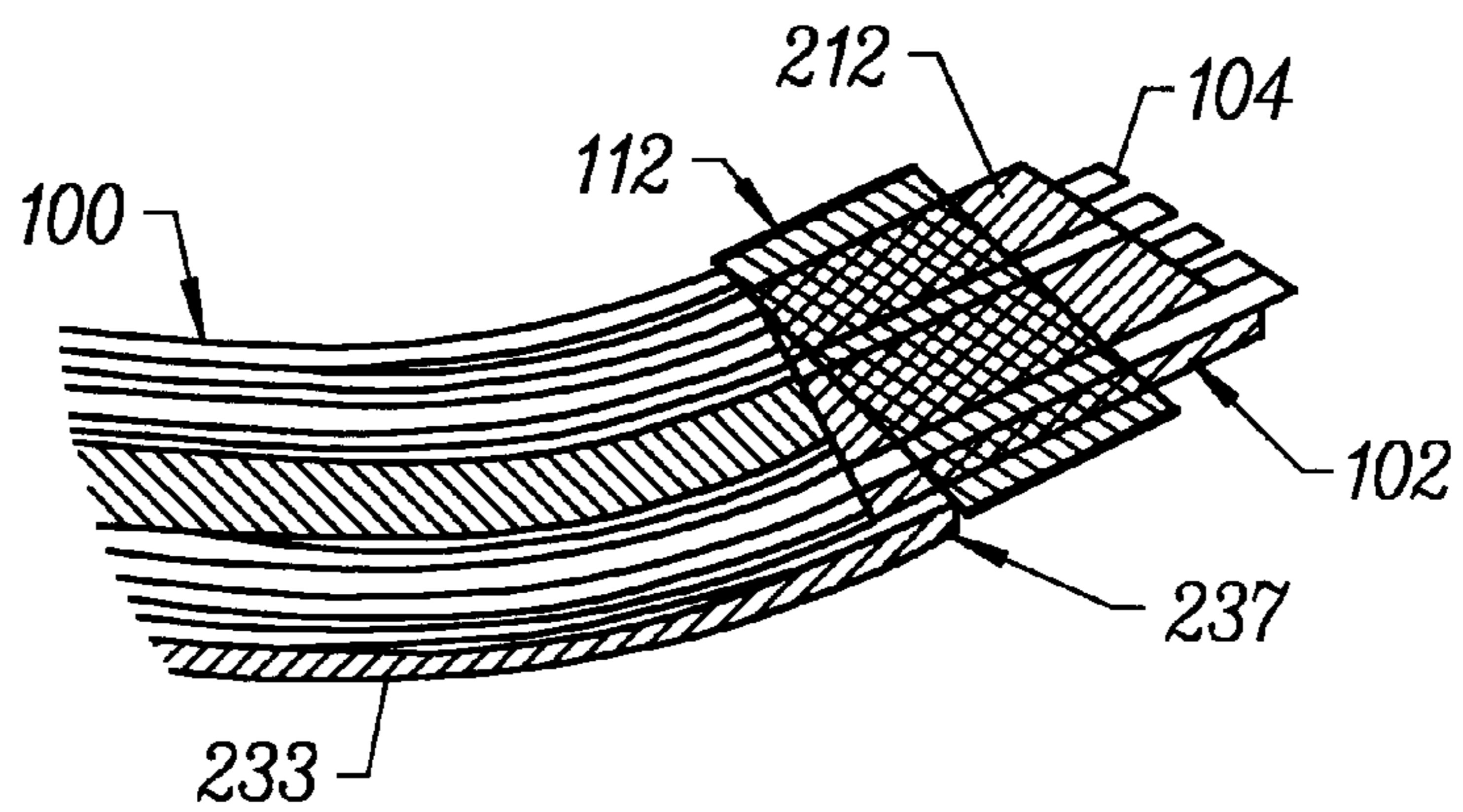
FIG. 6
