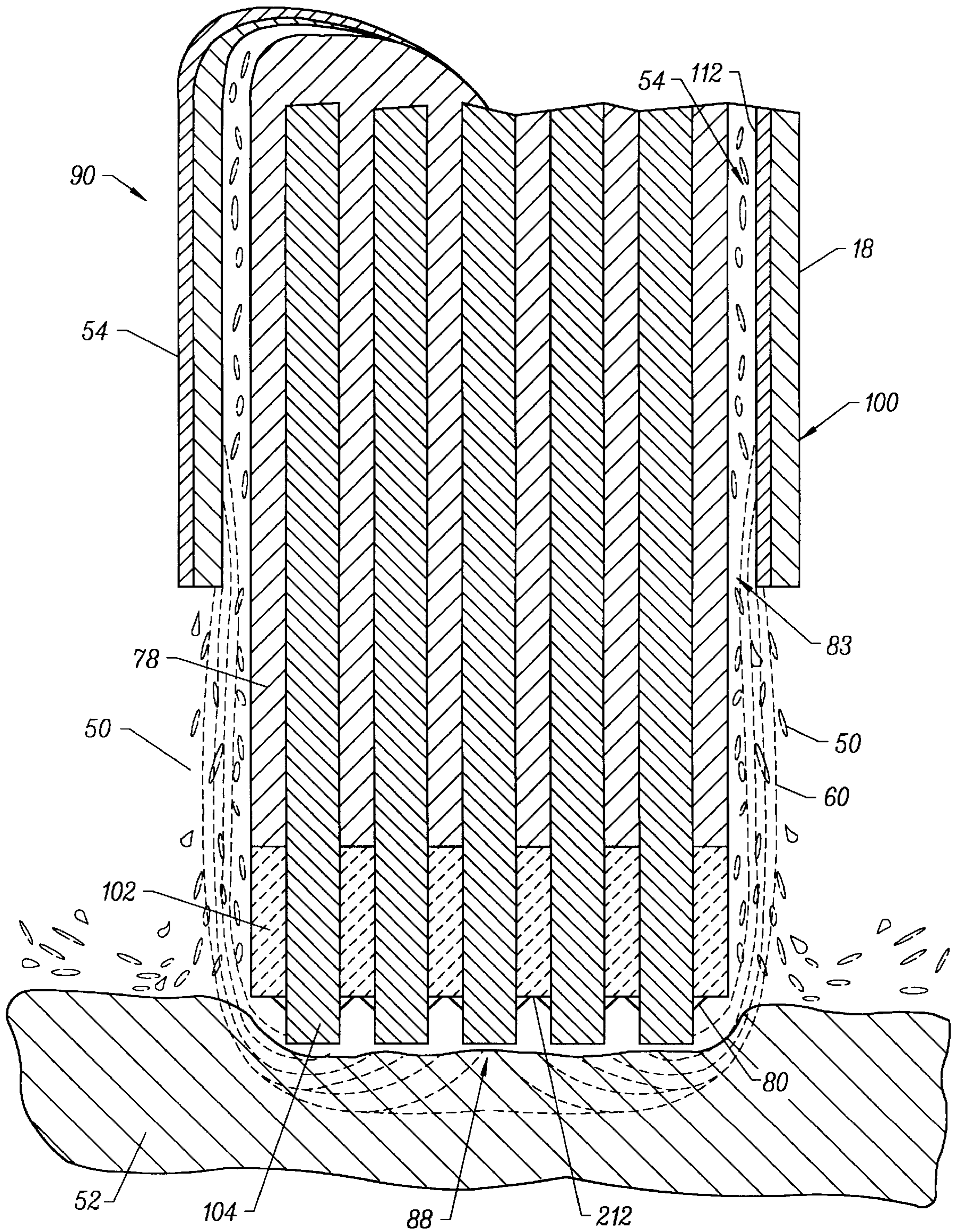
FIG. 12A
