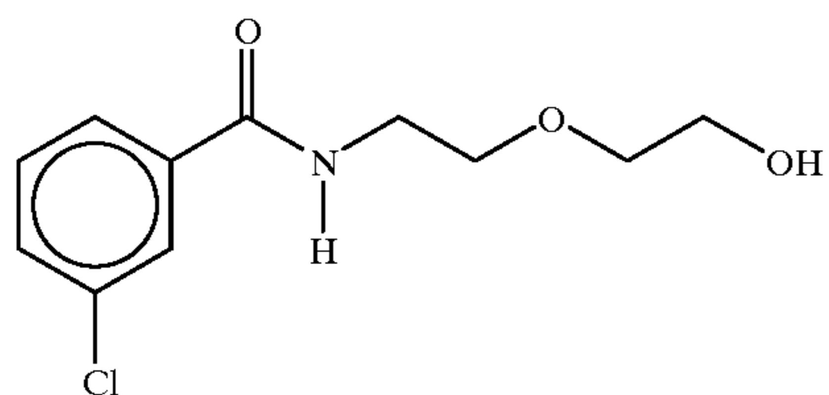
2-[2-N-(3-chlorobenzoyl)aminoethoxy]ethanol
