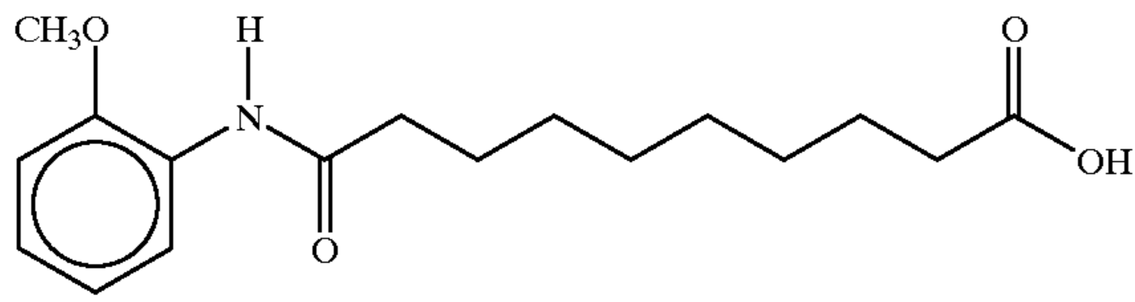
10-(N-2-Methoxyanilino)sebacic acid
