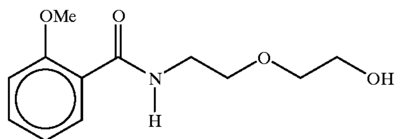
2-[2-N-(2-methoxybenzoyl)aminoethoxy]ethanol
