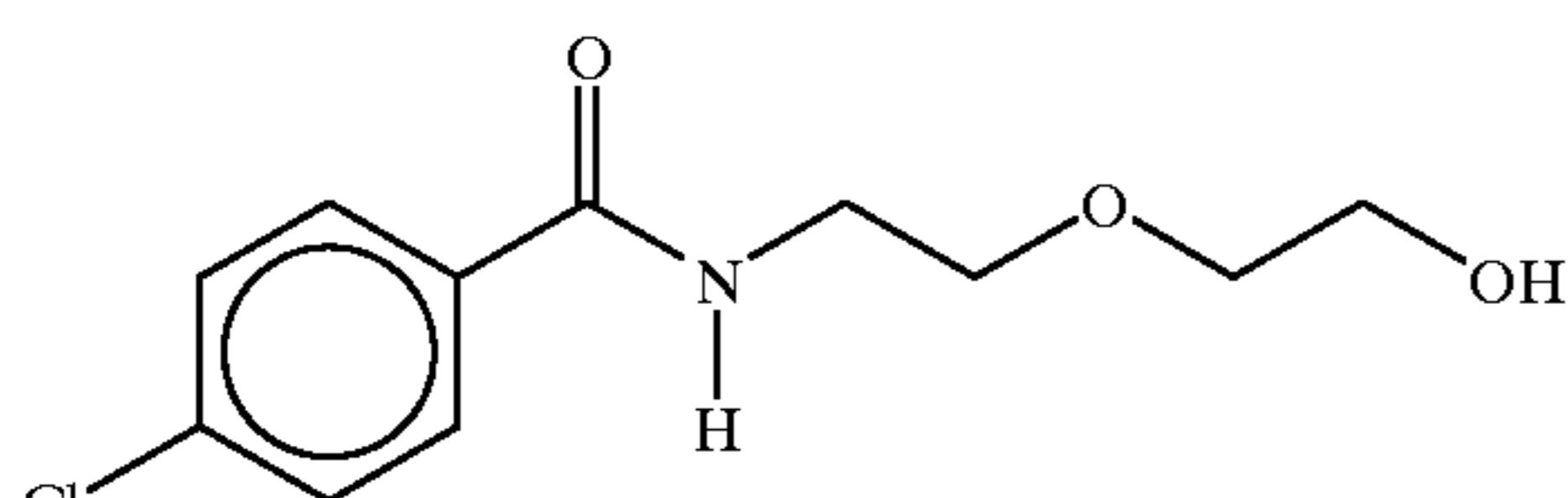
2-[2-N-(4-chlorobenzoyl)aminoethoxy]ethanol
