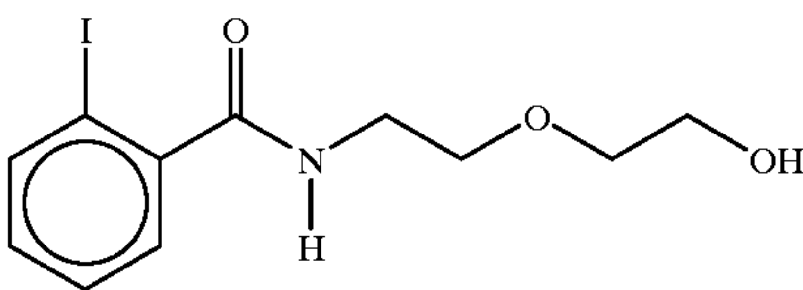
2-[N-(2-iodobenzoyl)aminoethoxy]ethanol
