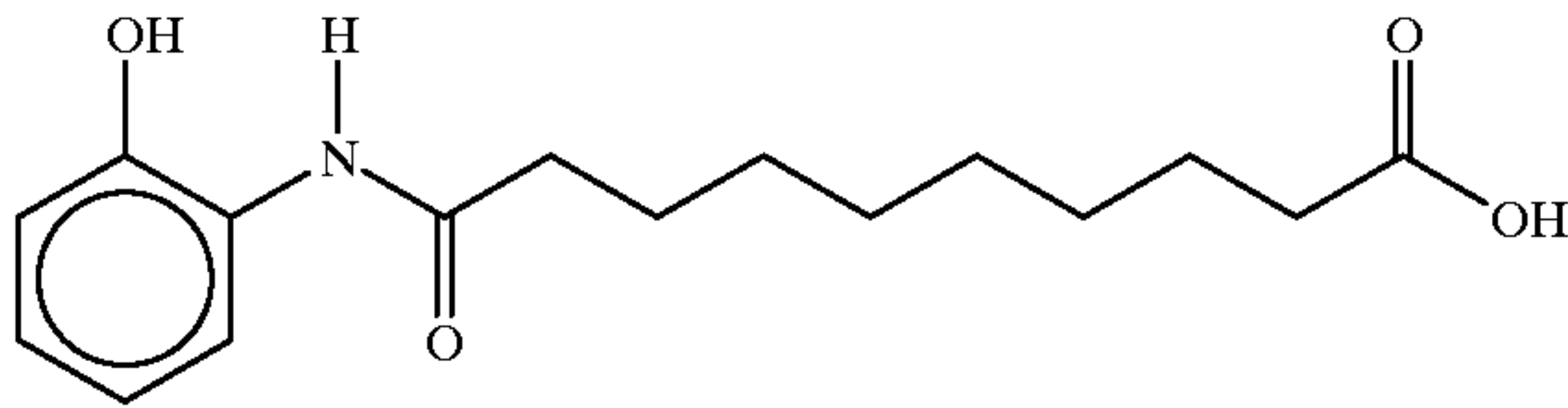
10-(N-2-Methoxyanilino)sebacic acid
