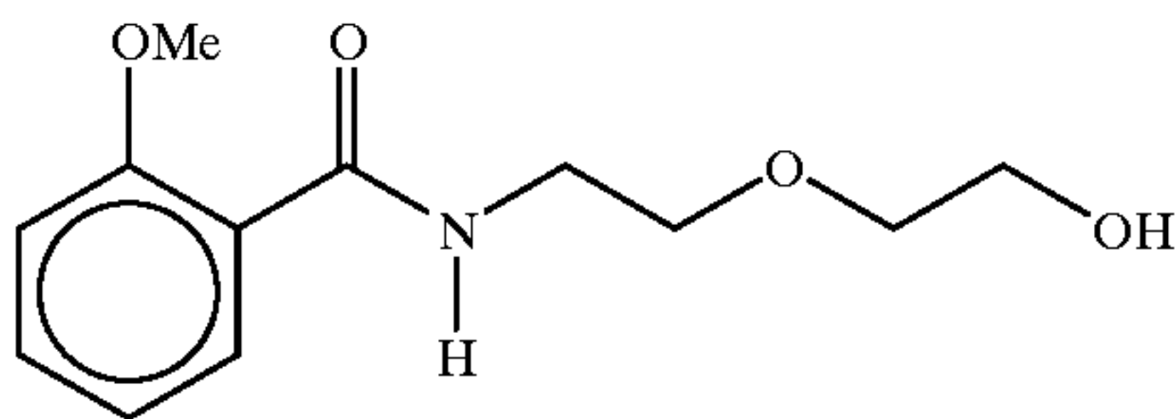
2-[2-N-(2-methoxybenzoyl)aminoethoxy]ethanol
