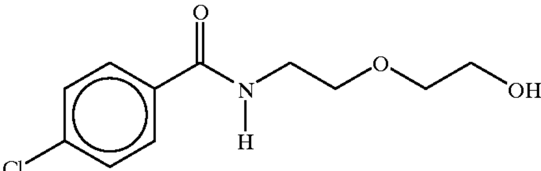
2-[2-N-(4-chlorobenzoyl)aminoethoxy]ethanol
