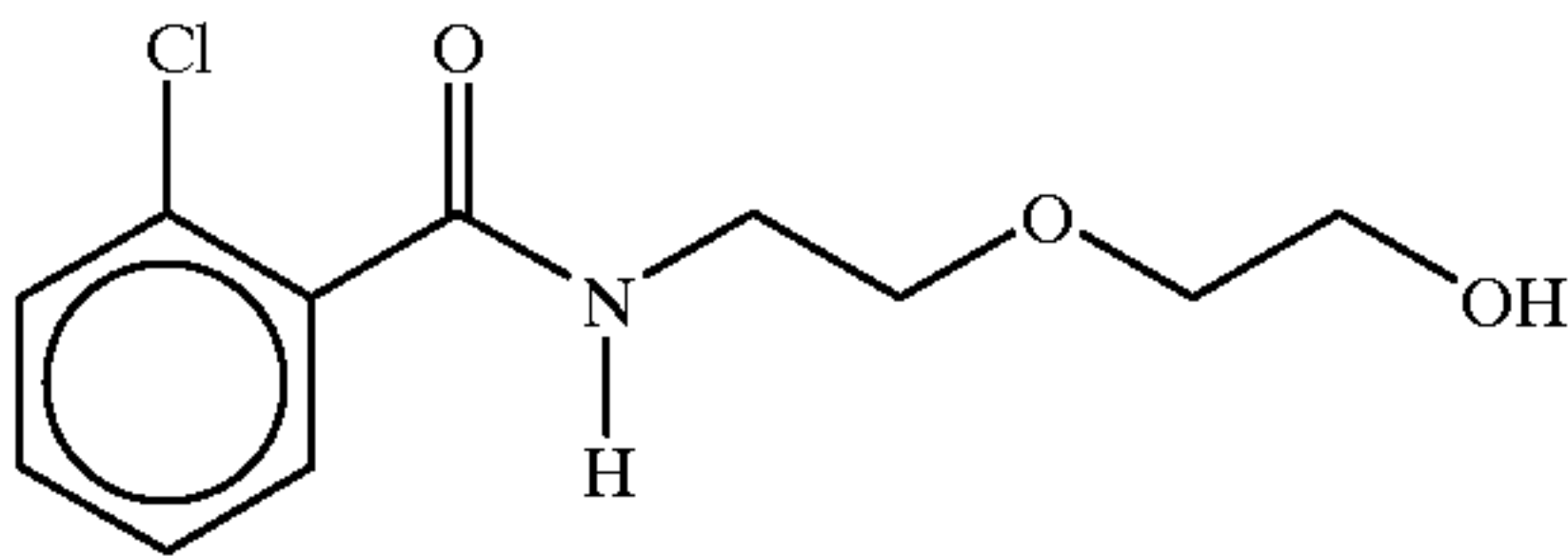
2-[2-N-(2-chlorobenzoyl)aminoethoxy]ethanol
