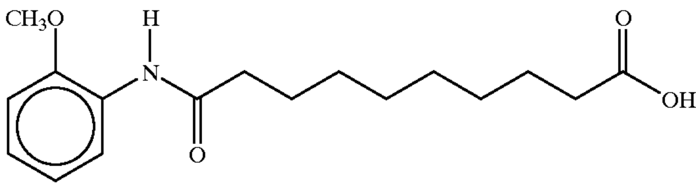
10-(N-2-Methoxyanilino)sebacic acid
