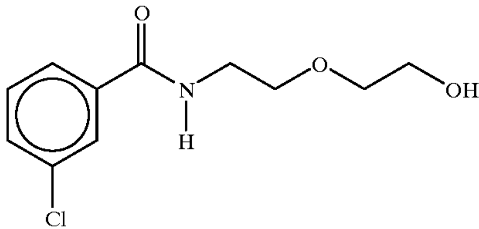
2-[2-N-(3-chlorobenzoyl)aminoethoxy]ethanol
