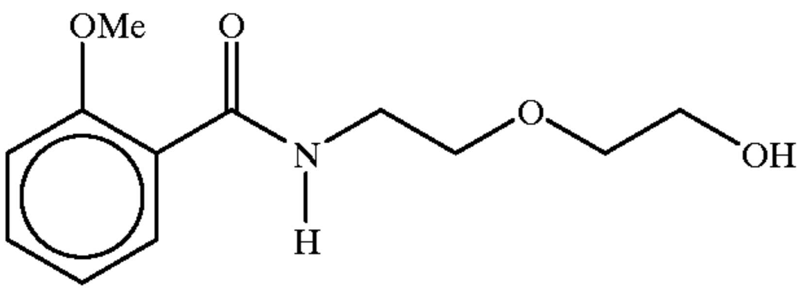
2-[2-N-(2-methoxybenzoyl)aminoethoxy]ethanol
