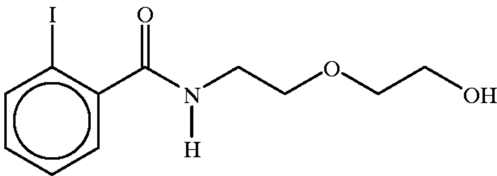
2-[N-(2-iodobenzoyl)aminoethoxy]ethanol
