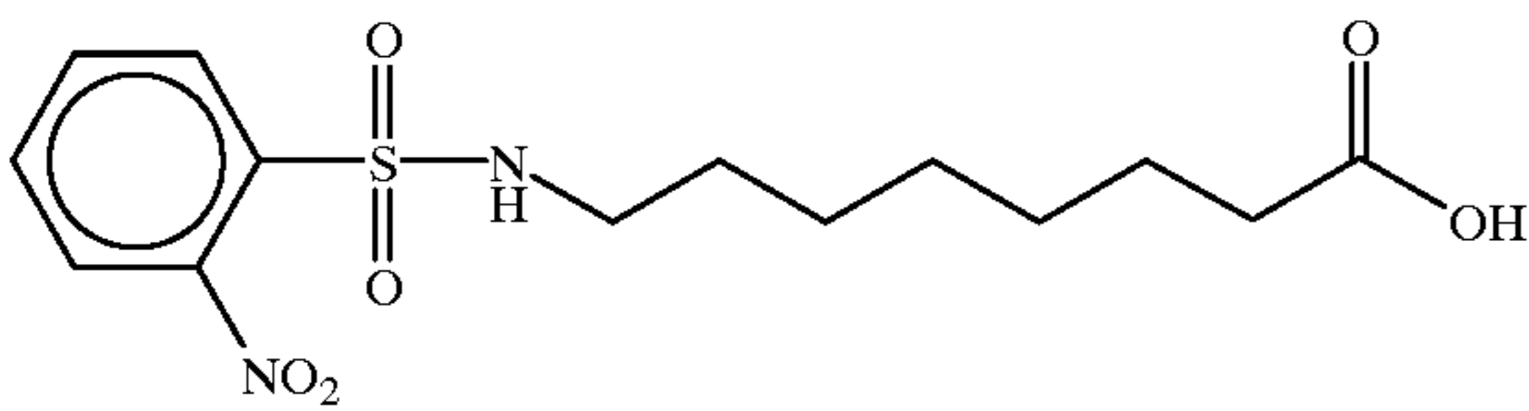
8-(2-nitrobenzenesulfonyl)aminocaprylic acid
