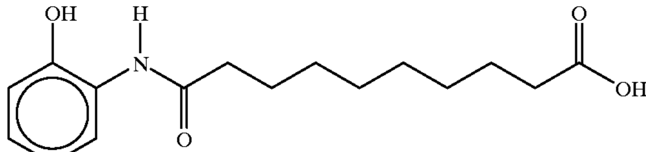
10-(N-2-Methoxyanilino)sebacic acid
