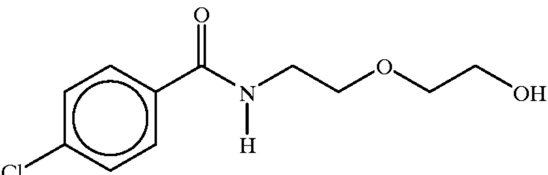
2-[2-N-(4-chlorobenzoyl)aminoethoxy]ethanol
