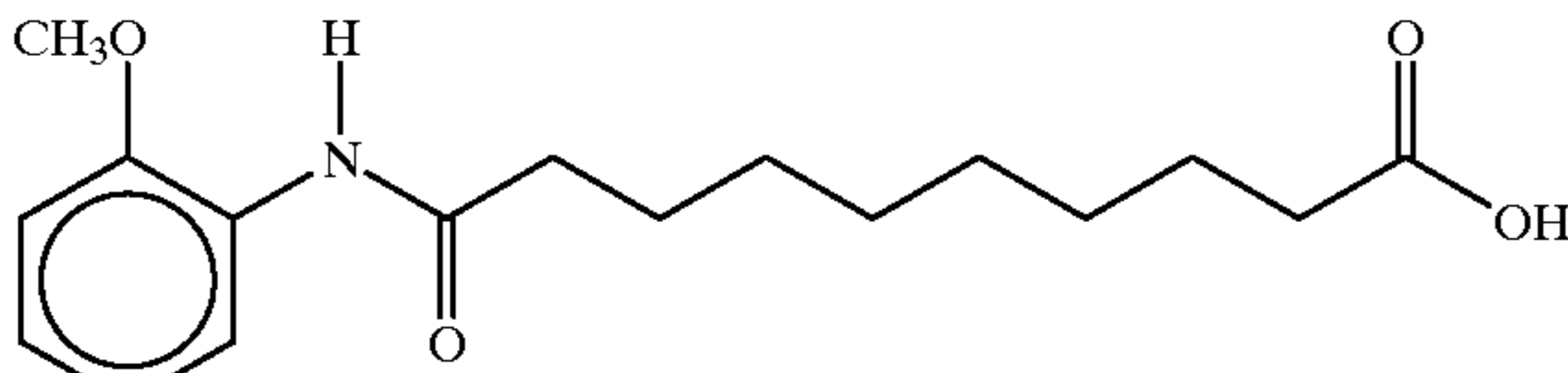
10-(N-2-Methoxyanilino)sebacic acid
