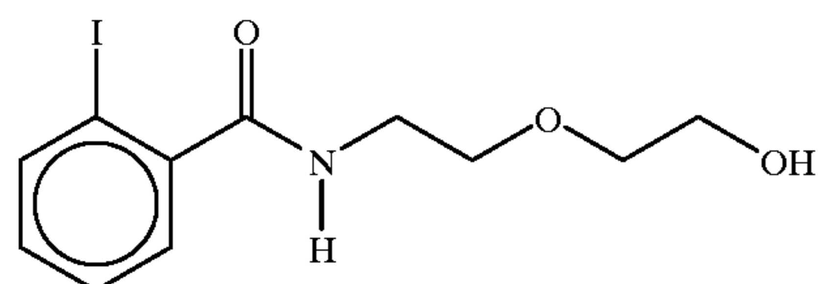
2-[N-(2-iodobenzoyl)aminoethoxy]ethanol
