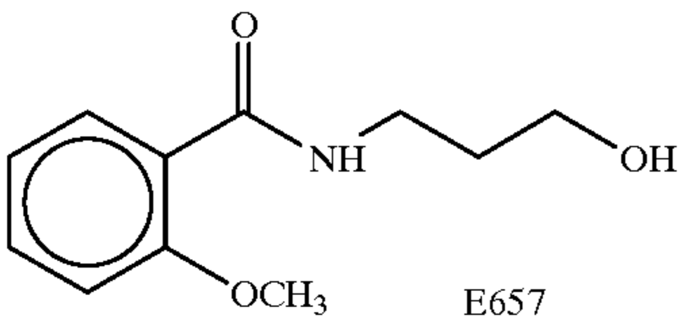
3-(2-methoxybenzoylamino)-1-propanol
