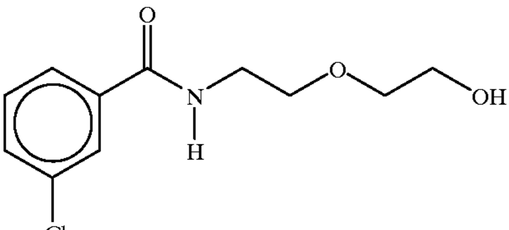
2-[2-N-(3-chlorobenzoyl)aminoethoxy]ethanol
