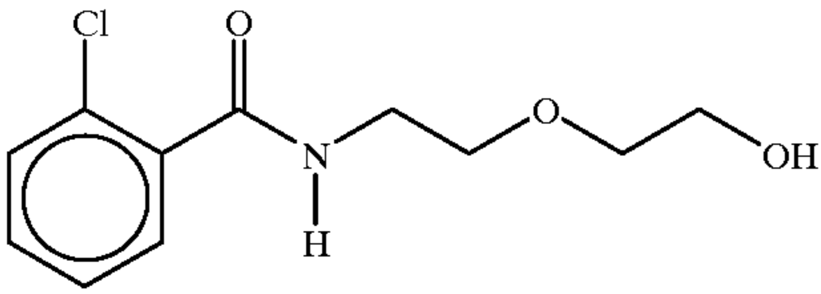
2-[2-N-(2-chlorobenzoyl)aminoethoxy]ethanol
