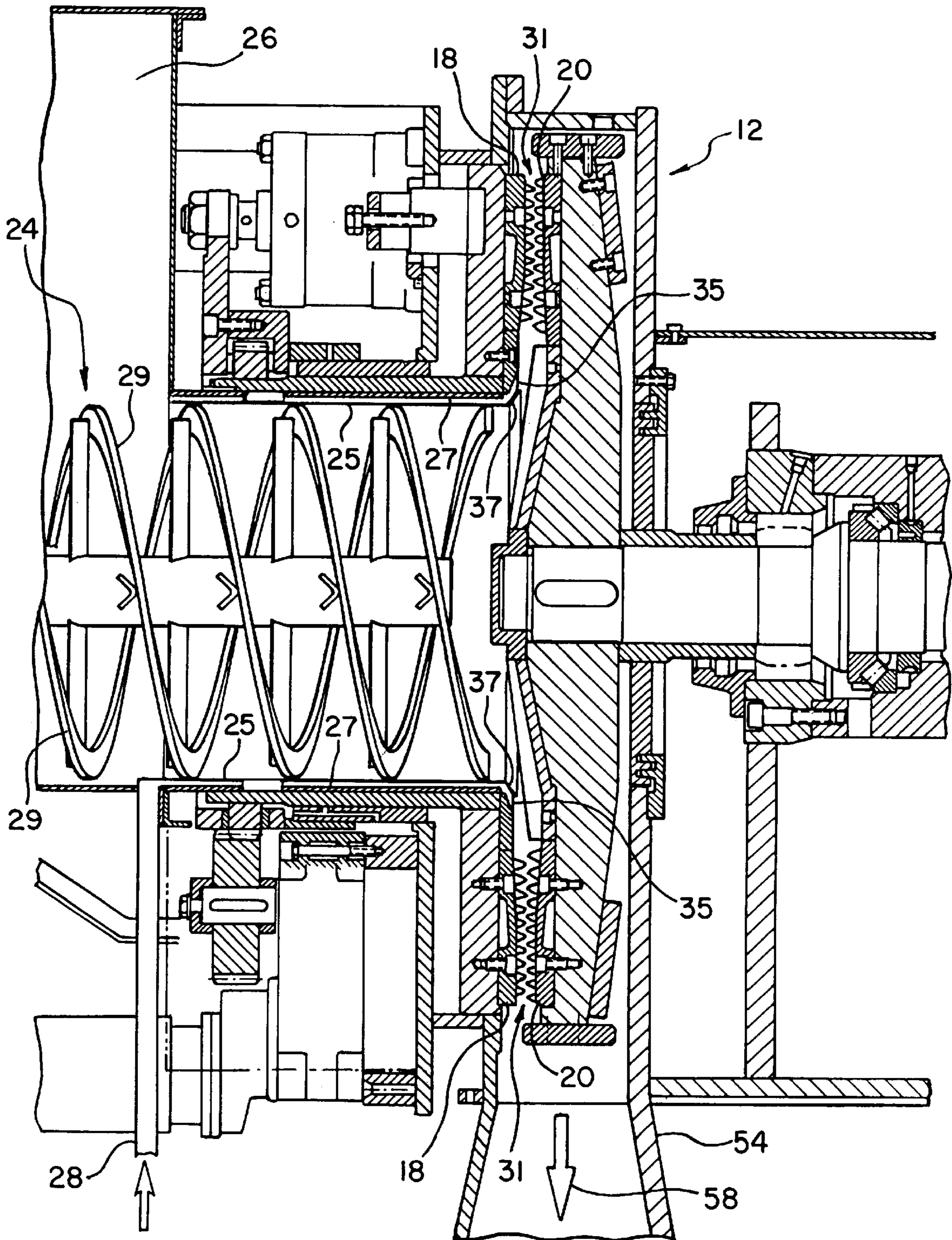
FIG. 1B
