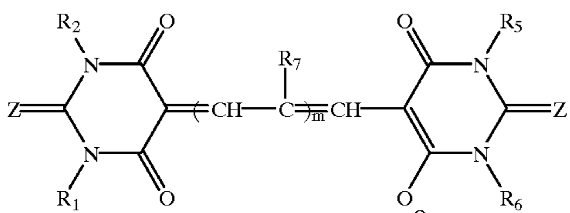
OXONOL
