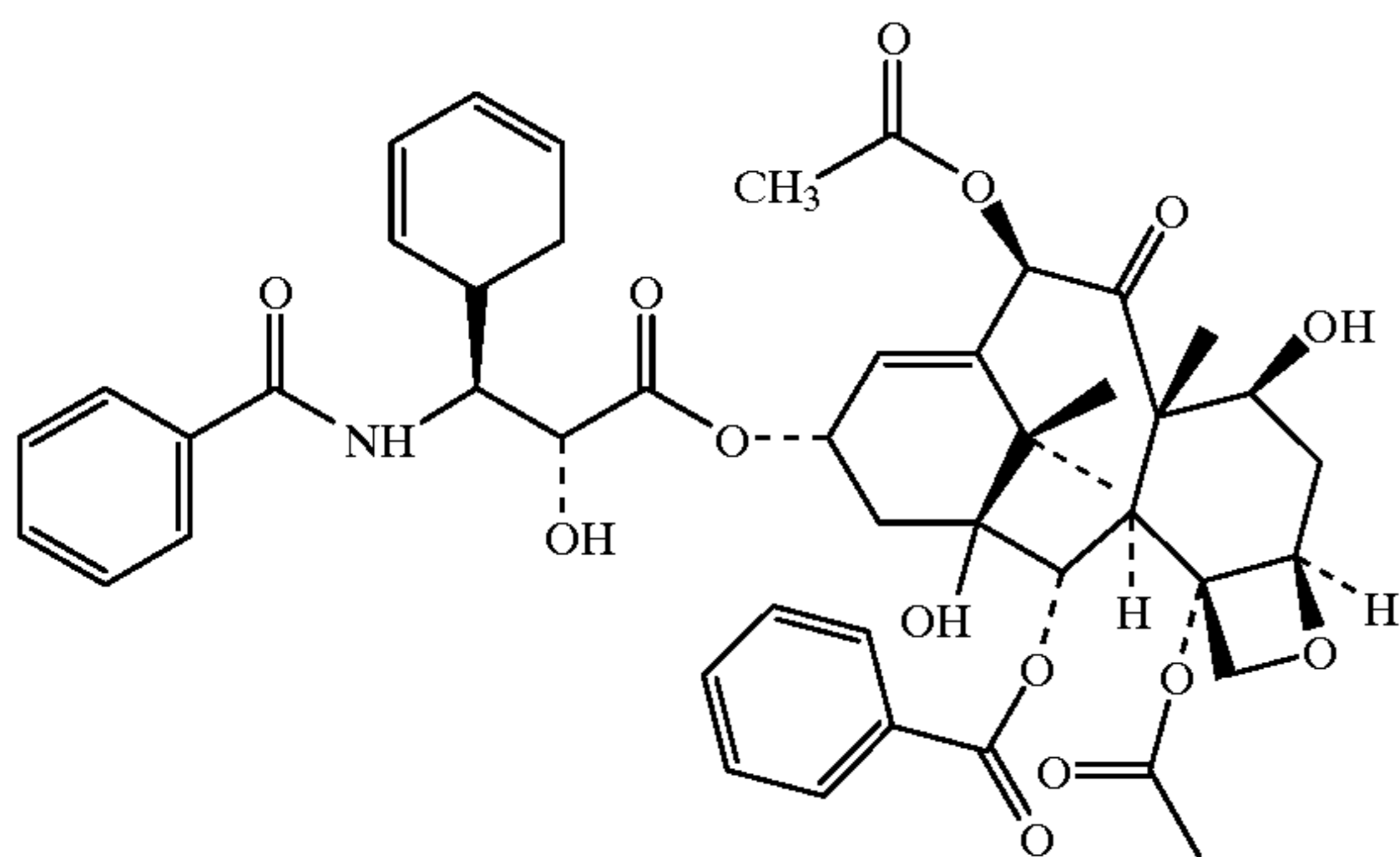
Taxol
