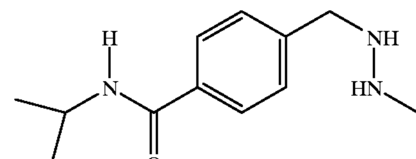
Procarbazine
