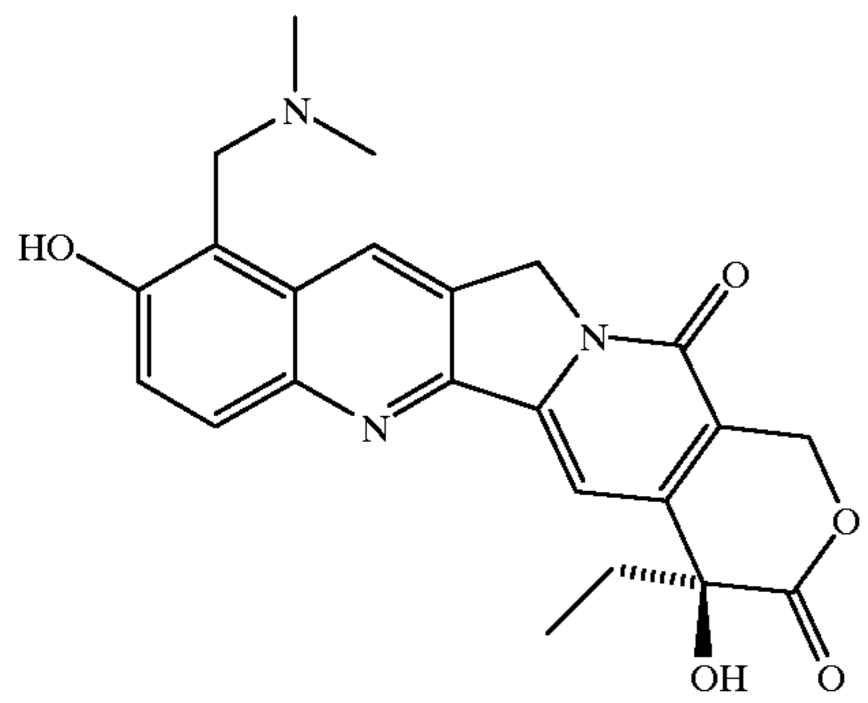
Topotecan
