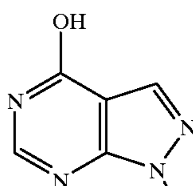
Allopurinol
