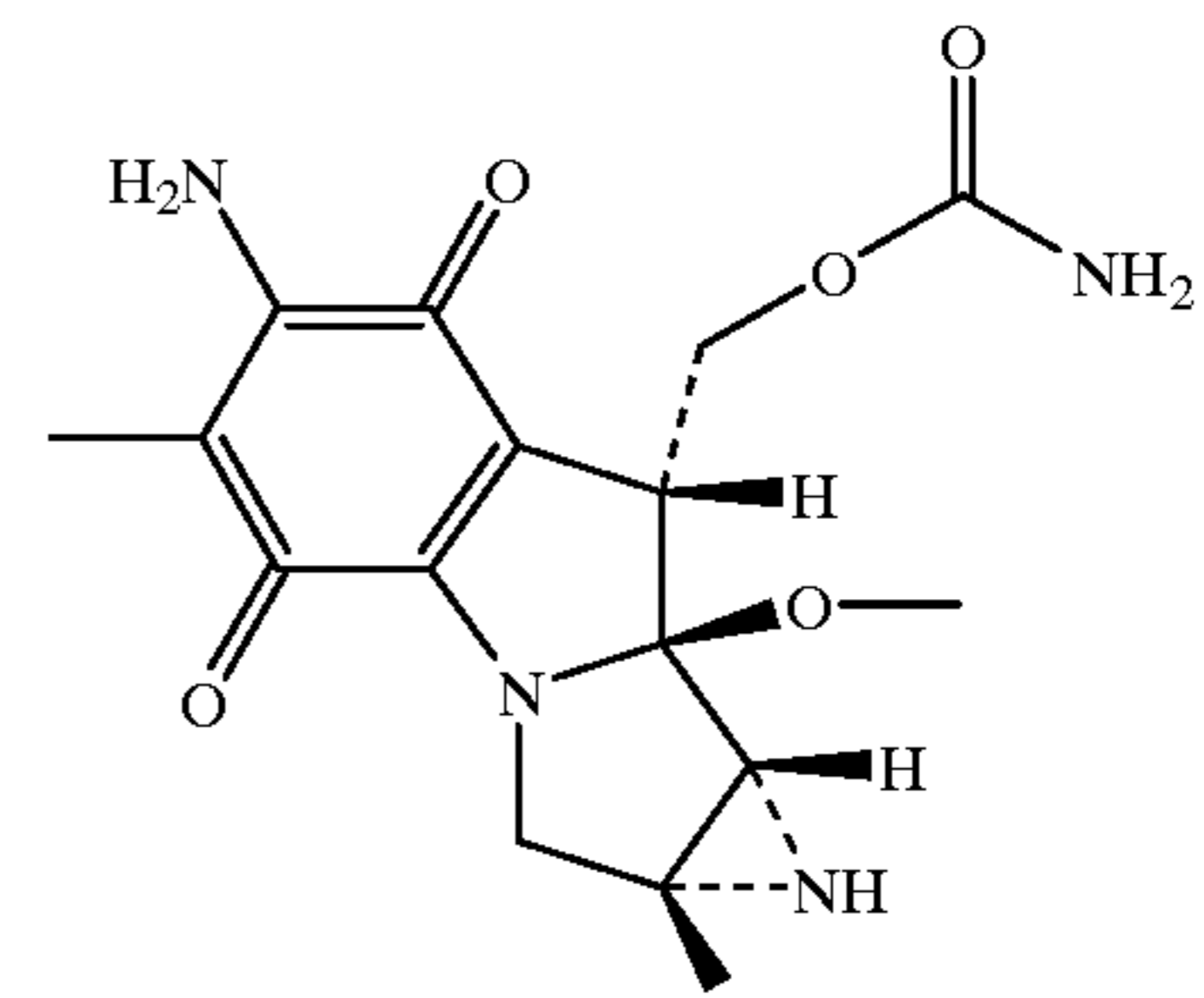
Mitomycin
