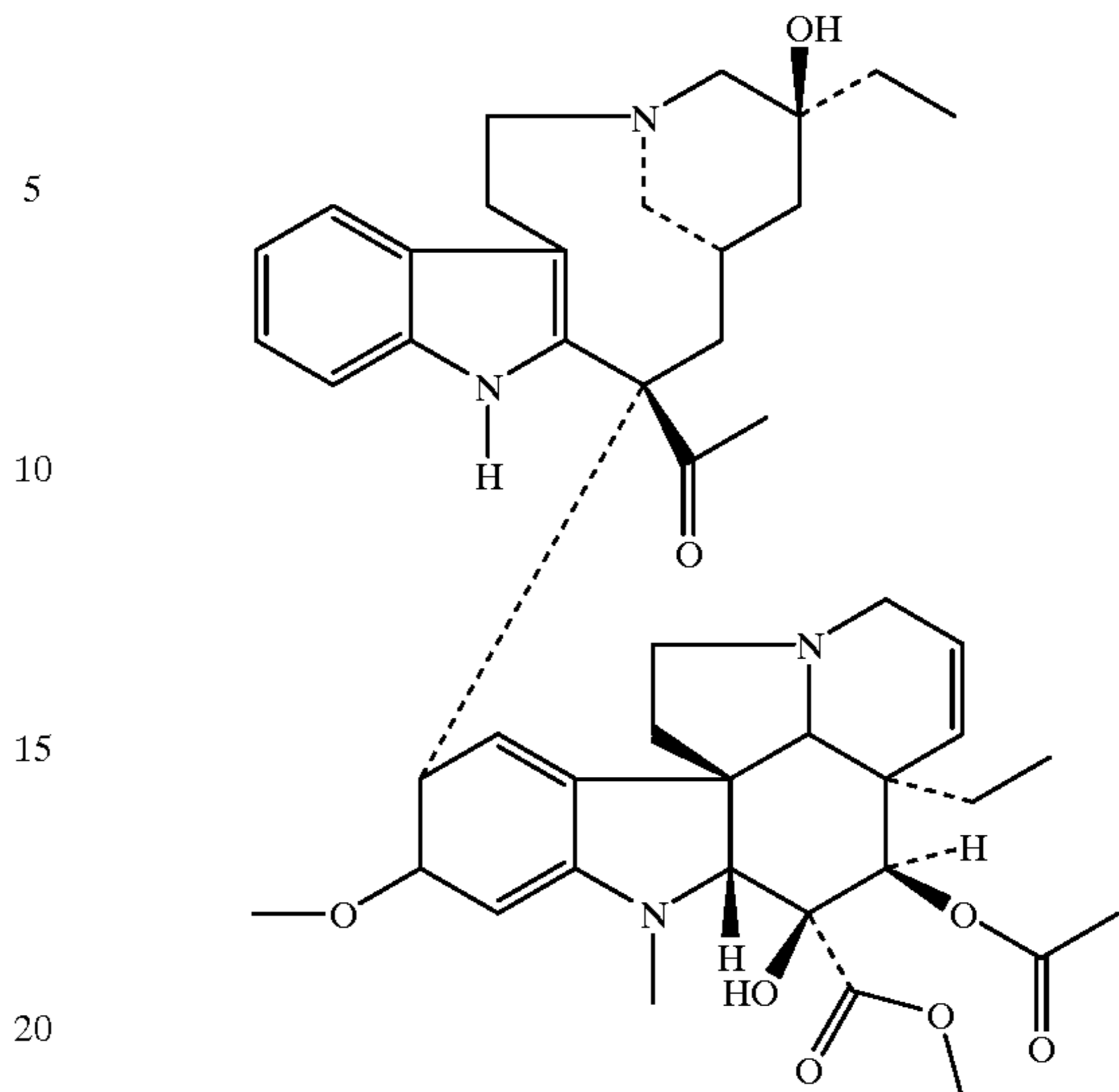
Vinblastine
