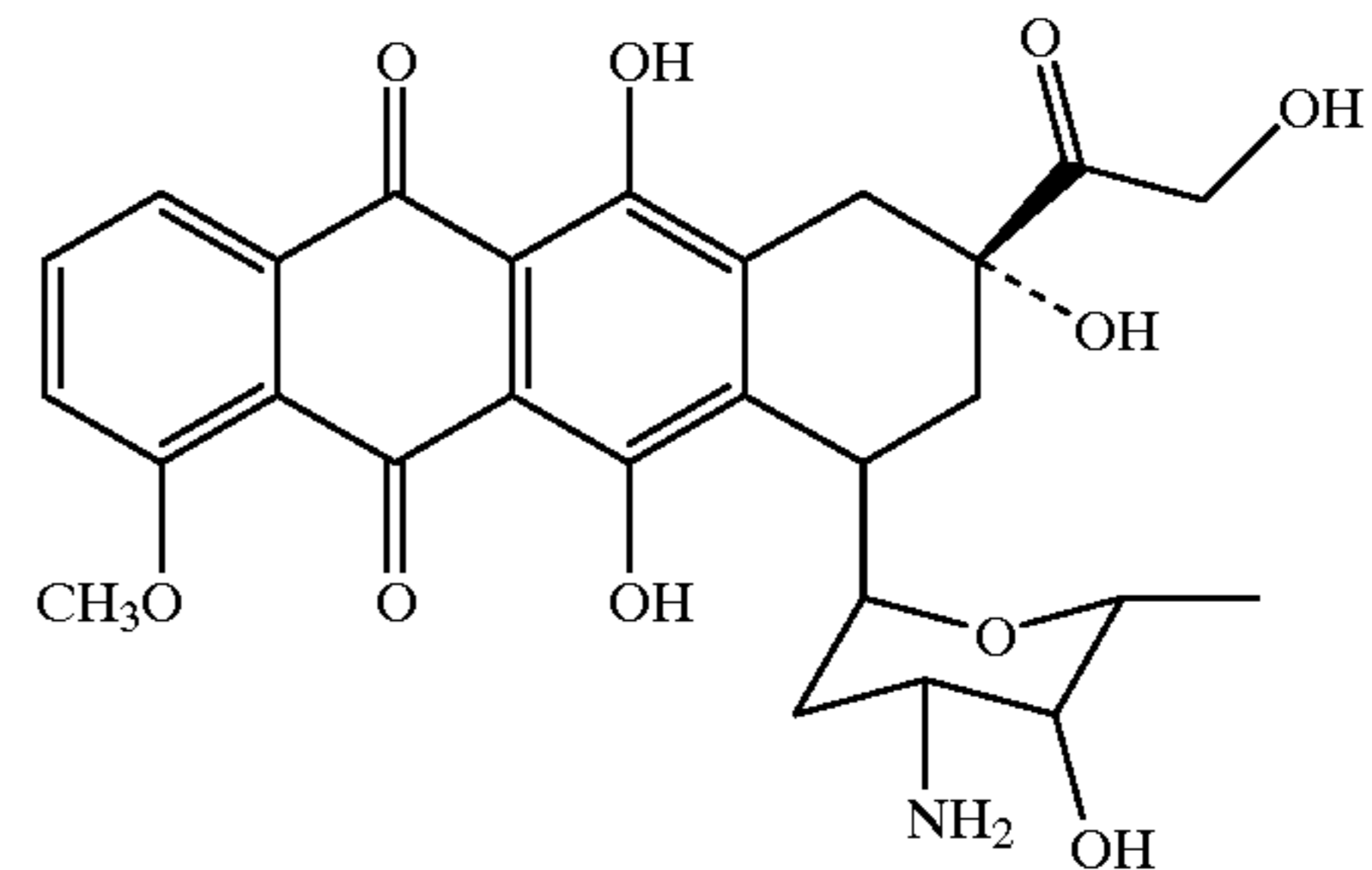
Doxorubicin
