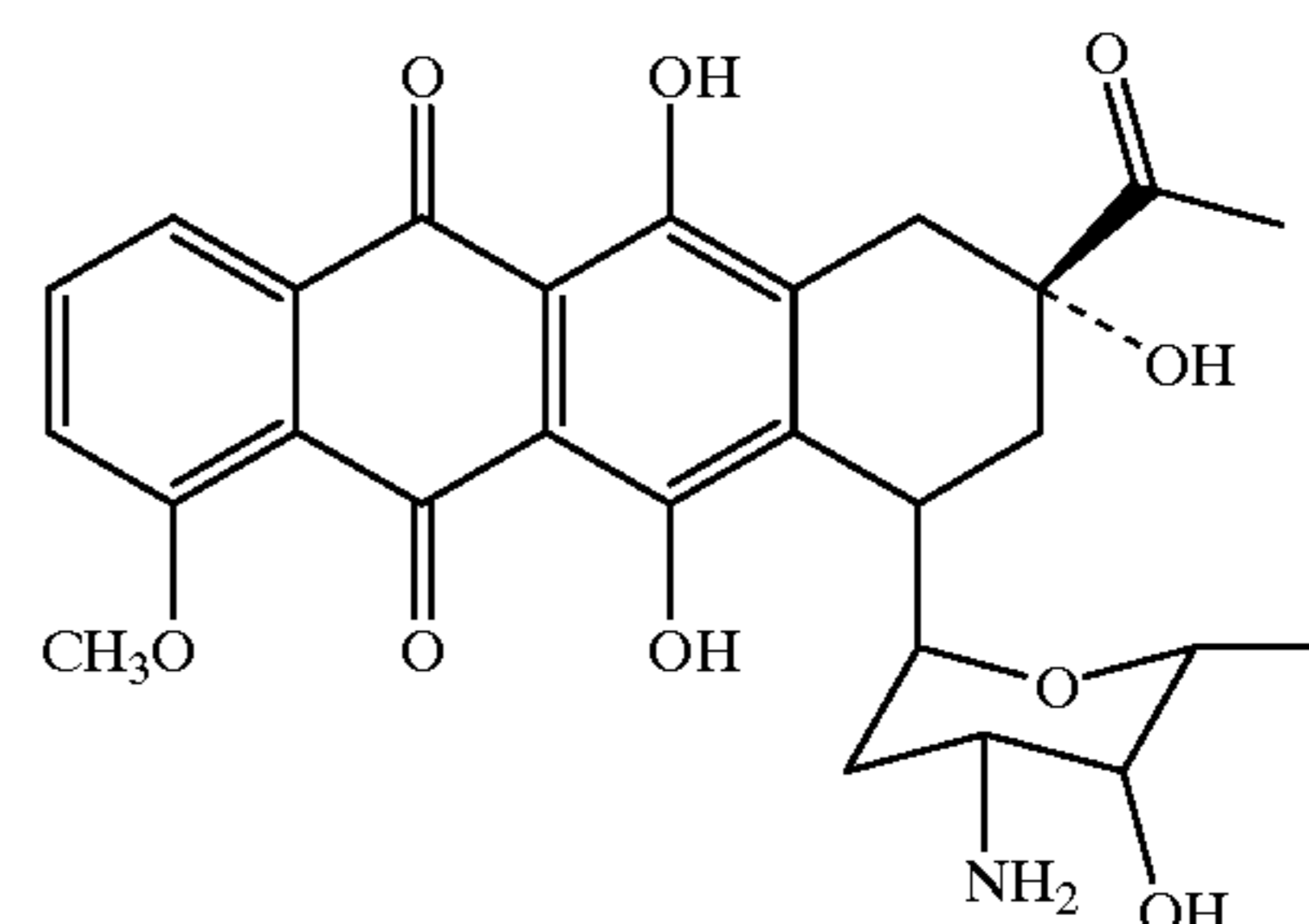
Daunorubicin
