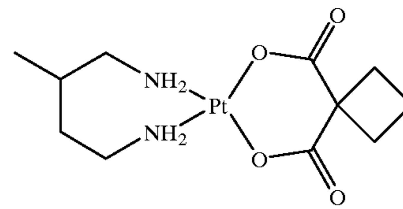
CI-973
