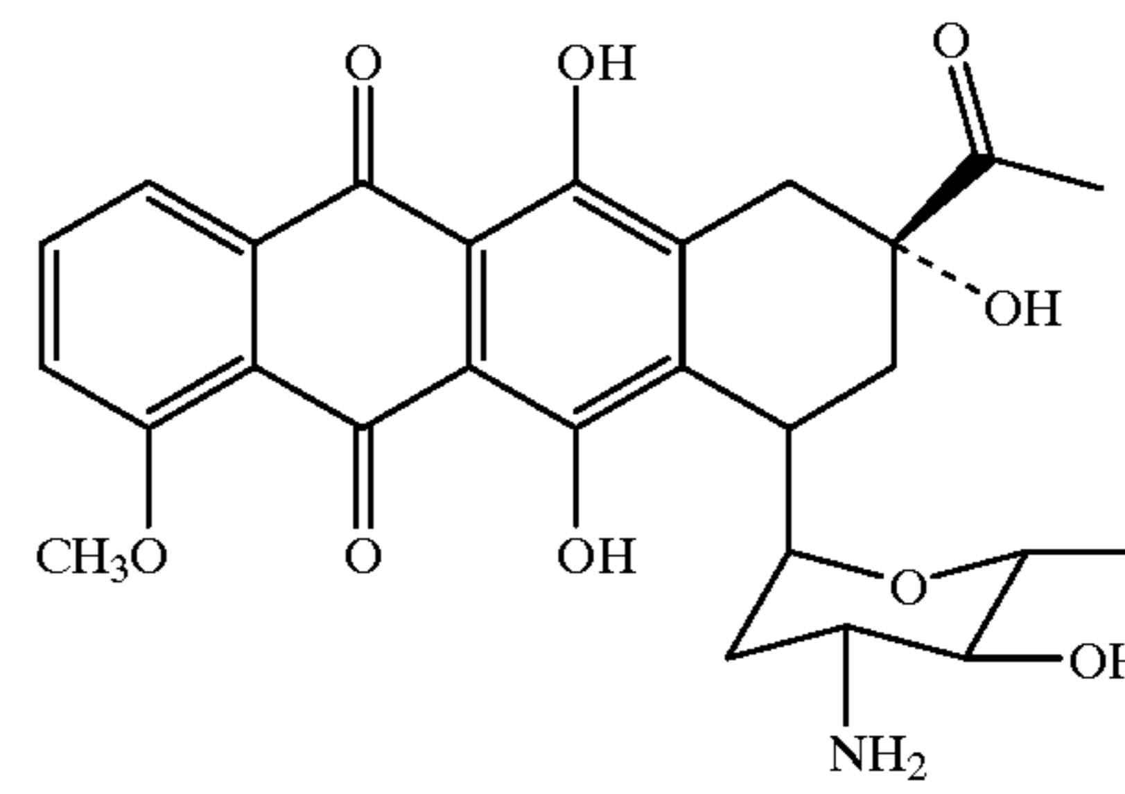
Epirubicin
