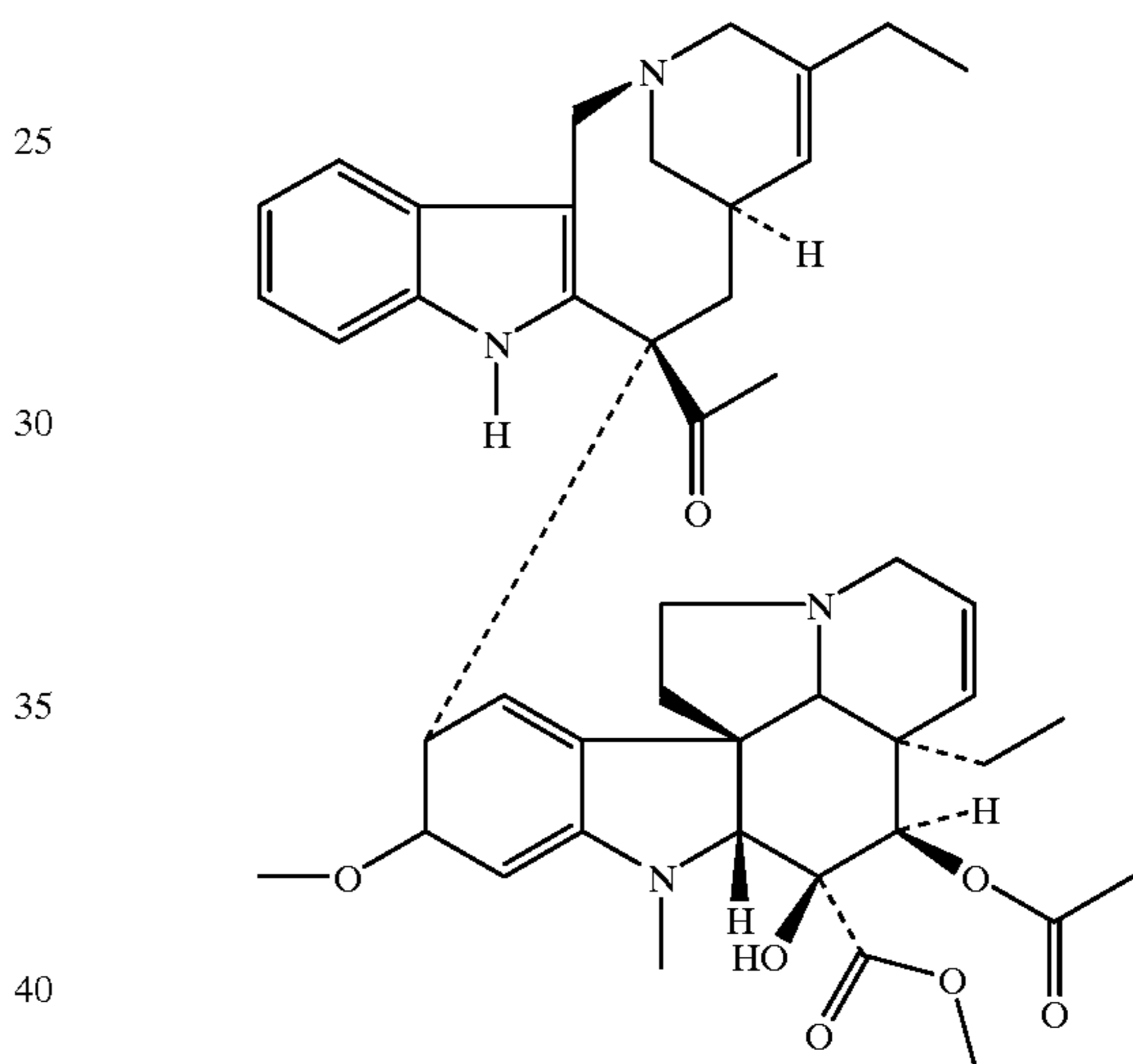
Vinorelbine
