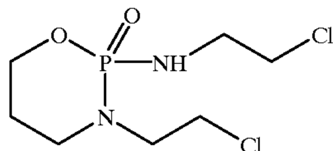
Ifosfamide
