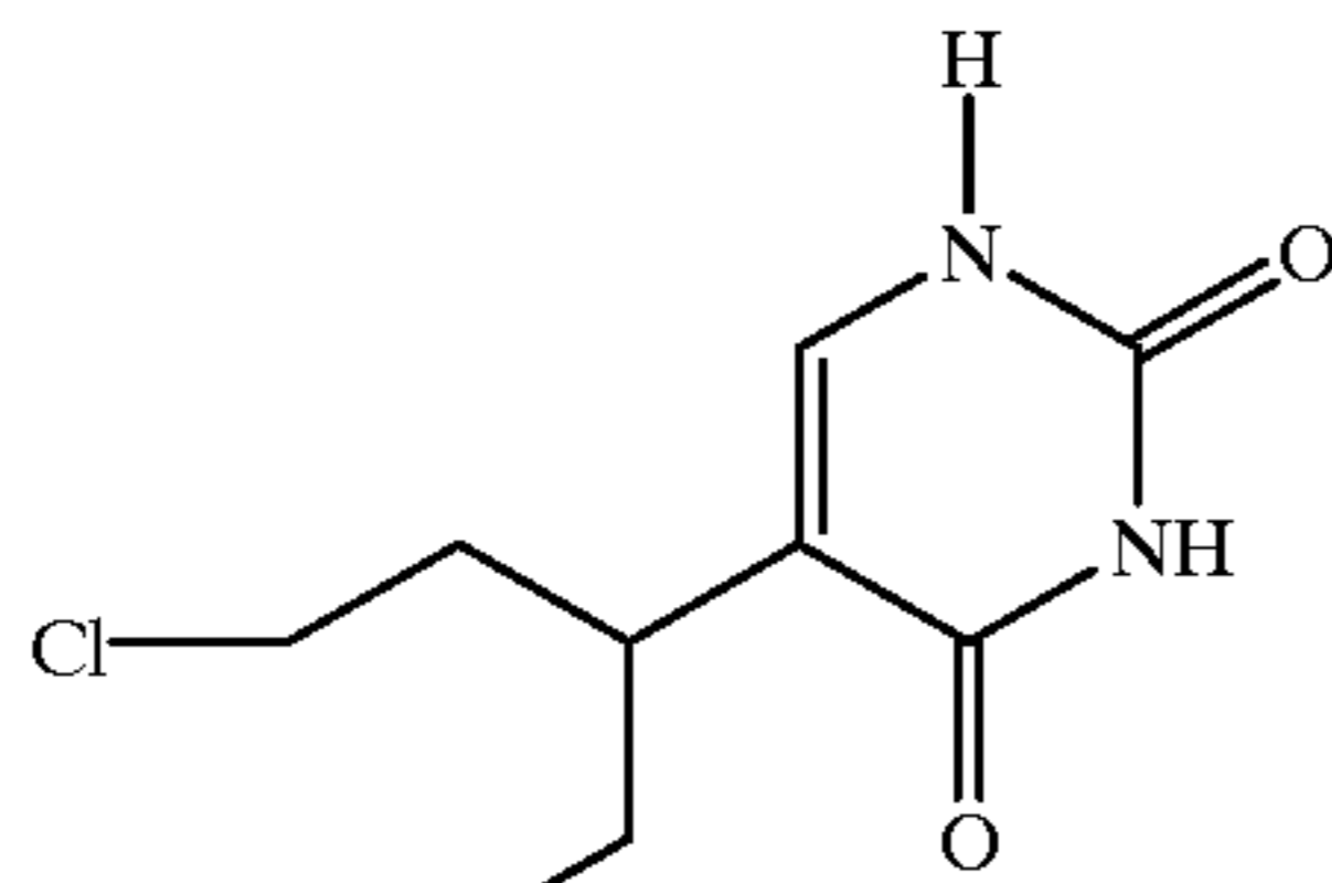
Uracil Mustard
