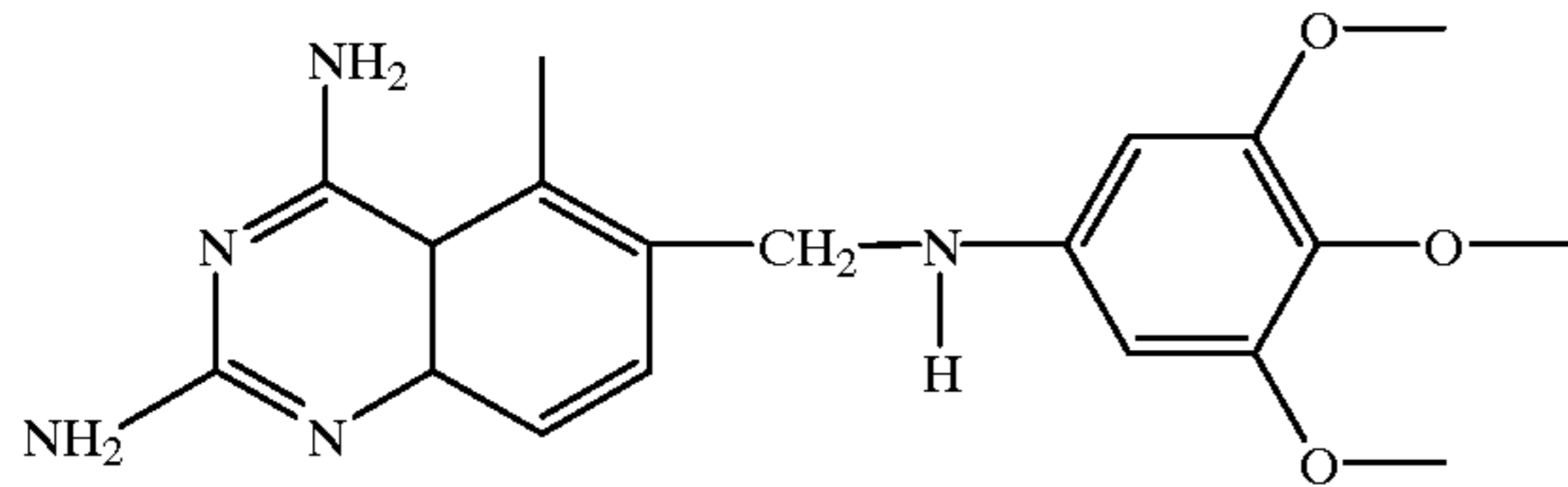
Trimetrexate
