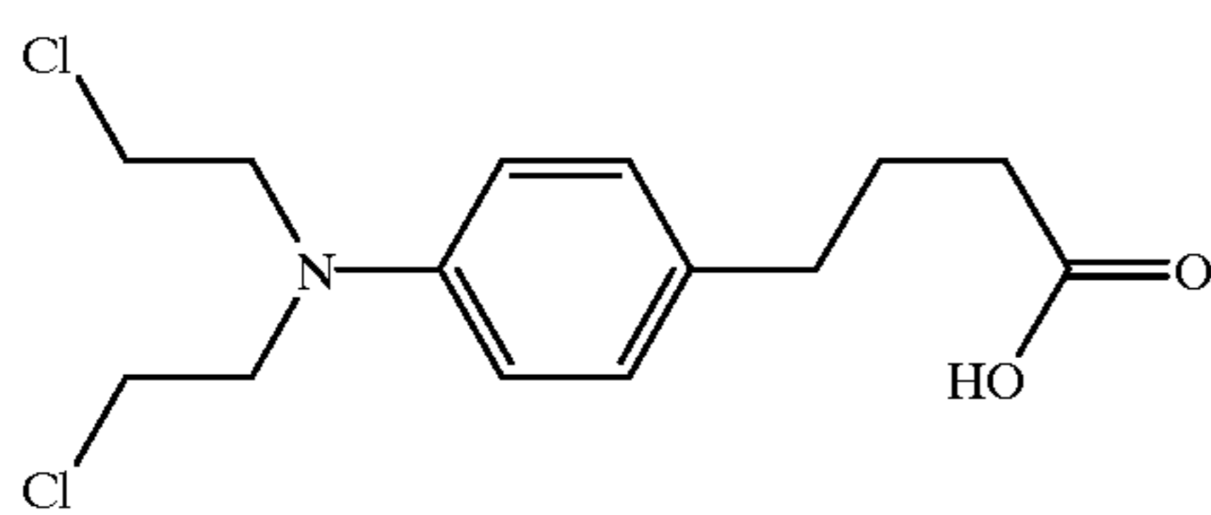
Chlorambucil
