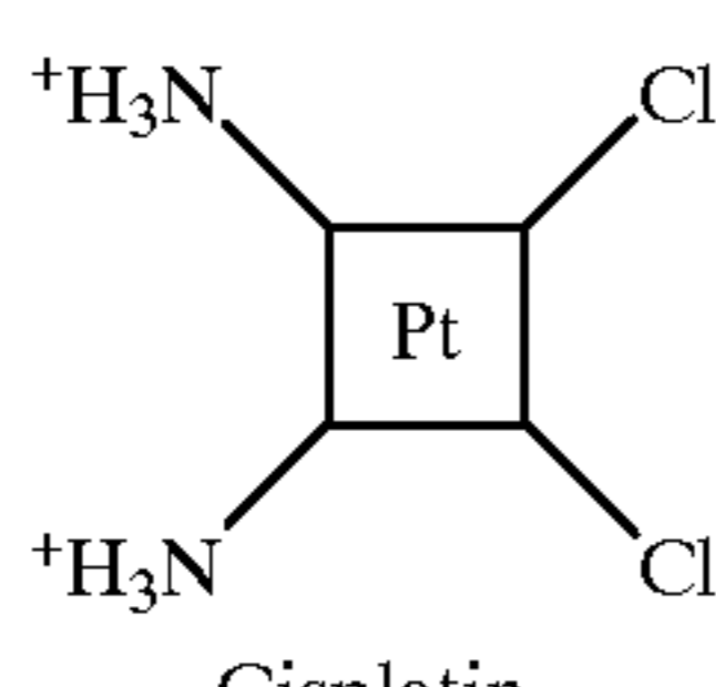
Cisplatin
