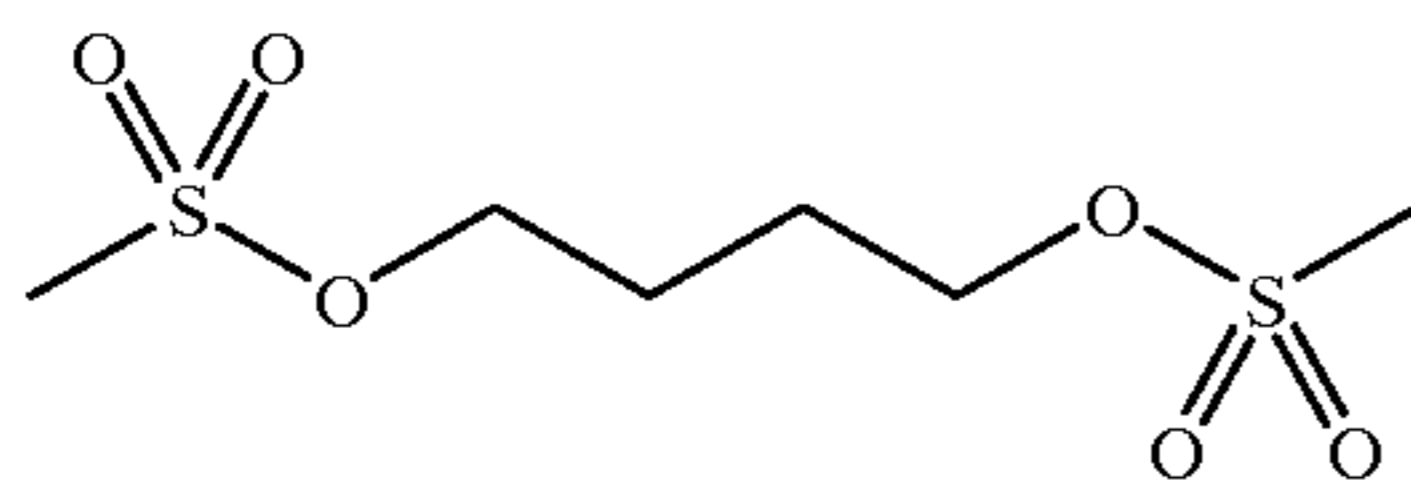
Busulfan
