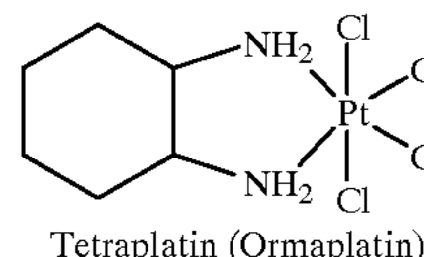
Tetraplatin (Ormaplatin)
