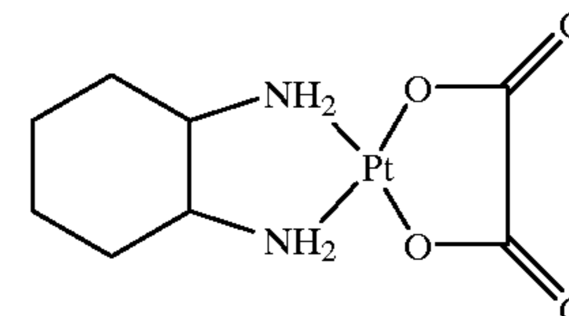
Oxaliplatin
