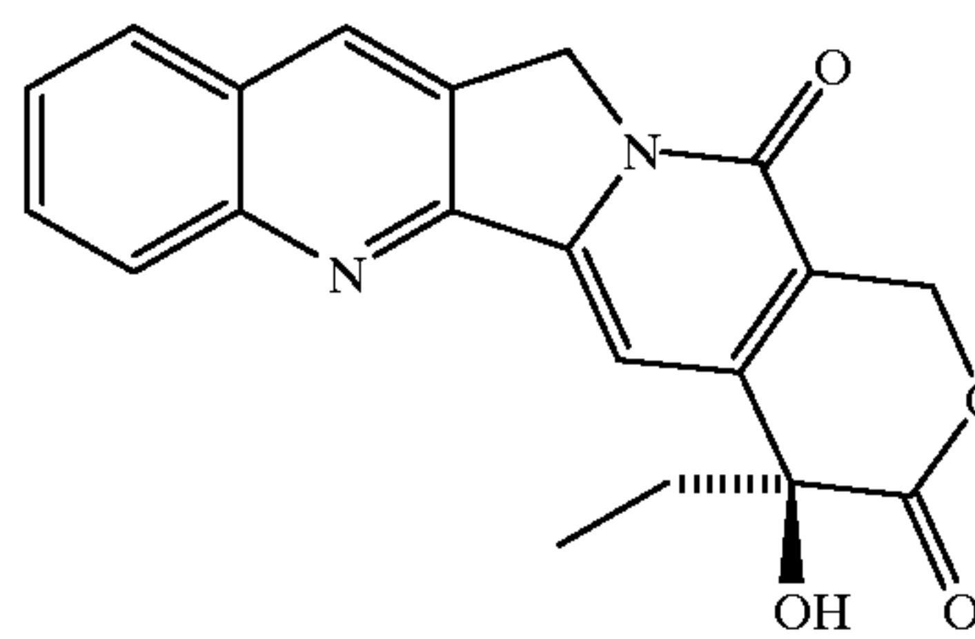
Camptothecin
