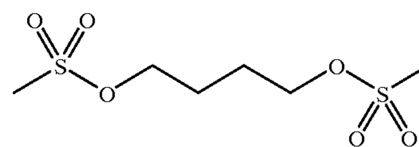
Busulfan
