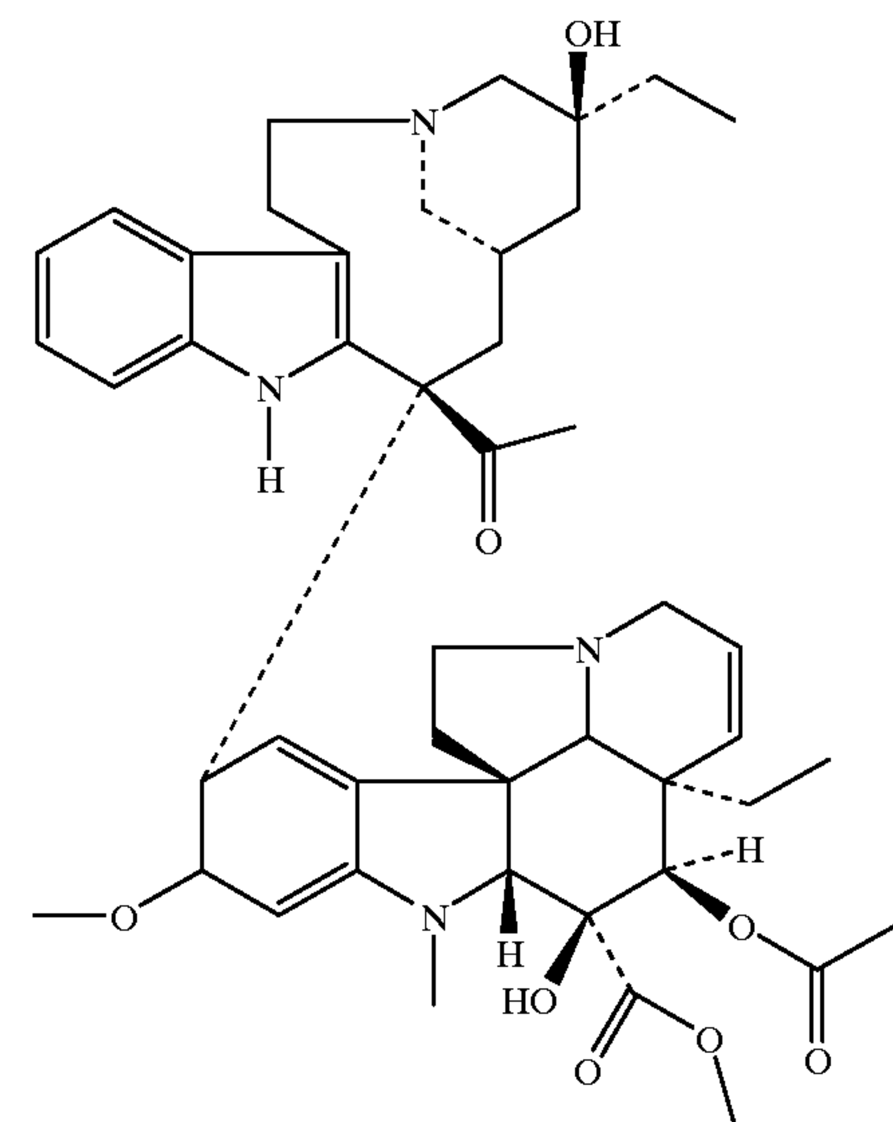
Vinblastine
