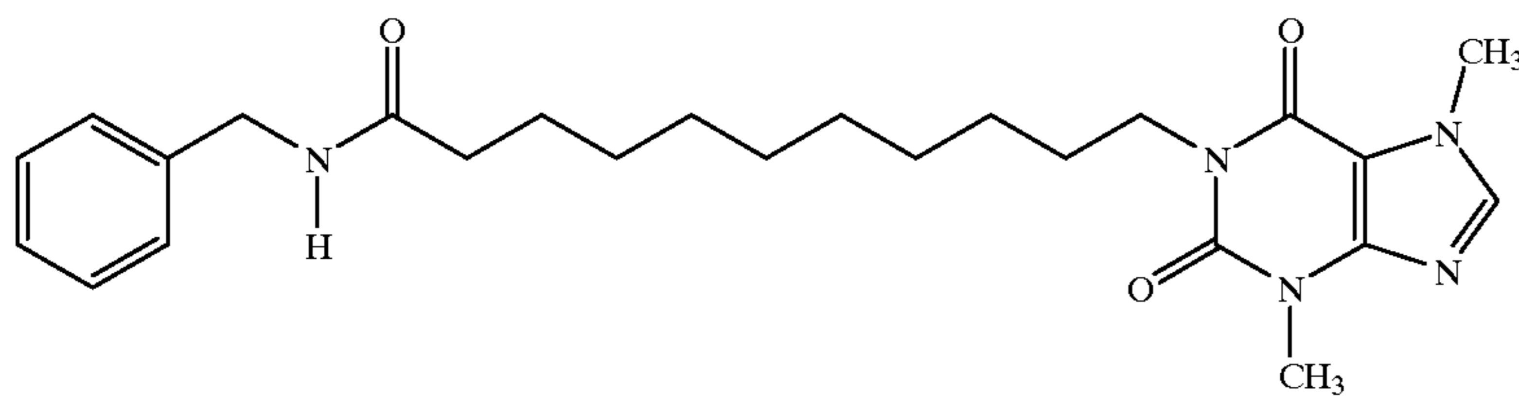
1-[N-(Benzyl)-11-yl-undecanoamide]-3,7-dimethylxanthine
