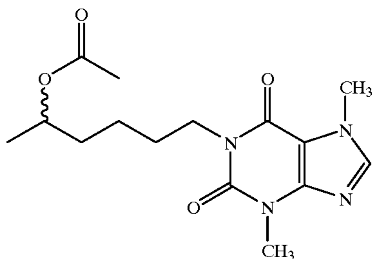
1-(5-Acetoxyhexyl)-3,7-dimethylxanthine
