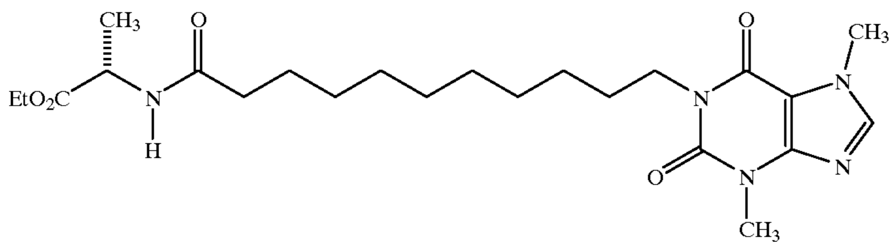
1-[11-(1-Ethoxycarbonylpropylamino)-11-oxoundecyl]-3,7-dimethylxanthine
