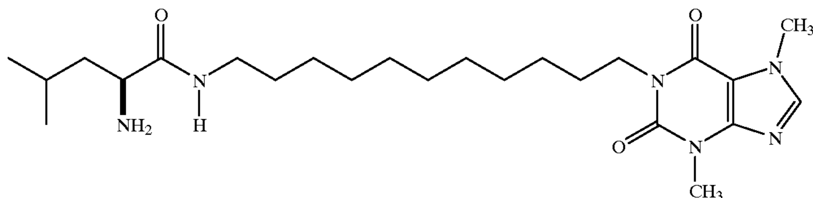
1-[11-(2-Amino-4-methylpentanamido)undecyl]-3, 7-dimethylxanthine
