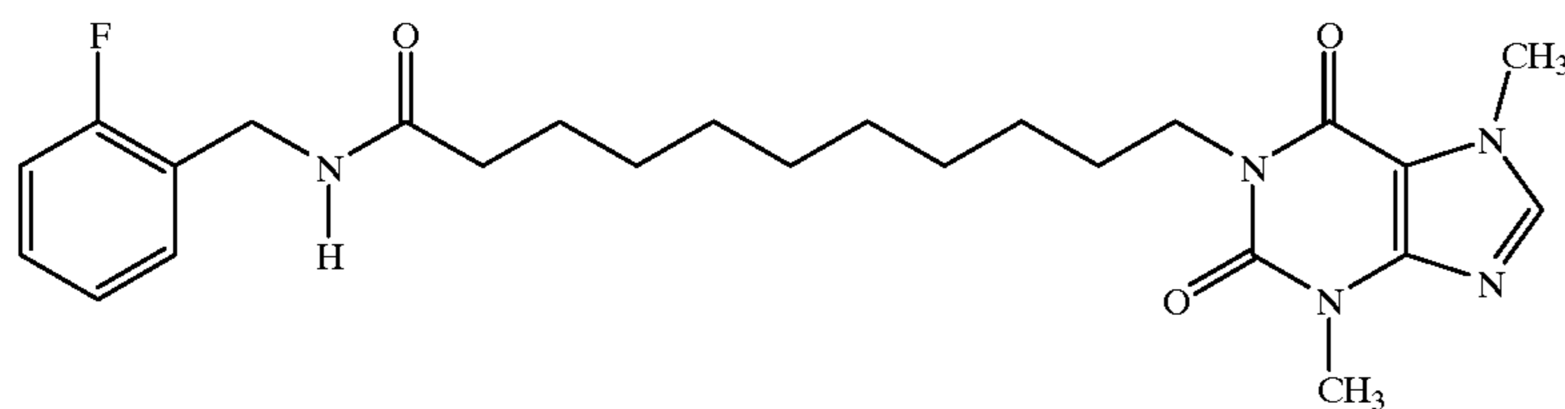
1-[N-(2-Fluorobenzyl)-11-yl-undecanamide]-3,7-dimethylxanthine
