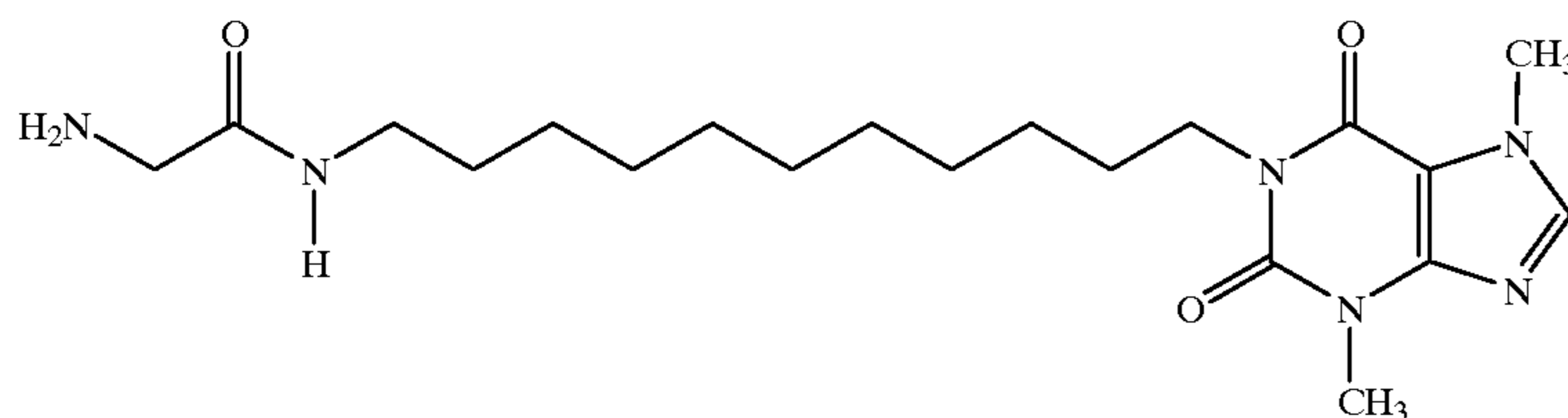
1-[11-(Aminoacetamido)undecyl]-3, 7-dimethylxanthine
