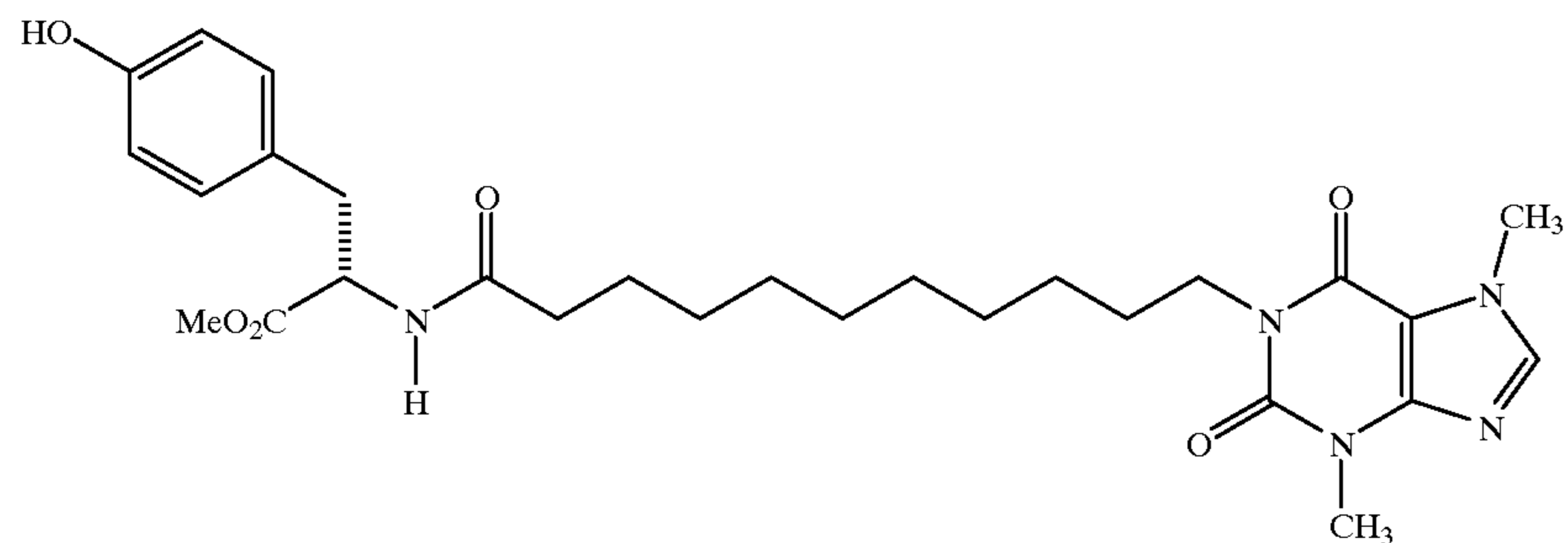
1-(11-[1-Methoxycarbonyl-2-(4-hydroxyphenyl)ethylamino]-11-oxoundecyl)-3,7-dimethylxanthine
