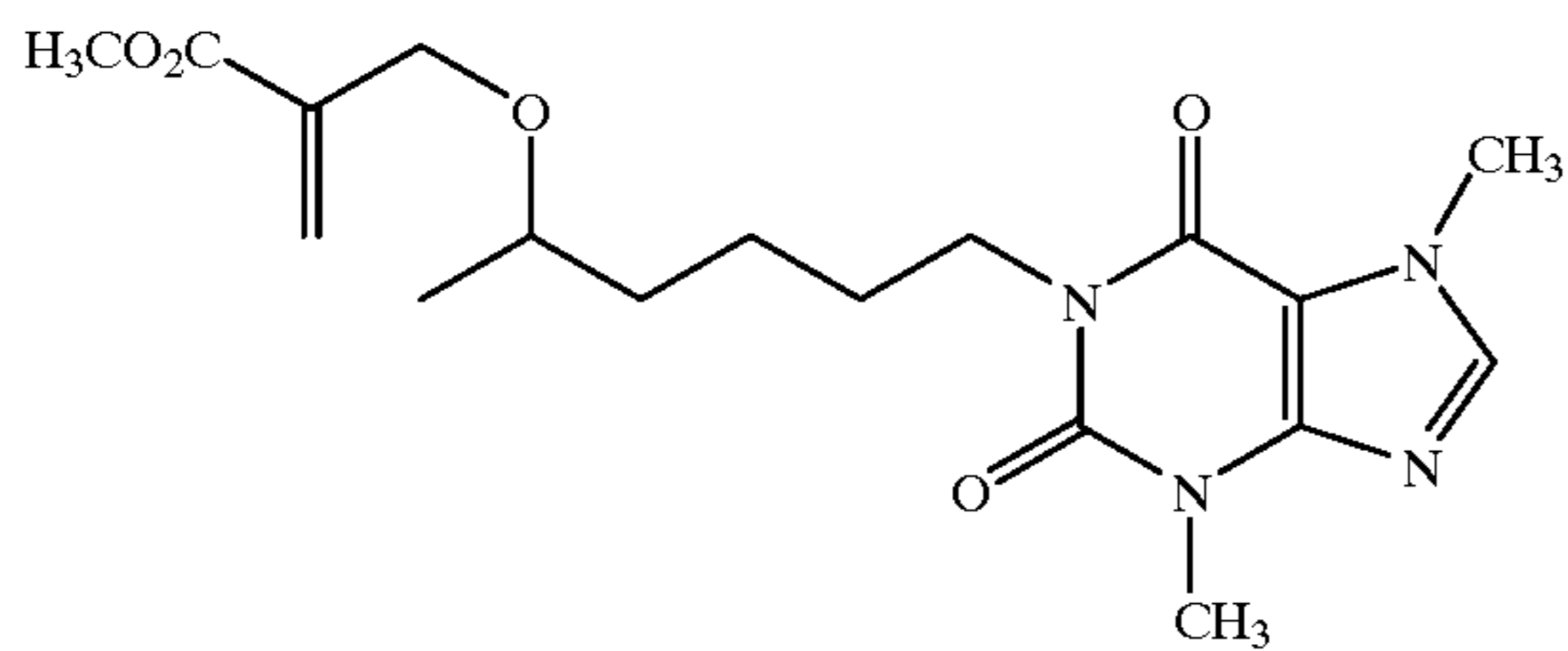
1-(5R-(2-Carbomethoxyallyloxy)hexyl)-3, 7-dimethylxanthine
