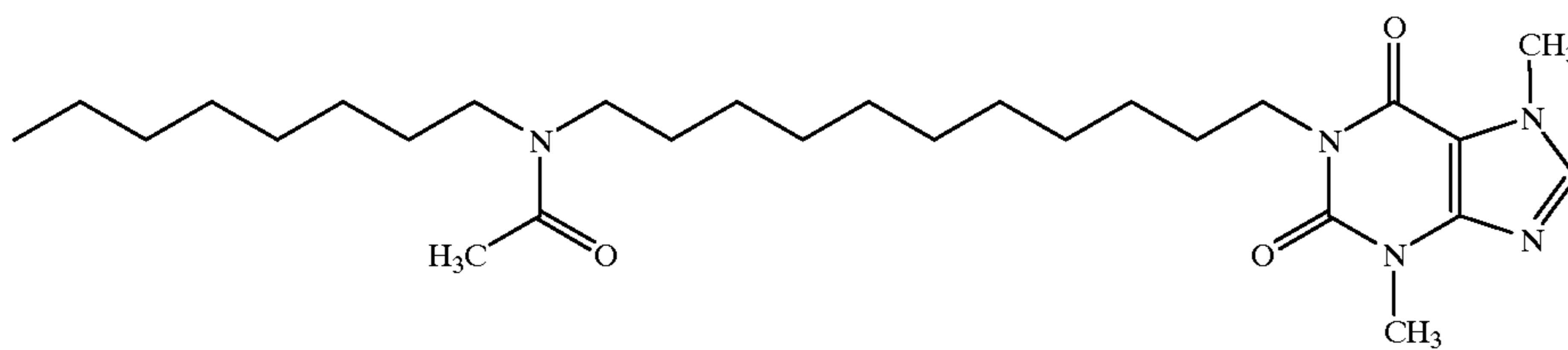
1-[11-(N-Octyl acetamido)undecyl]-3,7-dimethylxanthine
