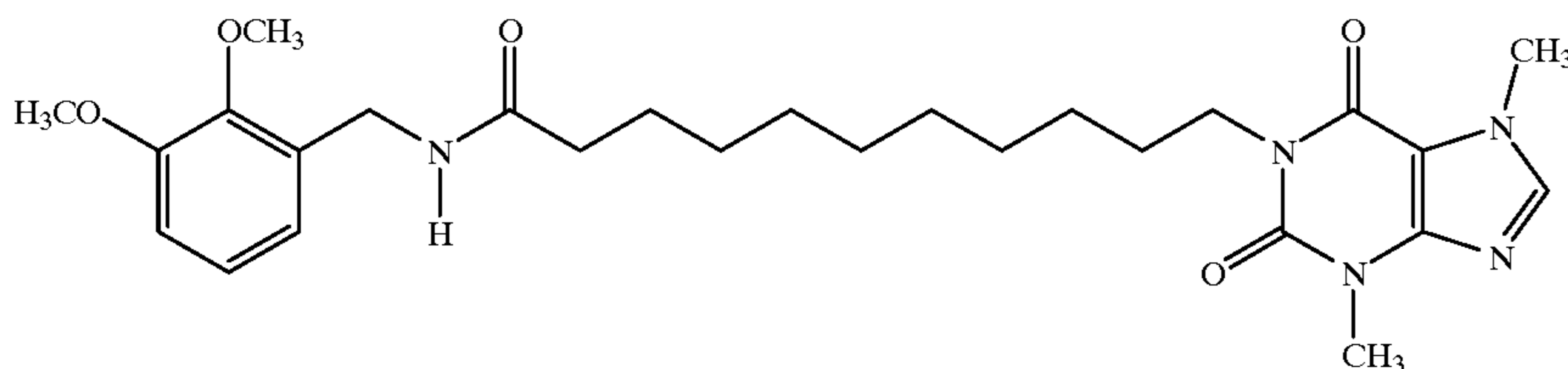
1-[N-(2,3-Dimethoxybenzyl)-11-yl-undecanoamide]-3,7-dimethylxanthine
