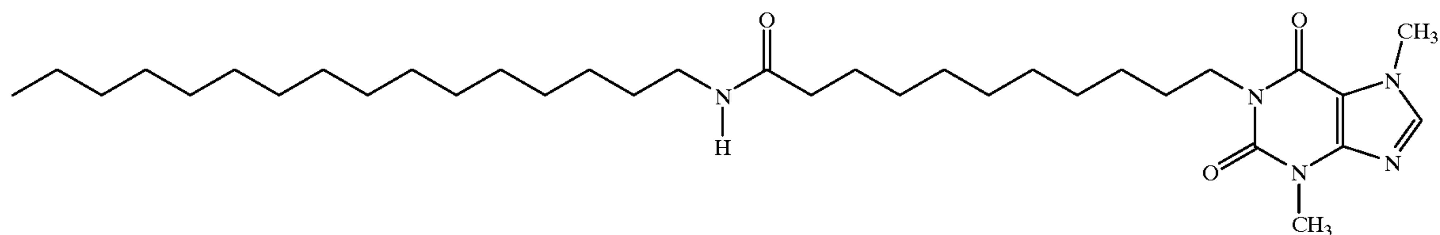
1-(N-Hexadecyl-11-yl-undecanamide)-3,7-dimethylxanthine
