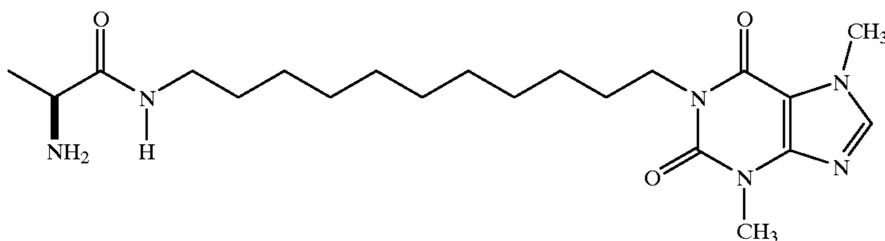
(S)-1-[11-(2-Aminopropionamido)undecyl]-3,7-dimethylxanthine
