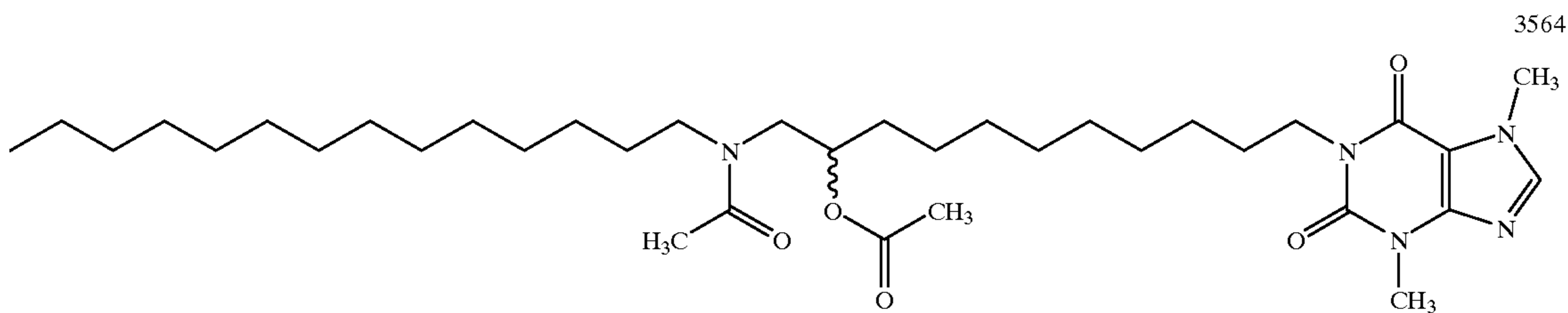
1-[11-N-Tetradecylacetamido)-10-acetoxyundecyl]-3, 7-dimethylxanthine
