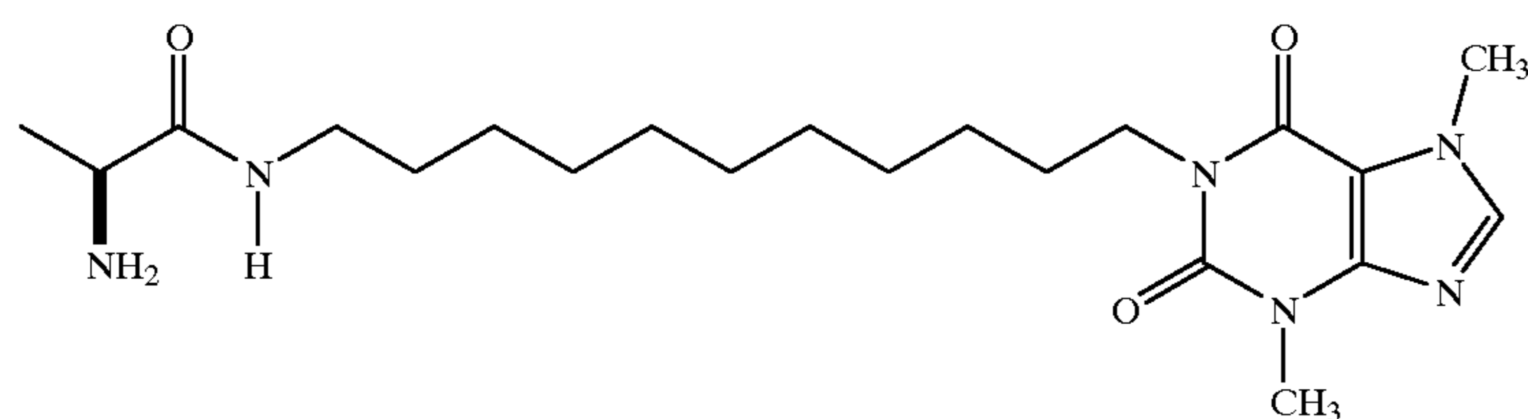
(S)-1-[11-(2-Aminopropionamido)undecyl]-3,7-dimethylxanthine
