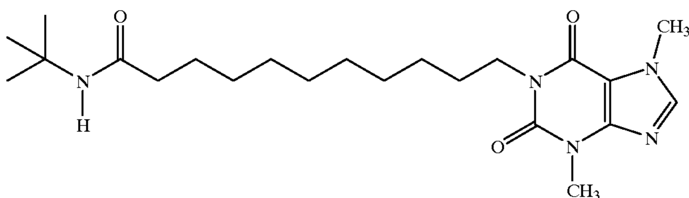
1-[(N-tert-Butyl)-11-yl-undecanamide]-3,7-dimethylxanthine
