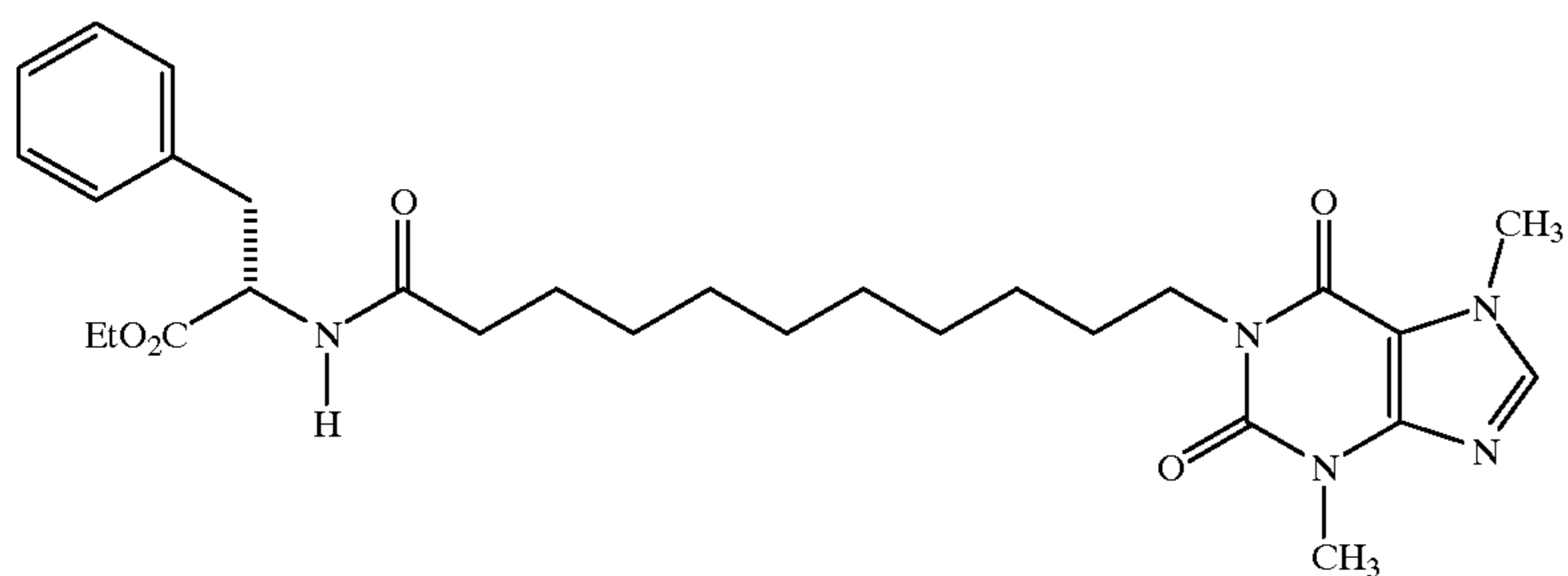
1-[11-(1-Ethoxycarbonyl-2-phenylethylamino)-11-oxoundecyl]-3,7-dimethylxanthine
