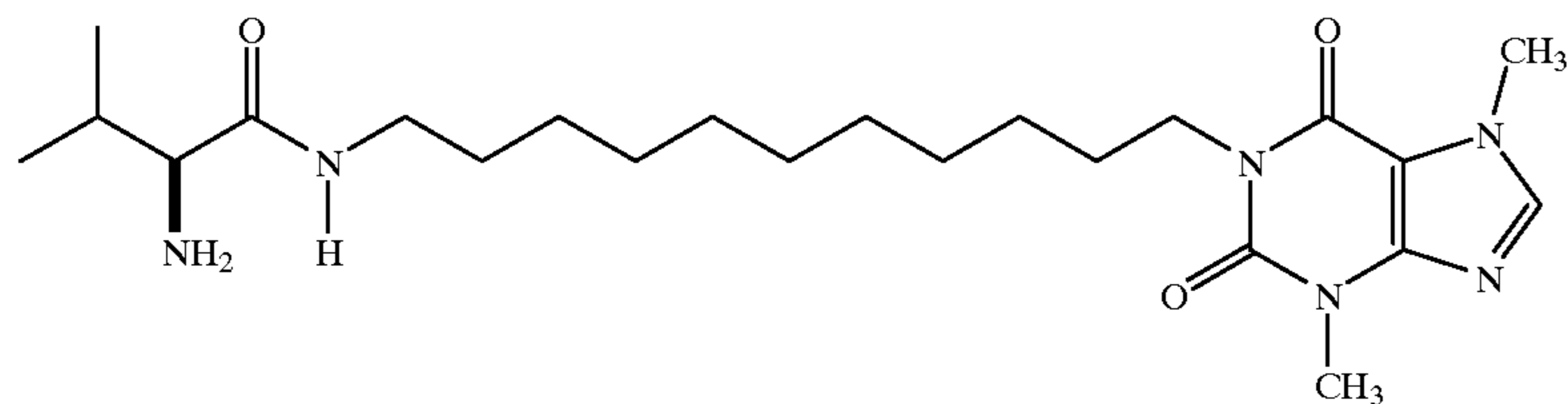
1-[11-(2-Amino-3-methylbutyramido)undecyl]-3,7-dimethylxanthine
