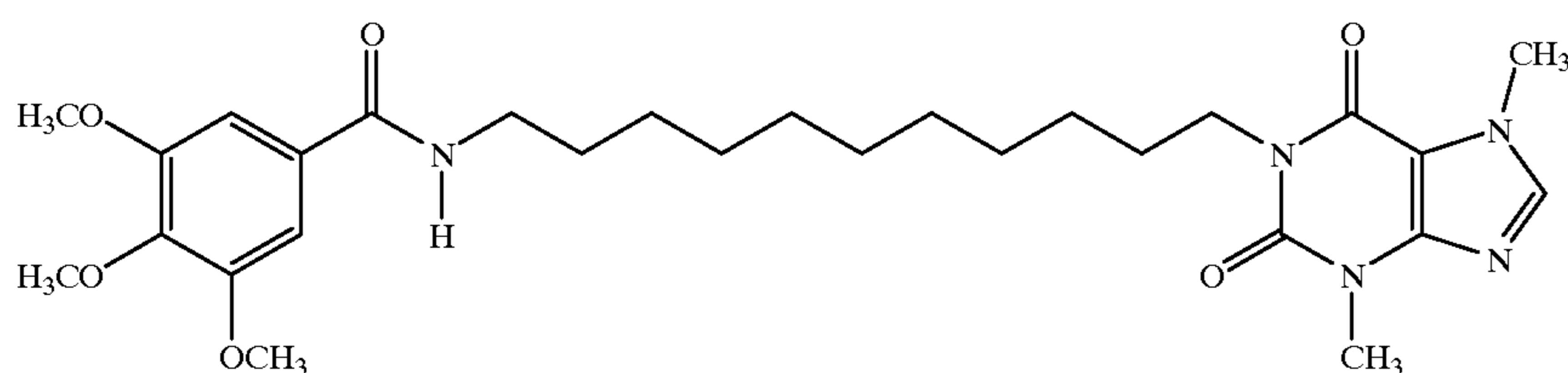
1-[11-(3,4,5-Trimethoxybenzamido)undecyl]-3,7-dimethylxanthine
