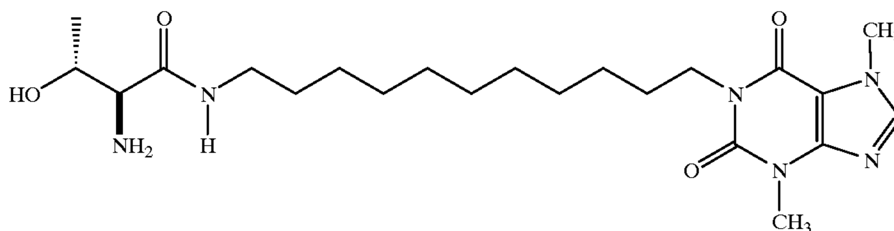
(S)-1-[11-(2-Amino-3-hydroxybutyramido)undecyl]-3,7-dimethylxanthine
