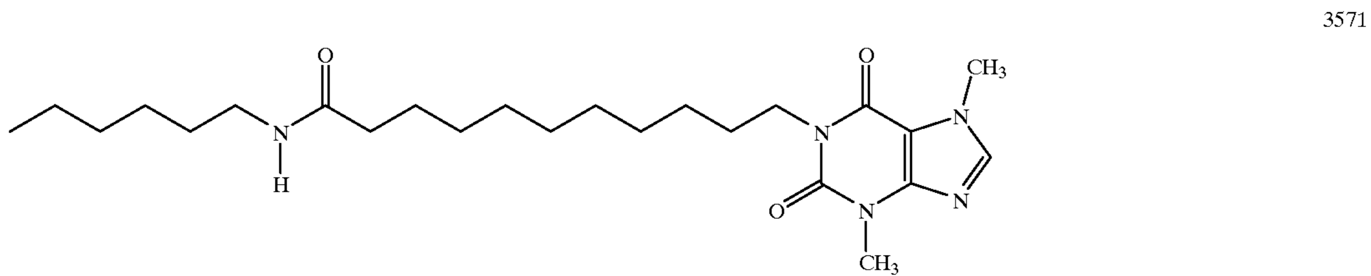
1-(N-Hexyl-11-yl-undecanamide)-3, 7-dimethylxanthine
