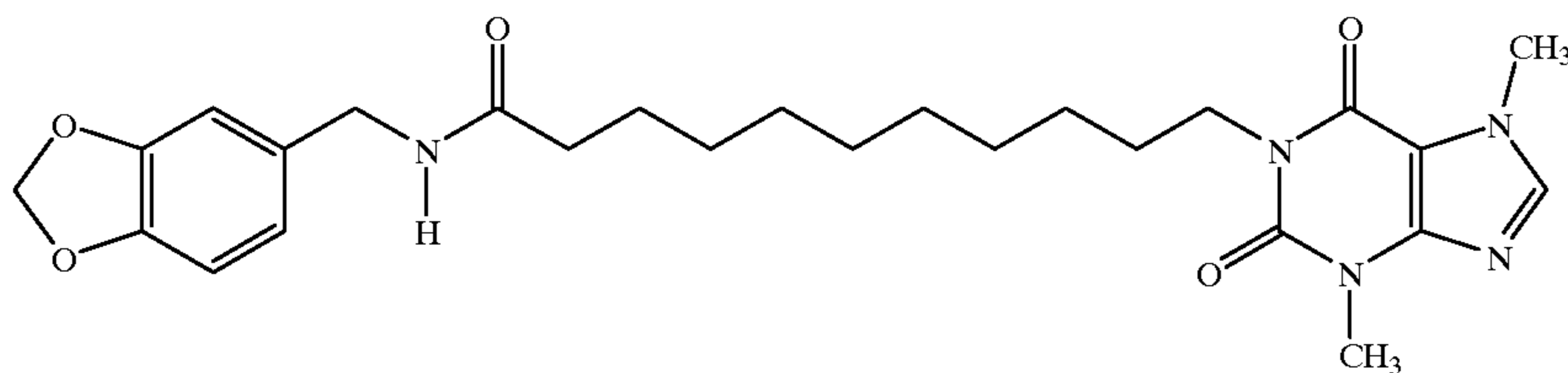
1-[N-(Piperonyl)-11-yl-undecanamide]-3,7-dimethylxanthine
