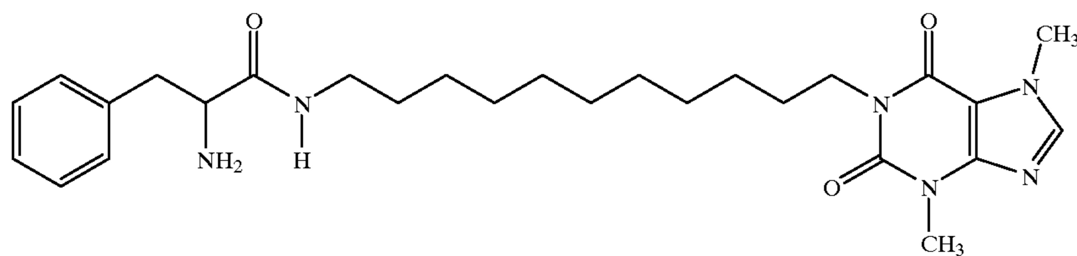
(S)-1-[11-(2-Amino-3-phenylpropionamido)undecyl]-3,7-dimethylxanthine
