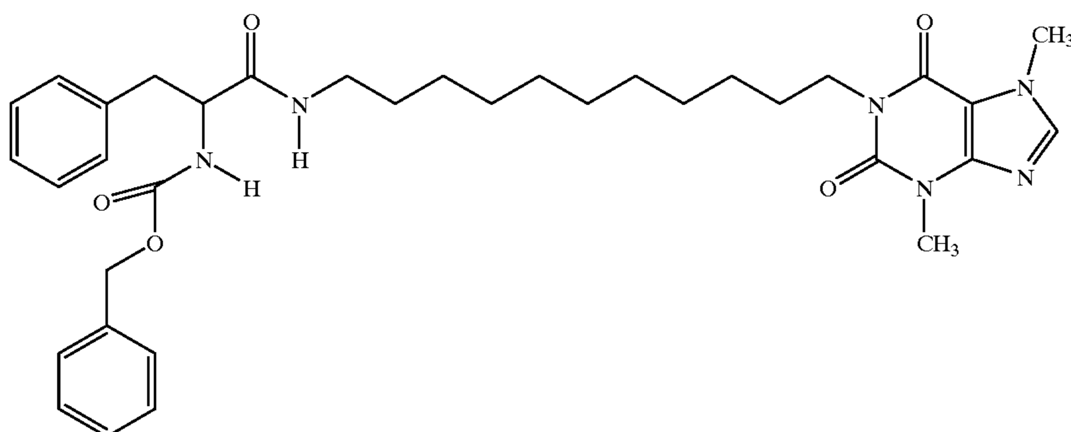
(S)-1-[11-(2-Carbobenzyloxyamino-3-phenylpropionamido)undecyl]-3,7-dimethylxanthine
