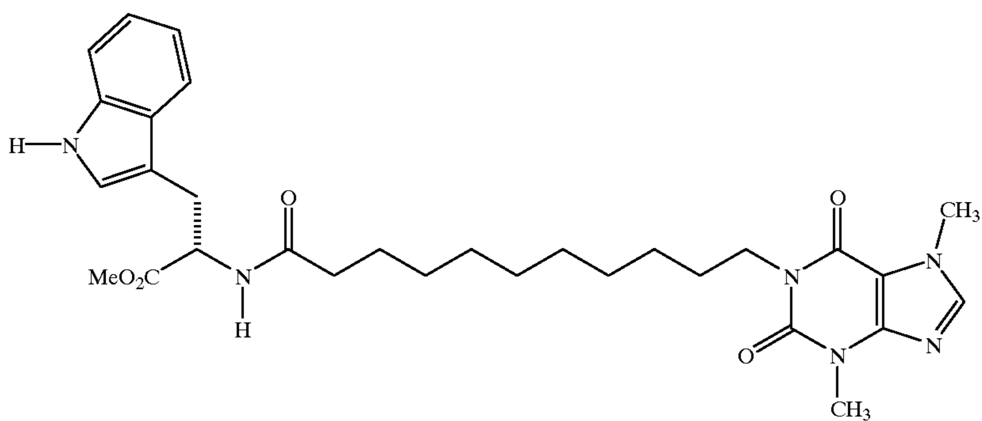
1-(11-[2-(3-Indolyl)-1-methoxycarbonyl ethylamino]-11-oxoundecyl)-3,7-dimethylxanthine
