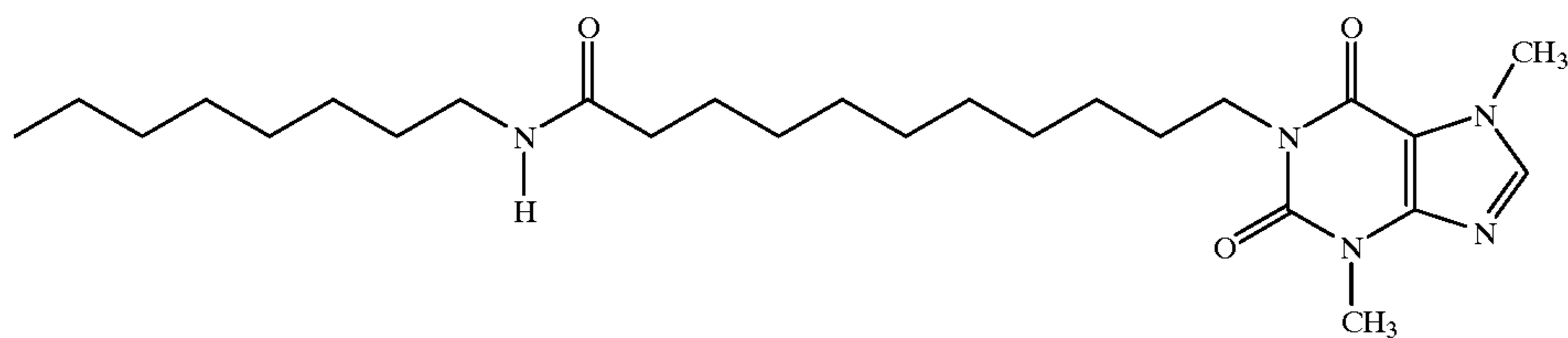
1-(N-OCyl-11-yl-undecanamide)-3,7-dimethylxanthine
