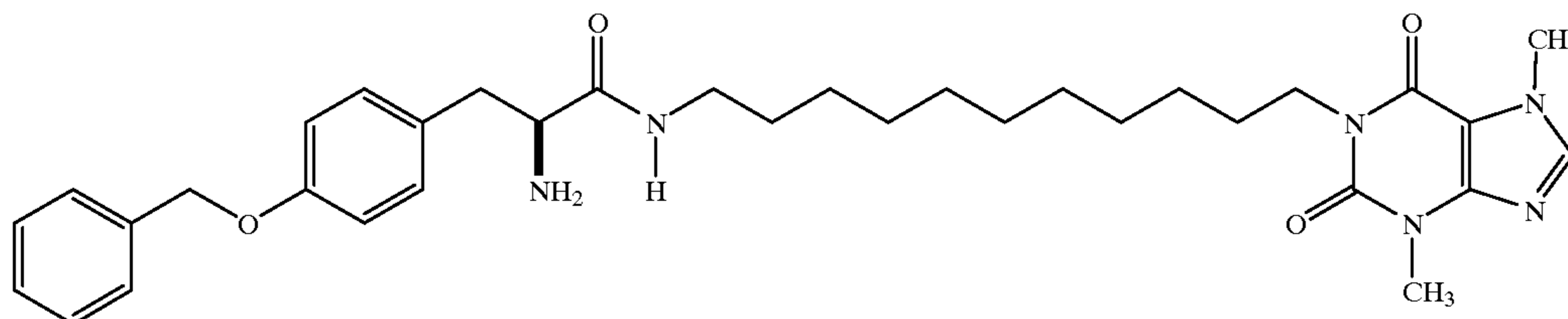
(S)-1-(11-[2-Amino-3-(4-benzyloxyphenyl)propionamido]undecyl)-3,7-dimethylxanthine
