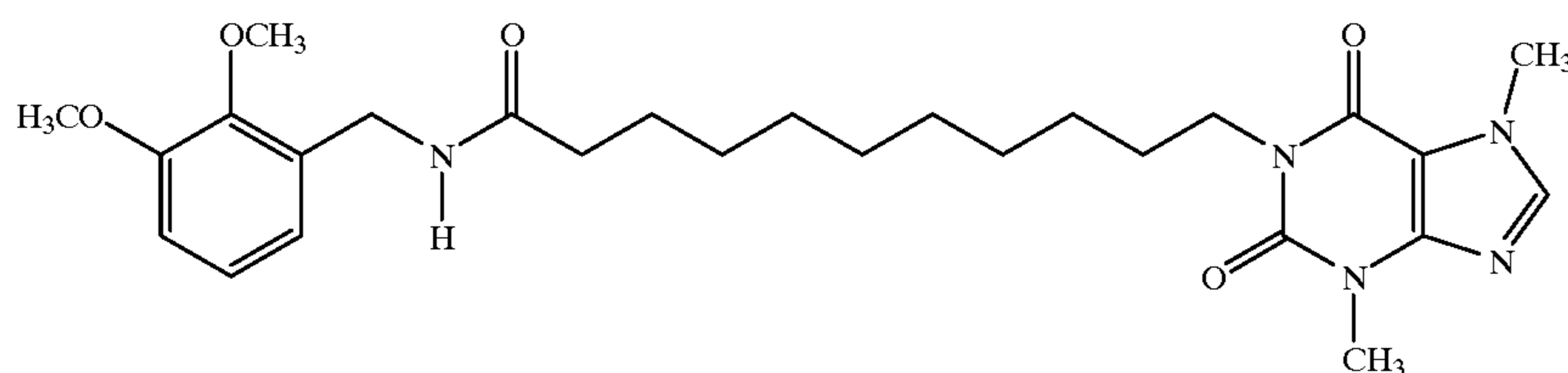
1-[N-(2,3-Dimethoxybenzyl)-11-yl-undecanoamide]-3,7-dimethylxanthine
