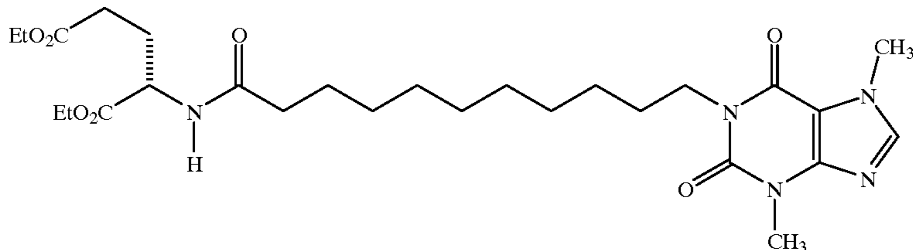
1-(11-[1,3-Bis(ethoxycarbonyl)propylamino]-11-oxoundecyl)-3,7-dimethylxanthine
