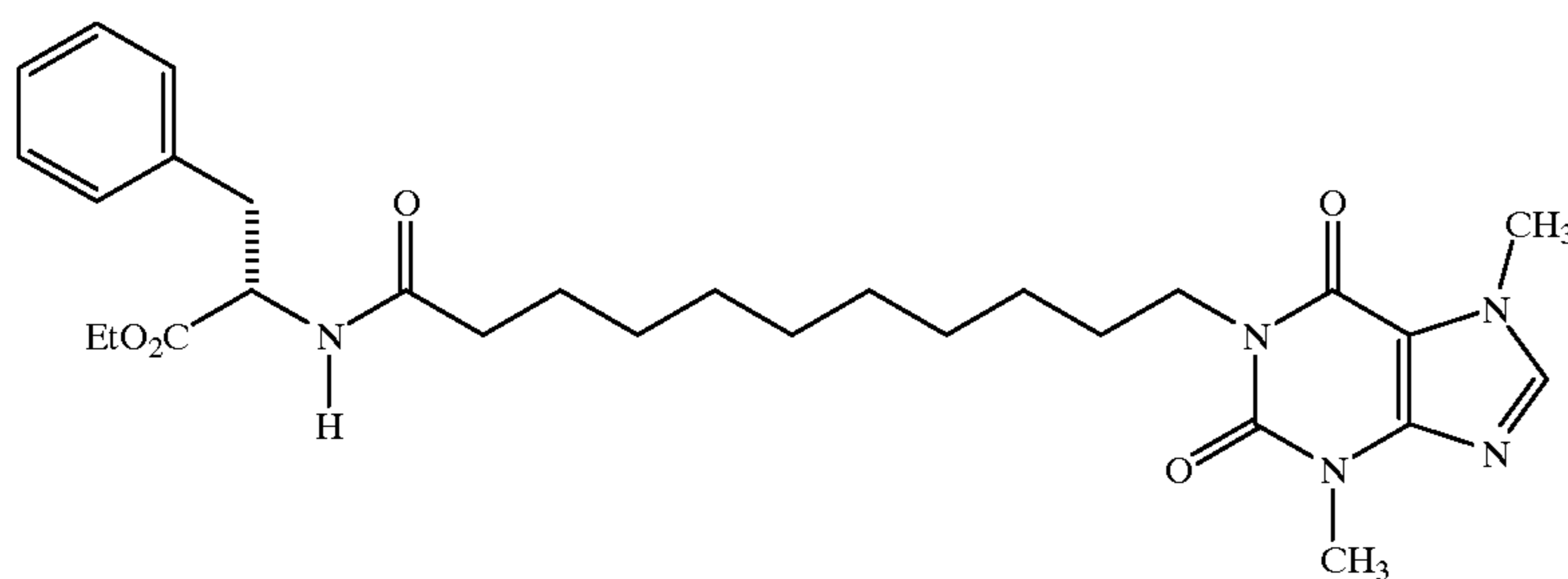
1-[11-(1-Ethoxycarbonyl-2-phenylethylamino)-11-oxoundecyl]-3,7-dimethylxanthine
