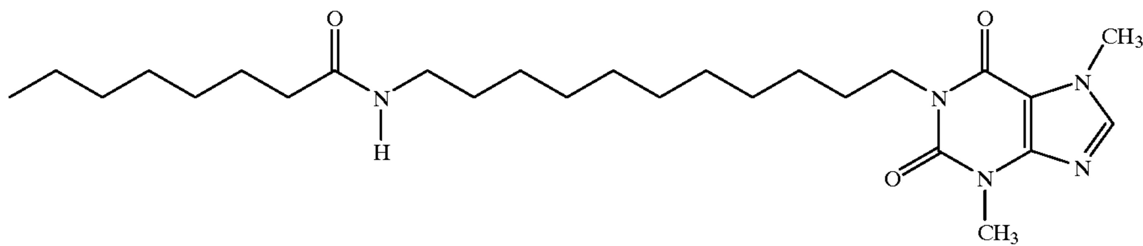
1-(11-(Octanoamido)undecyl)-3, 7-dimethylxanthine
