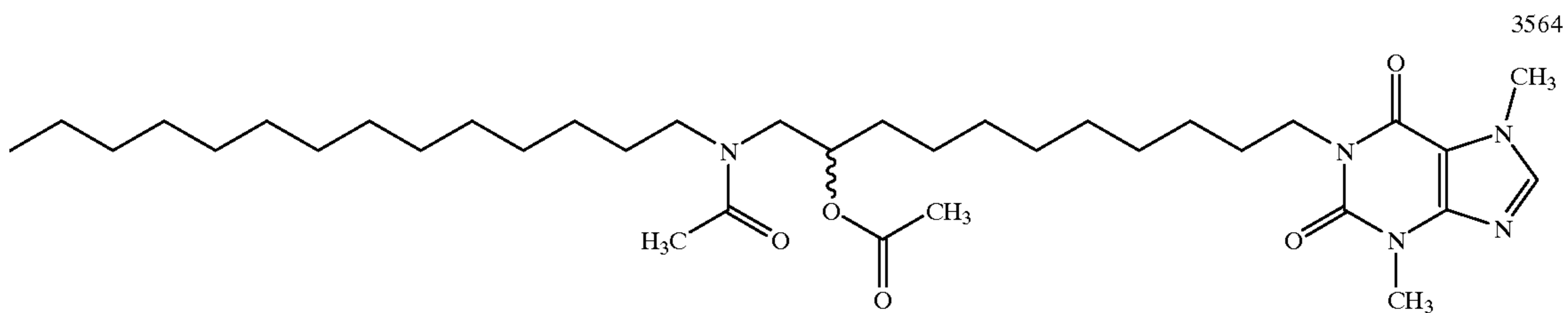
1-[11-N-Tetradecylacetamido)-10-acetoxyundecyl]-3, 7-dimethylxanthine
