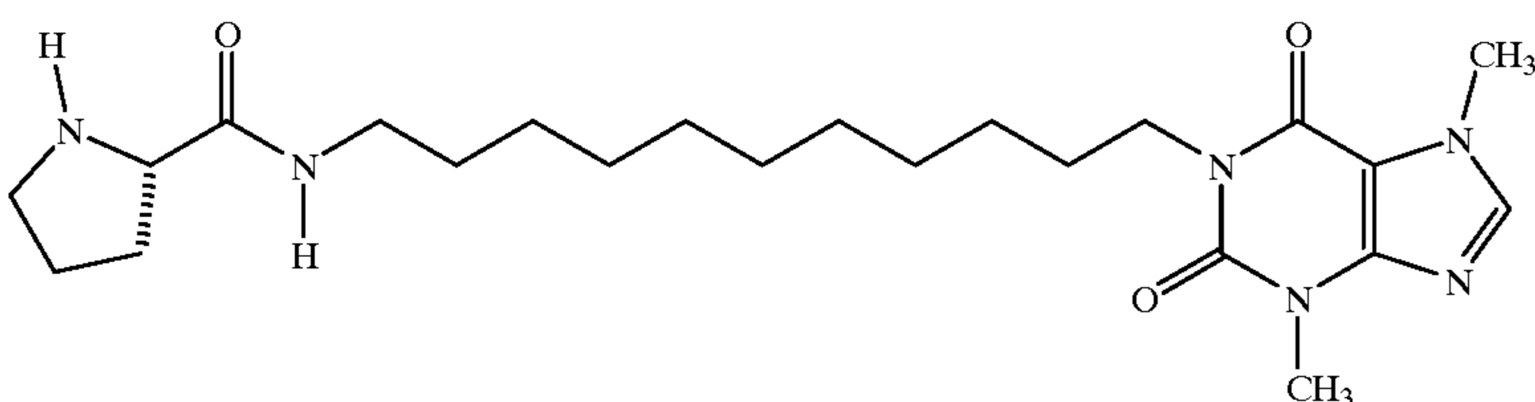
1-[11-(Pyrrolidin-2-yl-formamido)undecyl]-3,7-dimethylxanthine
