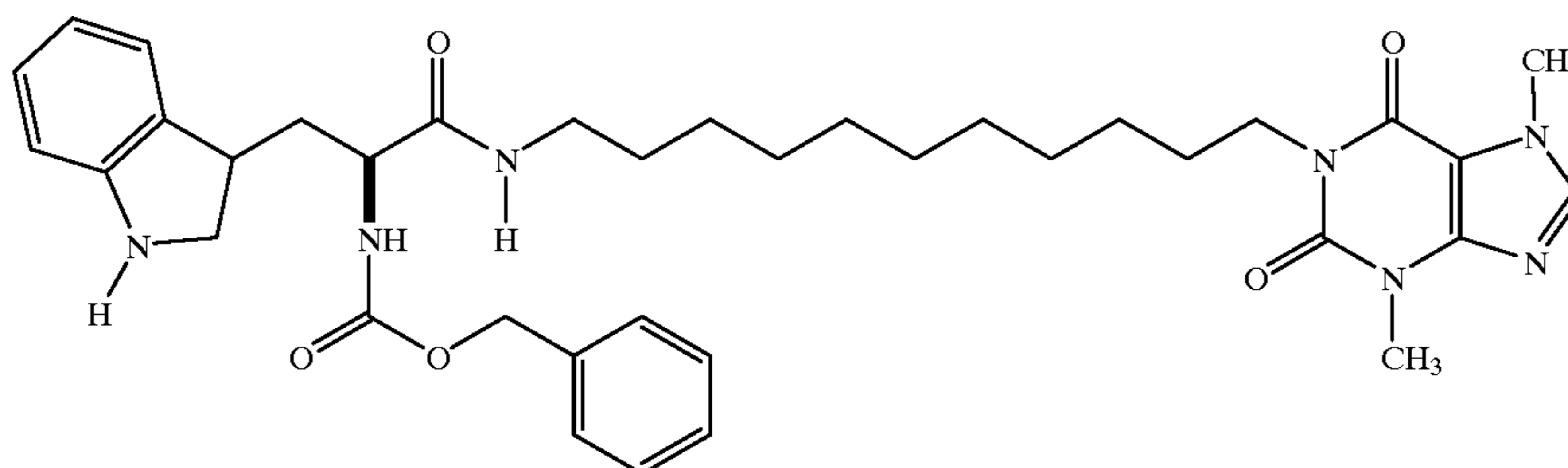
1-(11-[2-Carbobenzyloxyamino-3-(3-indolyl)propionamido]undecyl)-3, 7-dimethylxanthine
