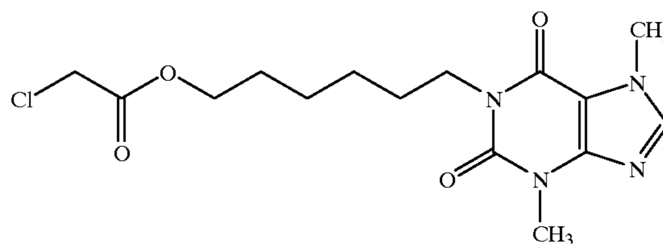
1-[6-(Chloroacetoxy)hexyl]-3,7-dimethylxanthine
