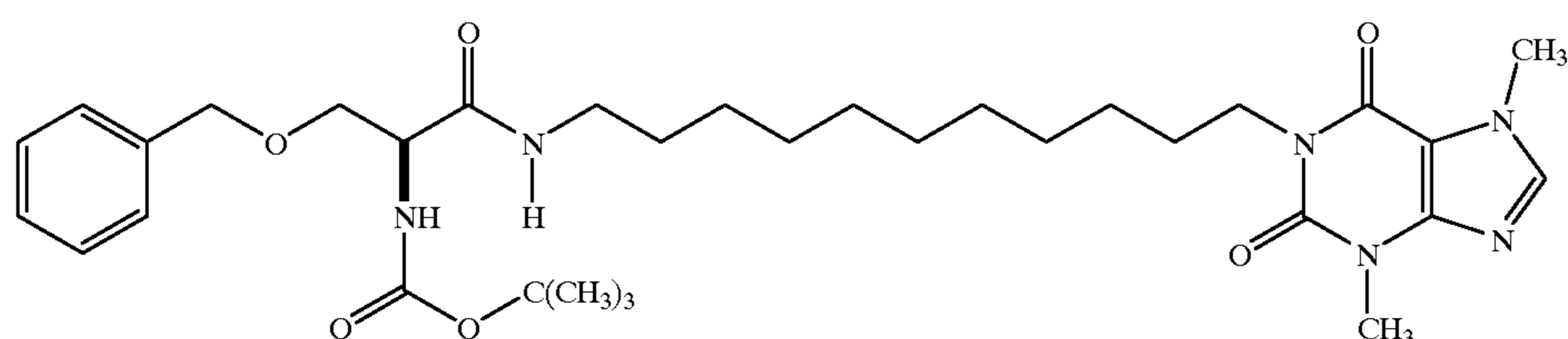
(S)-1-[11-(2-Carbobutoxyamino-3-benzyloxypropionamido)-undecyl]-3,7-dimethylxanthine
