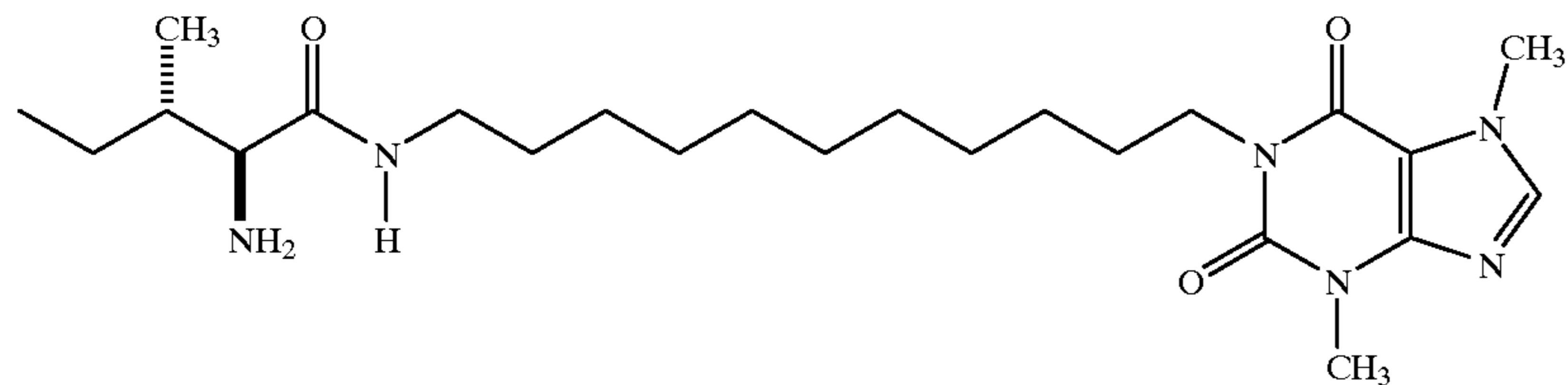
1-[11-(2-Amino-3-methylpentanamido)undecyl]-3,7-dimethylxanthine
