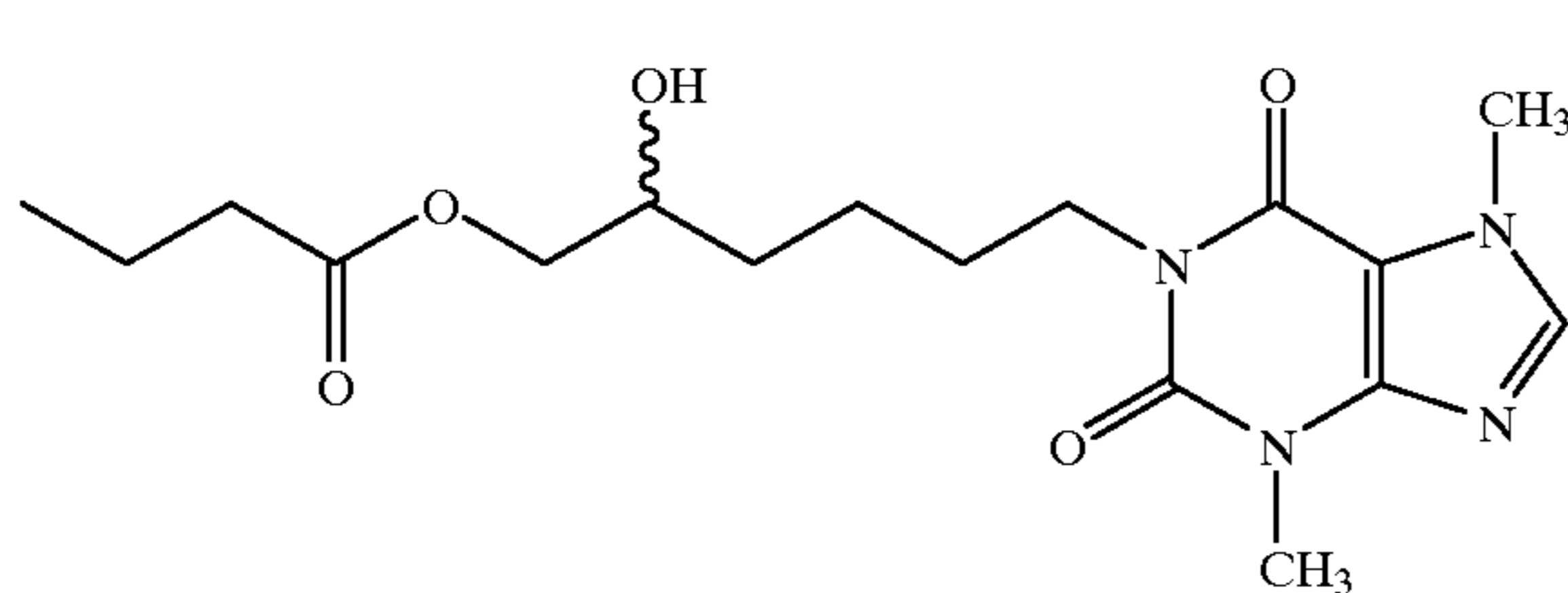
1-(6-Butyroy-5-hydroxyhexyl)-3,7-dimethylxanthine
