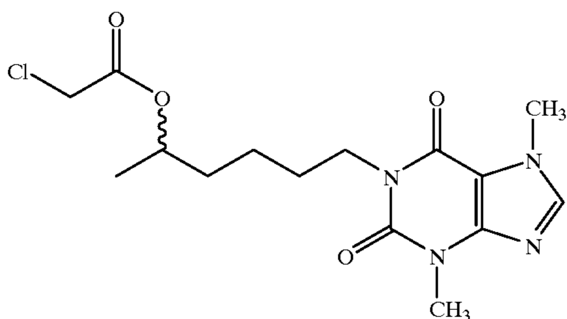
1-[5-(chloroacetoxy)hexyl]-3,7-dimethylxanthine
