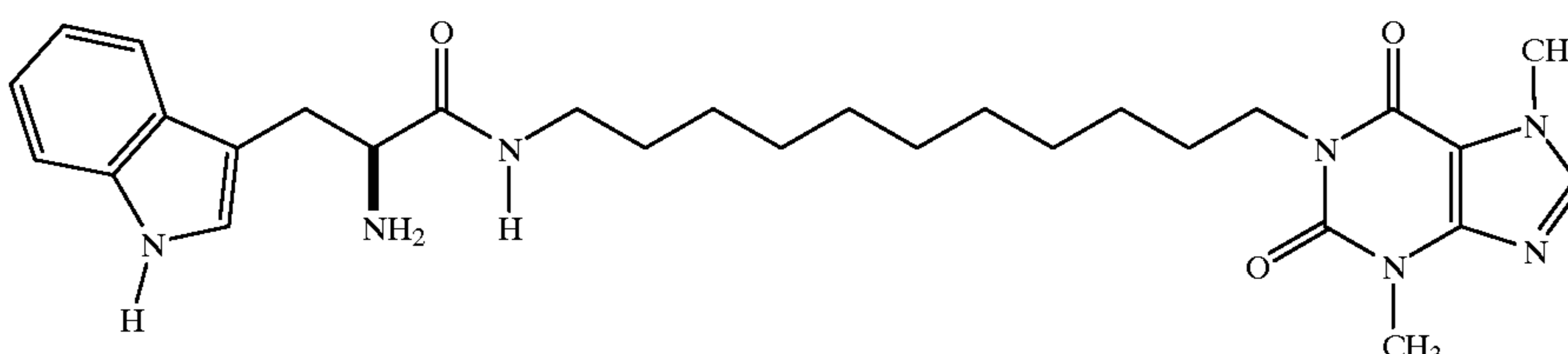
1-(11-[2-Amino-3-(3-indolyl)propionamido]undecyl)-3, 7-dimethylxanthine
