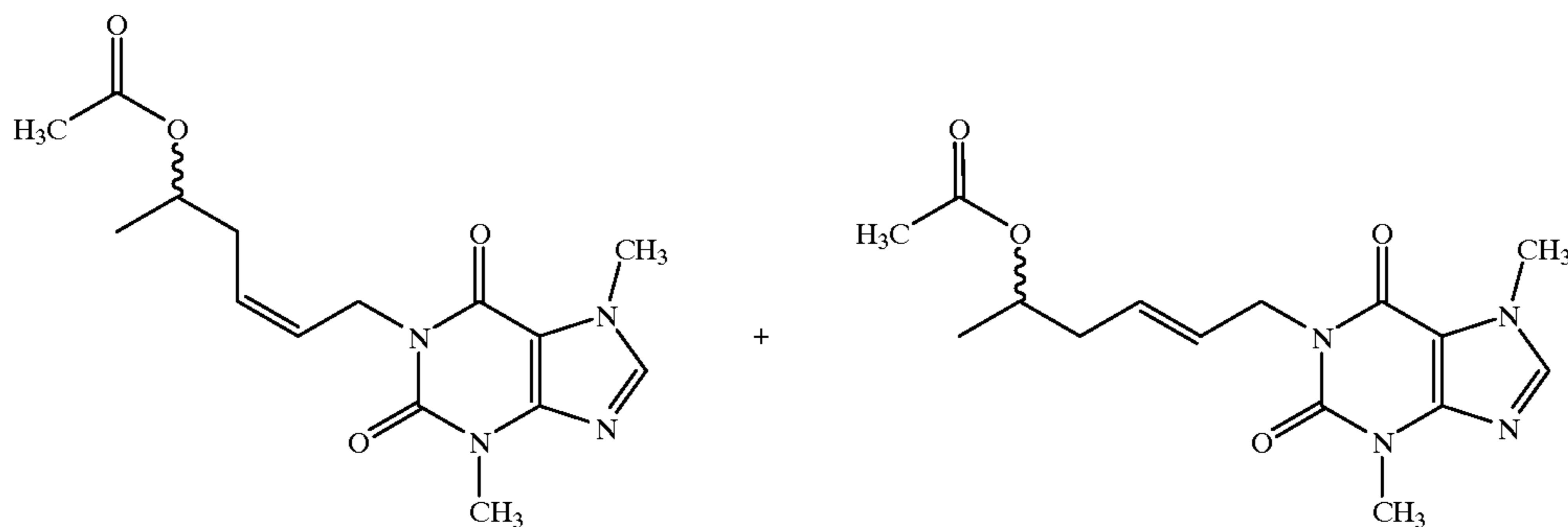
1-[5-Acetoxyhex-3-enyl]-3,7-dimethylxanthine
