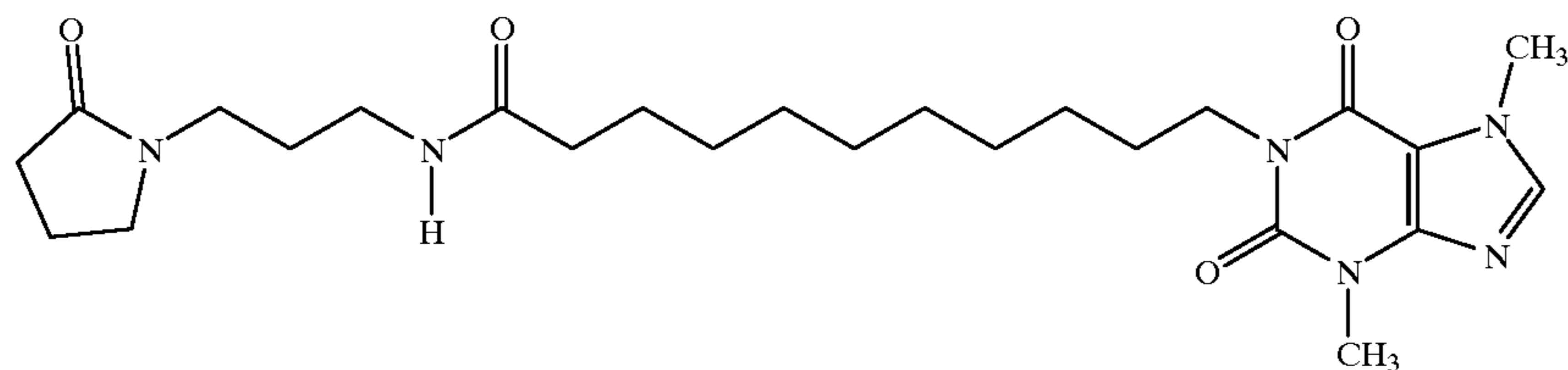
1-[N-(3-Pyrrolidinonylpropyl)-11-yl-undecanoamide]-3,7-dimethylxanthine
