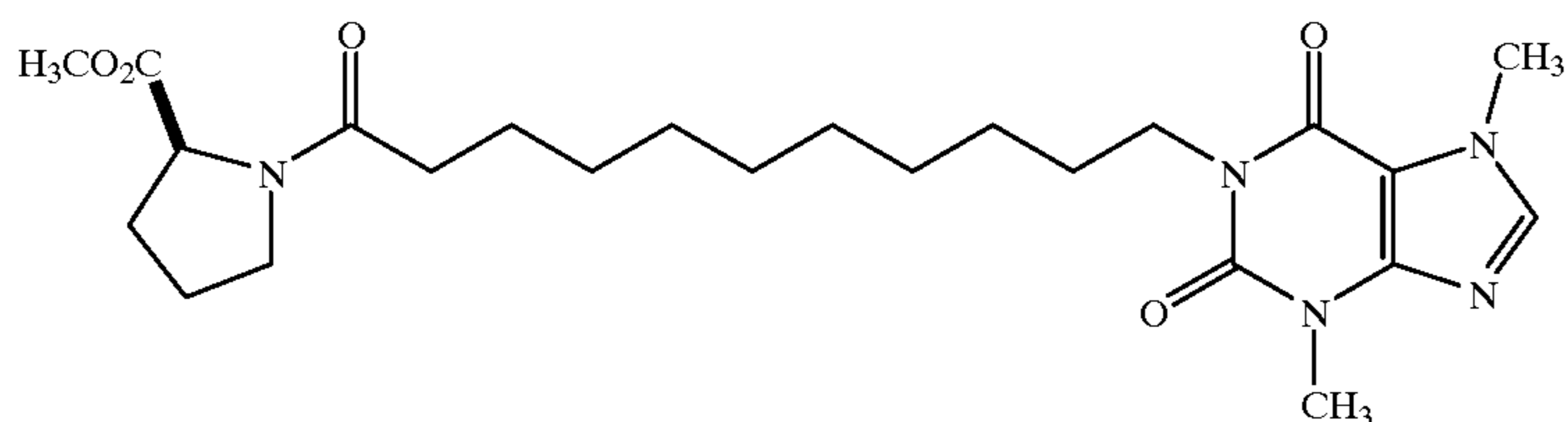
1-[11-(2-Methoxycarbonylpyrrolidin-1-yl)-11-oxoundecyl]-3,7-dimethylxanthine
