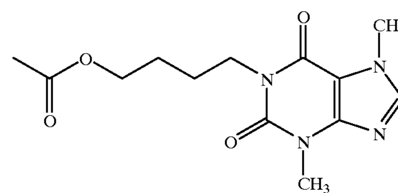
1-(4-Acetoxybutyl)-3,7-dimethylxanthine
