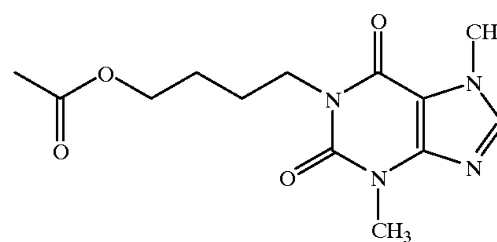
1-(4-Acetoxybutyl)-3,7-dimethylxanthine
