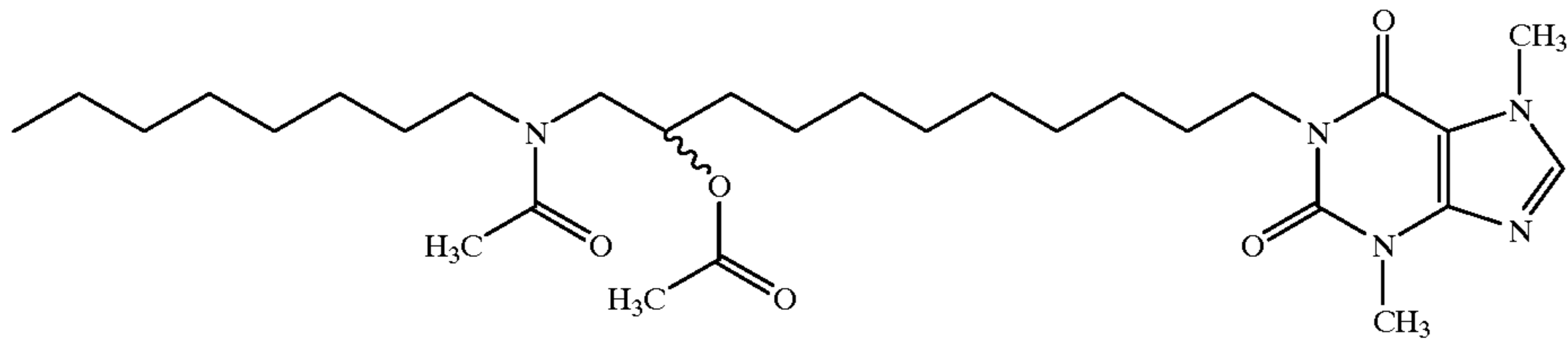
1-[11-(N-Octylacetamido)-10-acetoxyundecyl]-3, 7-dimethylxanthine
