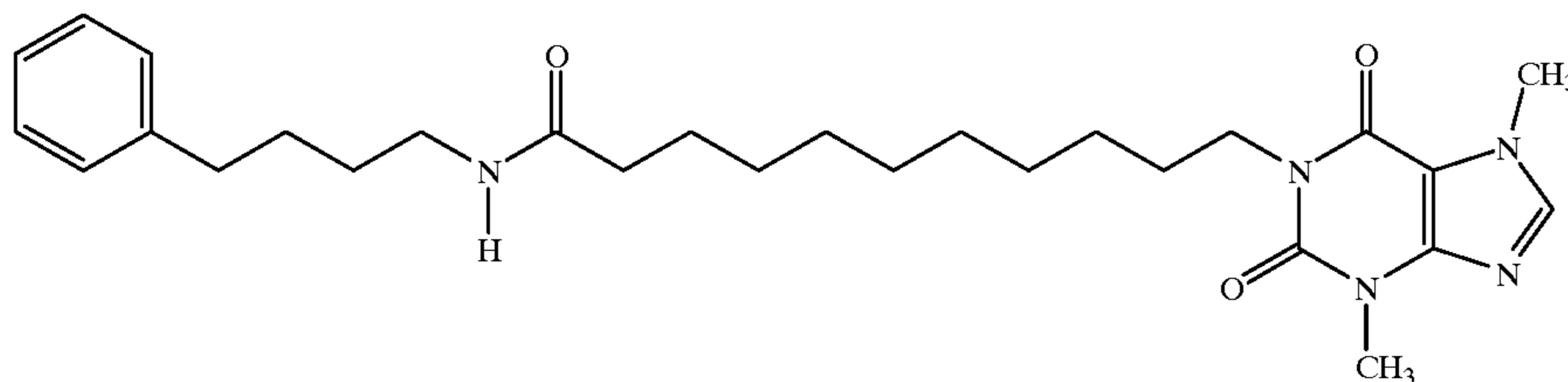
1-[N-(4-Phenylbutyl)-11-yl-undecanamide]-3,7-dimethylxanthine
