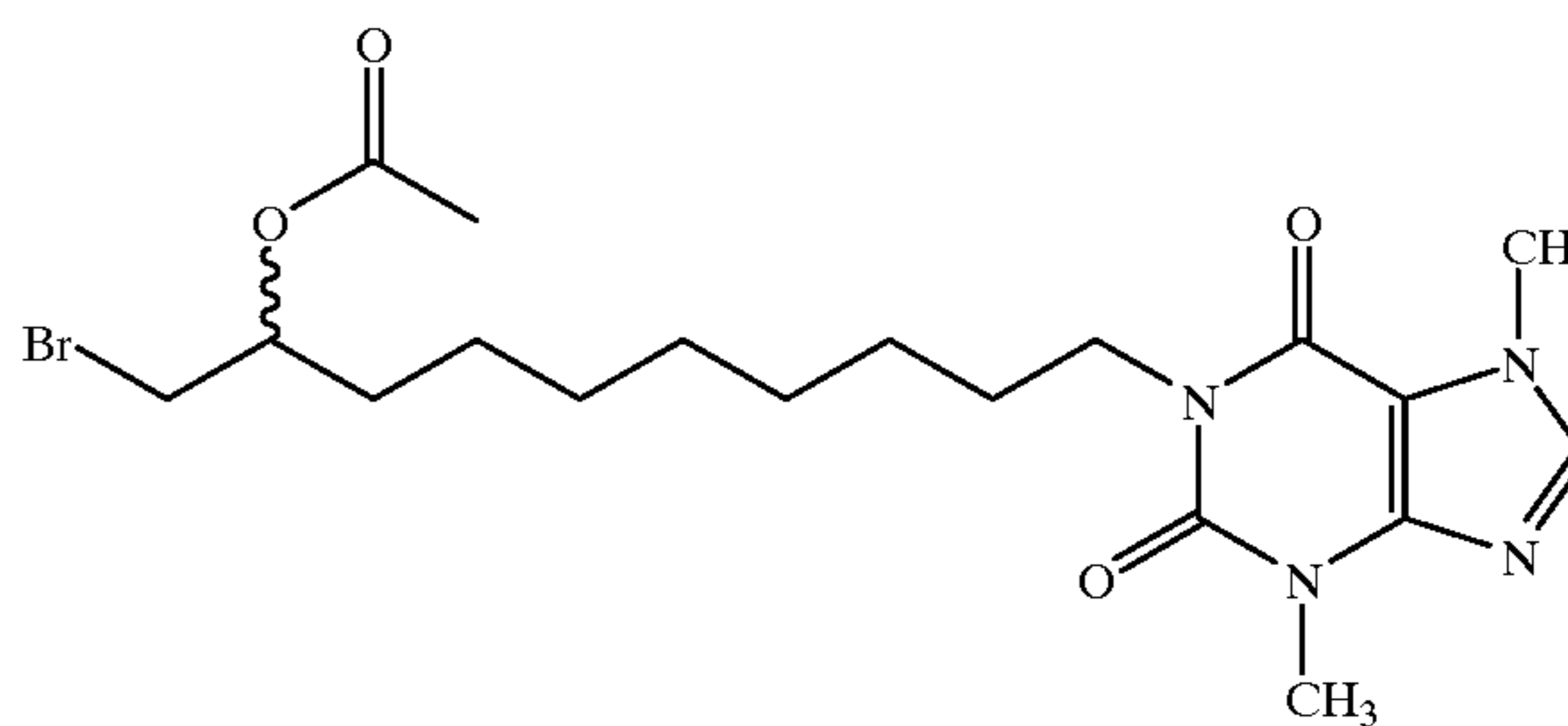
1-(9-Acetoxy-10-bromodecyl)-3,7-dimethylxanthine
