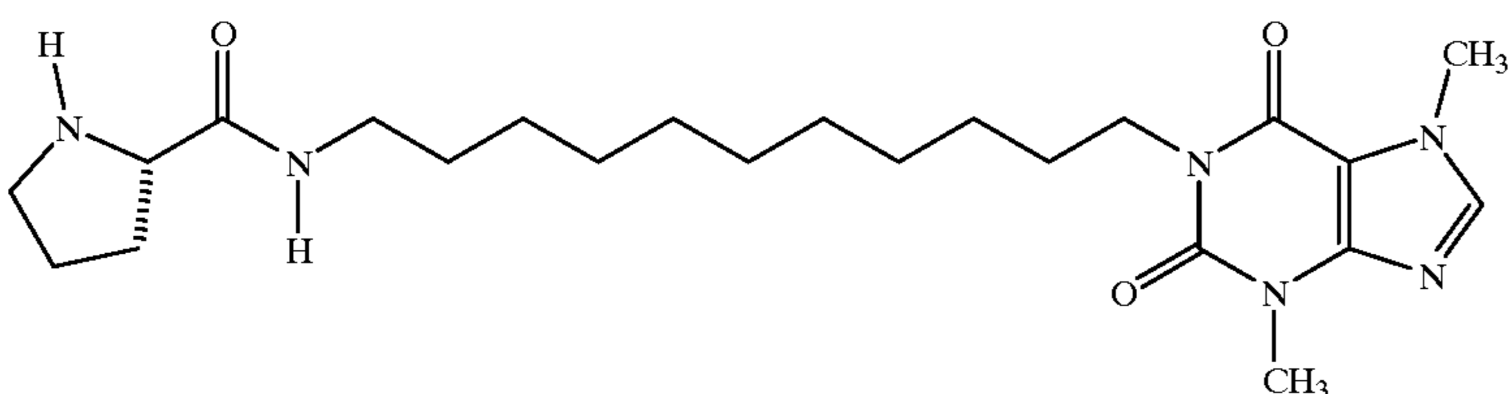
1-[11-(Pyrrolidin-2-yl-formamido)undecyl]-3,7-dimethylxanthine
