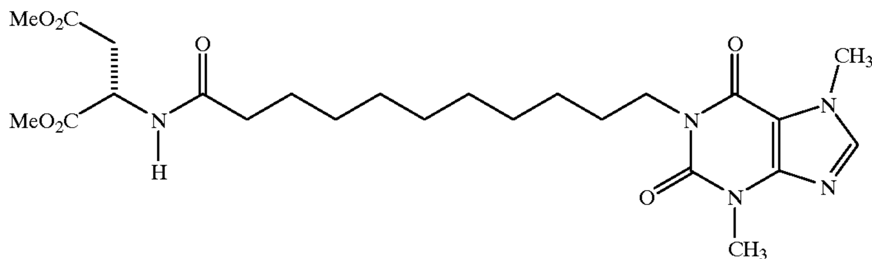
1-(11-[1,2-Bis(methoxycarbonyl)ethylamino]-11-oxoundecyl)-3,7-dimethylxanthine
