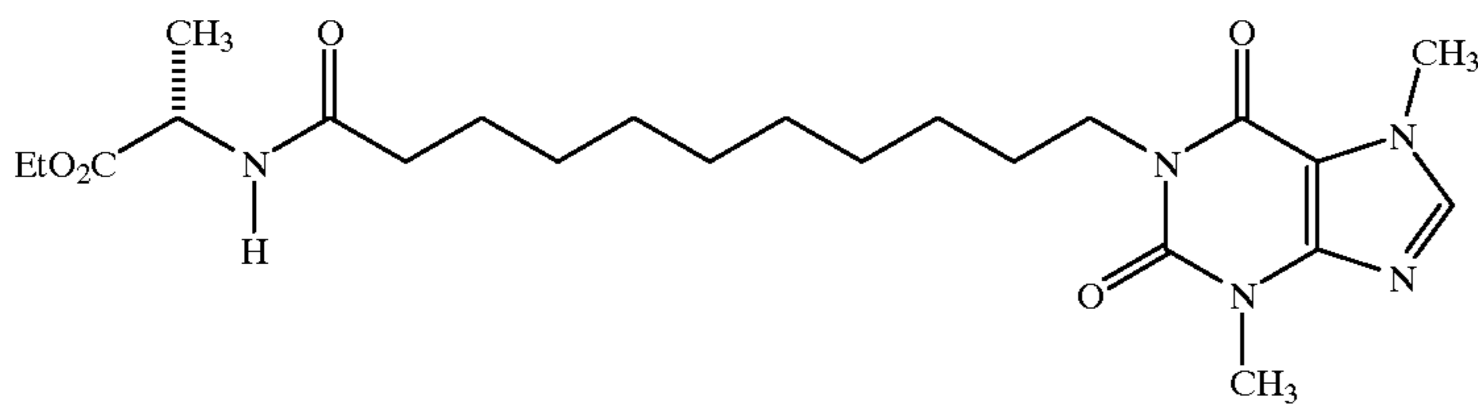
1-[11-(1-Ethoxycarbonylpropylamino)-11-oxoundecyl]-3,7-dimethylxanthine
