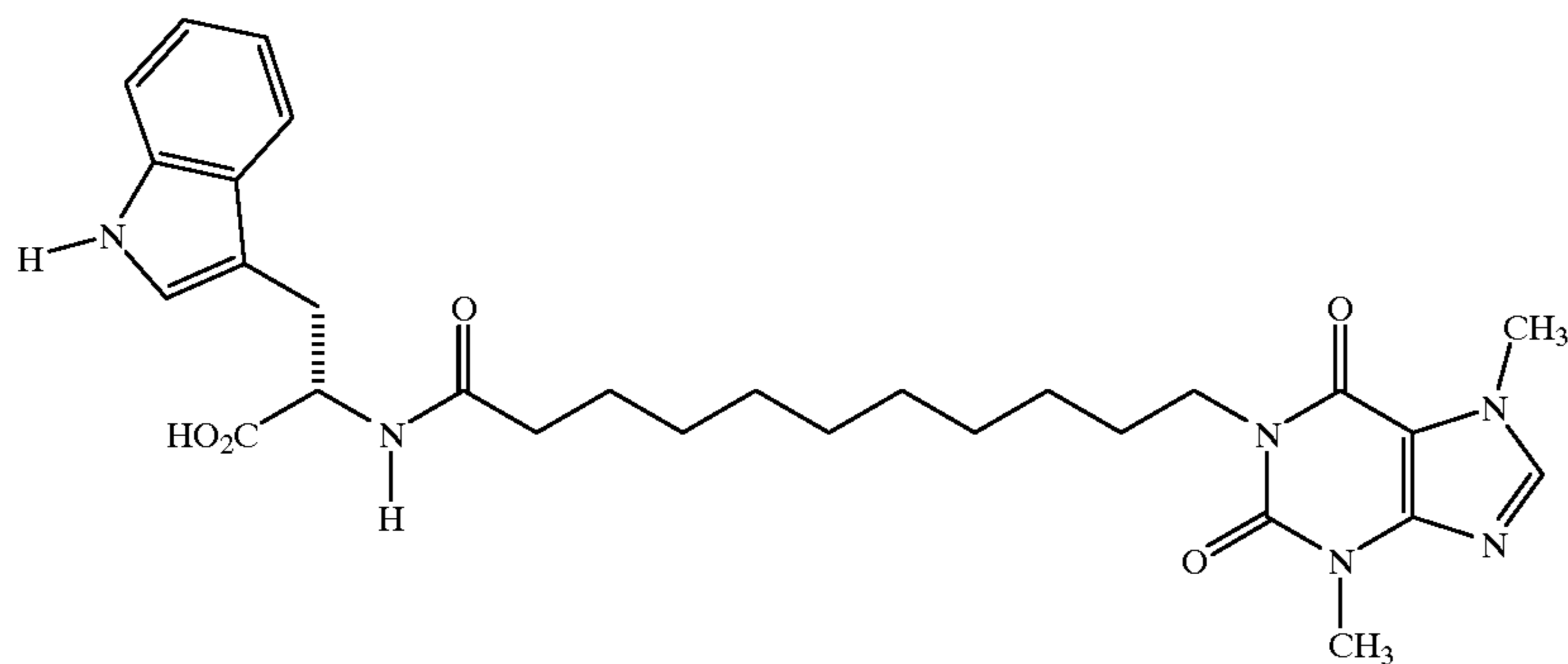
(S)-1-(11-[1-Carboxy-2-(3-Indolyl)ethylamino]-11-oxoundecyl)-3,7-dimethylxanthine
