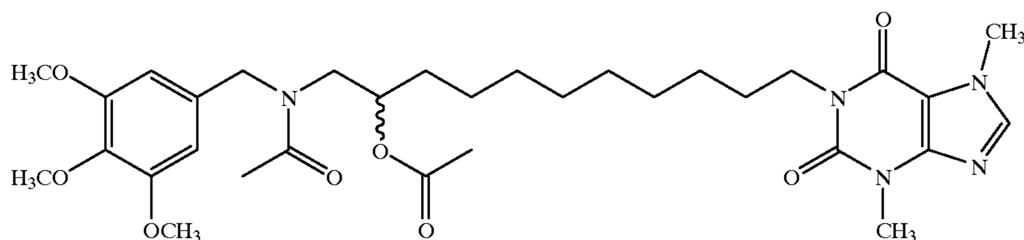
1-[11-(3,4,5-Trimethoxybenzylacetamido)-10-acetoxyundecyl]-3,7-dimethylxanthine
