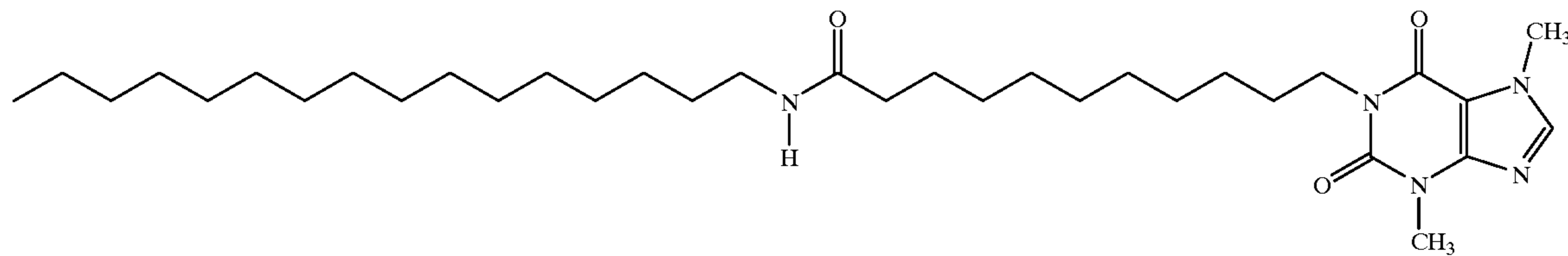
1-(N-Hexadecyl-11-yl-undecanamide)-3,7-dimethylxanthine
