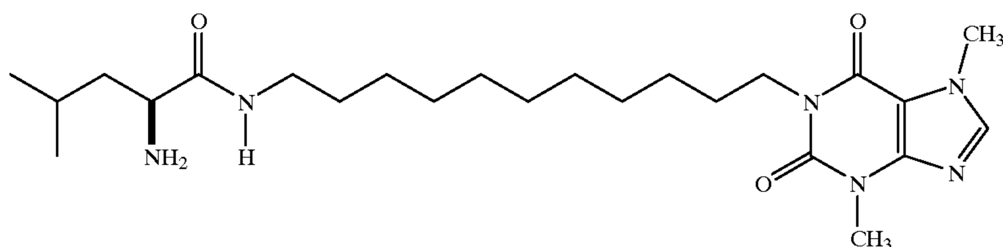
1-[11-(2-Amino-4-methylpentanamido)undecyl]-3,7-dimethylxanthine
