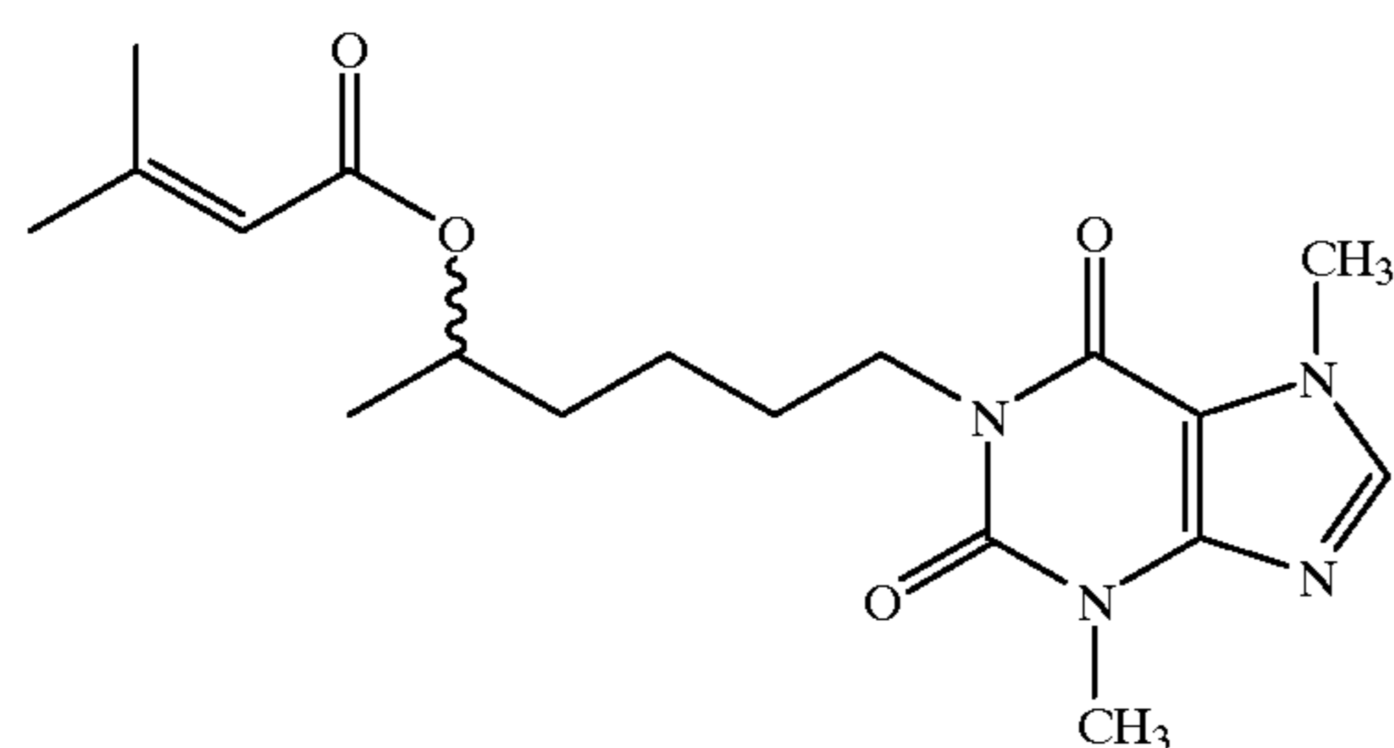
1-([5-(3-Methyl-2-butenoyl)]hexyl)-3,7-dimethylxanthine
