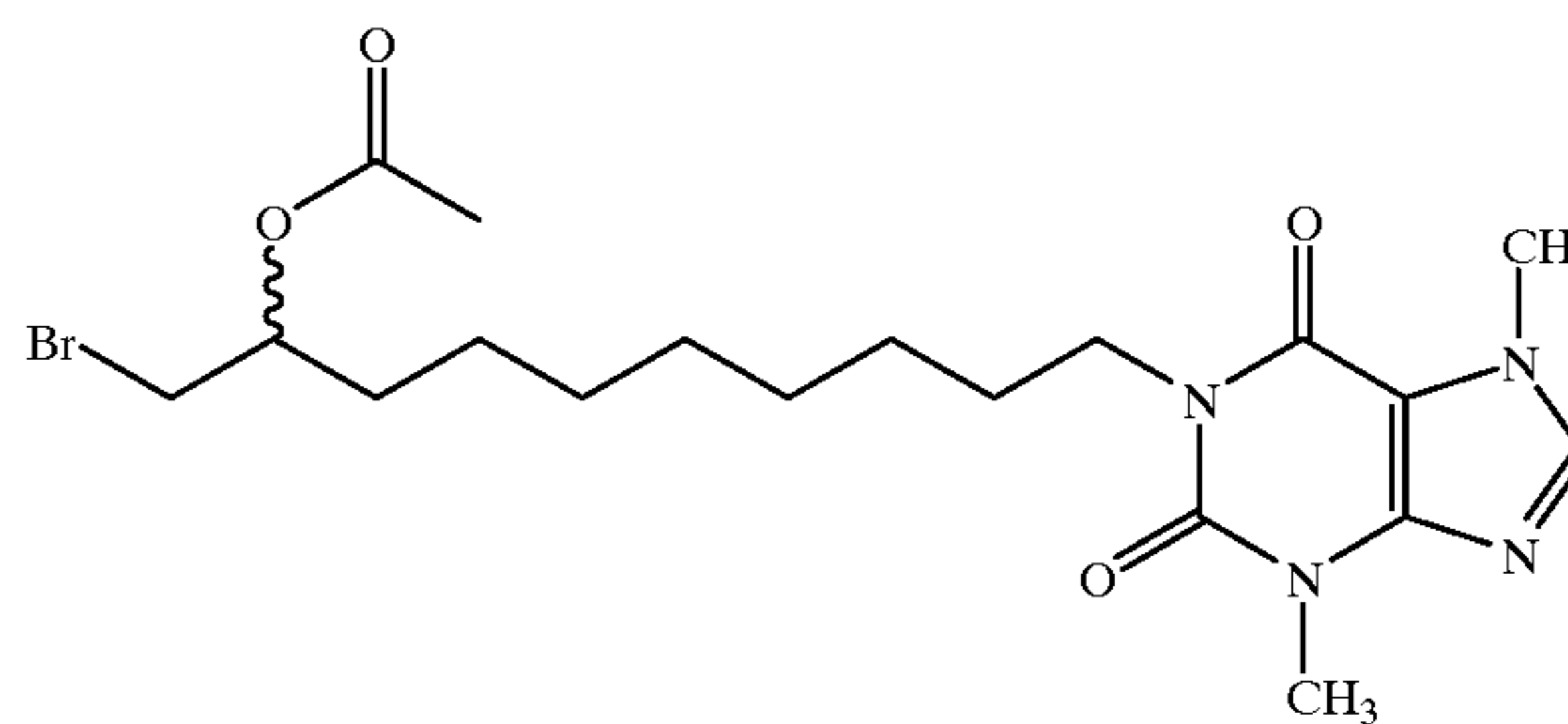
1-(9-Acetoxy-10-bromodecyl)-3,7-dimethylxanthine
