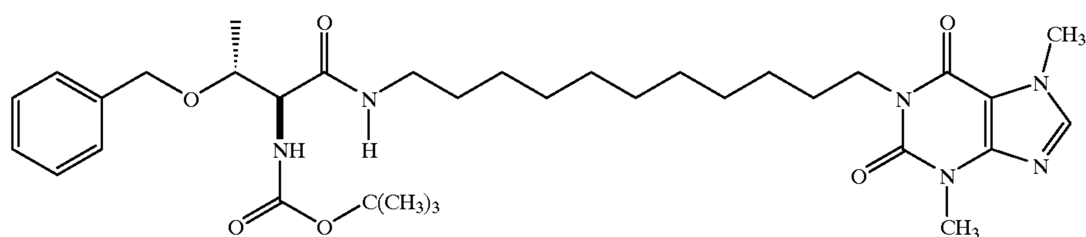
(S)-1-[11-(2-Carbobutoxyamino-3-benzyloxybutyronamido)-undecyl]-3,7-dimethylxanthine
