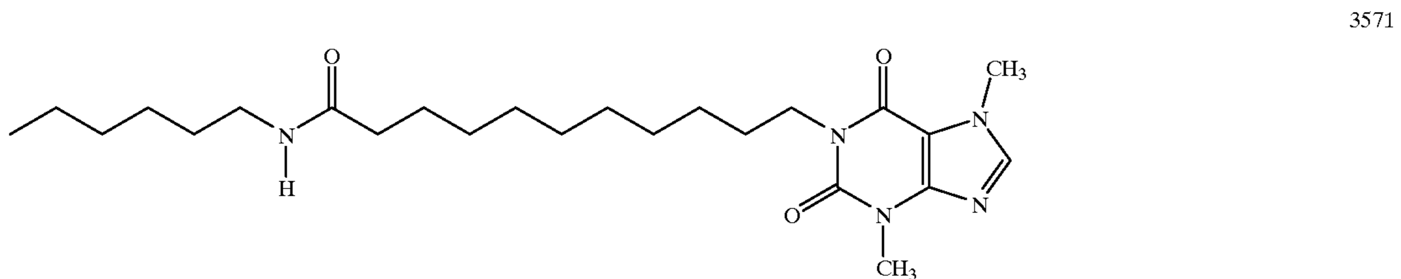
1-(N-Hexyl-11-yl-undecanamide)-3, 7-dimethylxanthine
