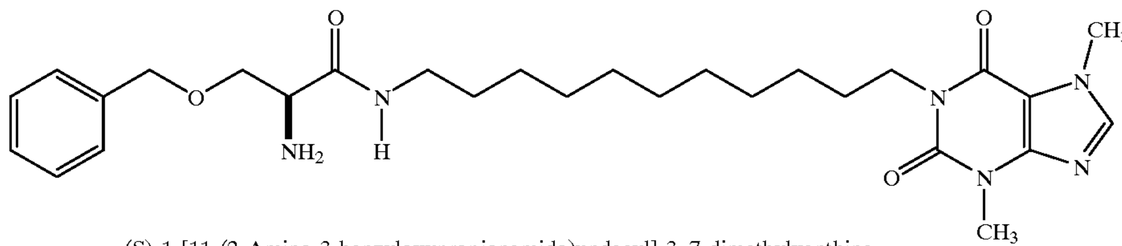
(S)-1-[11-(2-Amino-3-benzyloxypropionamido)undecyl]-3,7-dimethylxanthine
