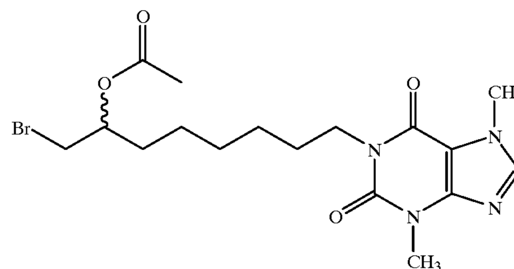
1-(7-Acetoxy-8-bromooctyl)-3,7-dimethylxanthine
