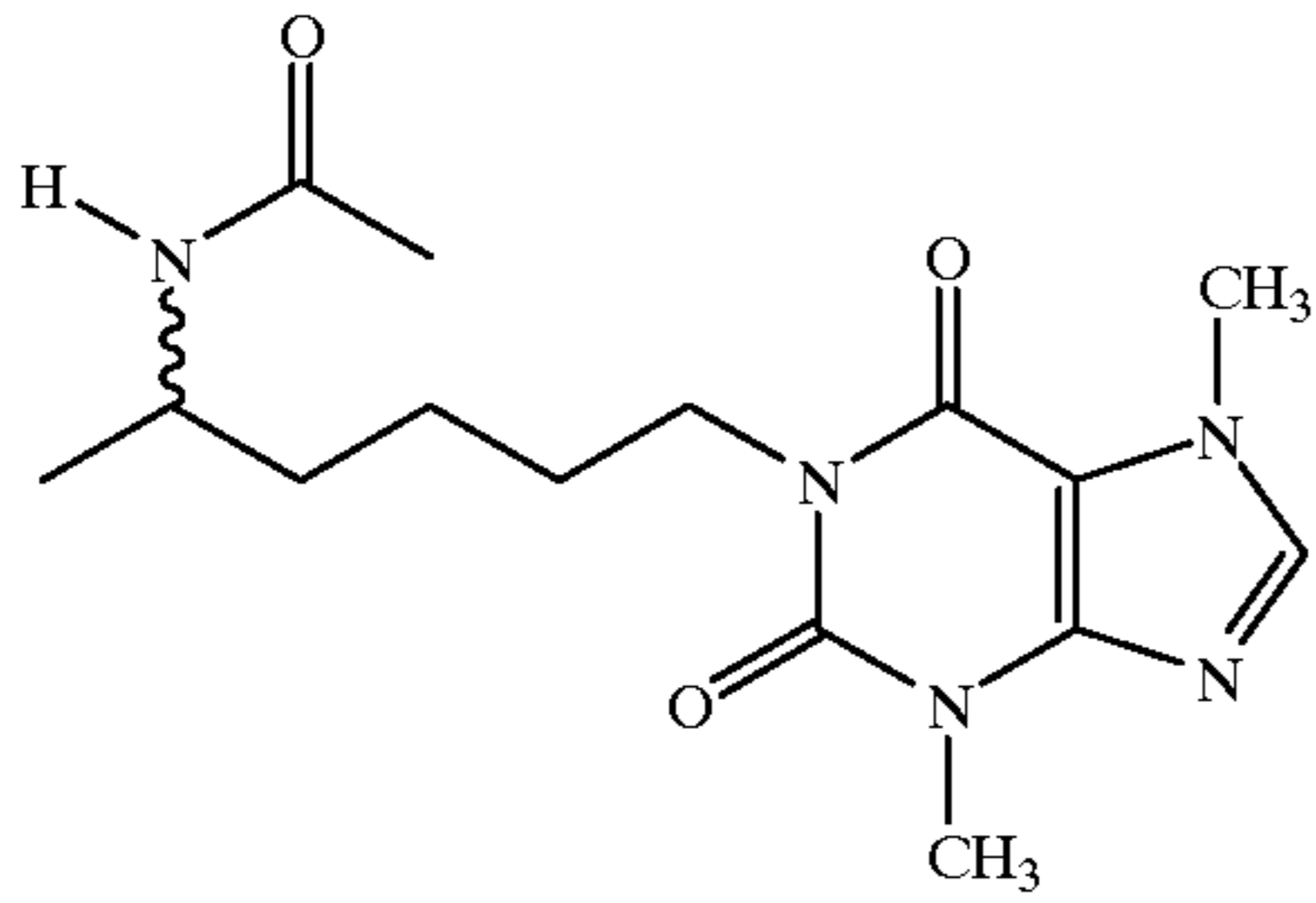
1-(5-Acetamidohexyl)-3,7-dimethylxanthine
