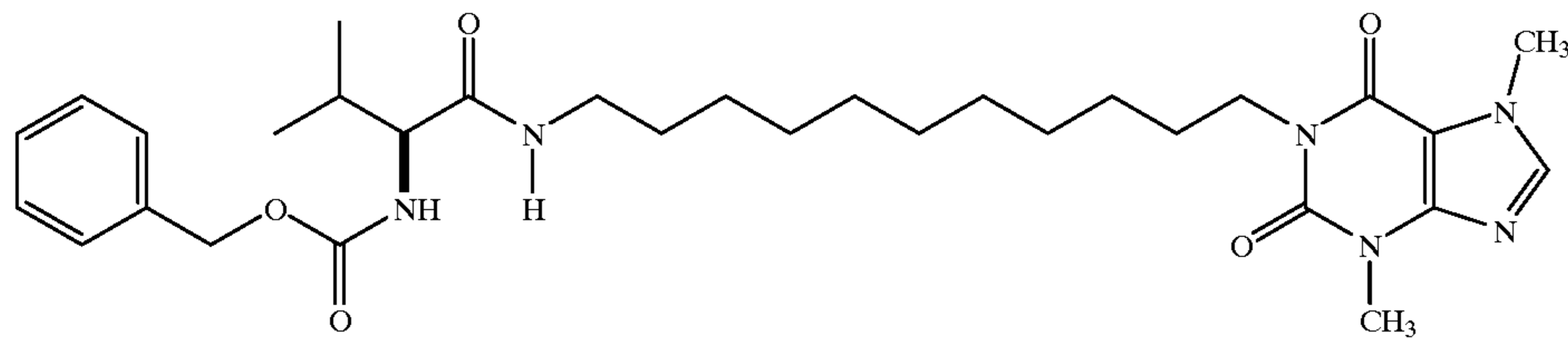
1-[11-(2-Carbobenzyloxyamino-3-methylbutyramido)undecyl]-3,7-dimethylxanthine
