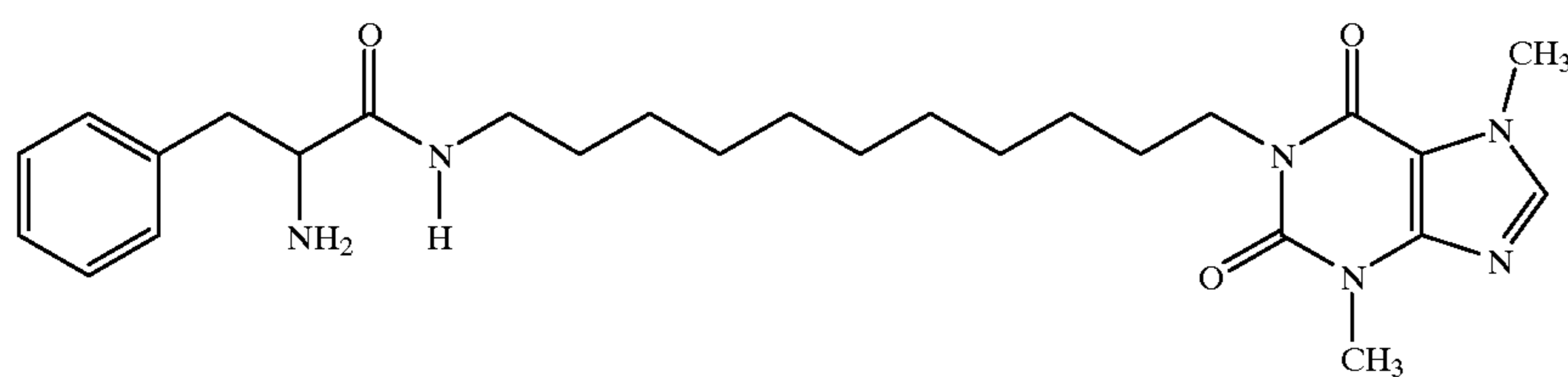
(S)-1-[11-(2-Amino-3-phenylpropionamido)undecyl]-3,7-dimethylxanthine
