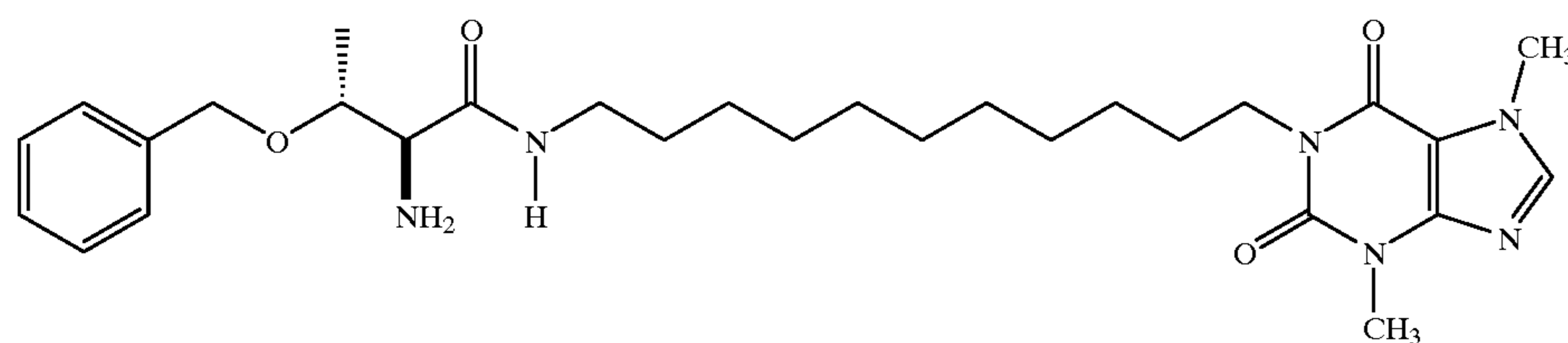
(S)-1-[11-(2-Amino-3-benzyloxybutyronamido)undecyl]-3,7-dimethylxanthine
