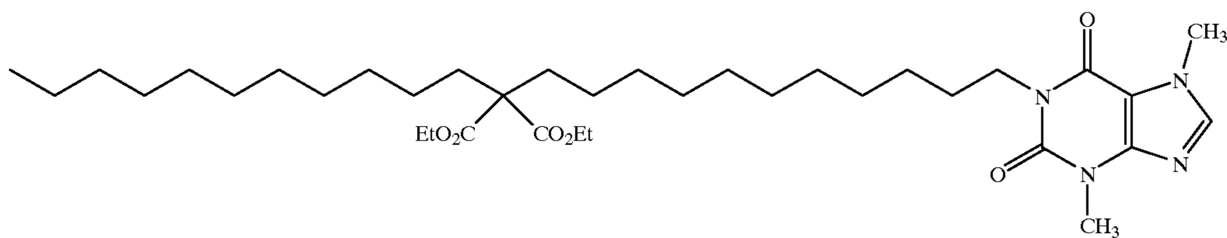
1-[12,12-bis(Ethoxycarbonyl)tricosanyl]-3,7-dimethylxanthine
