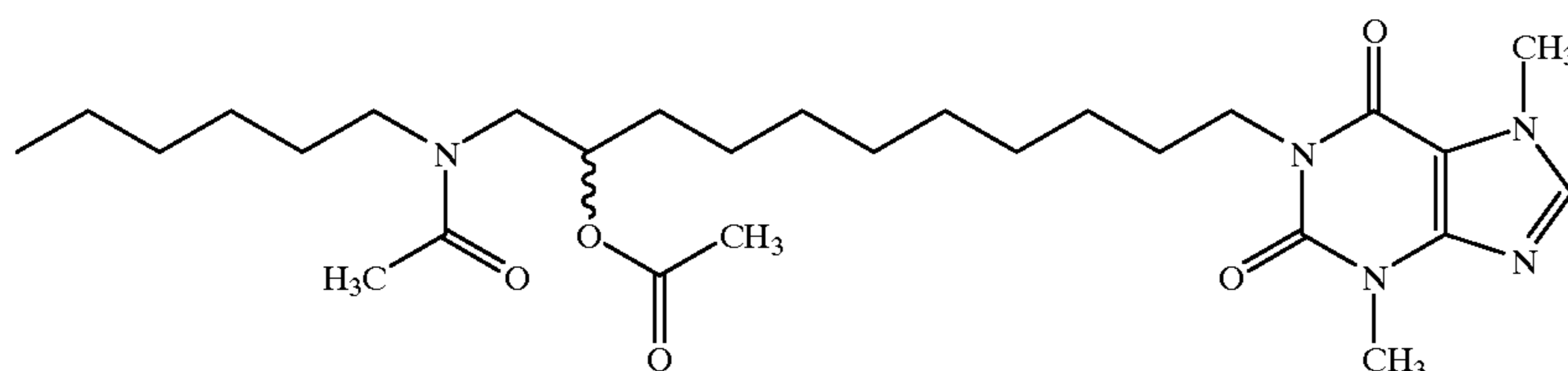
1-[11-(N-Hexylacetamido)-10-acetoxyundecyl]-3,7-dimethylxanthine
