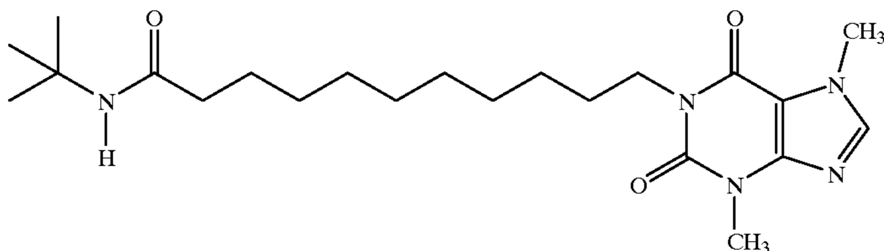
1-[(N-tert-Butyl)-11-yl-undecanamide]-3,7-dimethylxanthine
