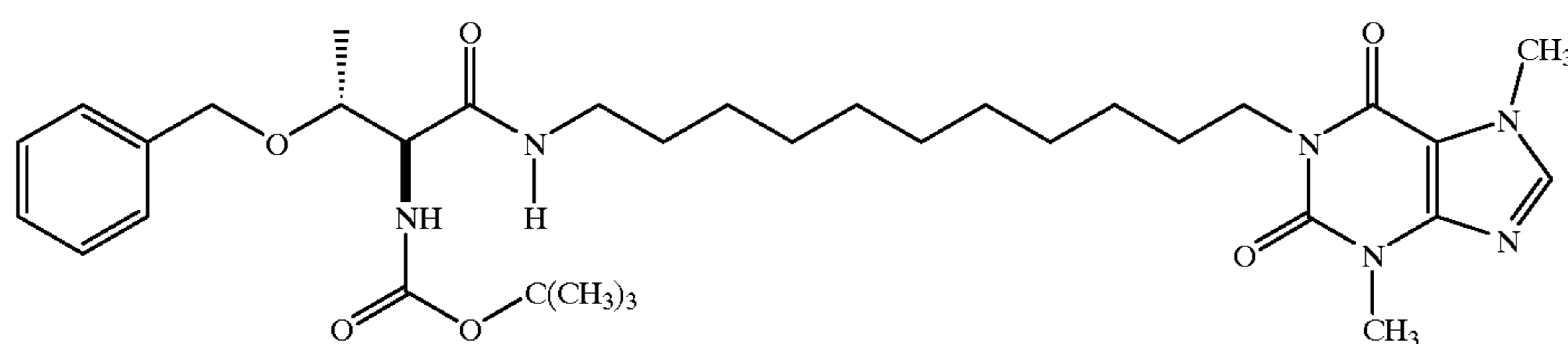
(S)-1-[11-(2-Carbobutoxyamino-3-benzyloxybutyronamido)-undecyl]-3, 7-dimethylxanthine
