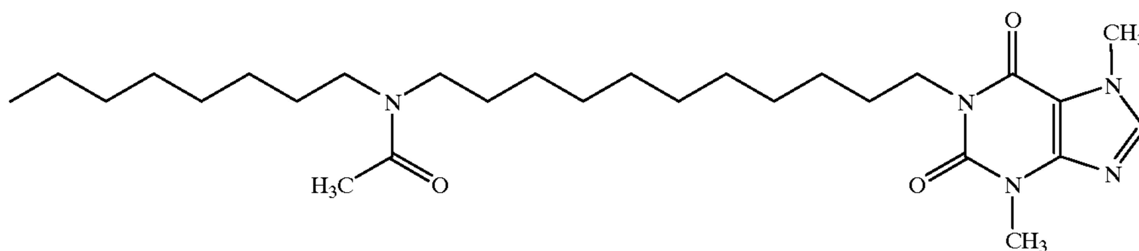
1-[11-(N-Octyl acetamido)undecyl]-3,7-dimethylxanthine
