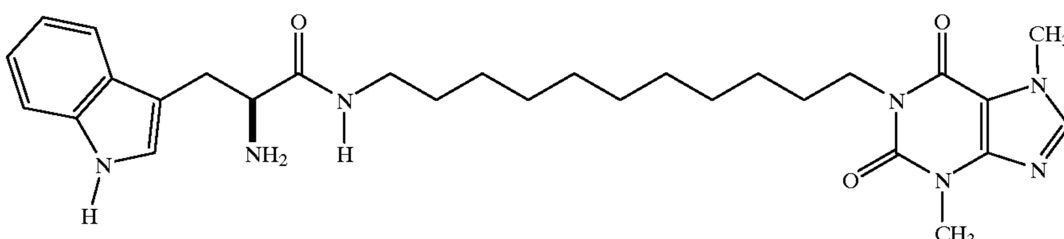
1-(11-[2-Amino-3-(3-indolyl)propionamido]undecyl)-3,7-dimethylxanthine
