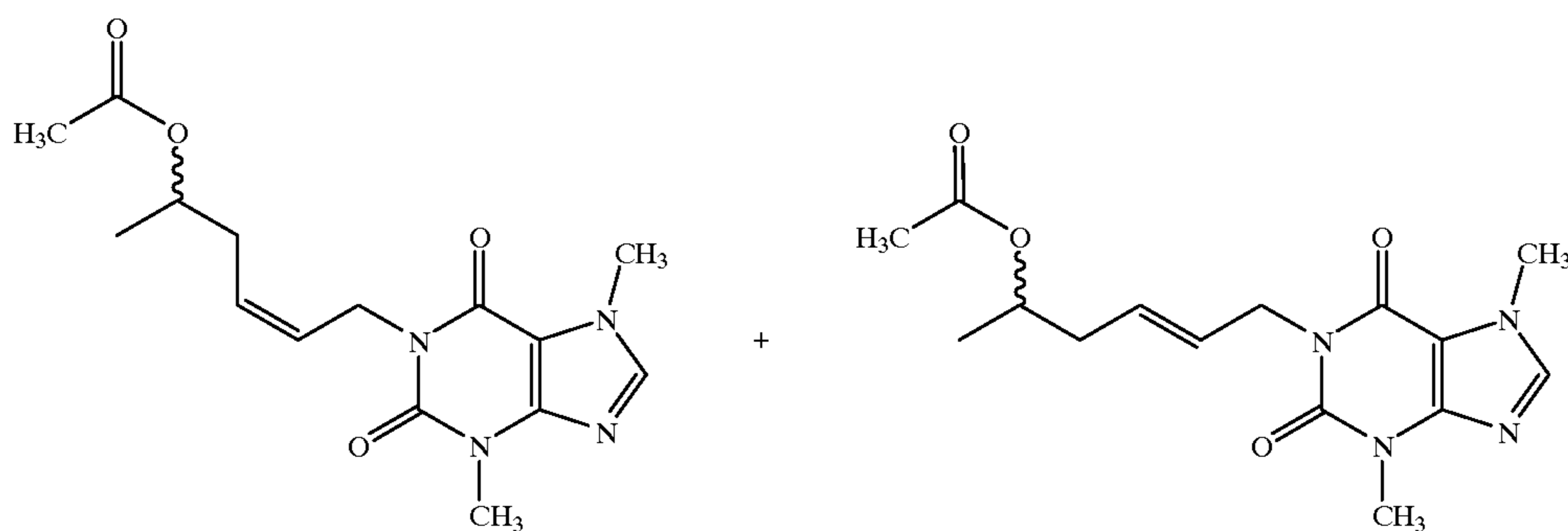
1-[5-Acetoxyhex-3-enyl]-3,7-dimethylxanthine
