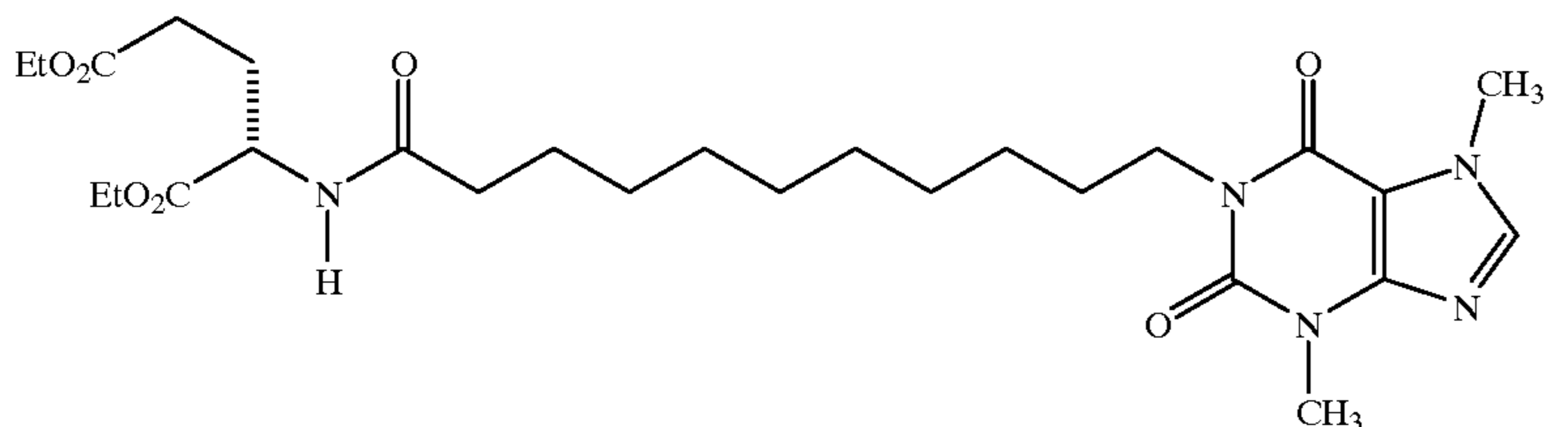
1-(11-[1,3-Bis(ethoxycarbonyl)propylamino]-11-oxoundecyl)-3,7-dimethylxanthine
