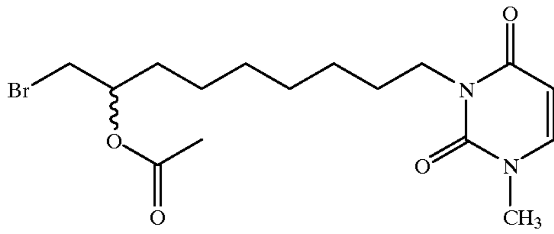
3-(8-Acetoxy-9-bromononyl)-1-methyluracil
