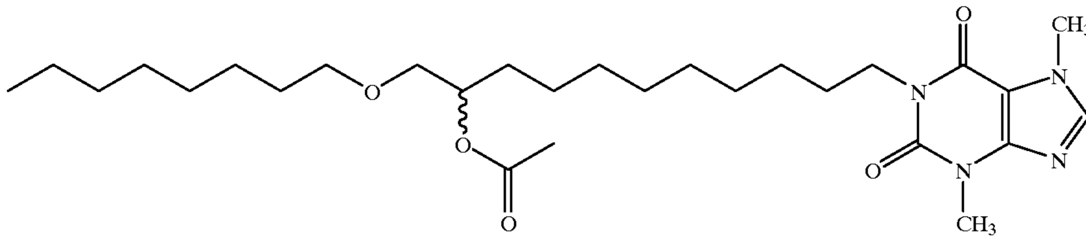
1-(11-Octoxy-10-acetoxyundecyl)-3, 7-dimethylxanthine
