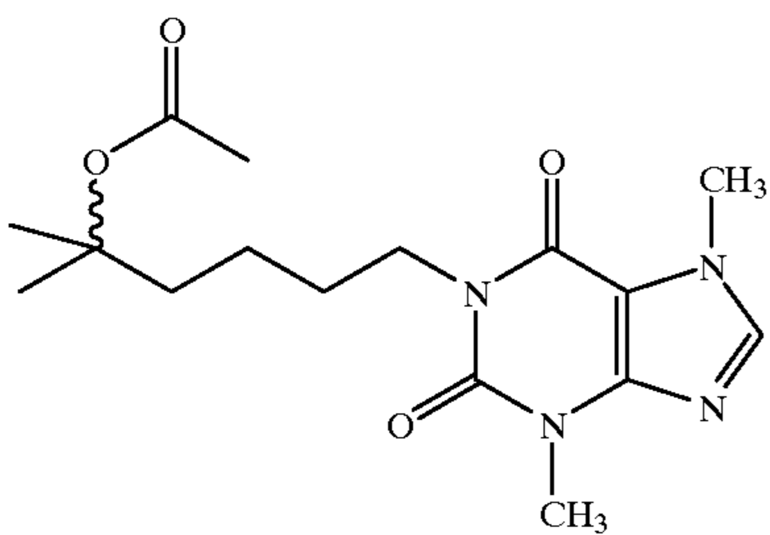
1-(5-Acetoxy-4-methylpentyl)-3,7-dimethylxanthine
