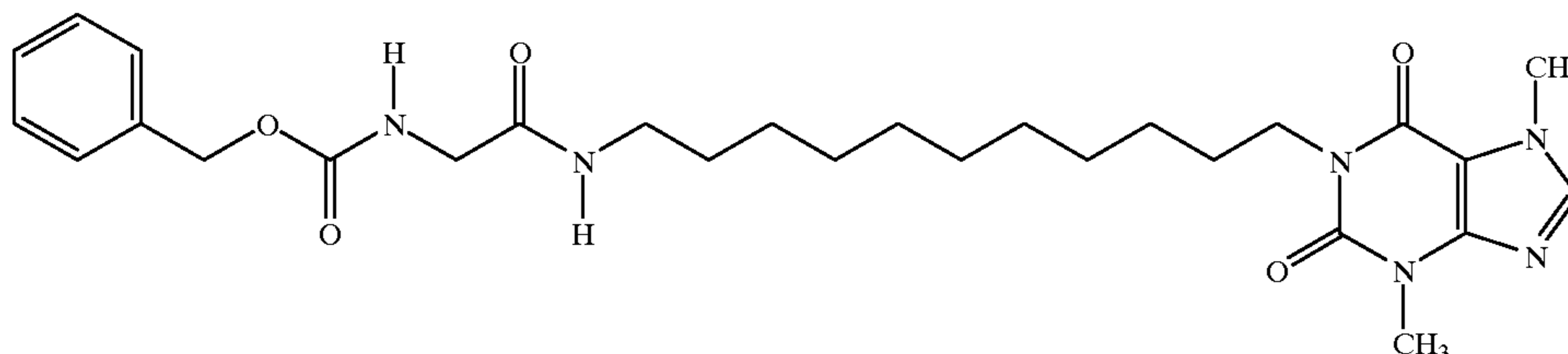
1-[11-(Carbobenzyloxyaminoacetamido)undecyl]-3, 7-dimethylxanthine
