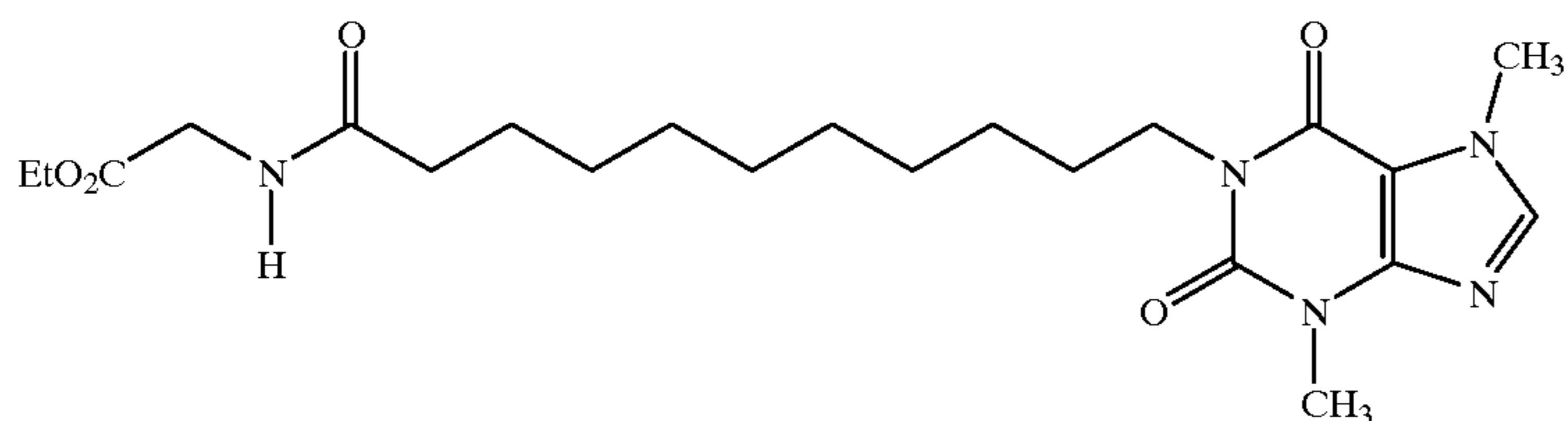
1-[11-(Ethoxycarbonylmethylamino)-11-oxoundecyl]-3,7-dimethylxanthine
