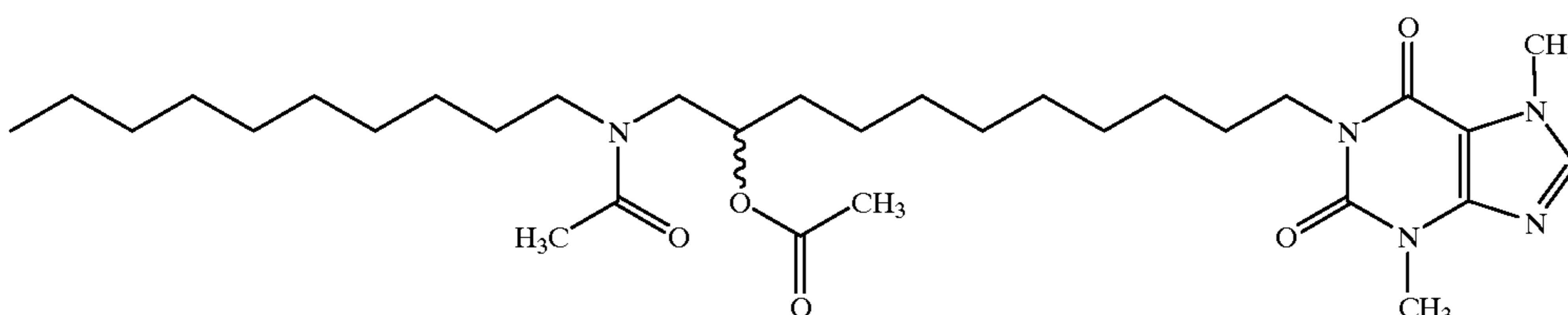
1-[11-(N-Decylacetamido)-10-acetoxyundecyl]-3,7-dimethylxanthine
