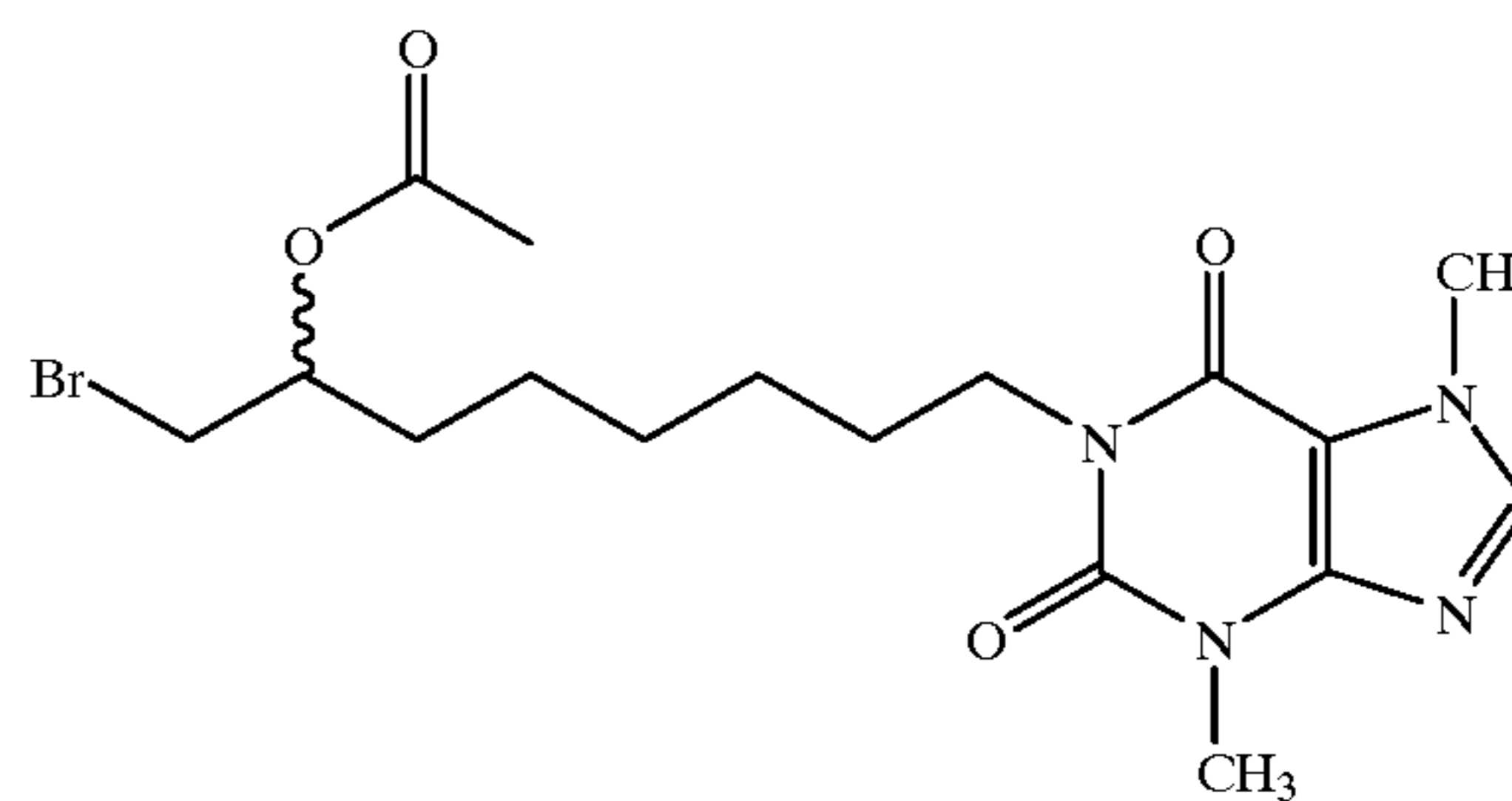
1-(7-Acetoxy-8-bromooctyl)-3,7-dimethylxanthine
