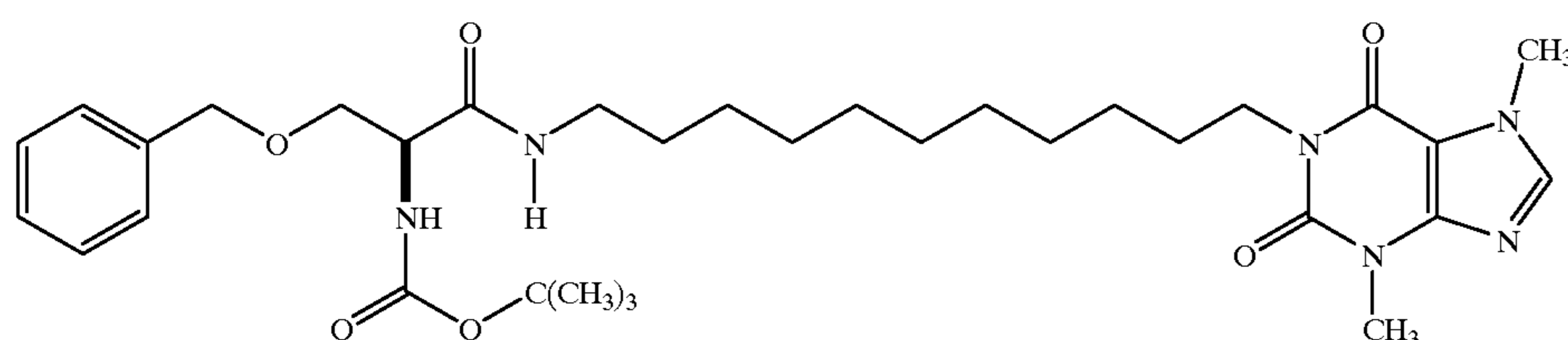
(S)-1-[11-(2-Carbobutoxyamino-3-benzyloxypropionamido)-undecyl]-3, 7-dimethylxanthine
