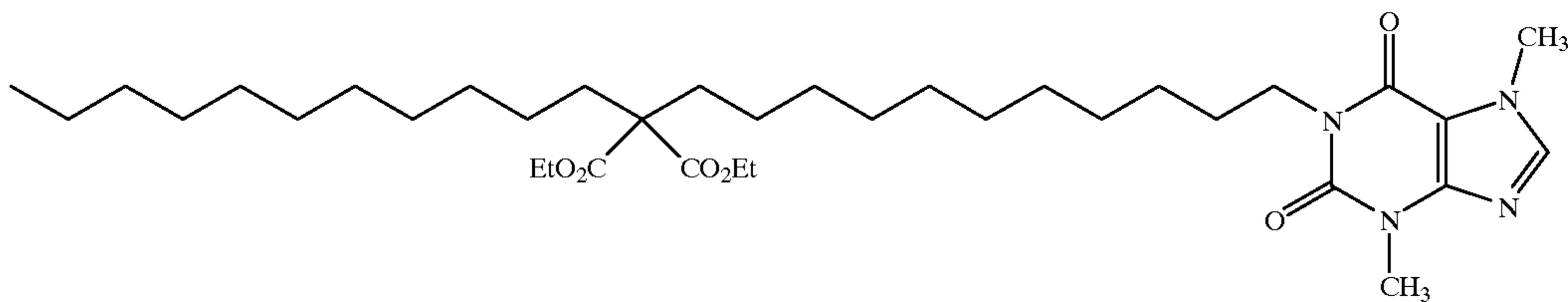
1-[12,12-bis(Ethoxycarbonyl)tricosanyl]-3,7-dimethylxanthine
