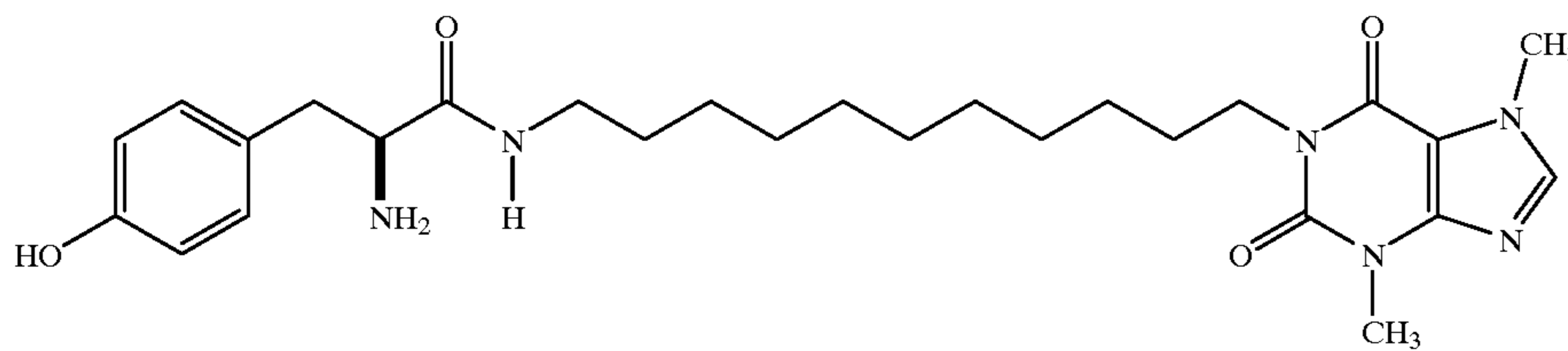
(S)-1-(11-[2-Amino-3-(4-hydroxyphenyl)propionamido]undecyl)-3,7-dimethylxanthine
