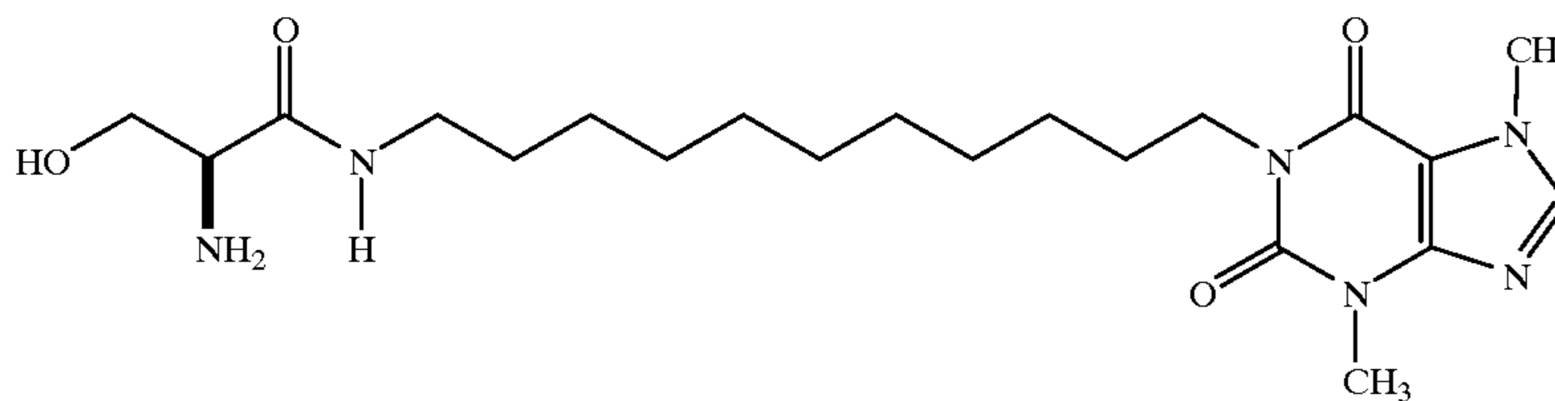
(S)-1-[11-(2-Amino-3-hydroxypropionamido)undecyl]-3,7-dimethylxanthine
