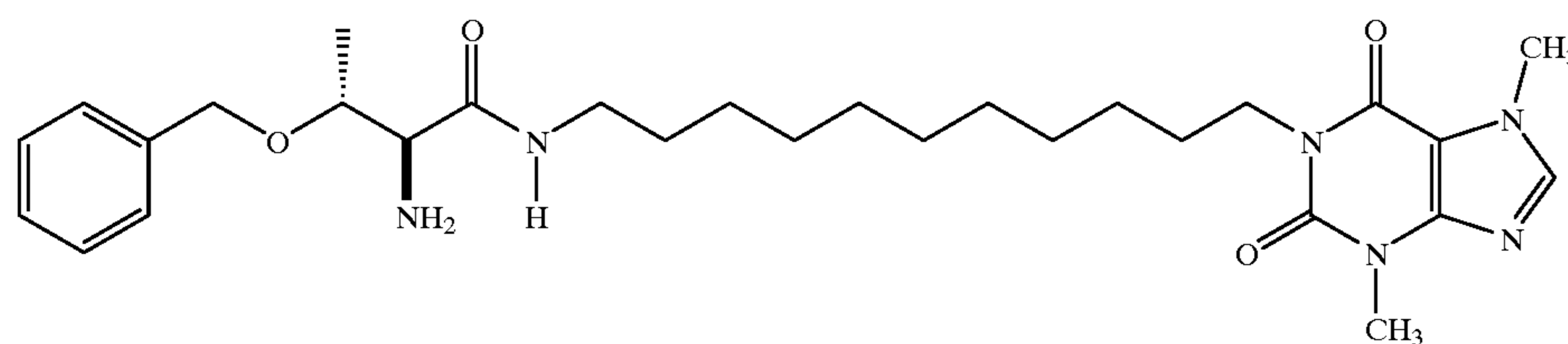
(S)-1-[11-(2-Amino-3-benzyloxybutyronamido)undecyl]-3,7-dimethylxanthine
