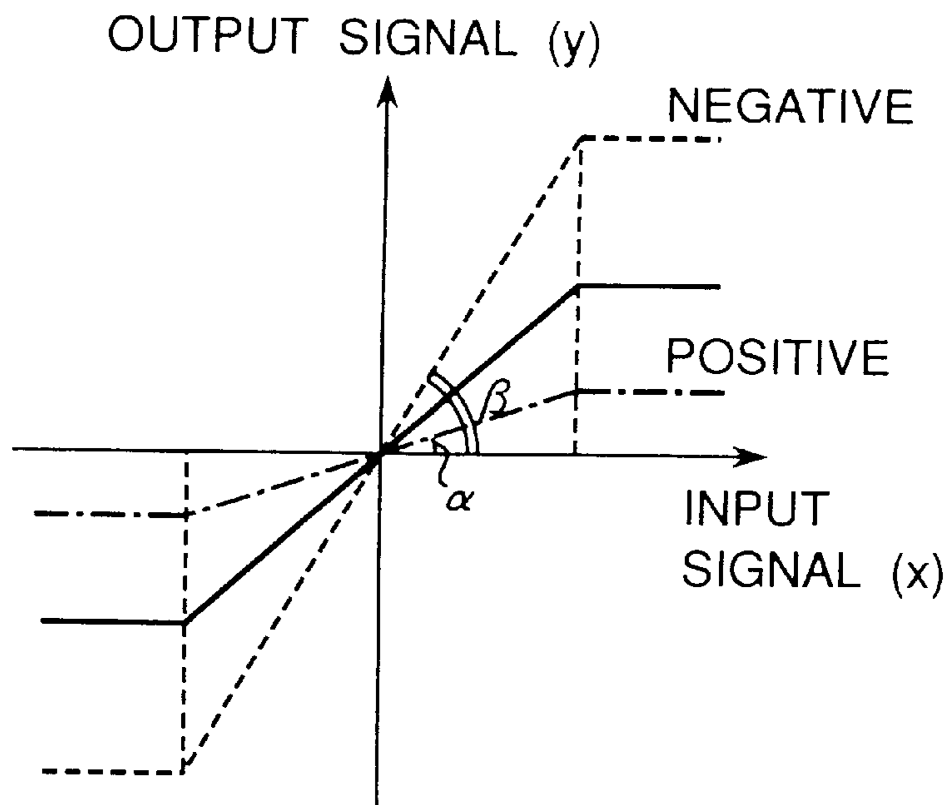
Fig. 18B
