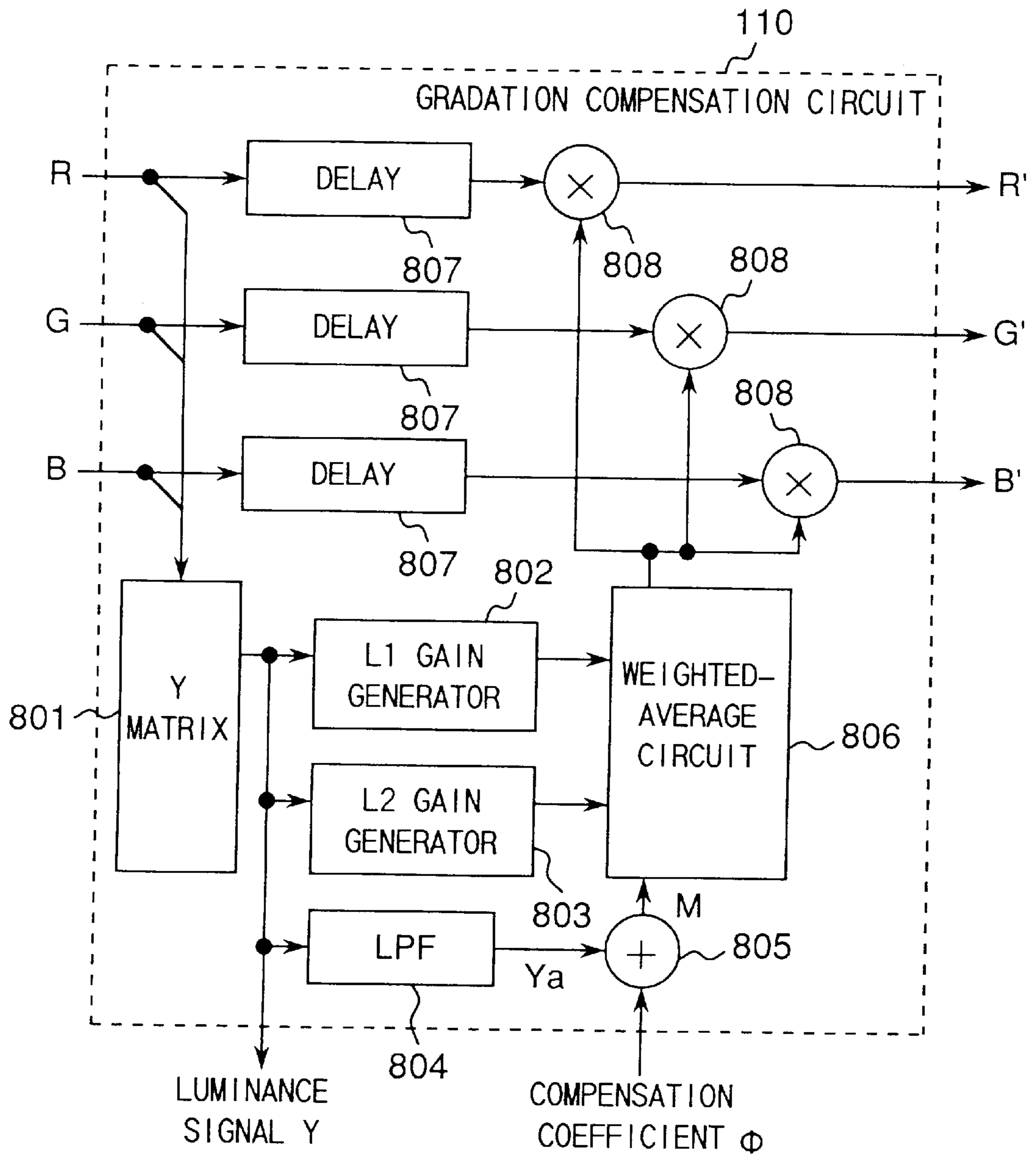
Fig. 9A
