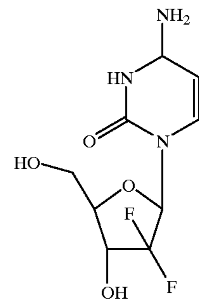
Gemcitabine
