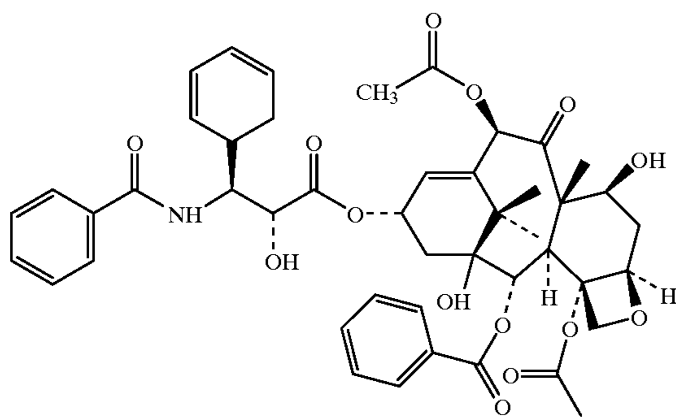
Taxol
