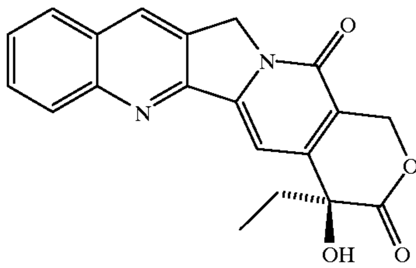
Camptothecin
