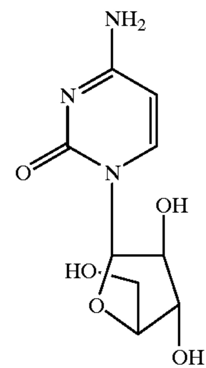
Cytarabine
