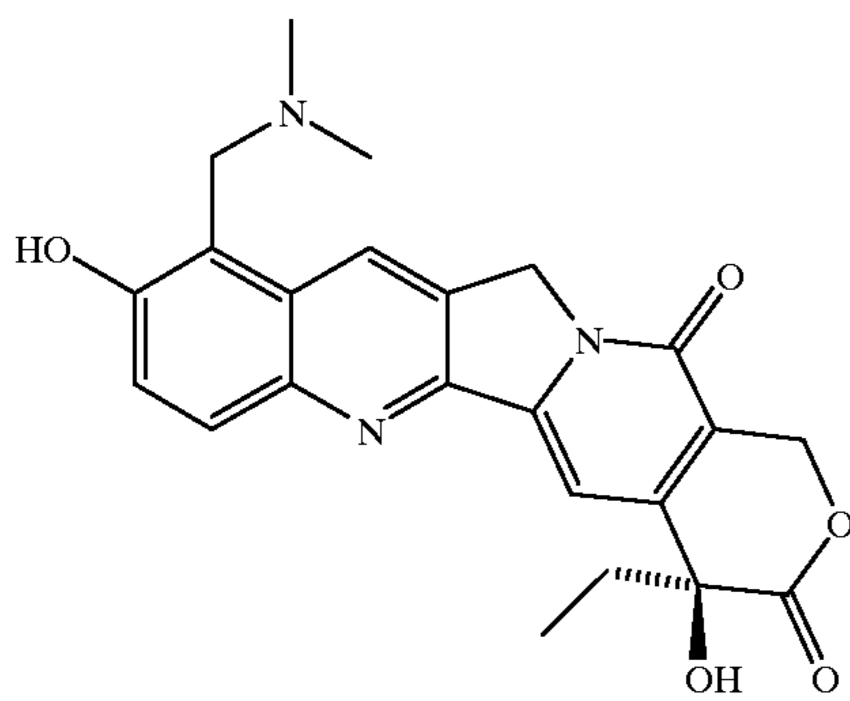
Topotecan
