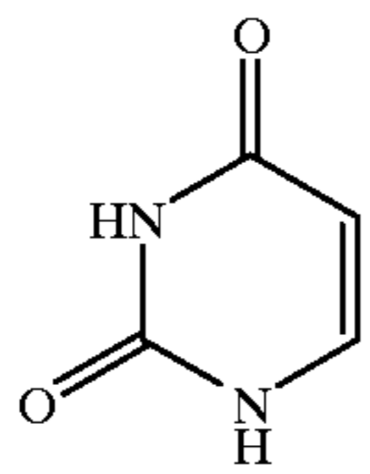
Uracil
