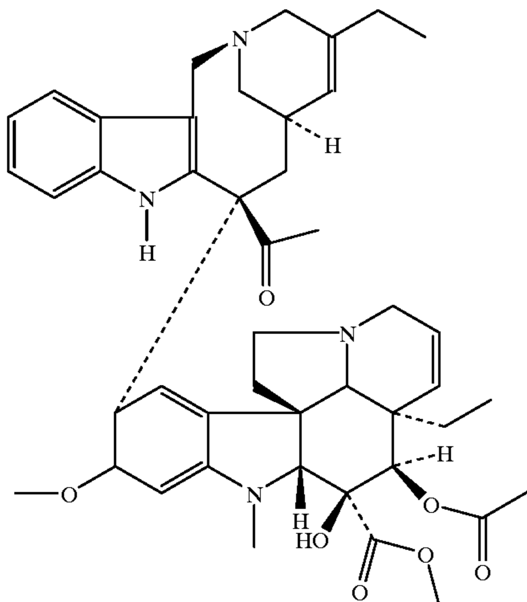
Vinorelbine
