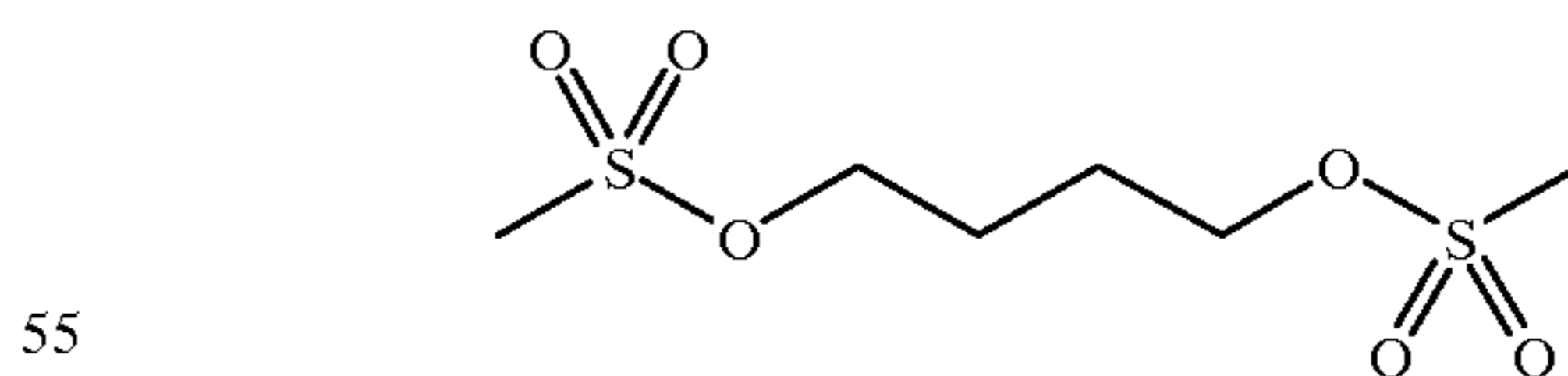
Busulfan
