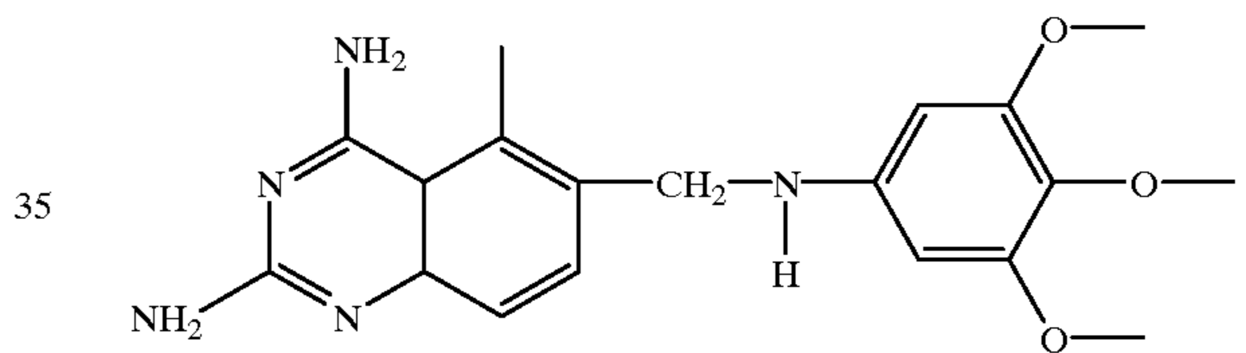
Trimetrexate
