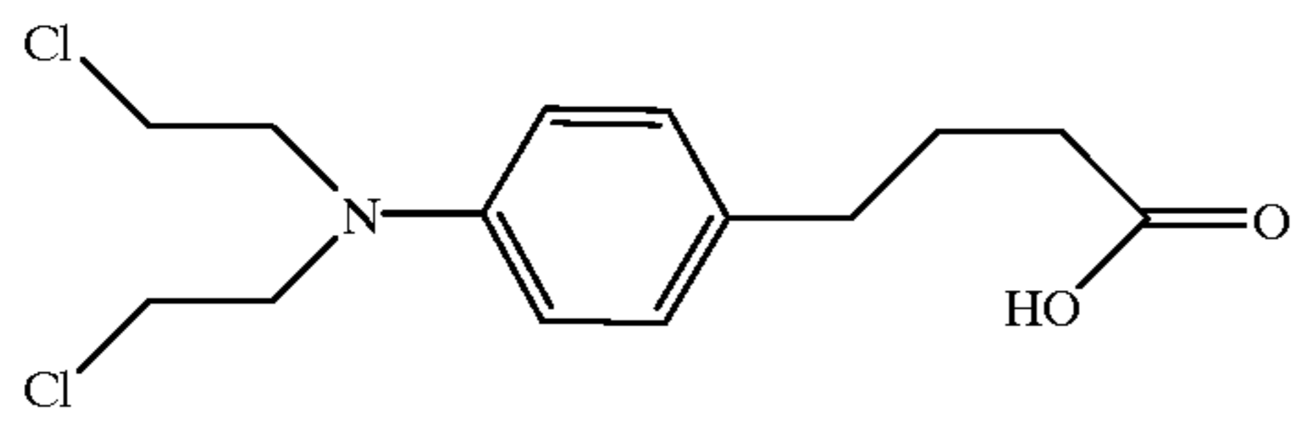
Chlorambucil
