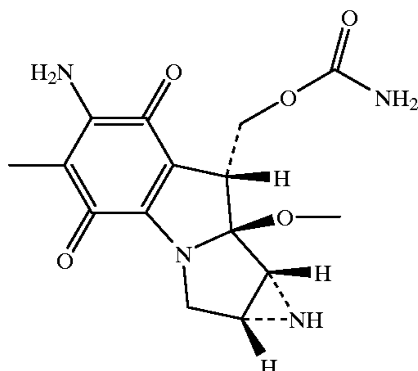
Mitomycin
