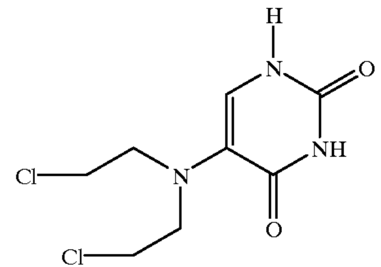
Uracil Mustard
