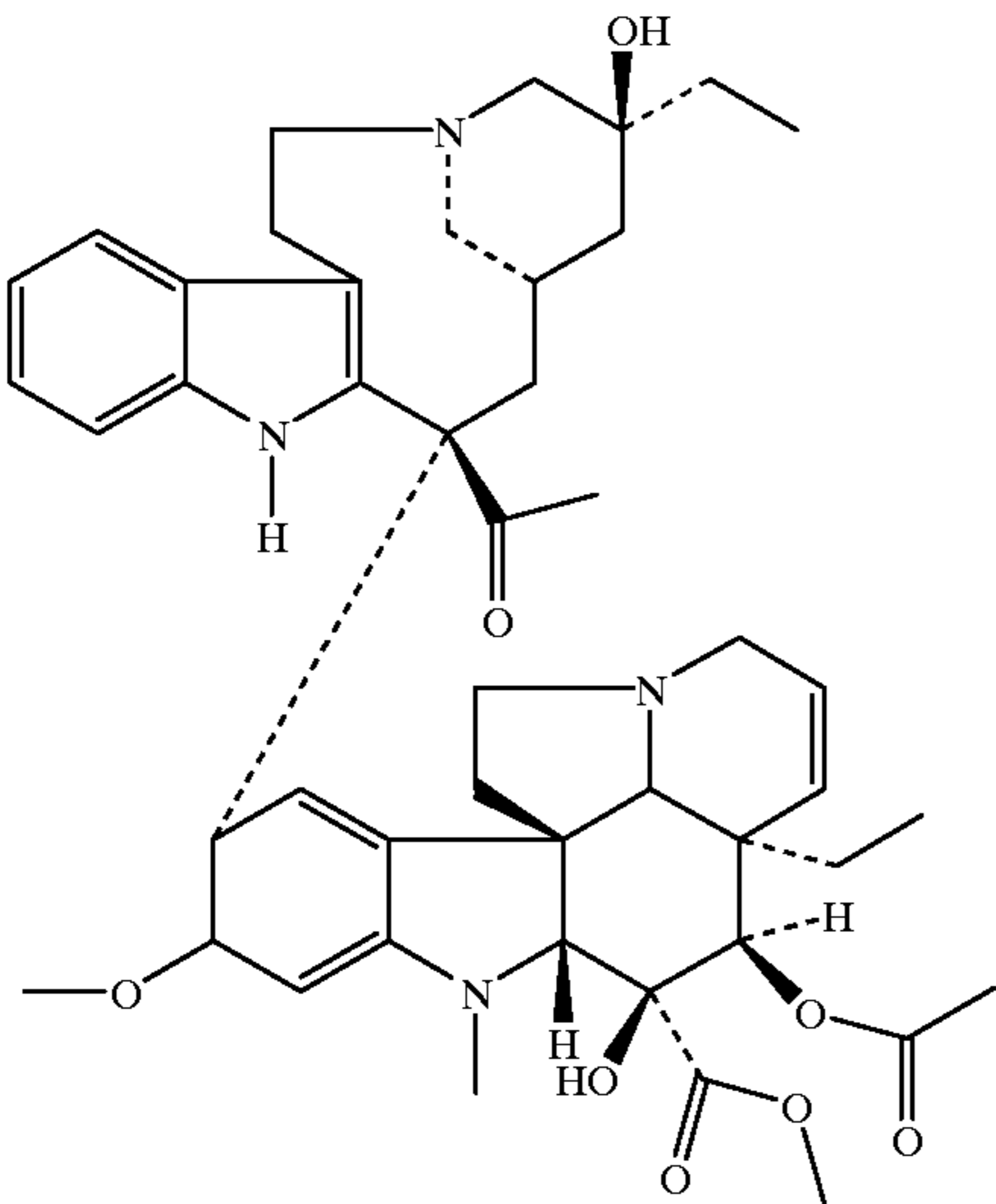
Vinblastine
