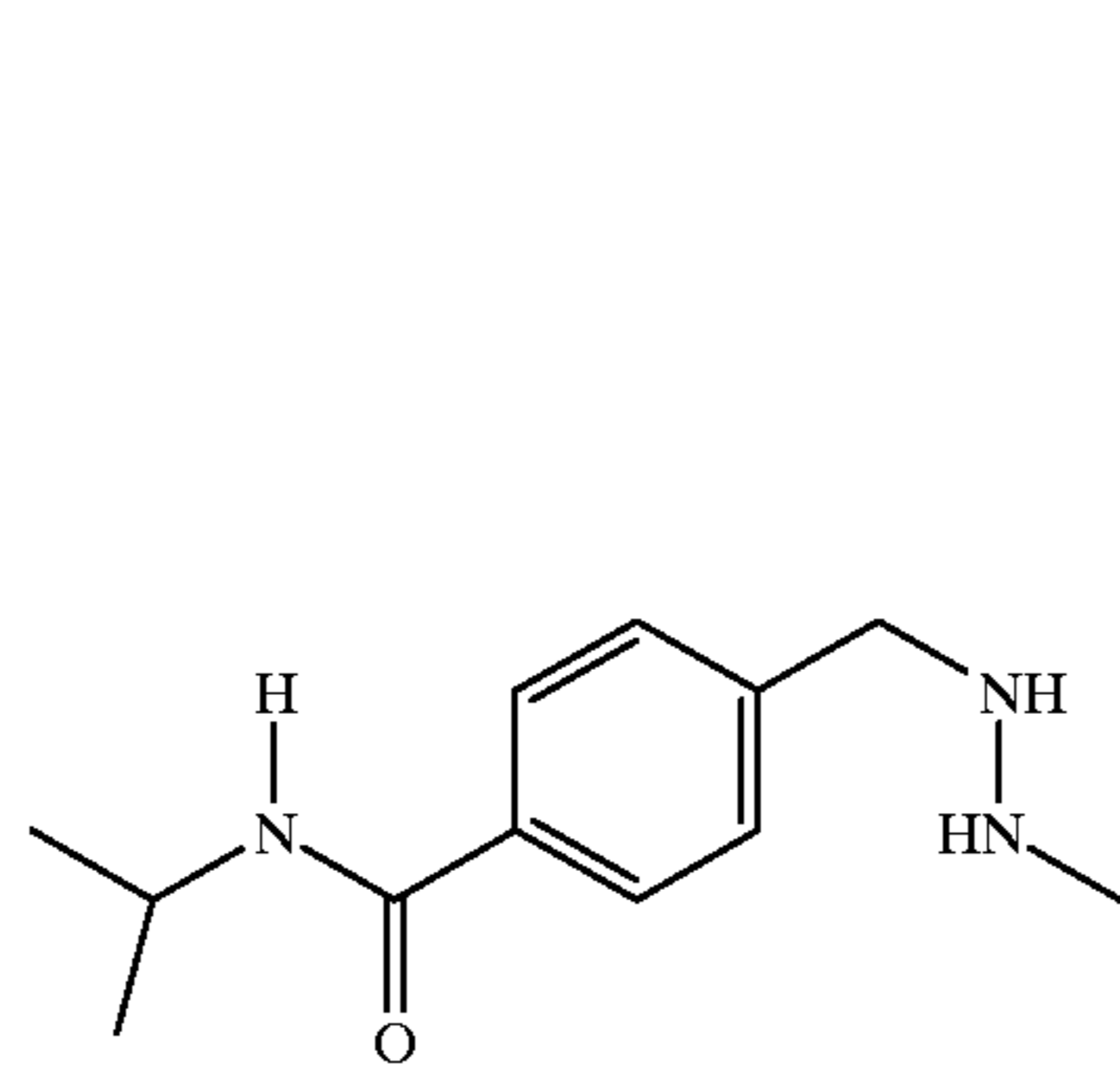
Procarbazine
