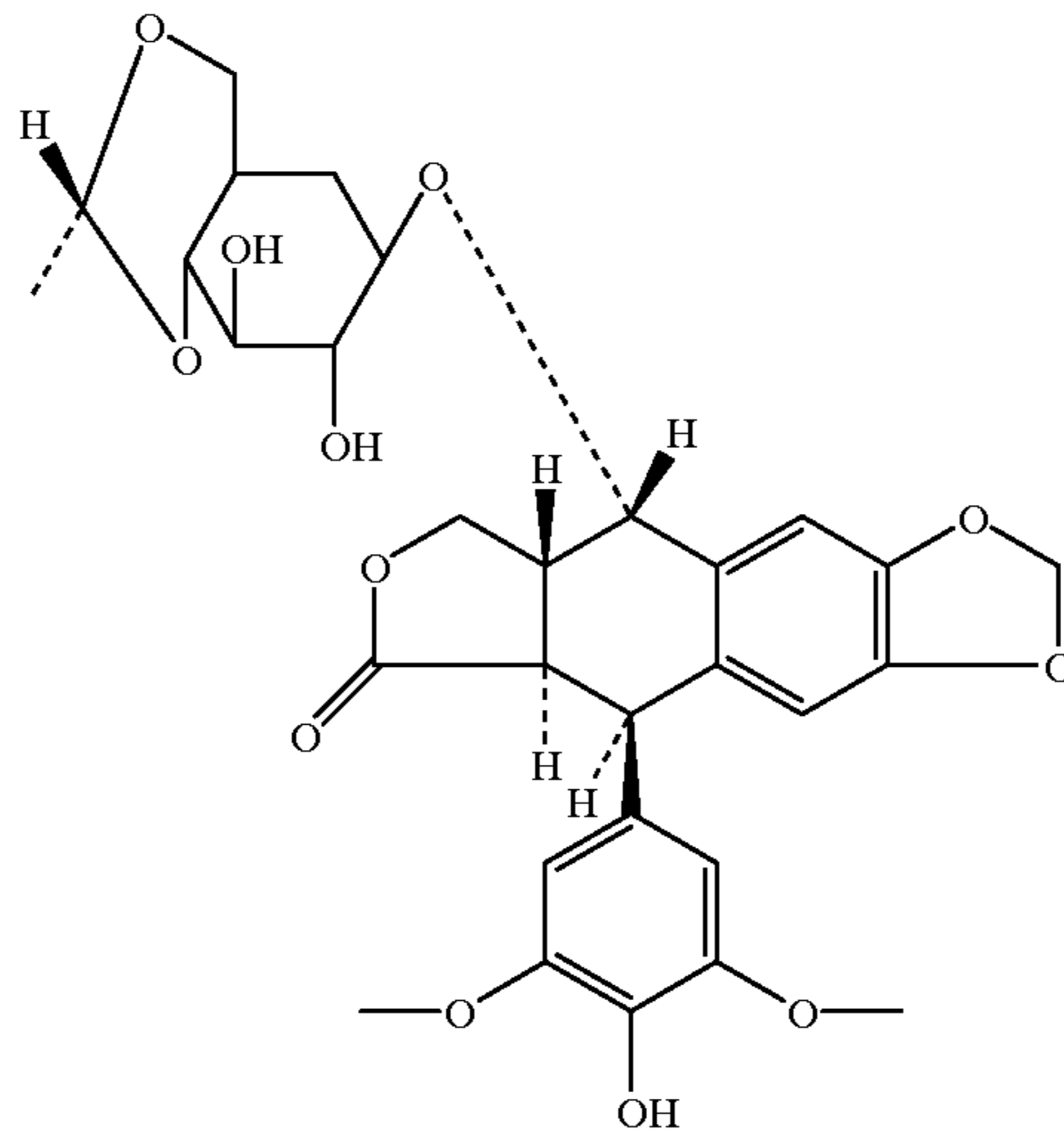
Etoposide
