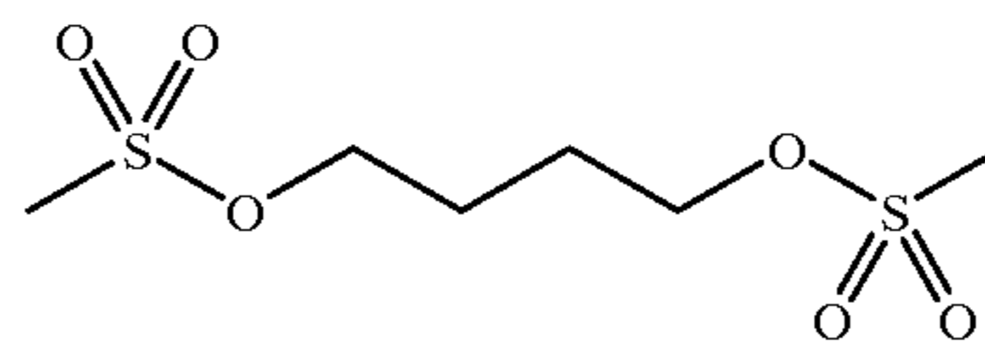
Busulfan
