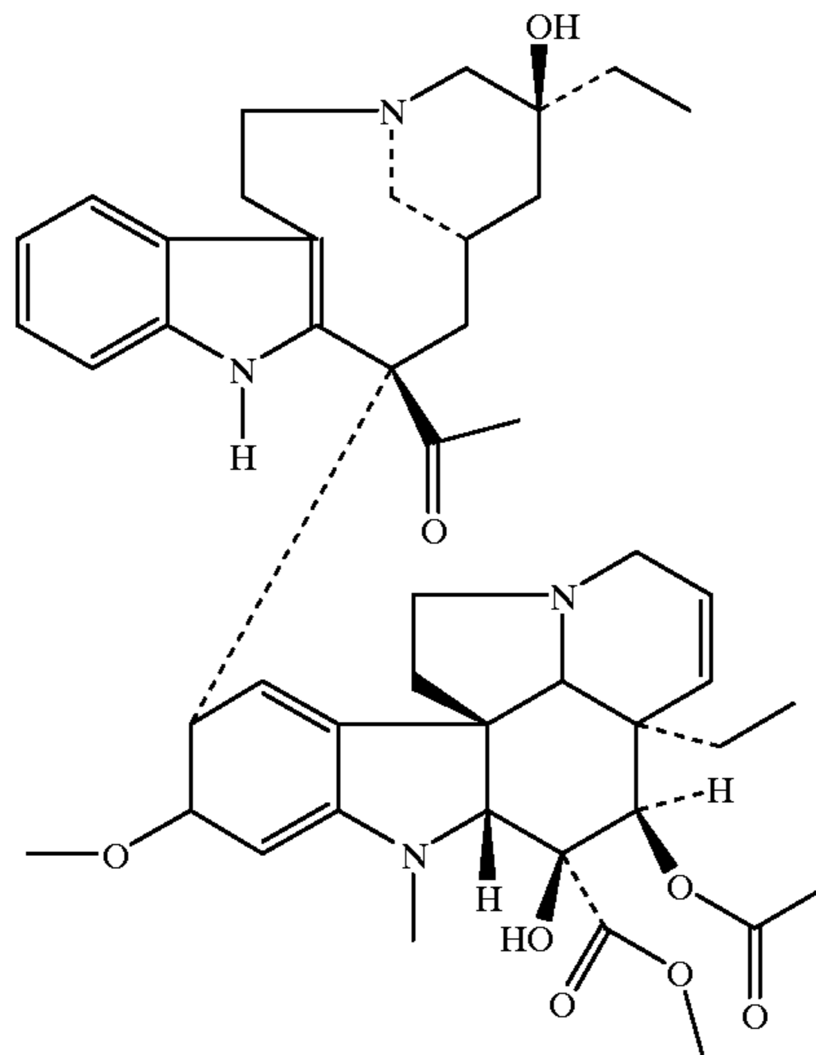
Vinblastine
