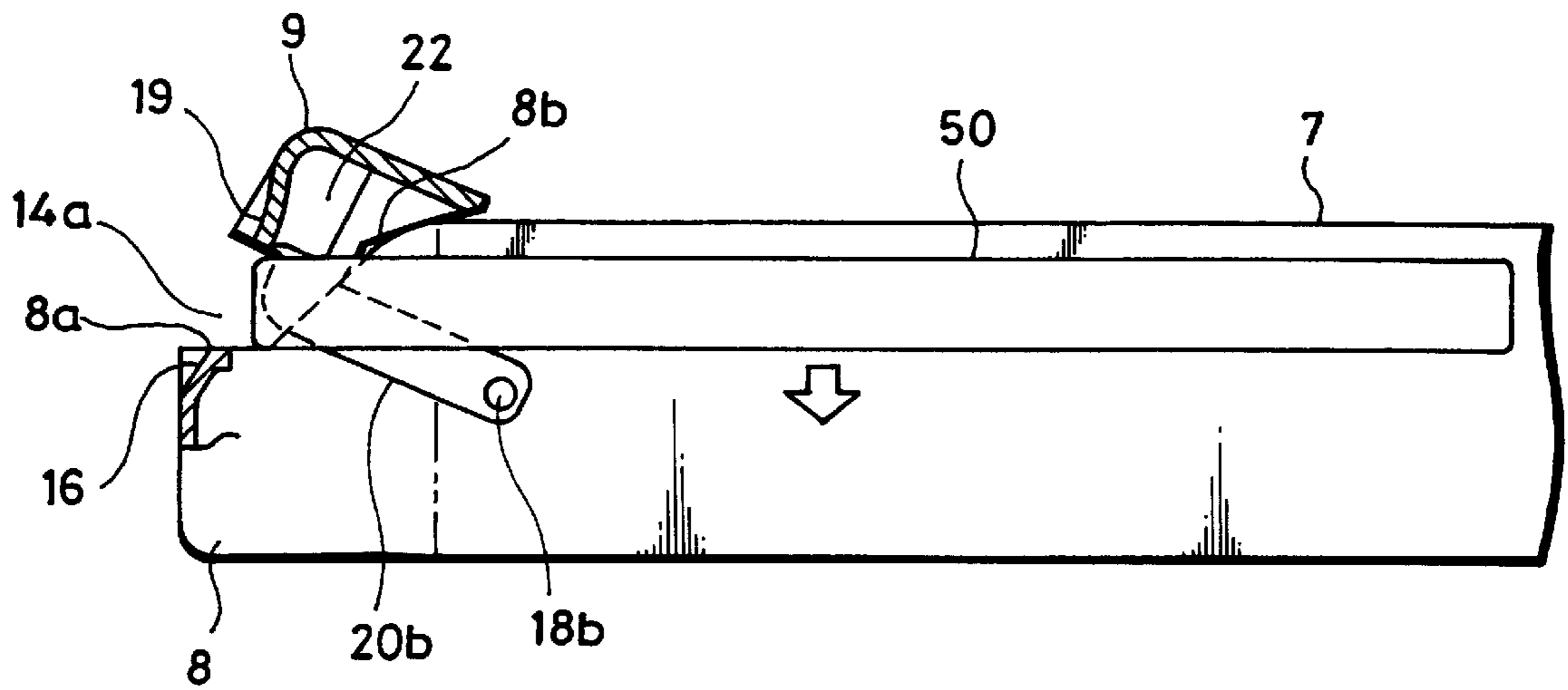
FIG. 9(B)
