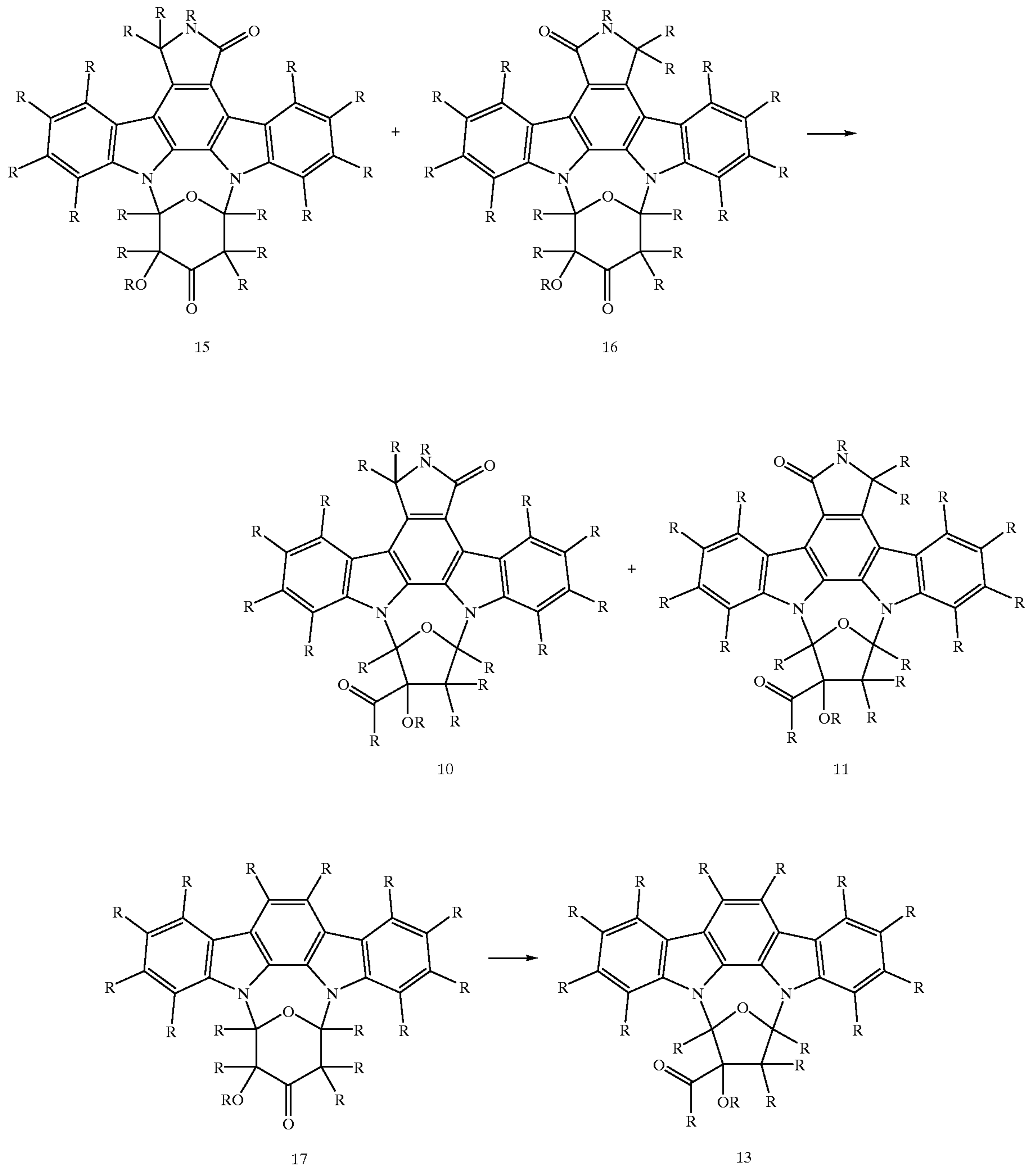
Scheme VI
