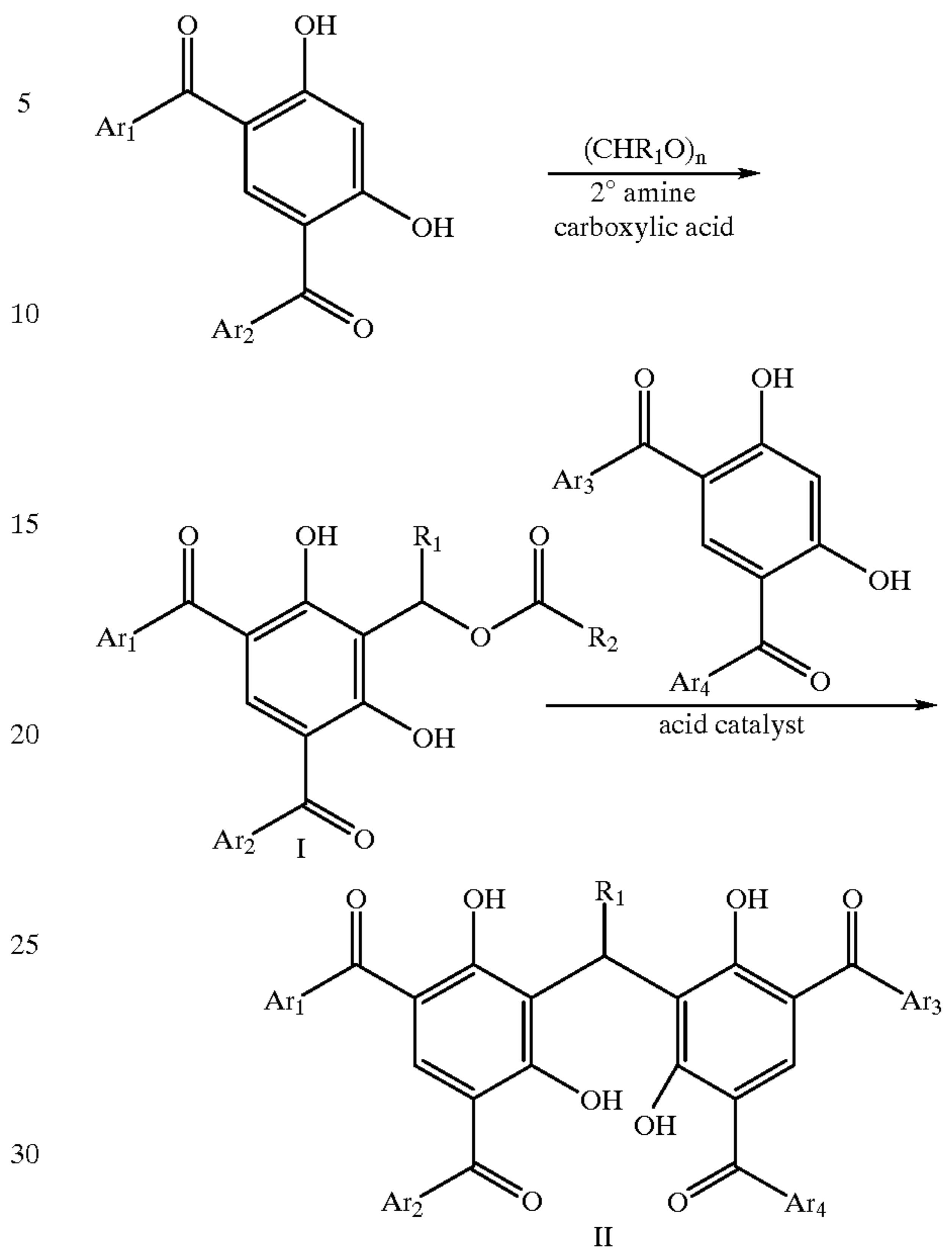
Scheme I.
