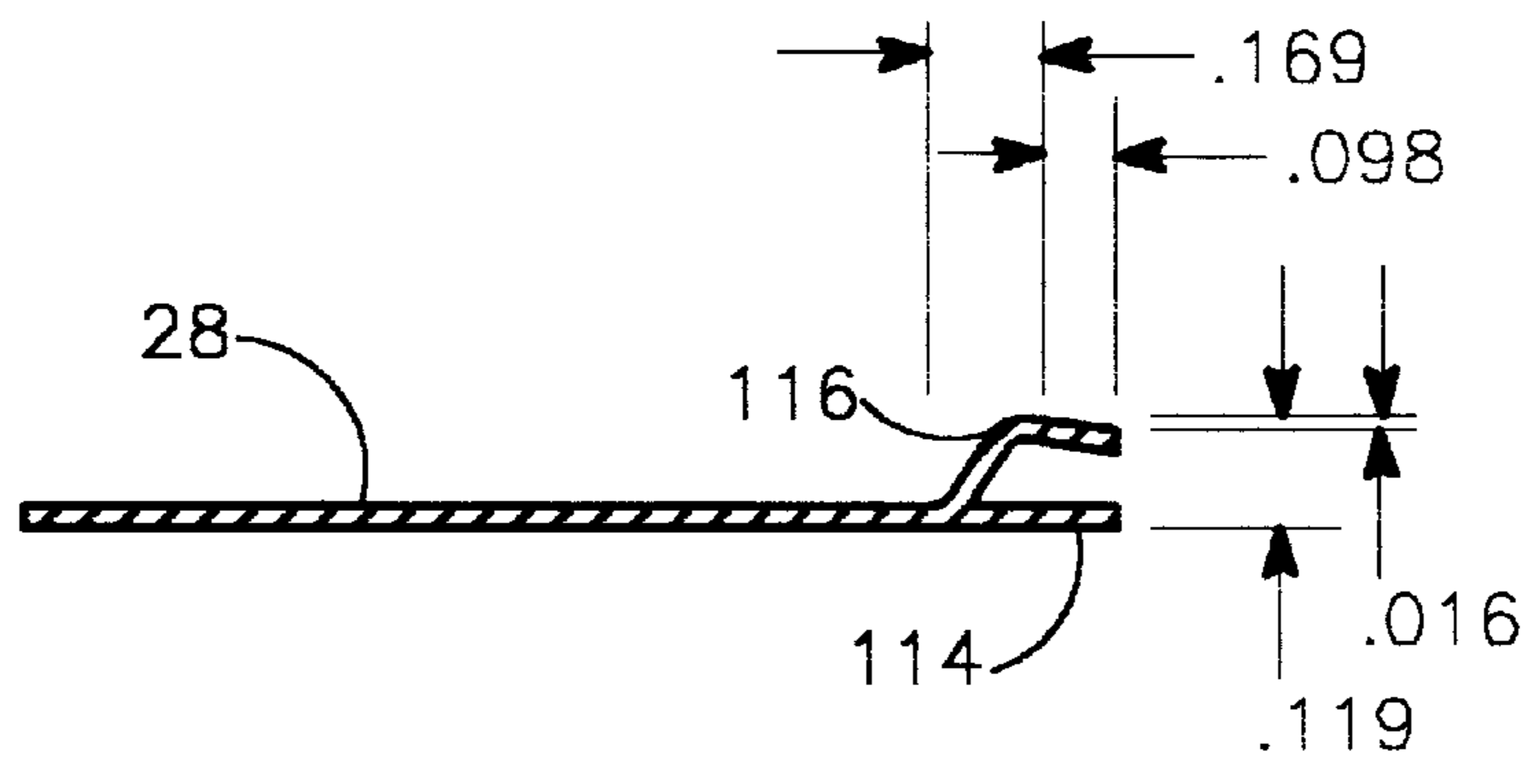
section A-A
