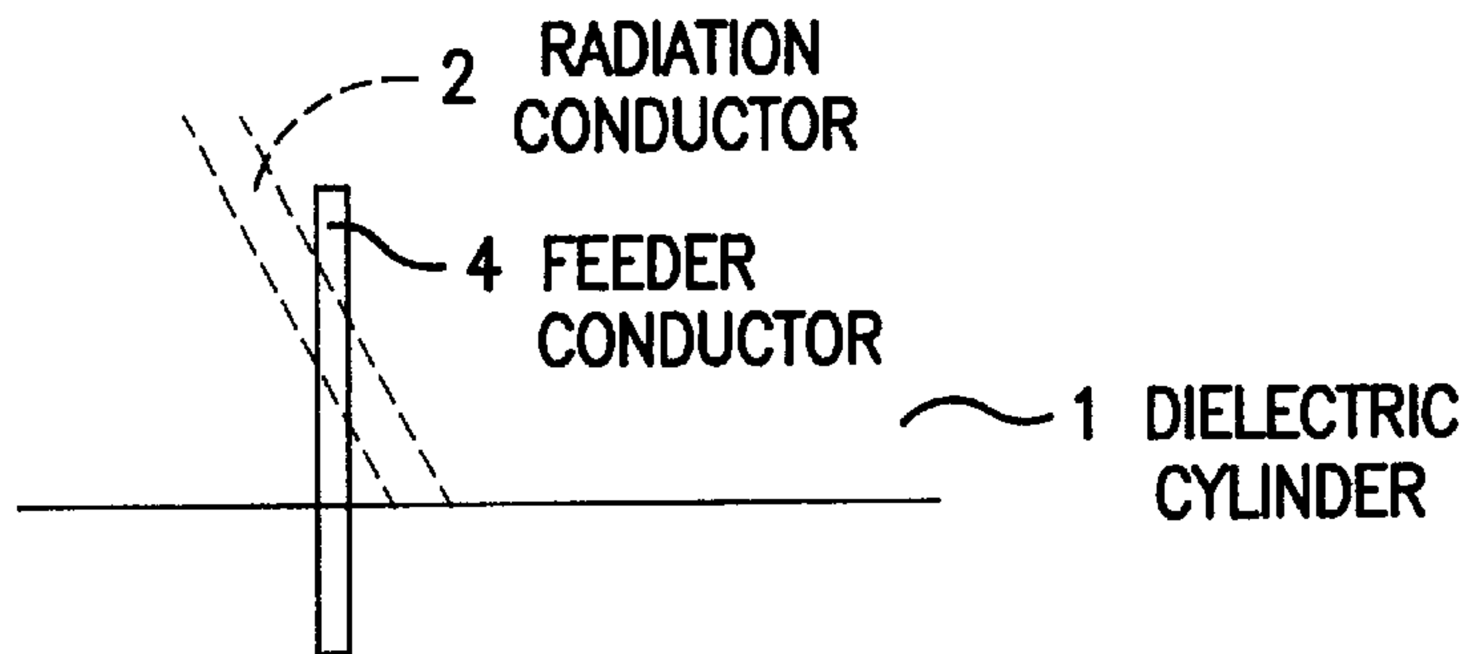
FIG. 4D
