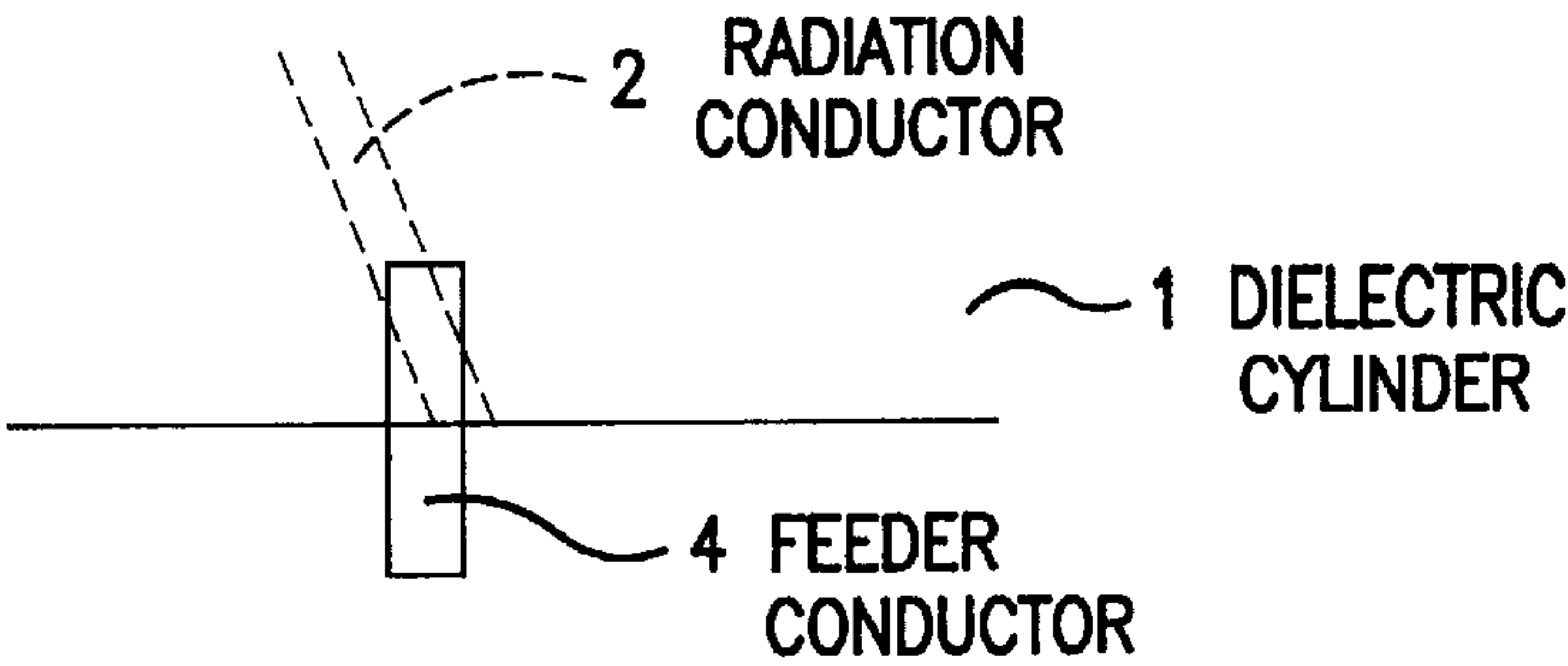
FIG. 4A
