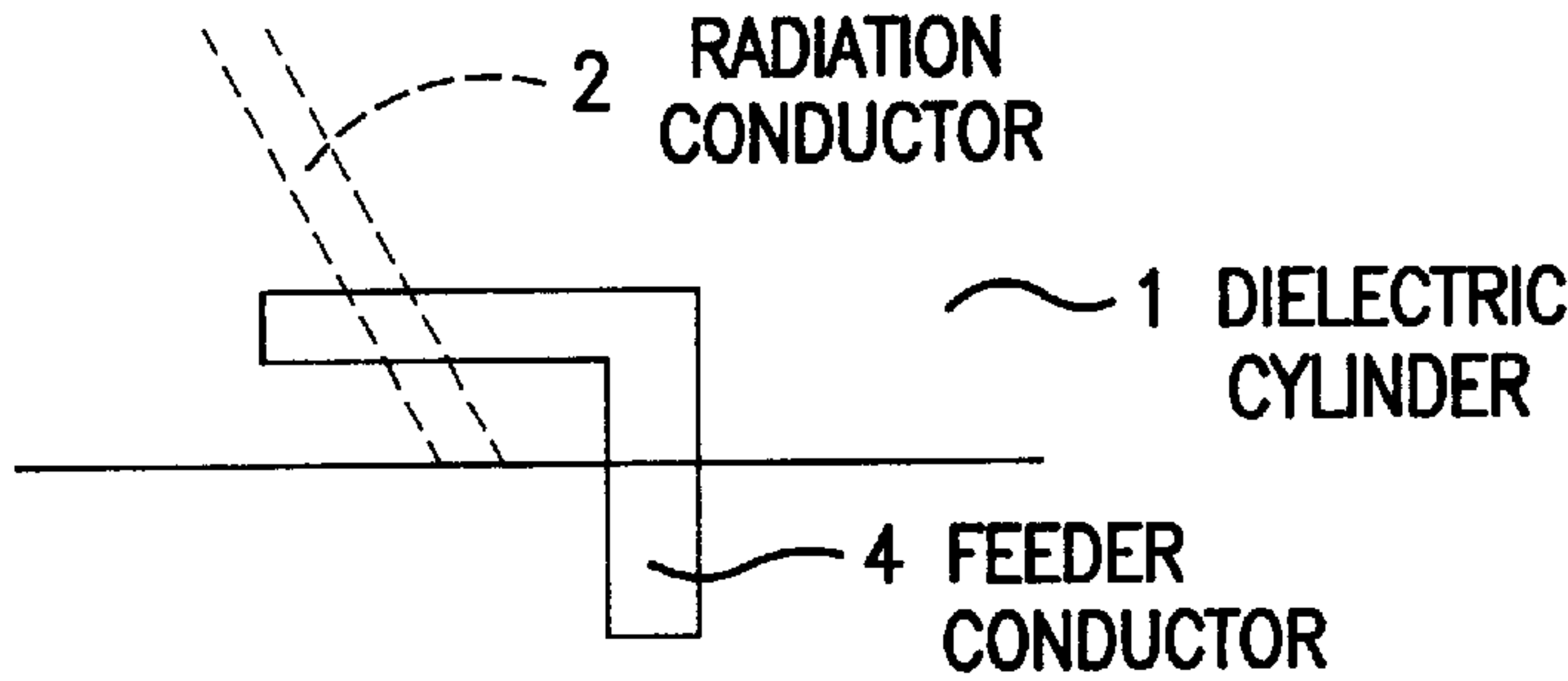
FIG. 4C
