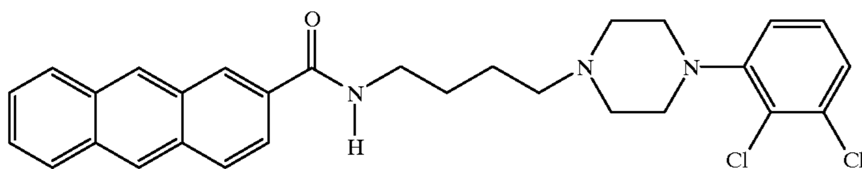
N-{4-[4-(2,3-Dichlorophenyl)-1-piperazinyl]butyl}- 2-anthracenecarboxamide
