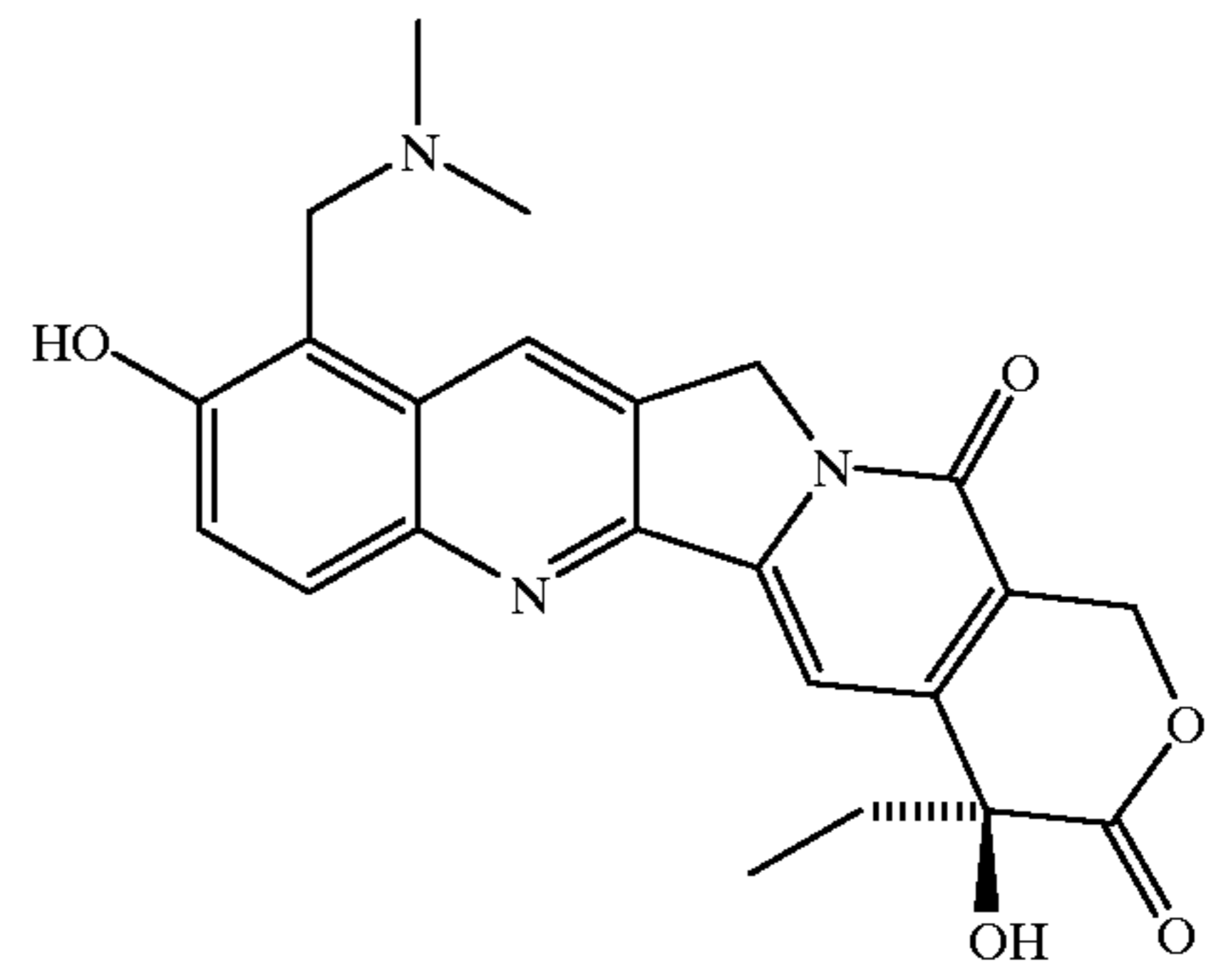
Topotecan
