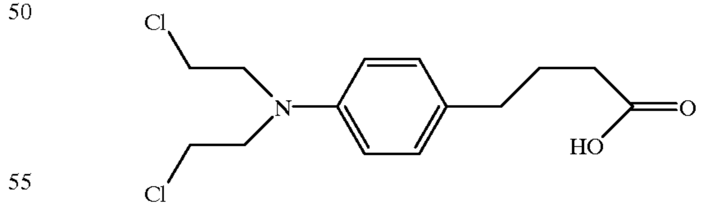
Chlorambucil
