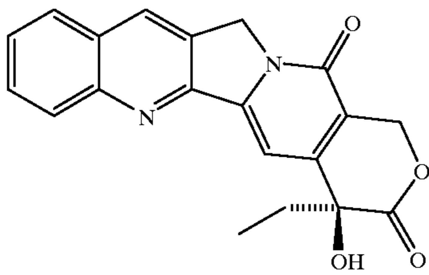
Camptothecin
