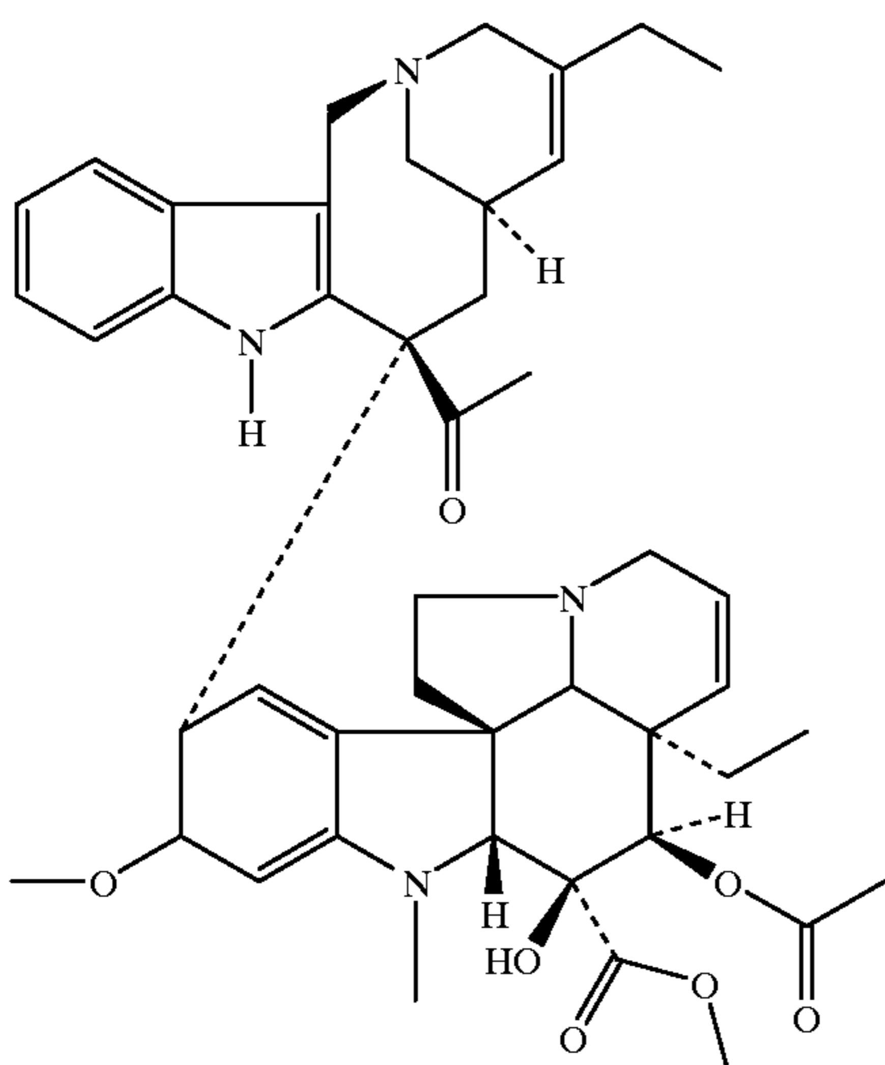
Vinorelbine
