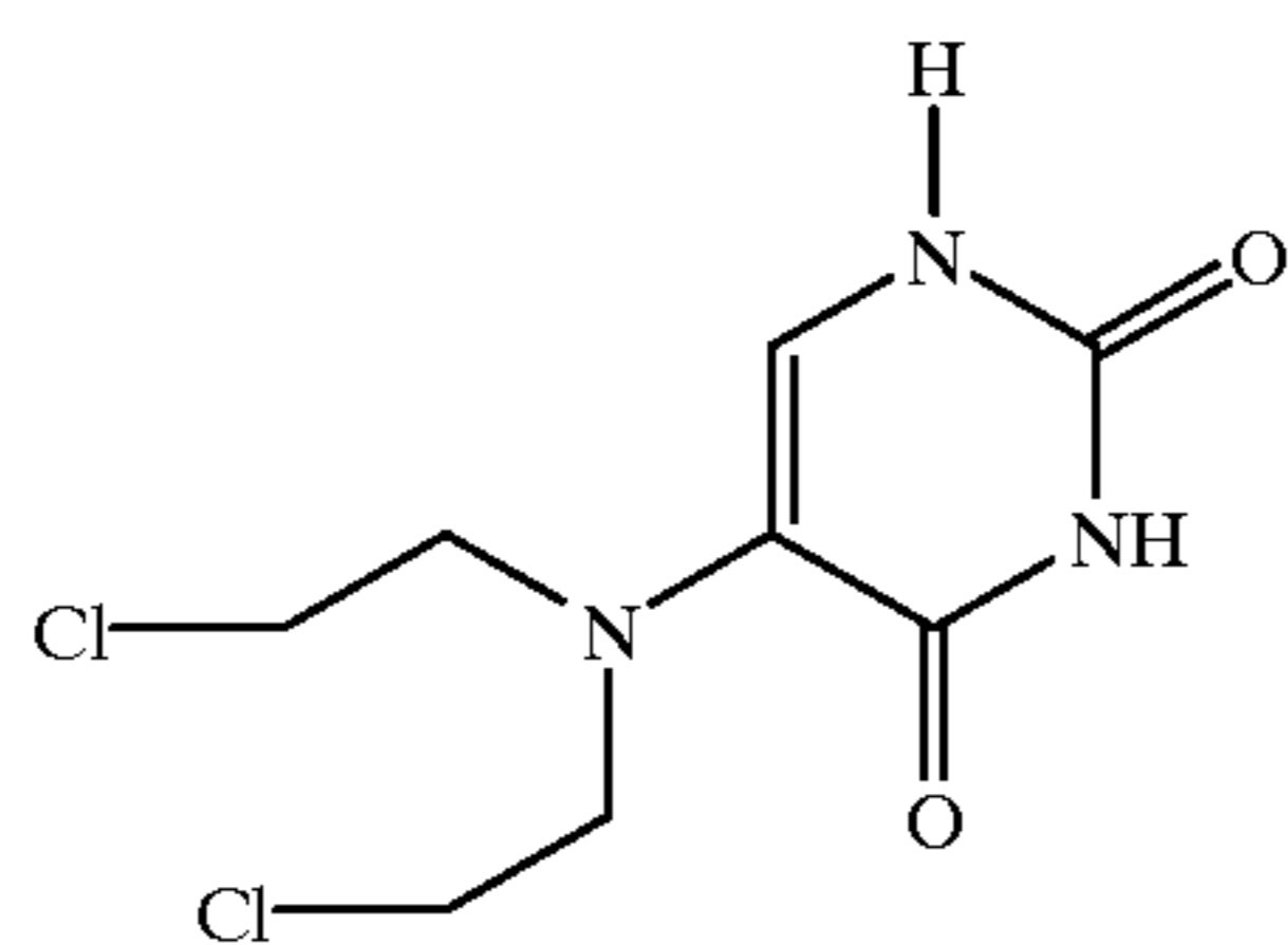
Uracil Mustard
