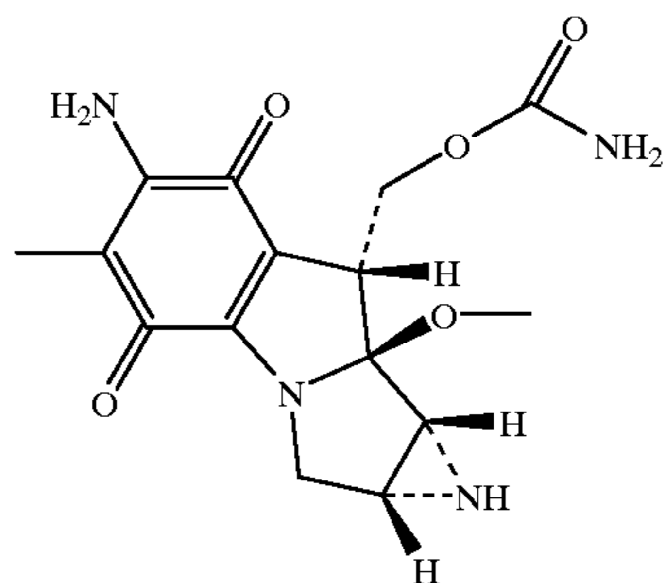
Mitomycin
