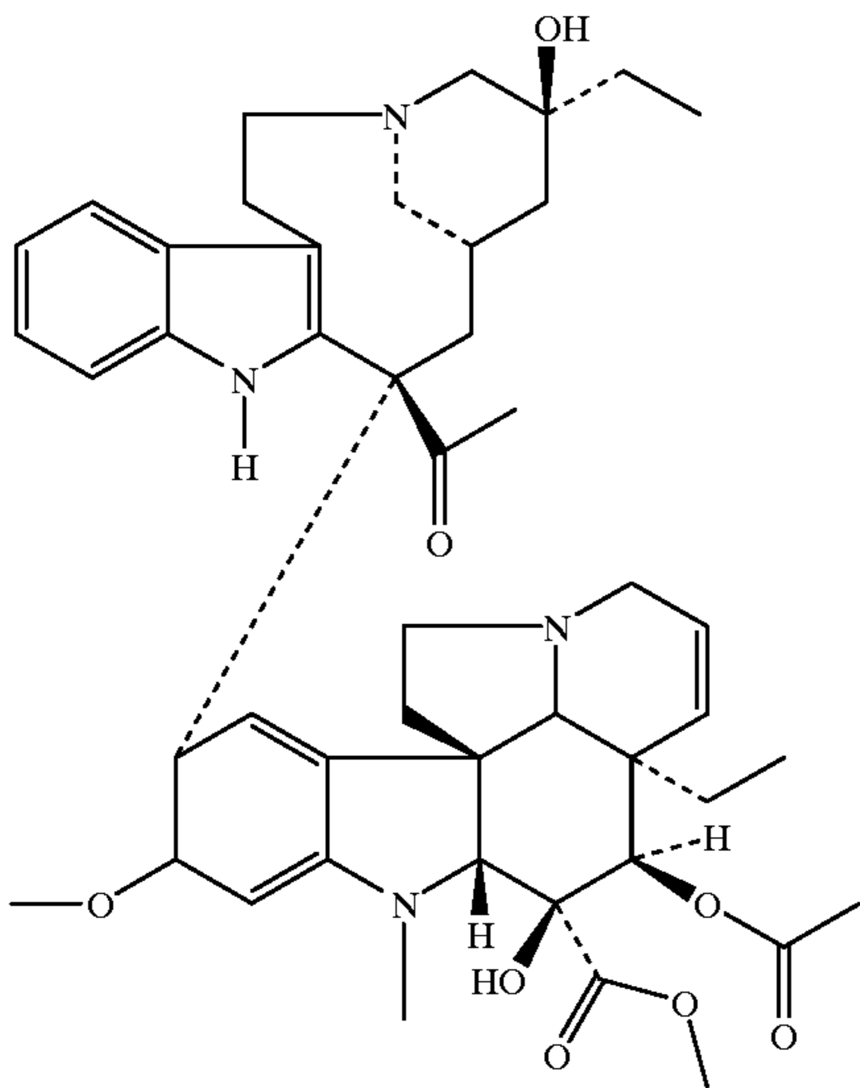
Vinblastine
