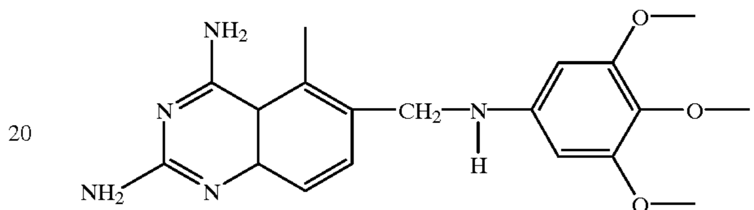
Trimetrexate
