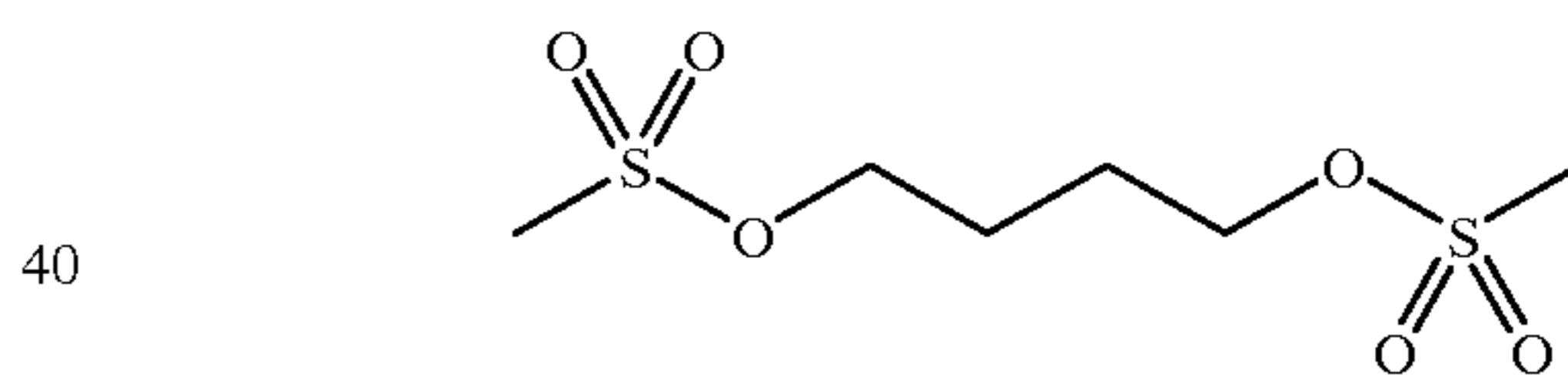
Busulfan
