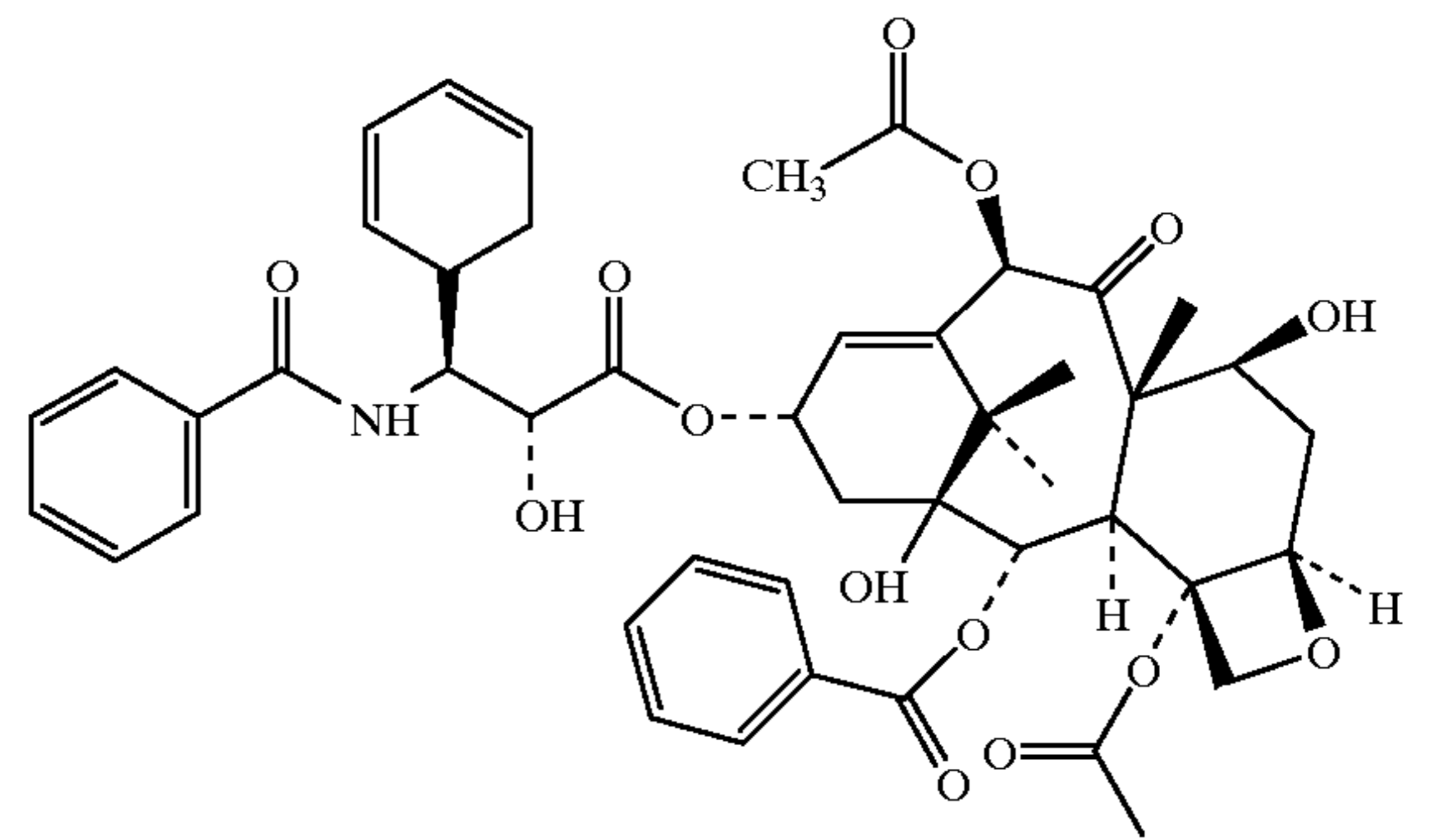
Taxol
