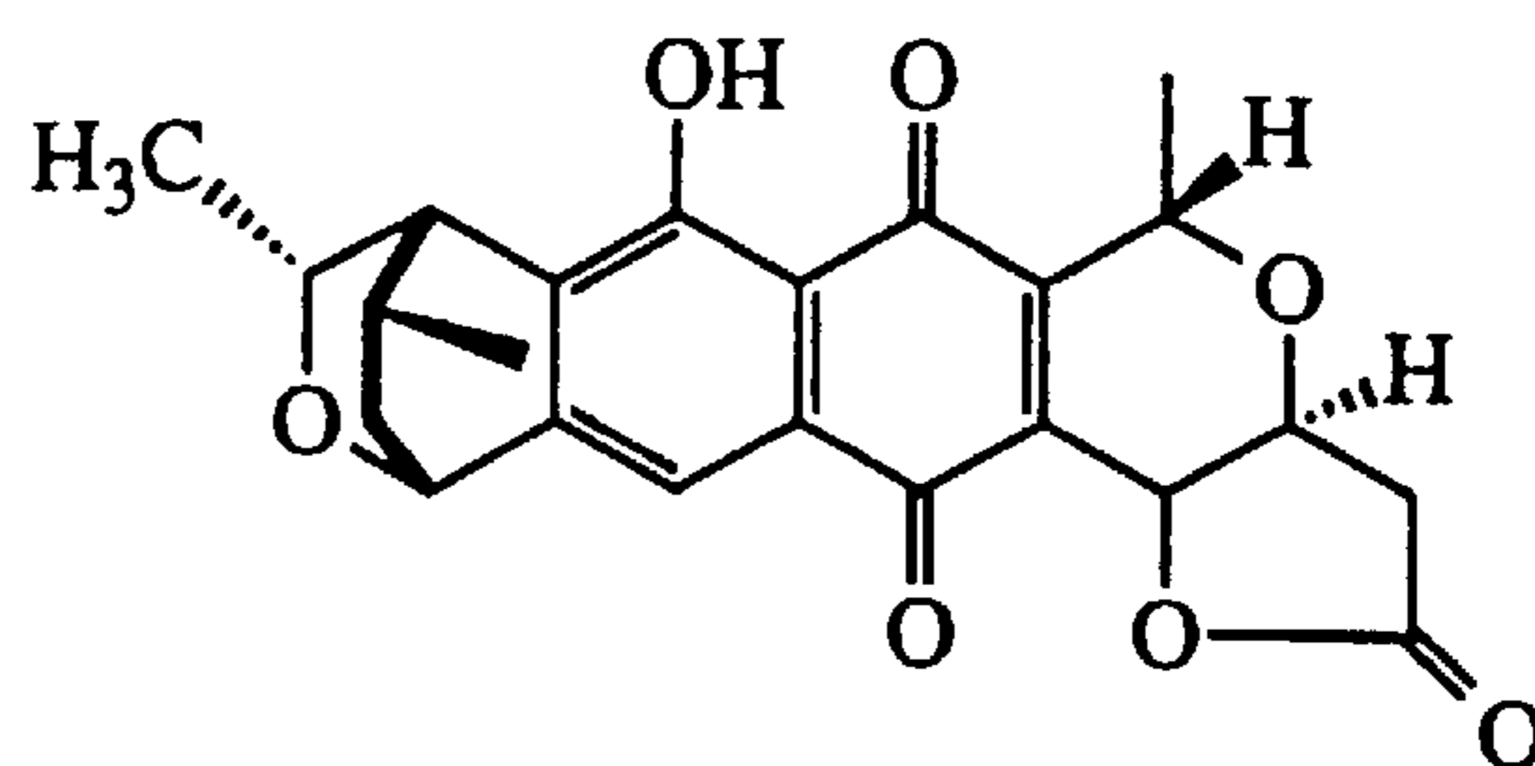
GRANATICIN (4)
