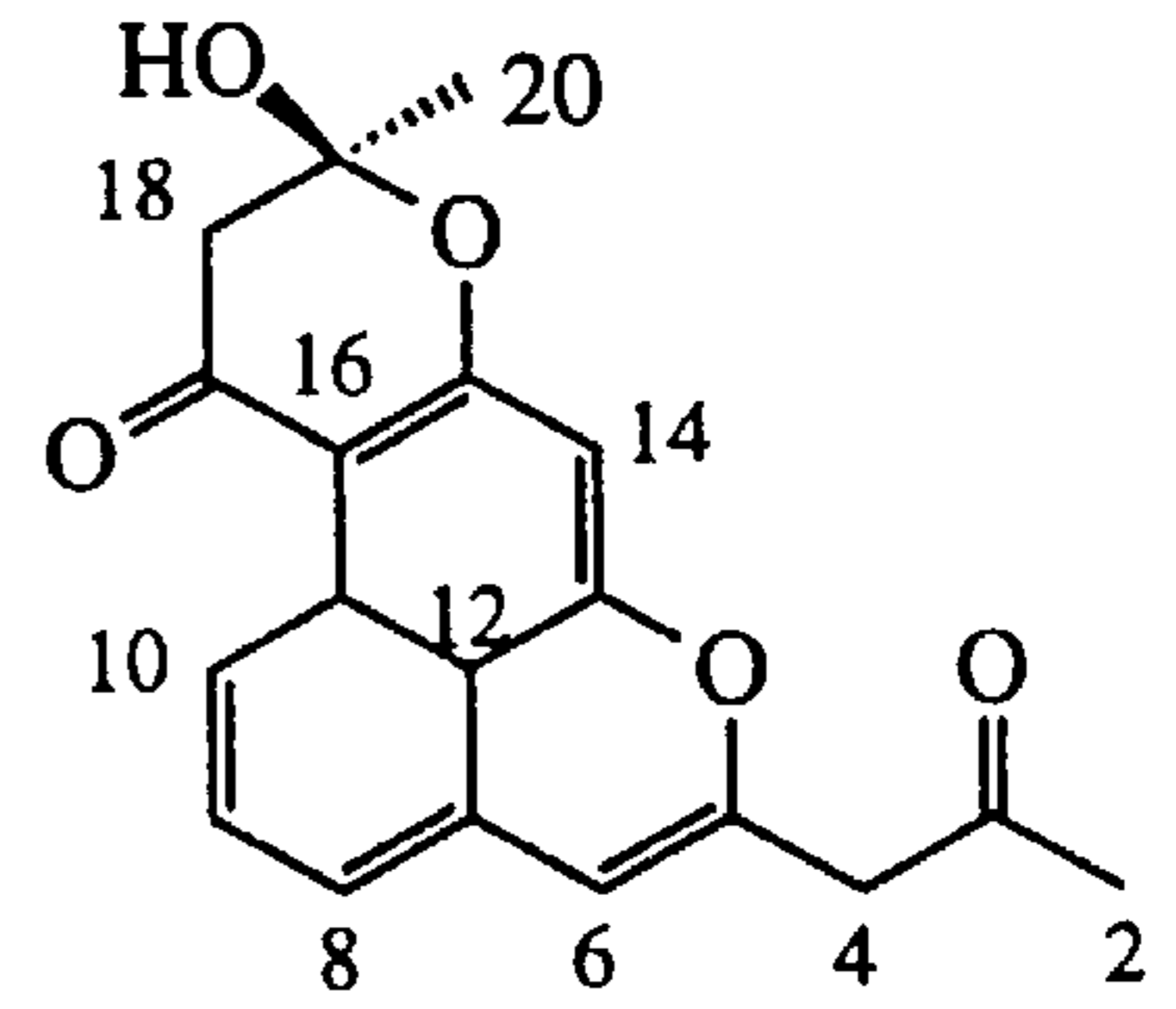
RM 20 (9)
