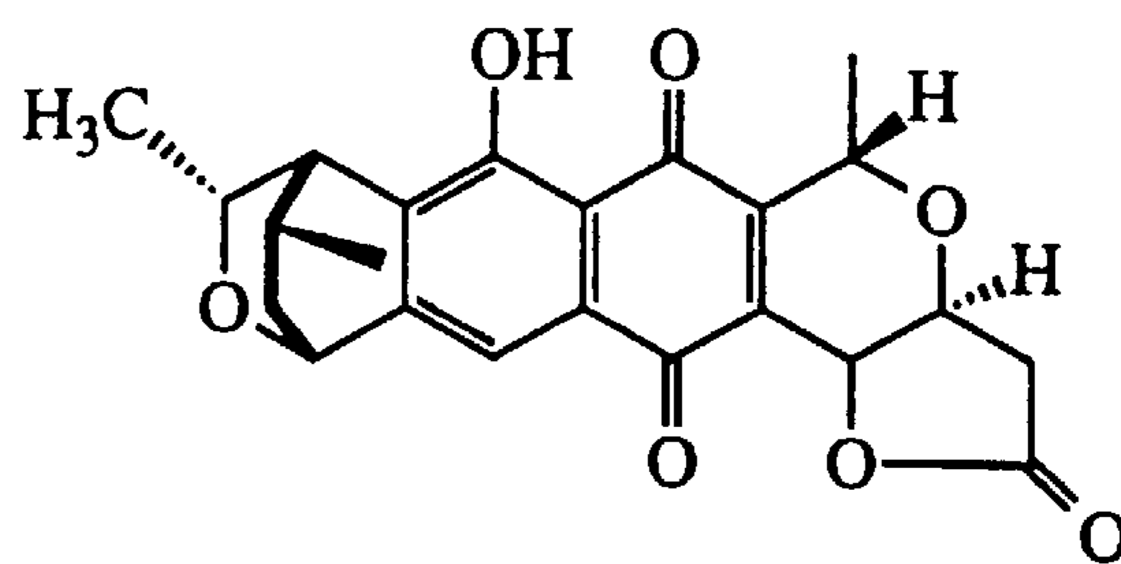
GRANATICIN (4)
