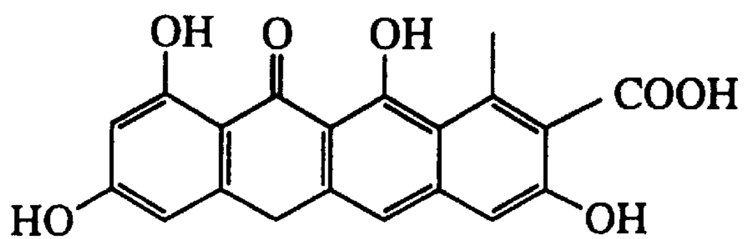
TETRACENOMYCIN F1 (5)
