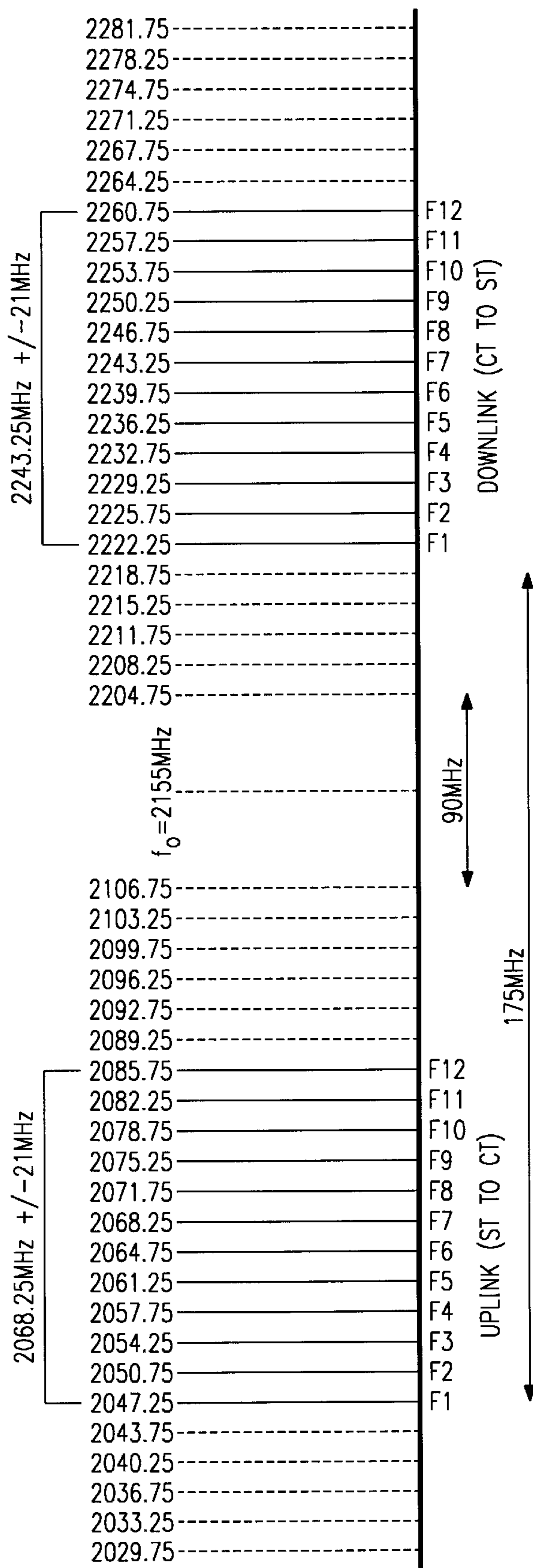
FIG. 4
