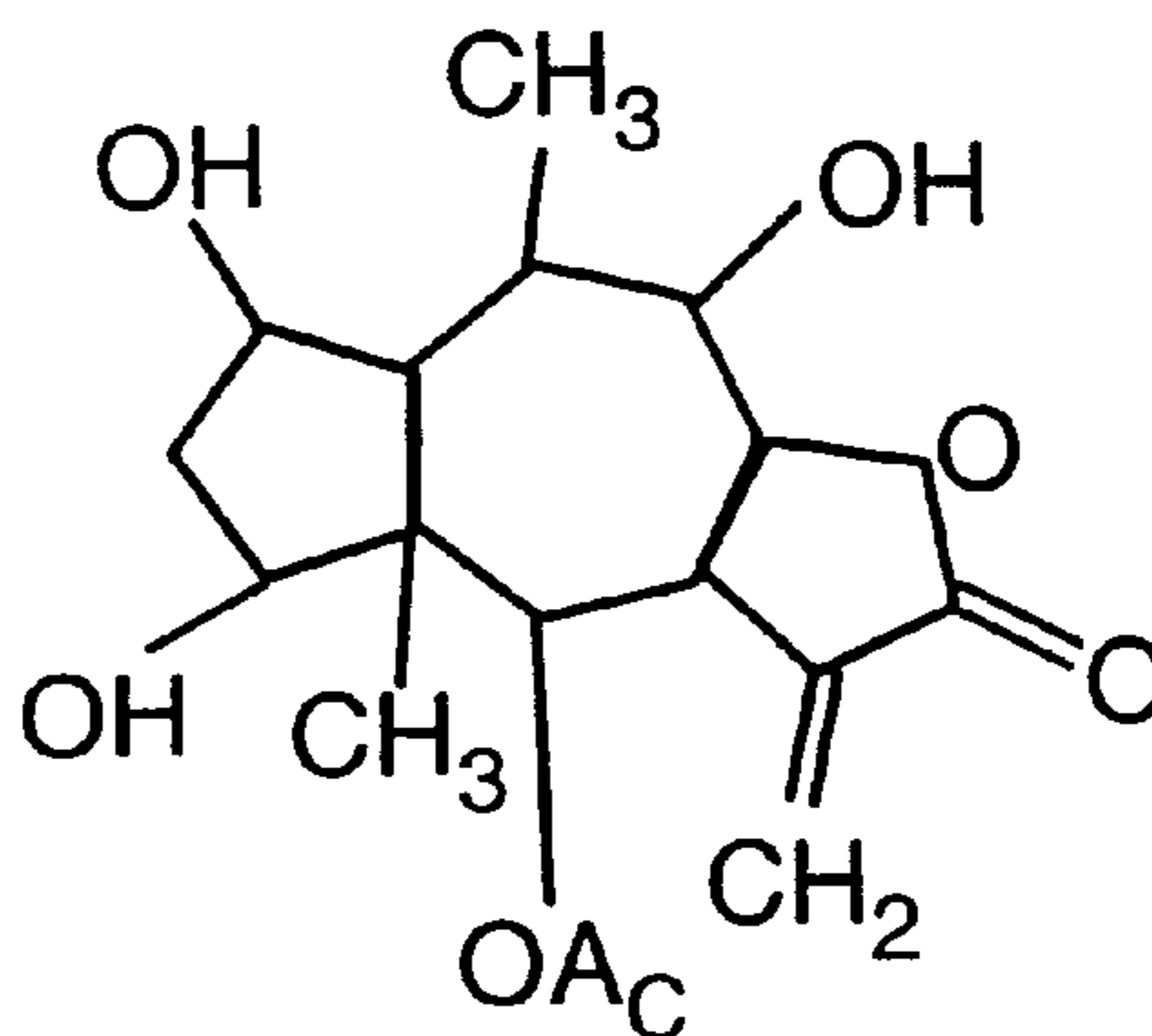
GAIGRANIN 21
