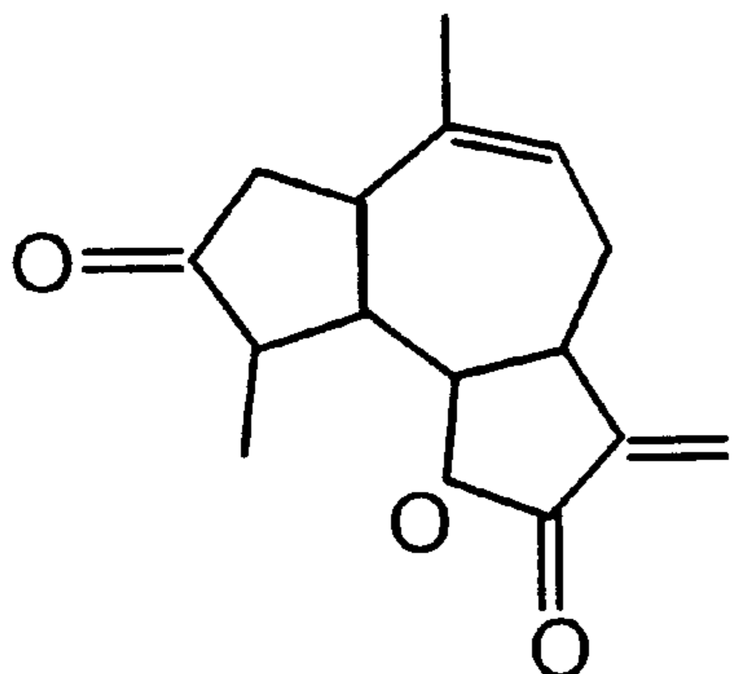
GLABELLIN 17
