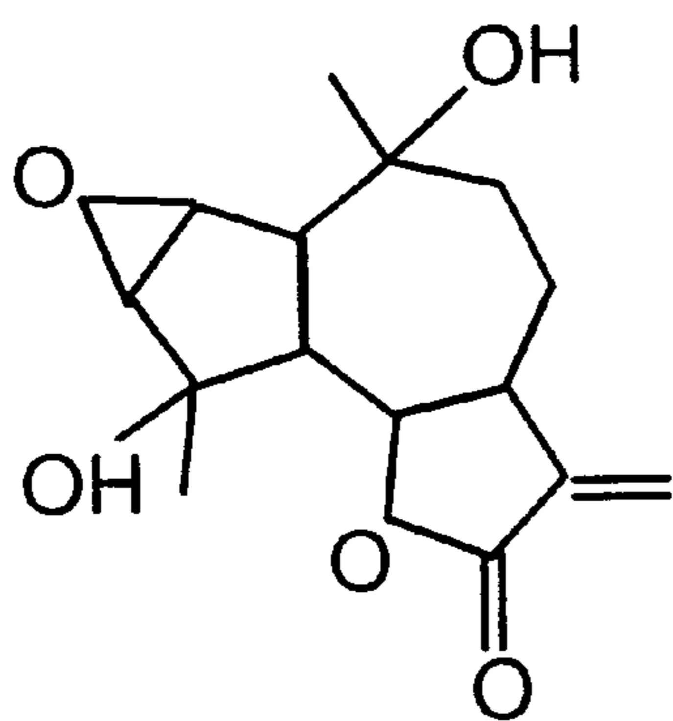
ANOBIN 19
