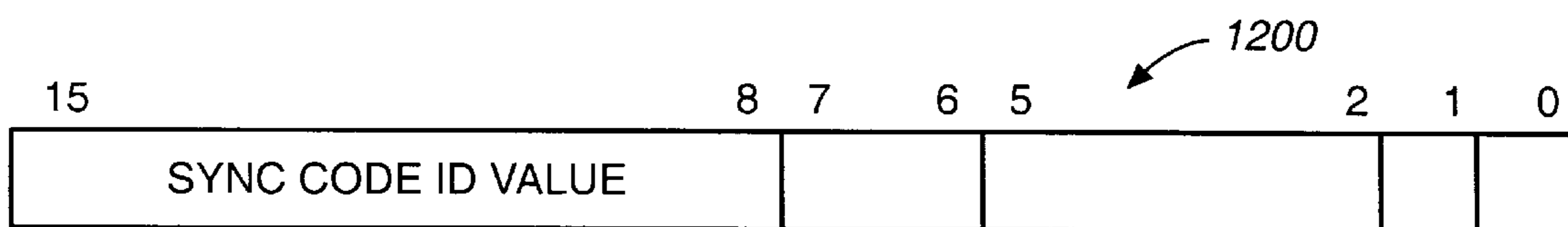
FIG._12 1201 1220 1215 1210 1205
