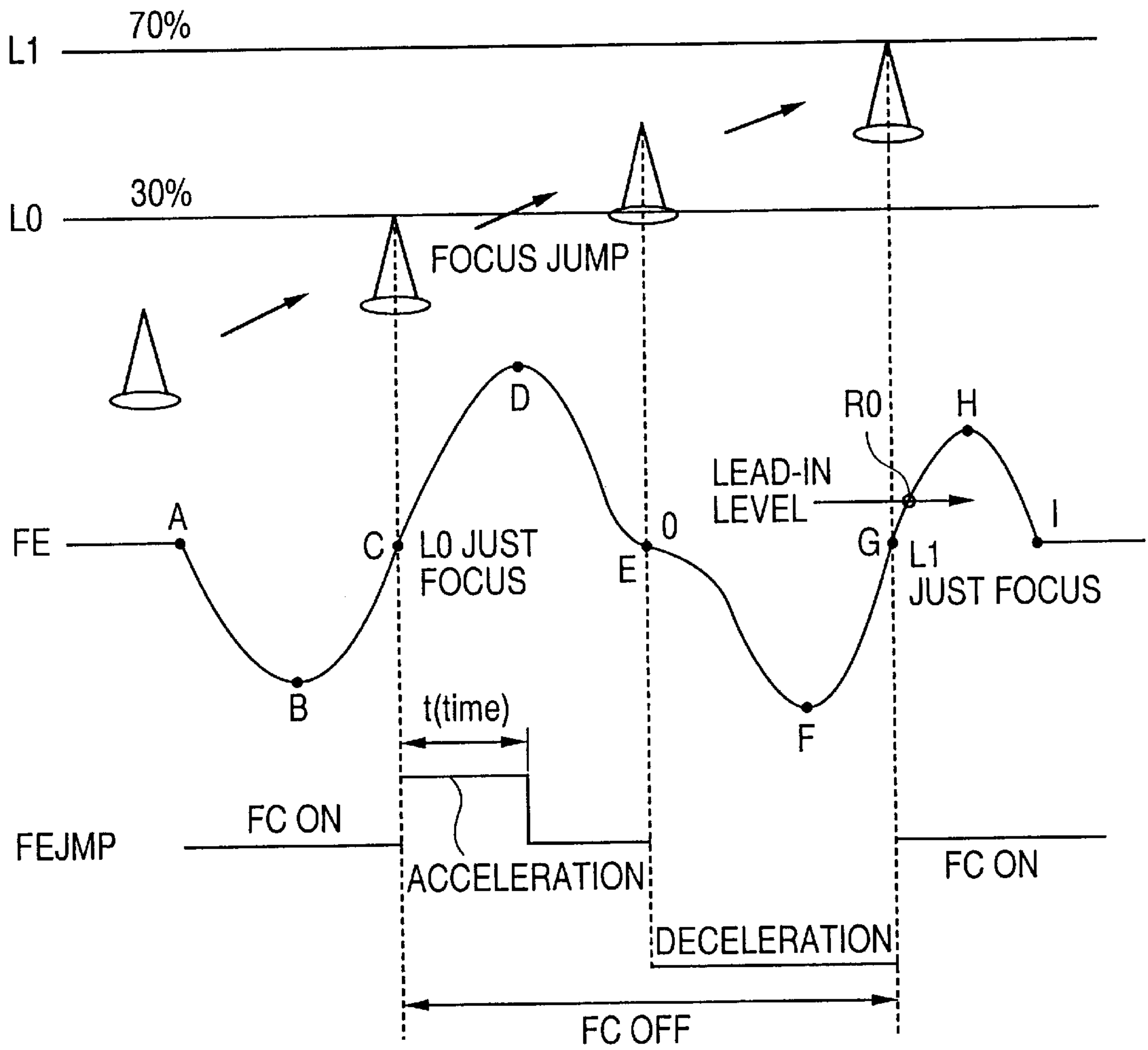
FIG. 18
