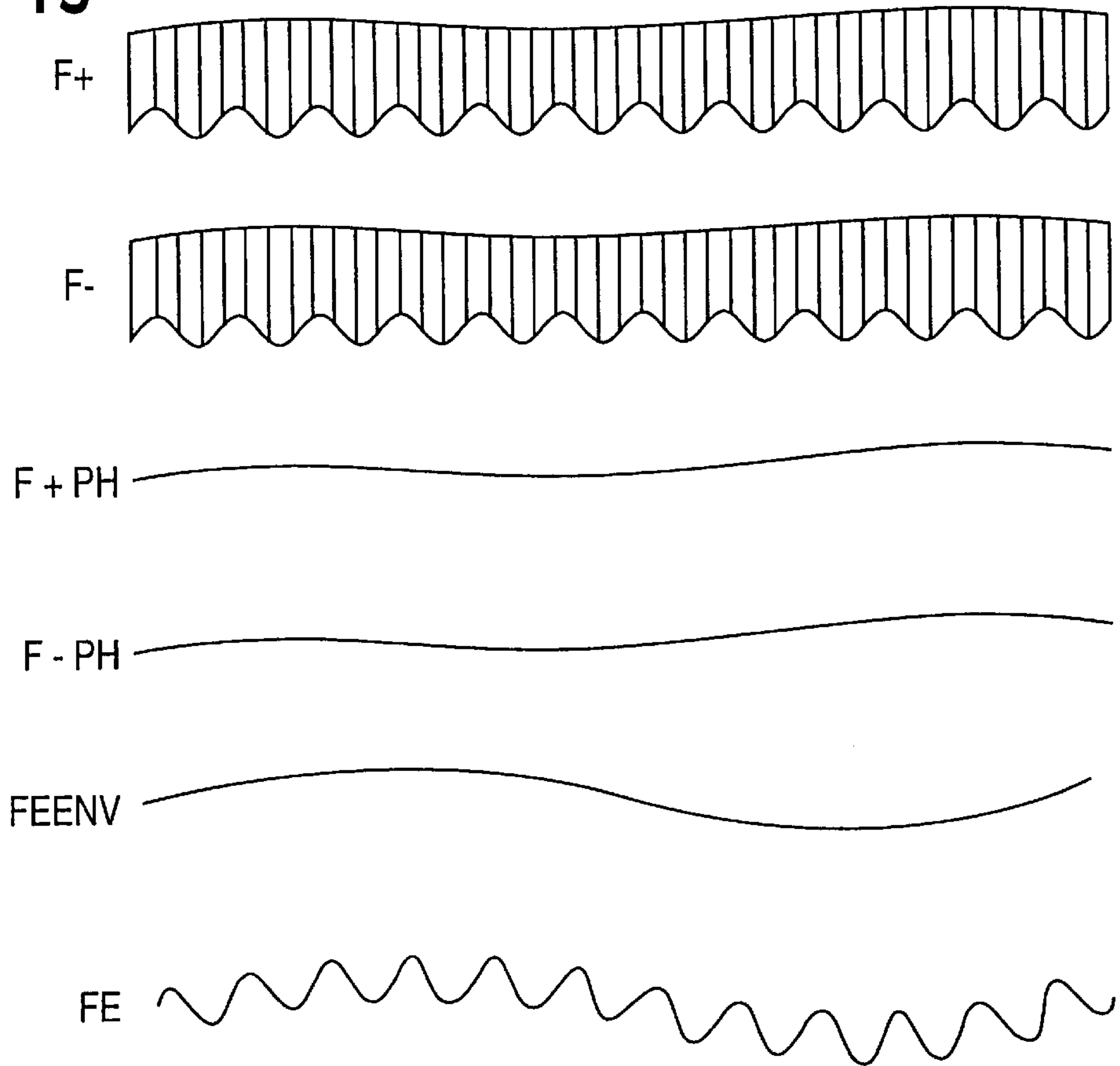
FIG. 15
