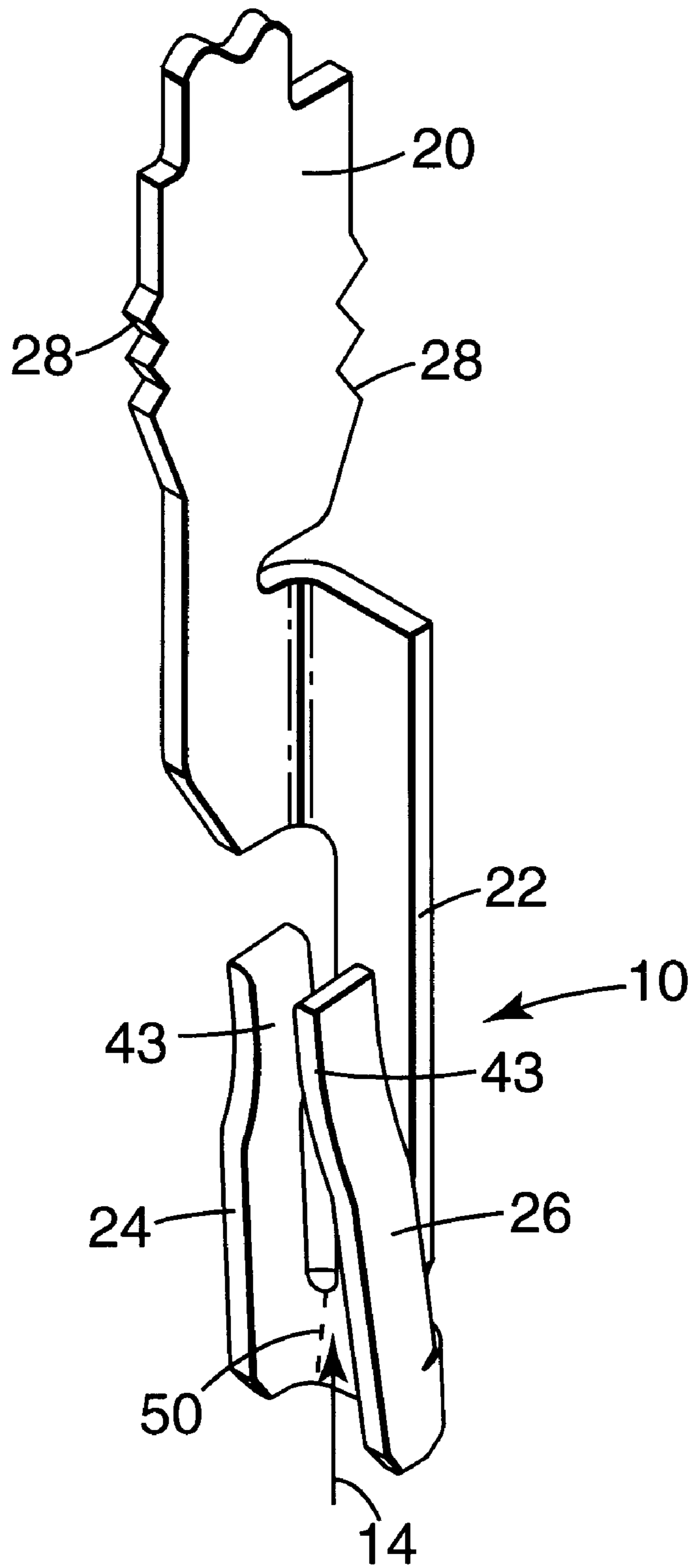
Fig. 2
