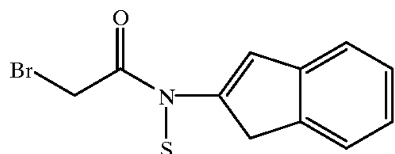
Bromo-N-(2'-benzothiazolyl)acetamide
