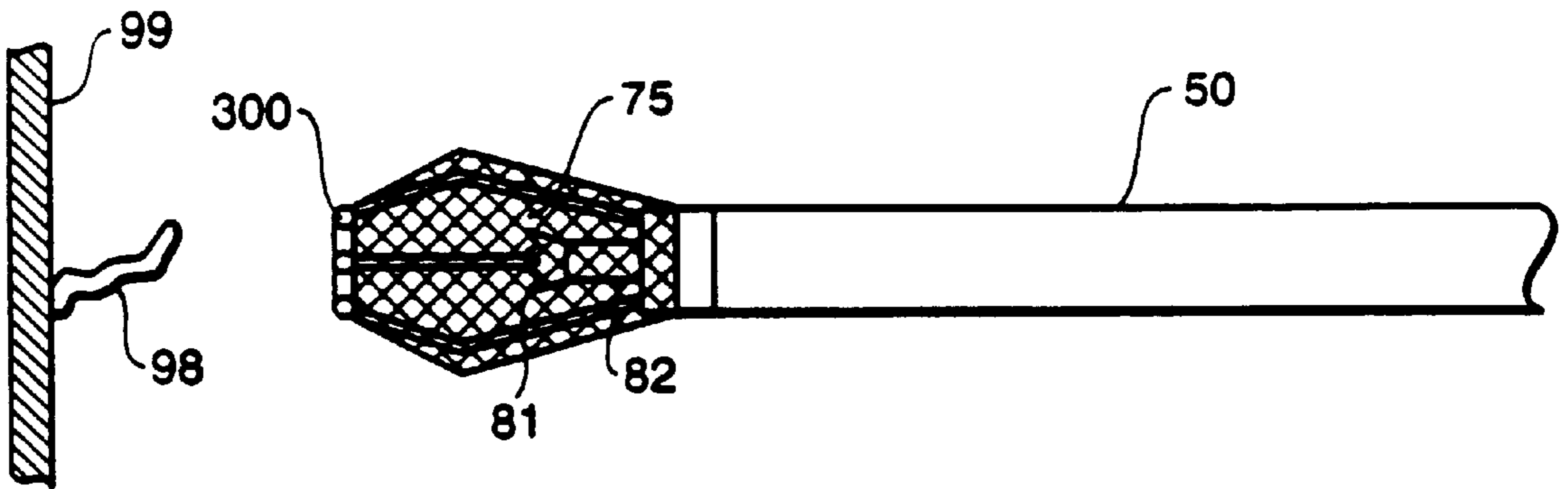
FIG. 22
