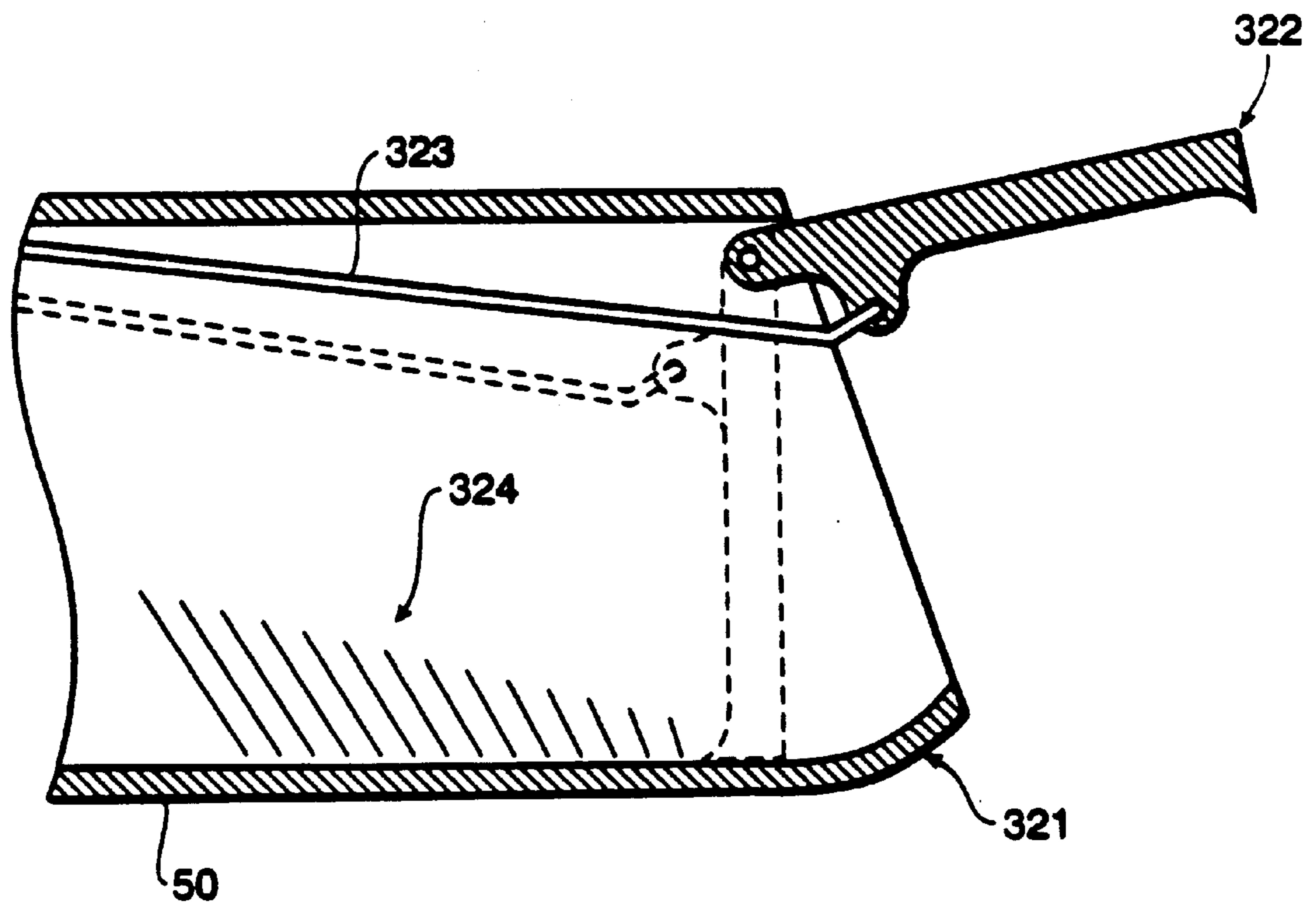
FIG. 23A
