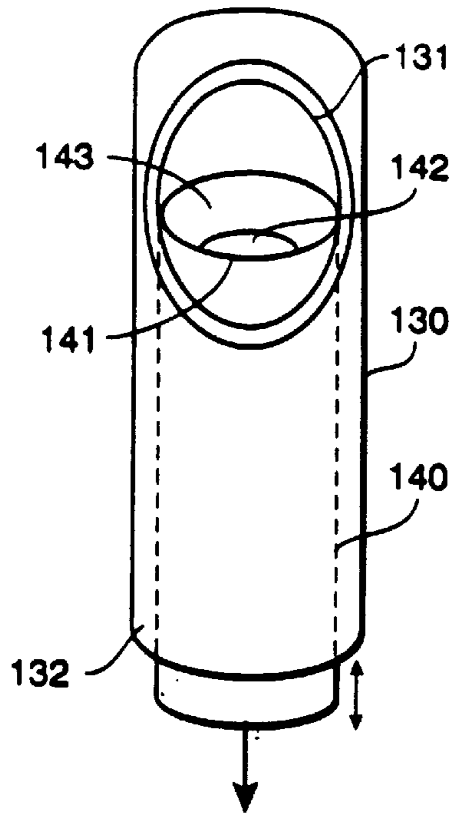
FIG. 4
