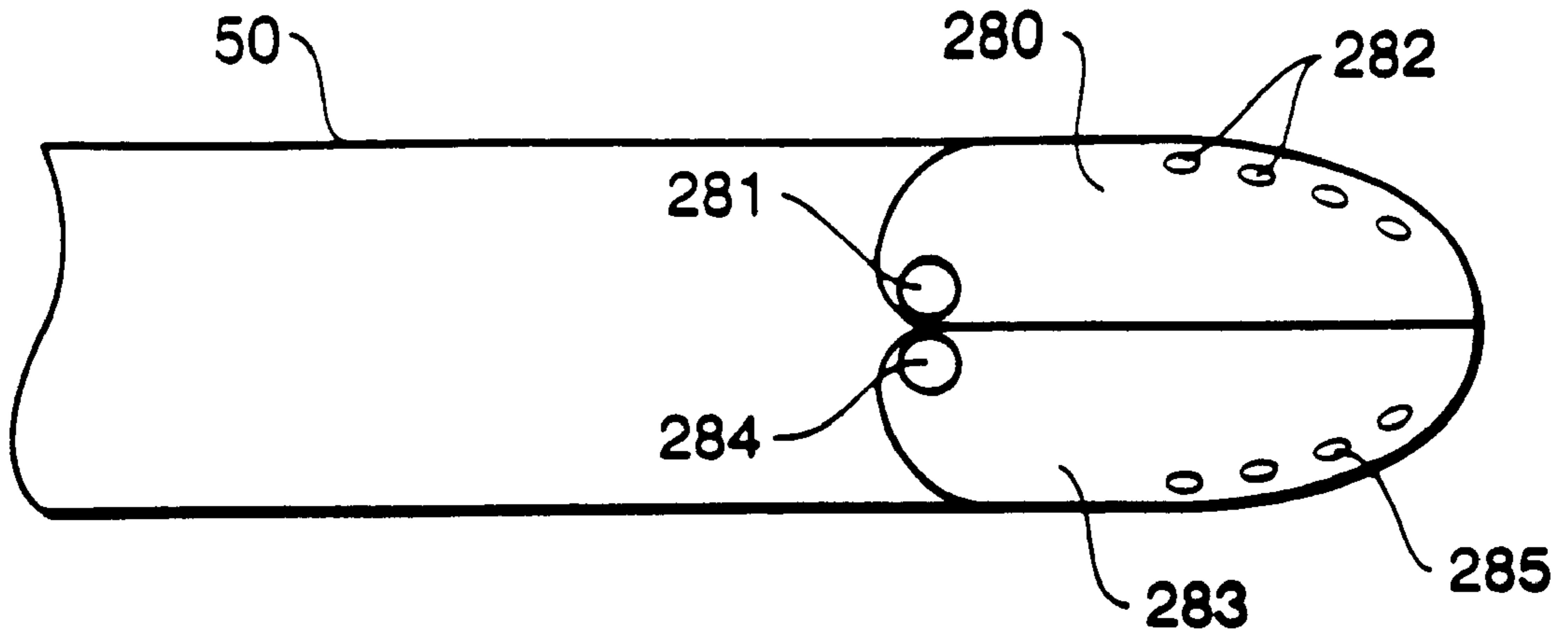
FIG. 15A
