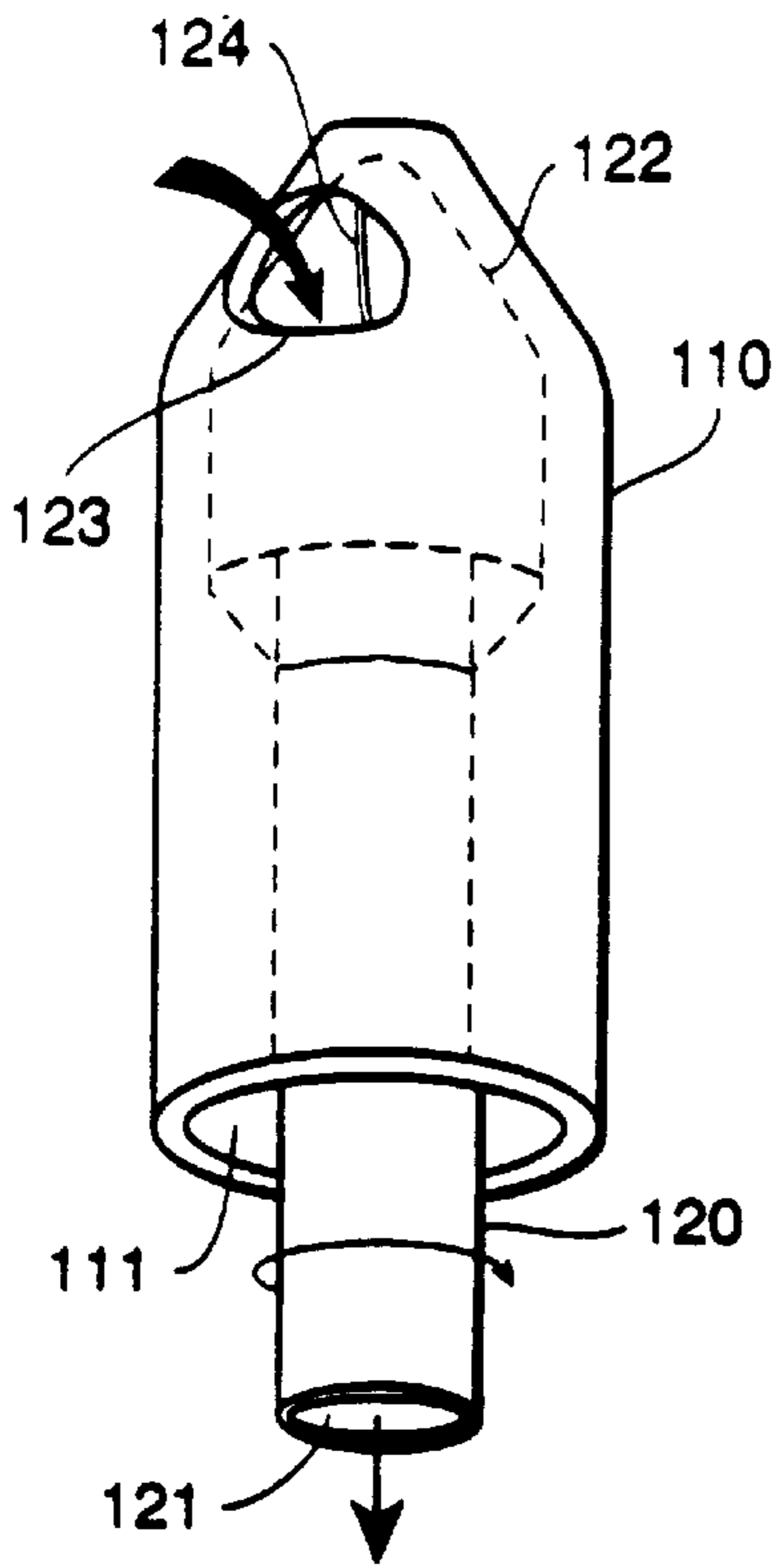
FIG. 3
