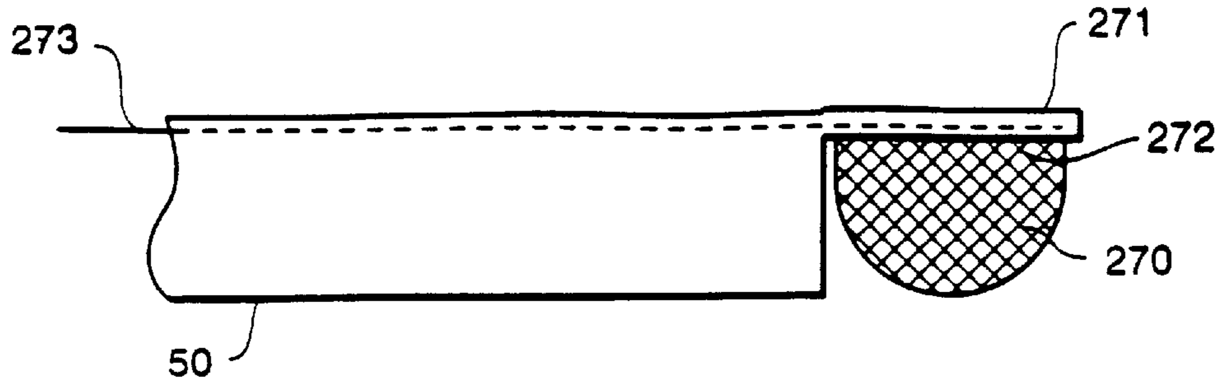
FIG. 14A
