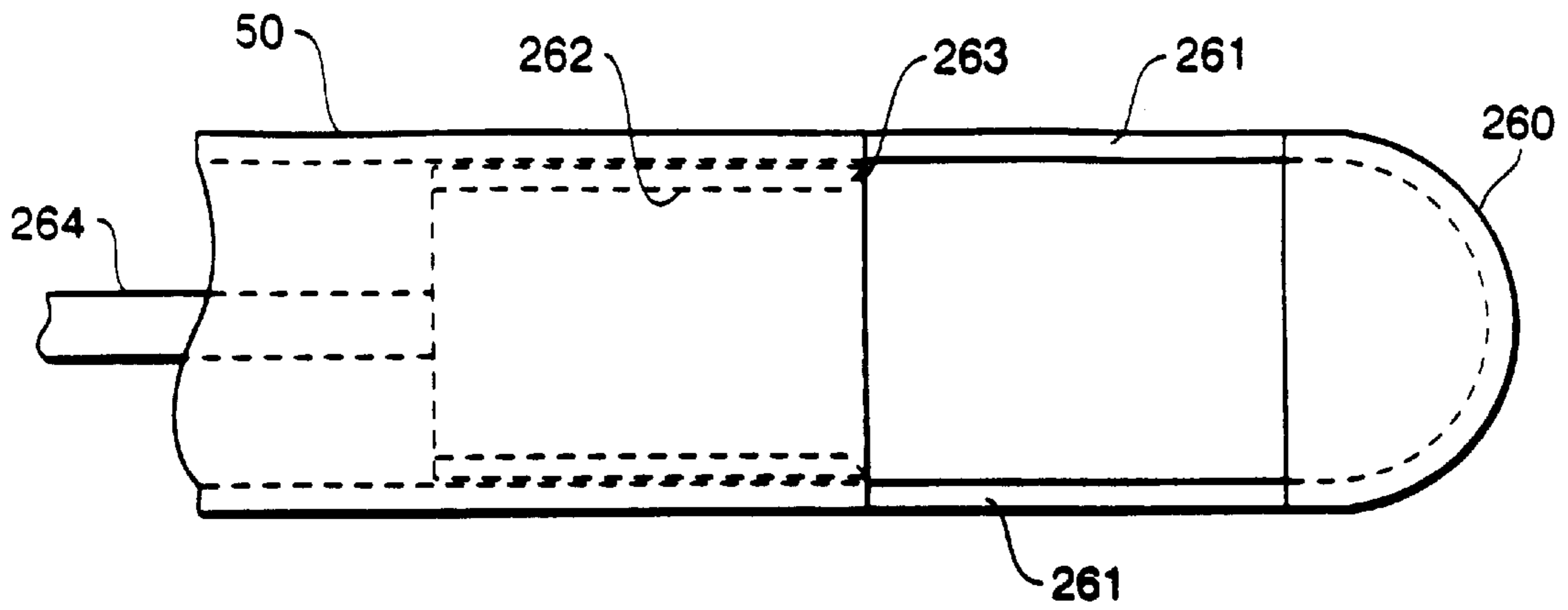
FIG. 13A
