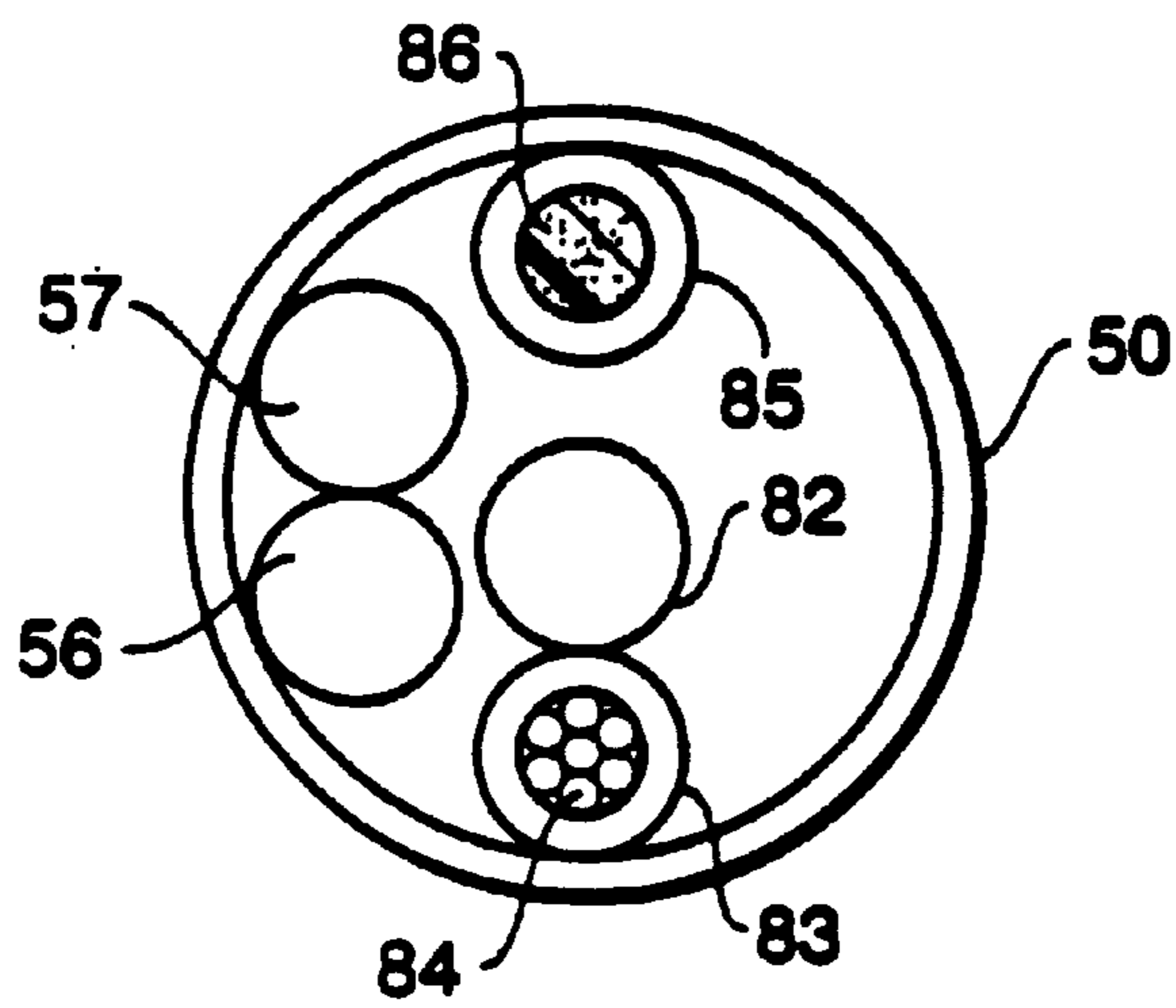
FIG. 2A
