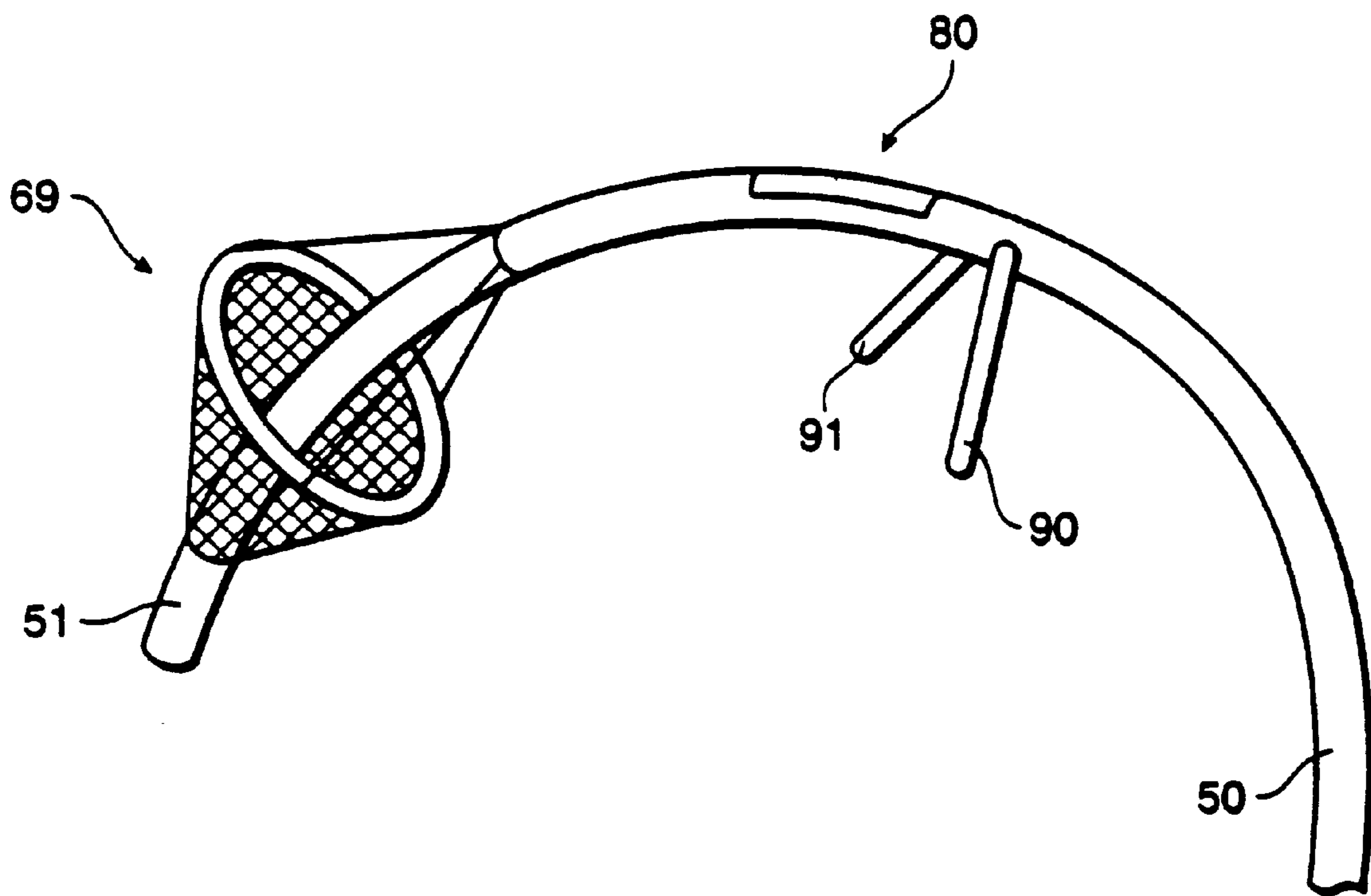
FIG. 17
