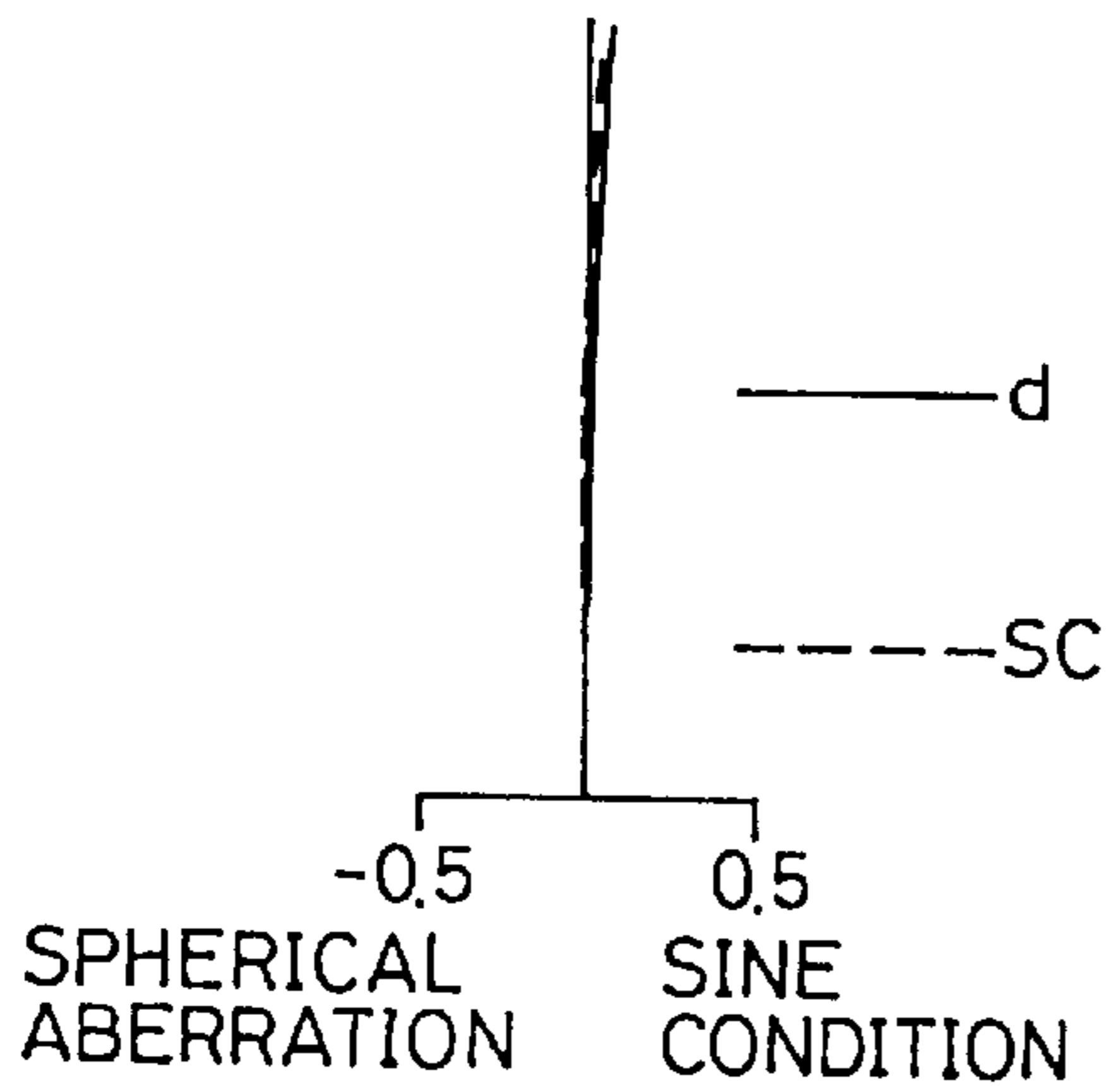
FIG. 16D FNO= 6.55
