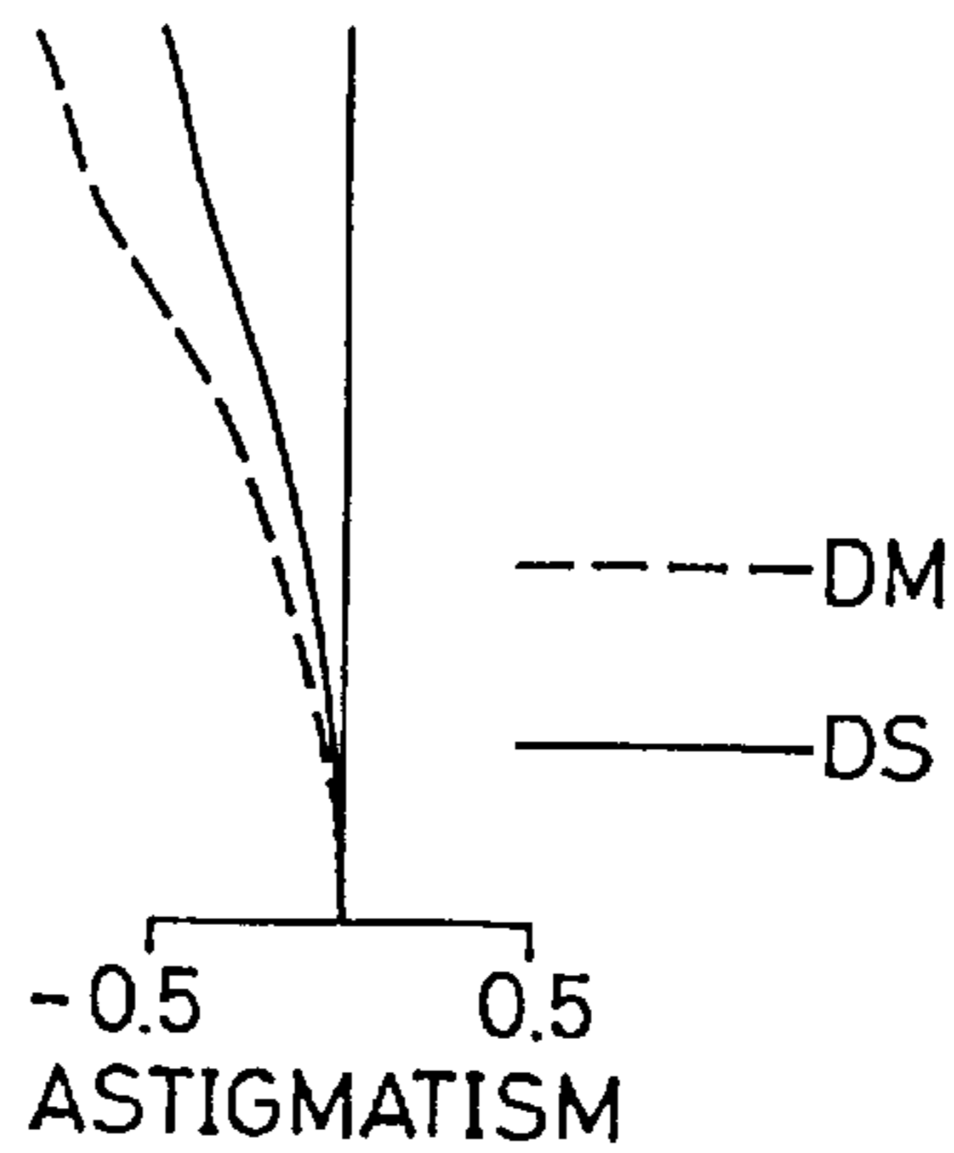
FIG. 16H Y'=21.6
