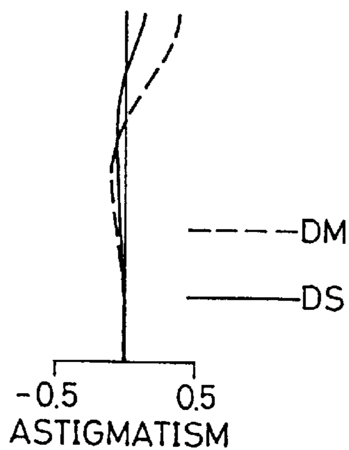
FIG. 14E Y'=21.6
