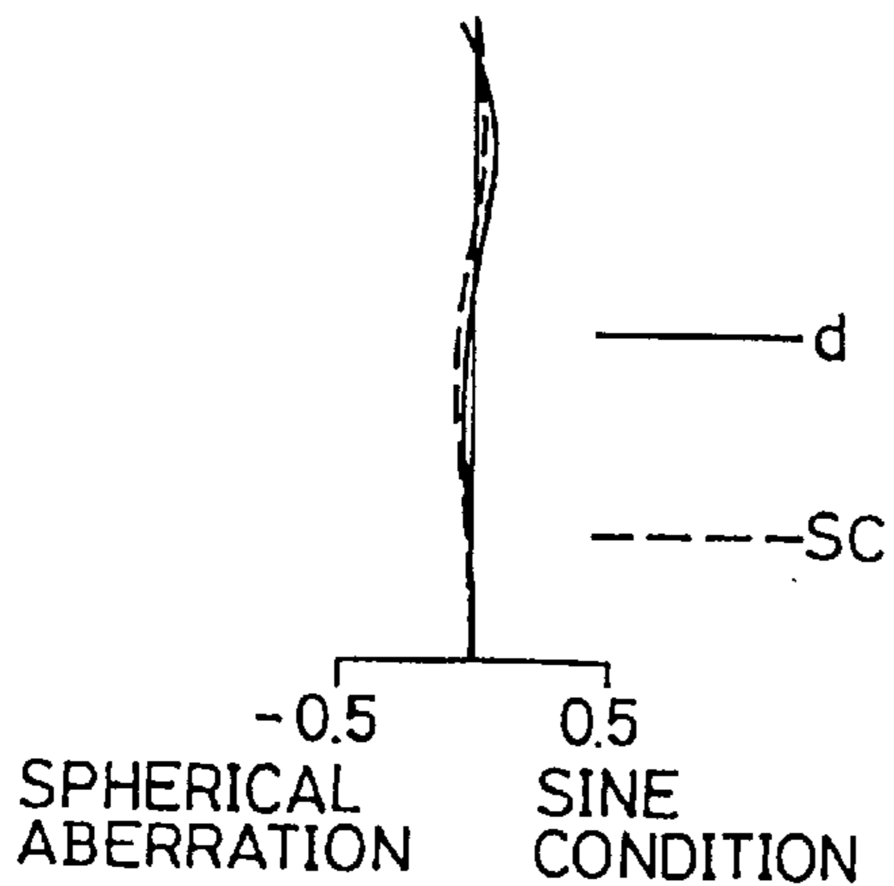
FIG. 16G FNO= 9.39
