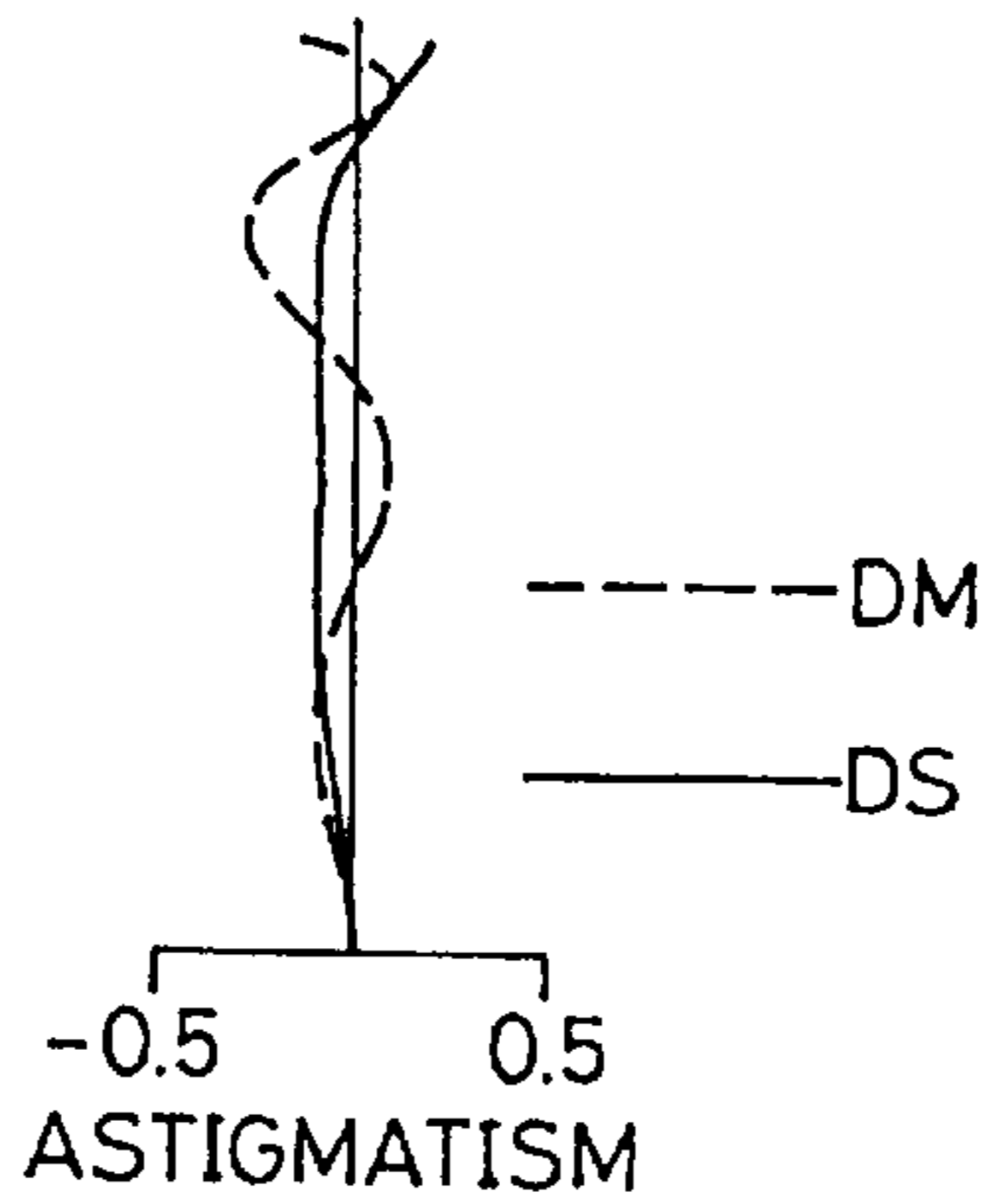
FIG. 16B Y'=21.6
