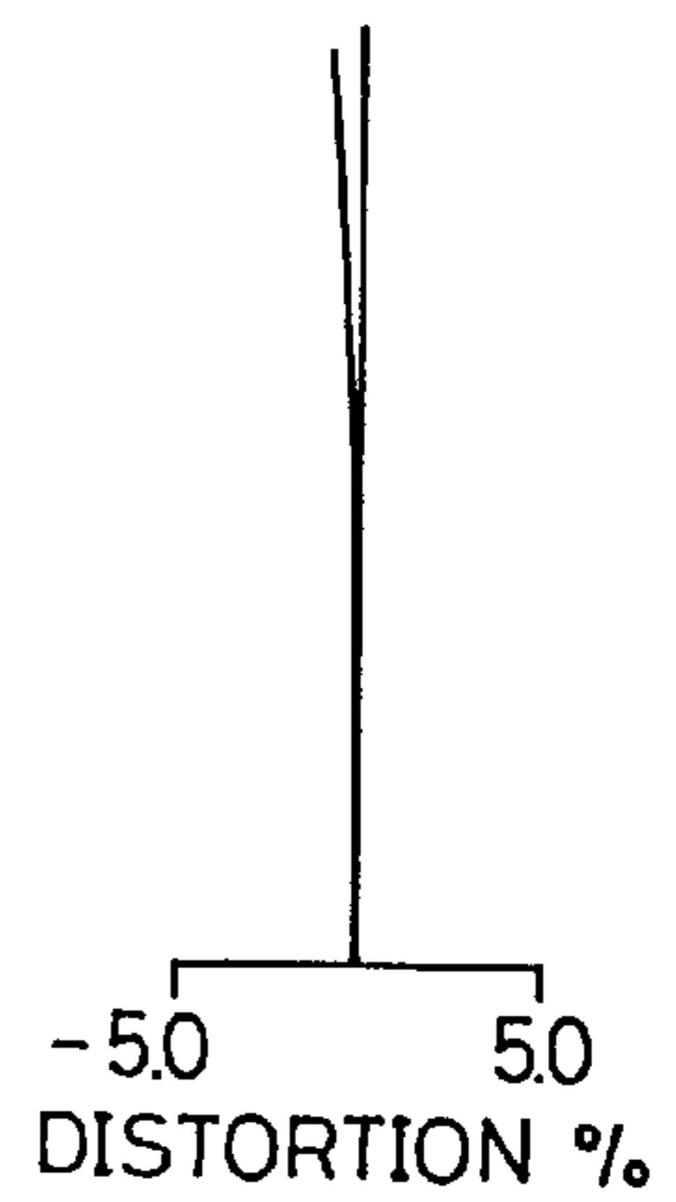
FIG. 14I Y'=21.6
