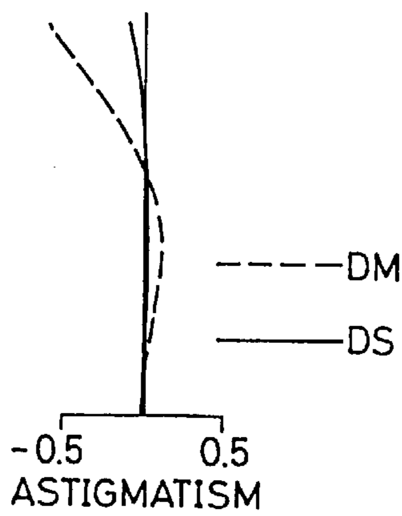
FIG. 14H Y'=21.6
