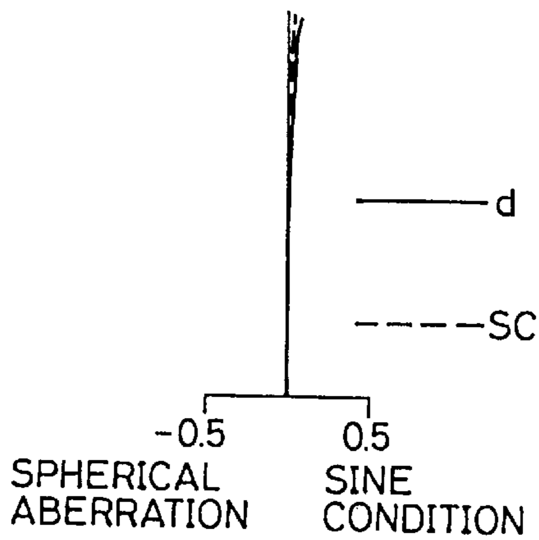
FIG. 16A FNO= 5.05
