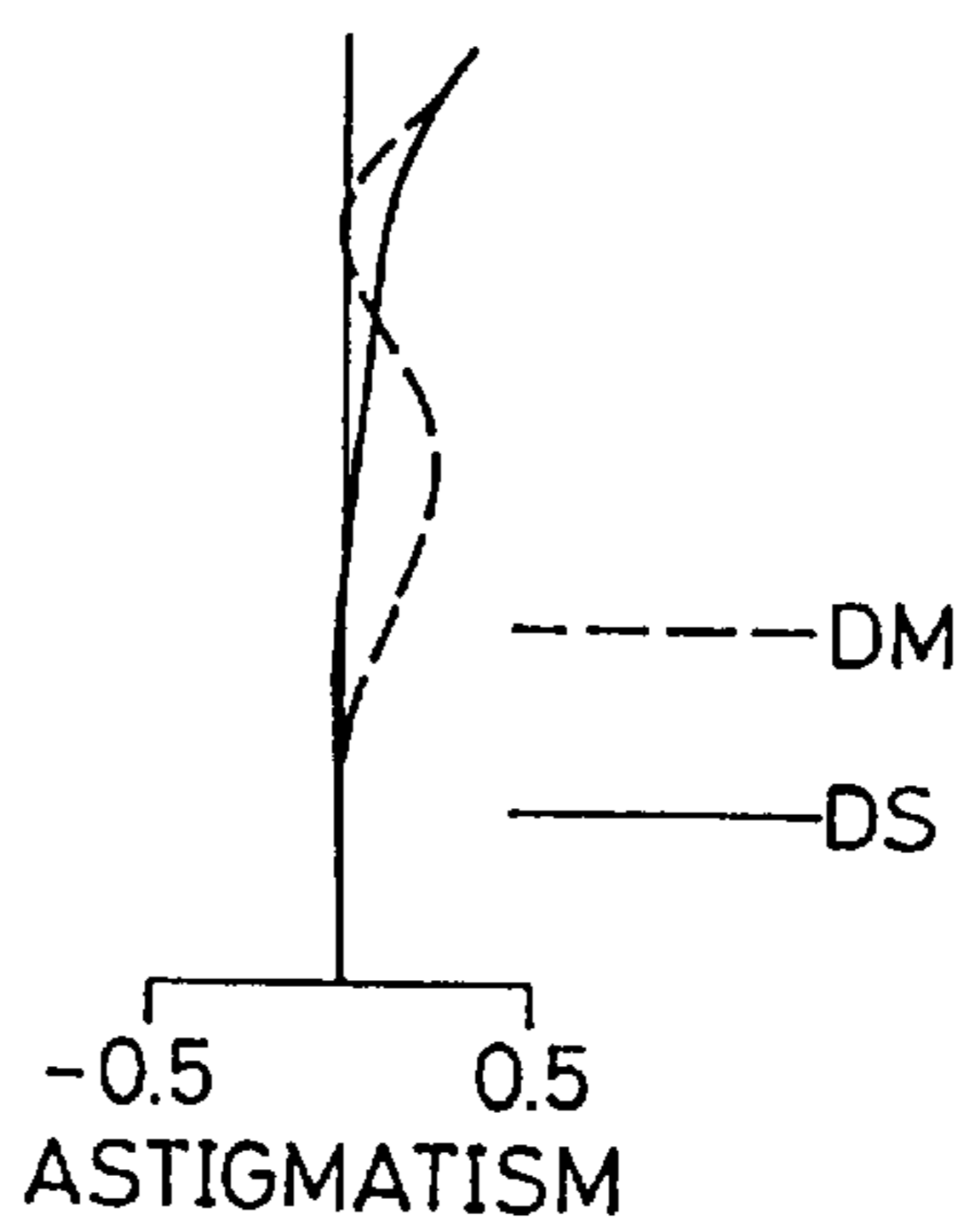
FIG. 14B Y'=21.6
