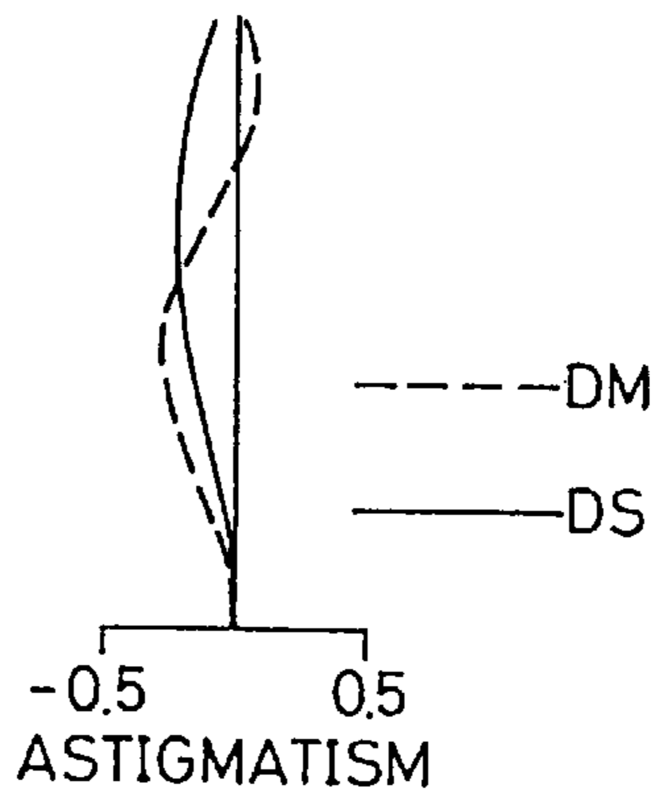
FIG. 16E Y'=21.6
