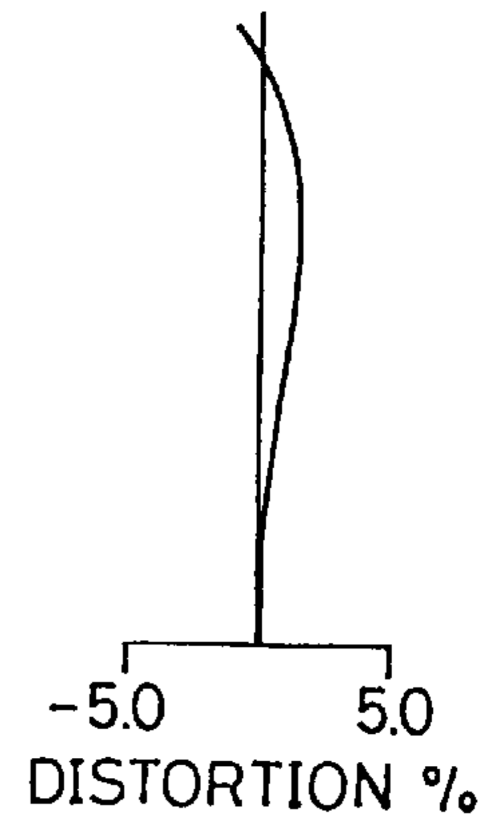
FIG. 16C Y'=21.6
