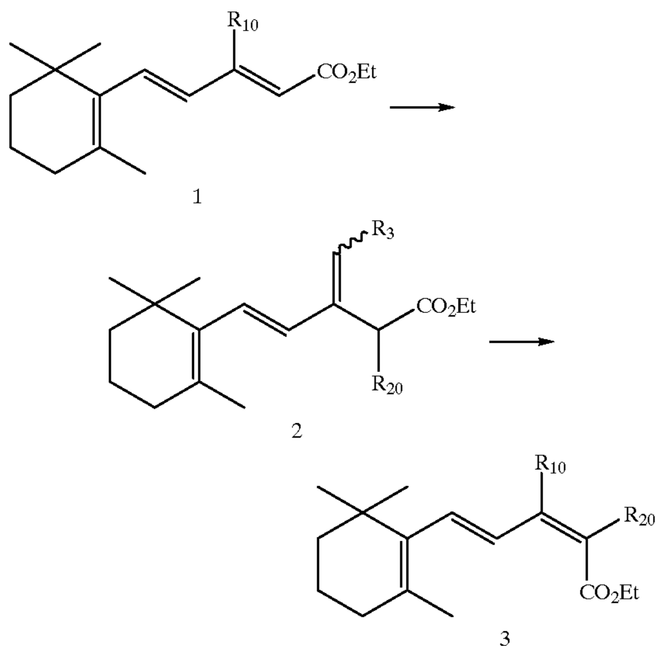
SCHEME 1a
