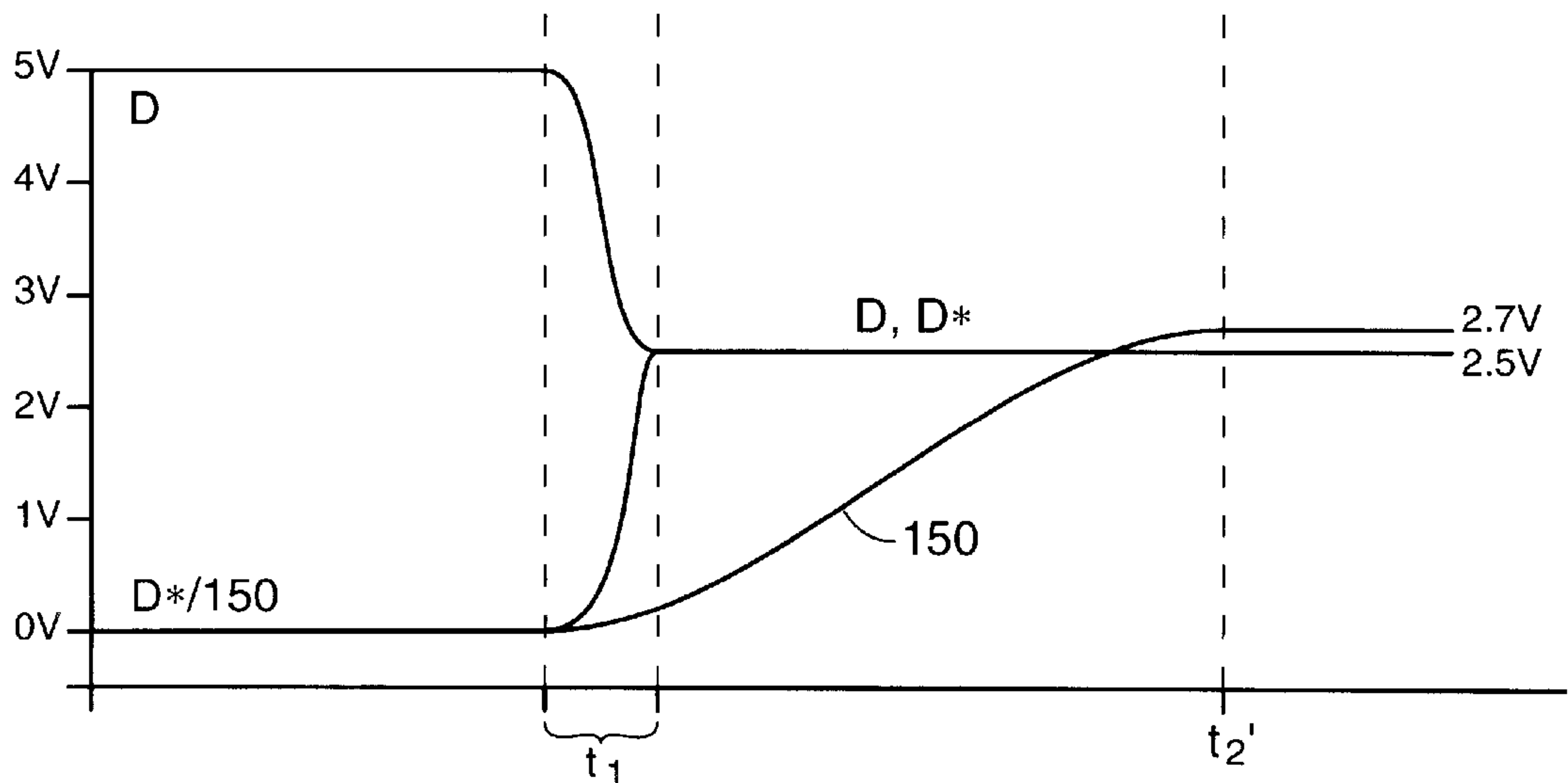
FIG. 9D
