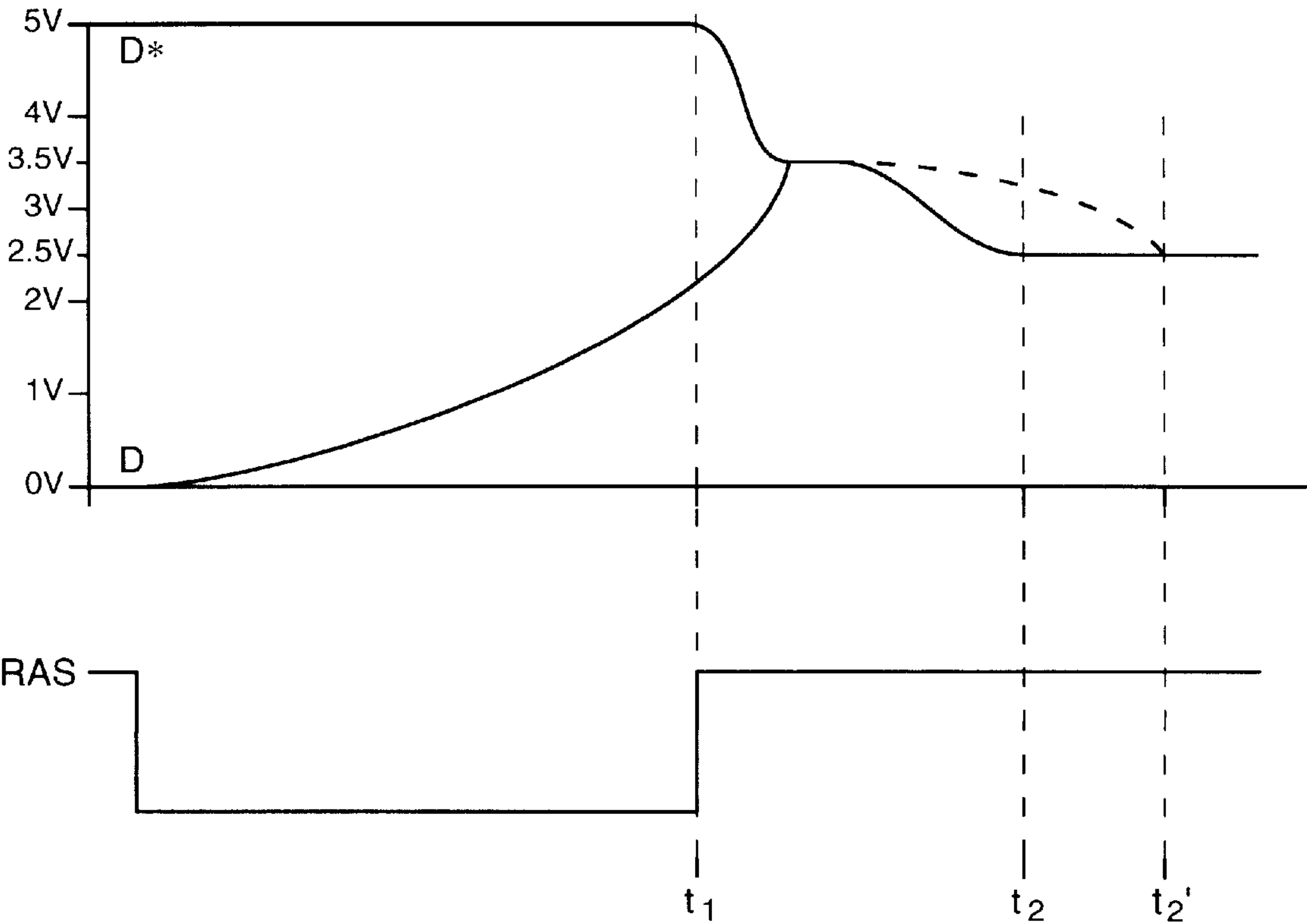
FIG. 8B
