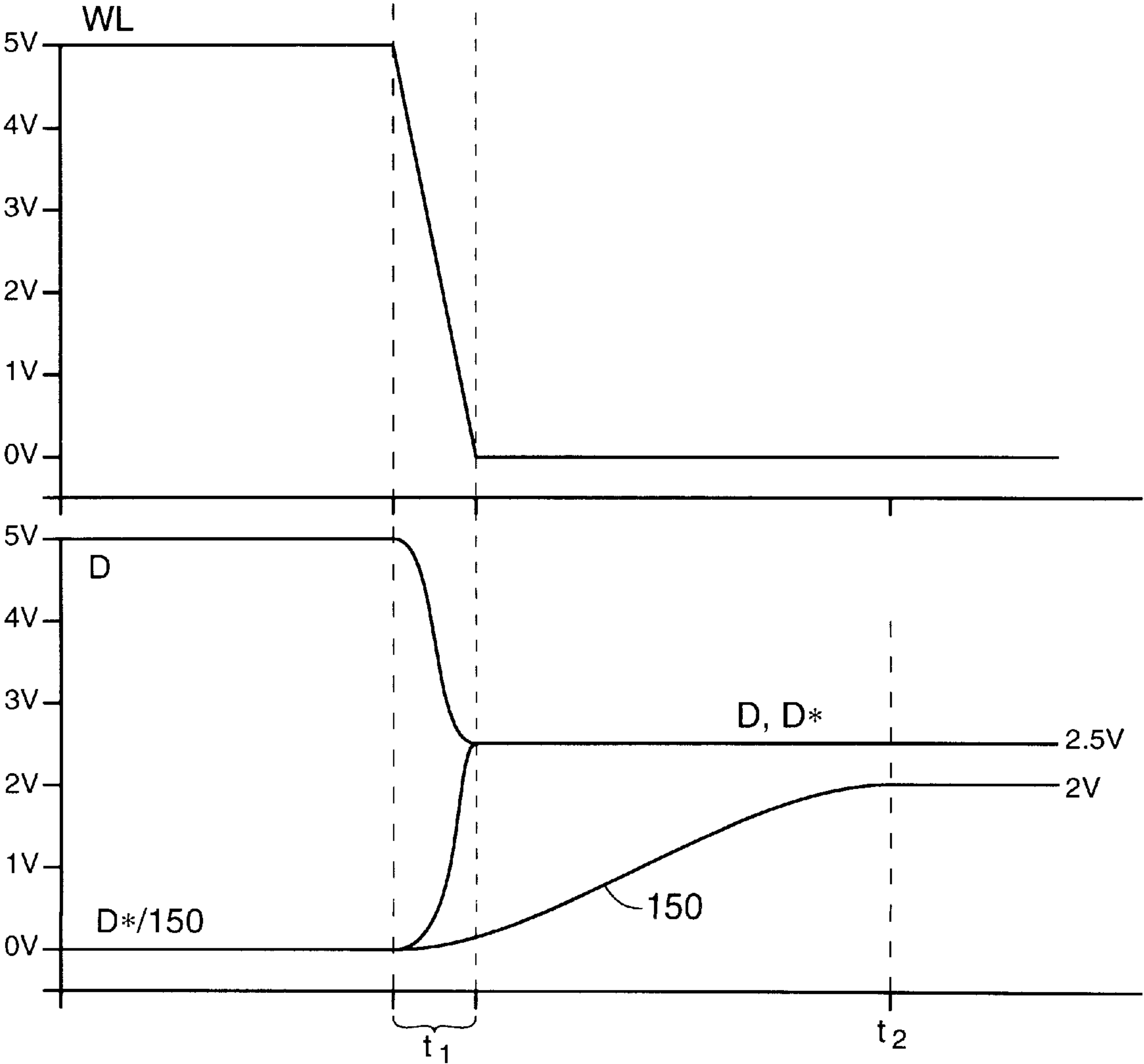
FIG. 9B
