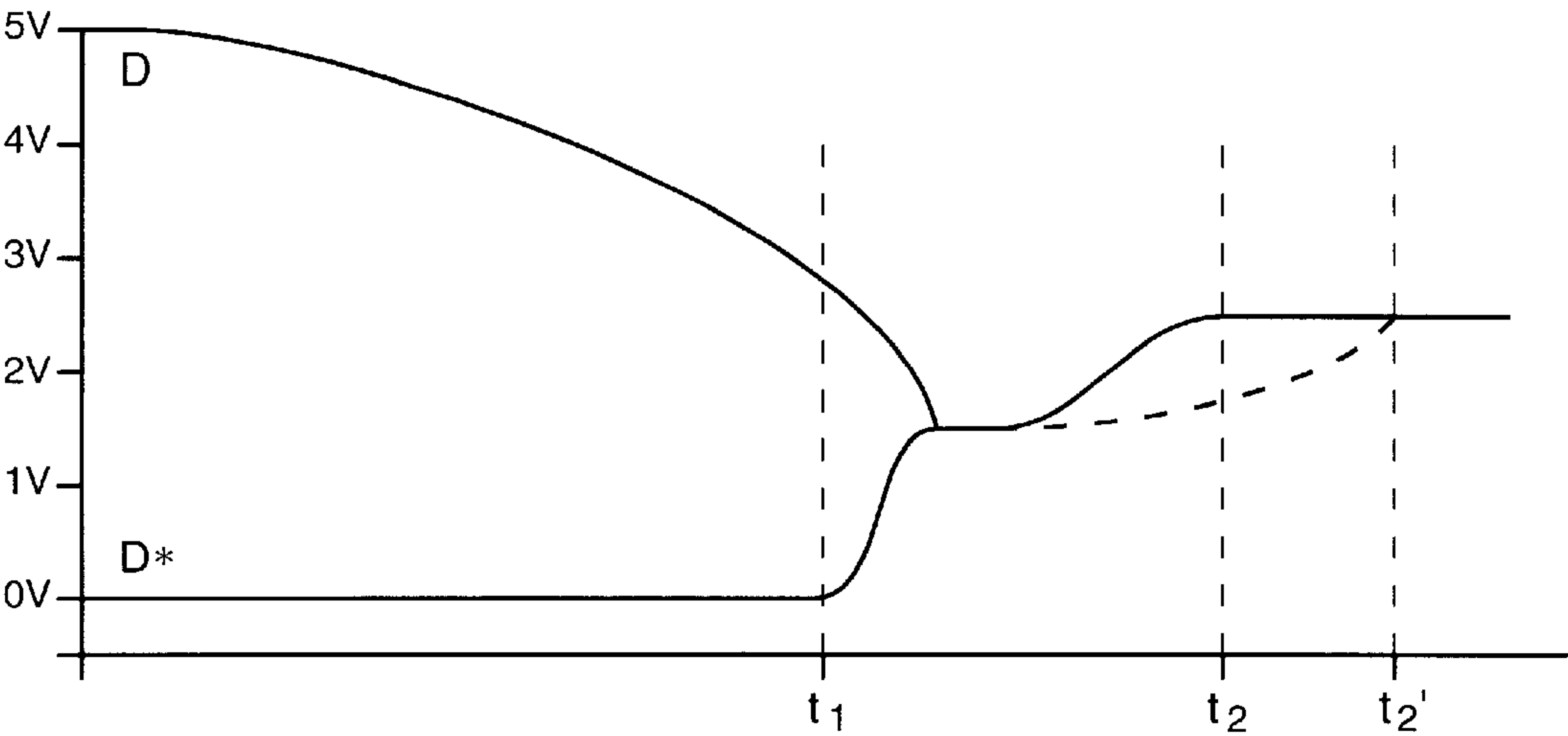
FIG. 8C
