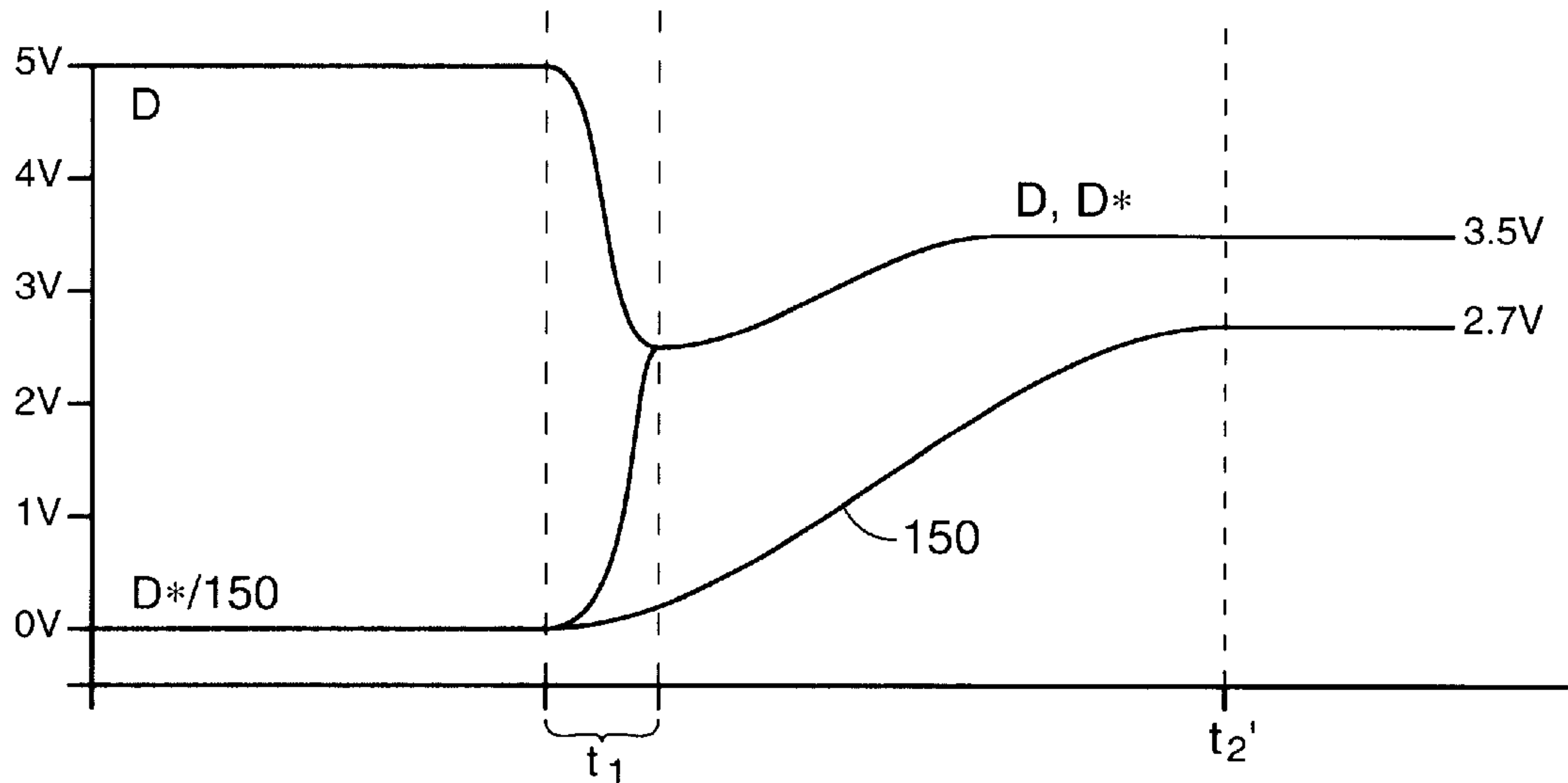
FIG. 9C
